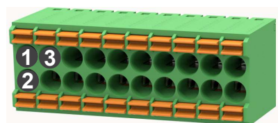
Figura 2.2: Pinagem do conector RS485 para o SCA700
