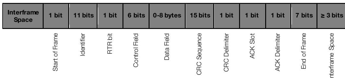
Figura 1.1: Frame de datos CAN
