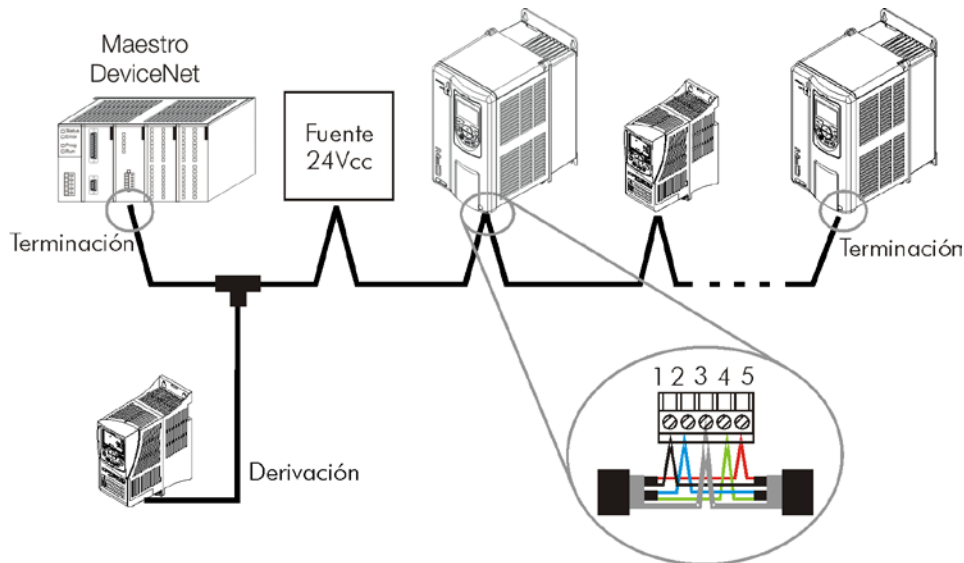
Figura 3.1: Ejemplo de instalación en red DeviceNet
