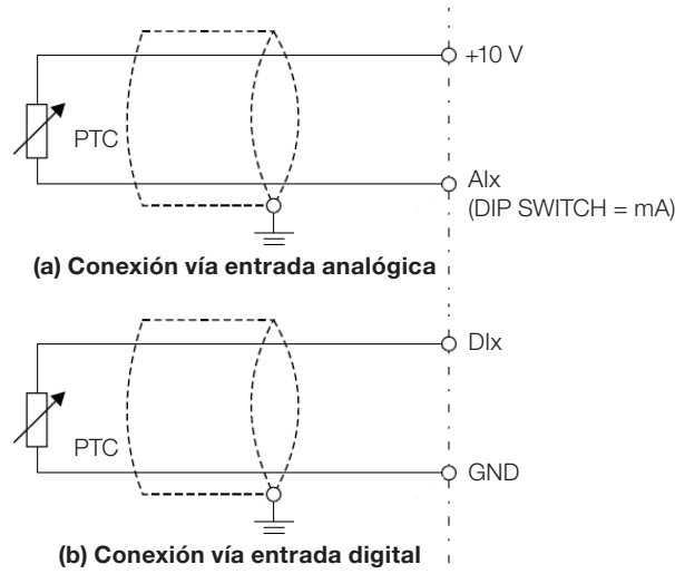
Figura 17.4: (a) y (b) Conexión del PTC al CFW500
