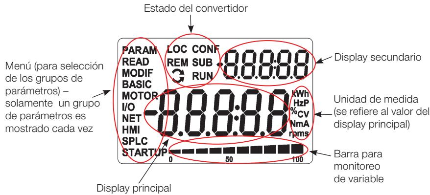
Figura 4.2: Áreas del display
