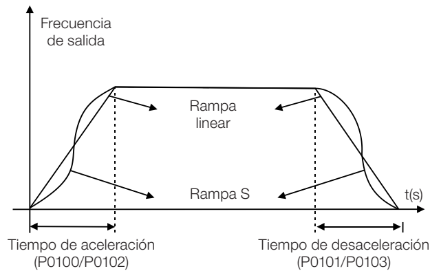
Figura 13.1: Rampa S o Linear
