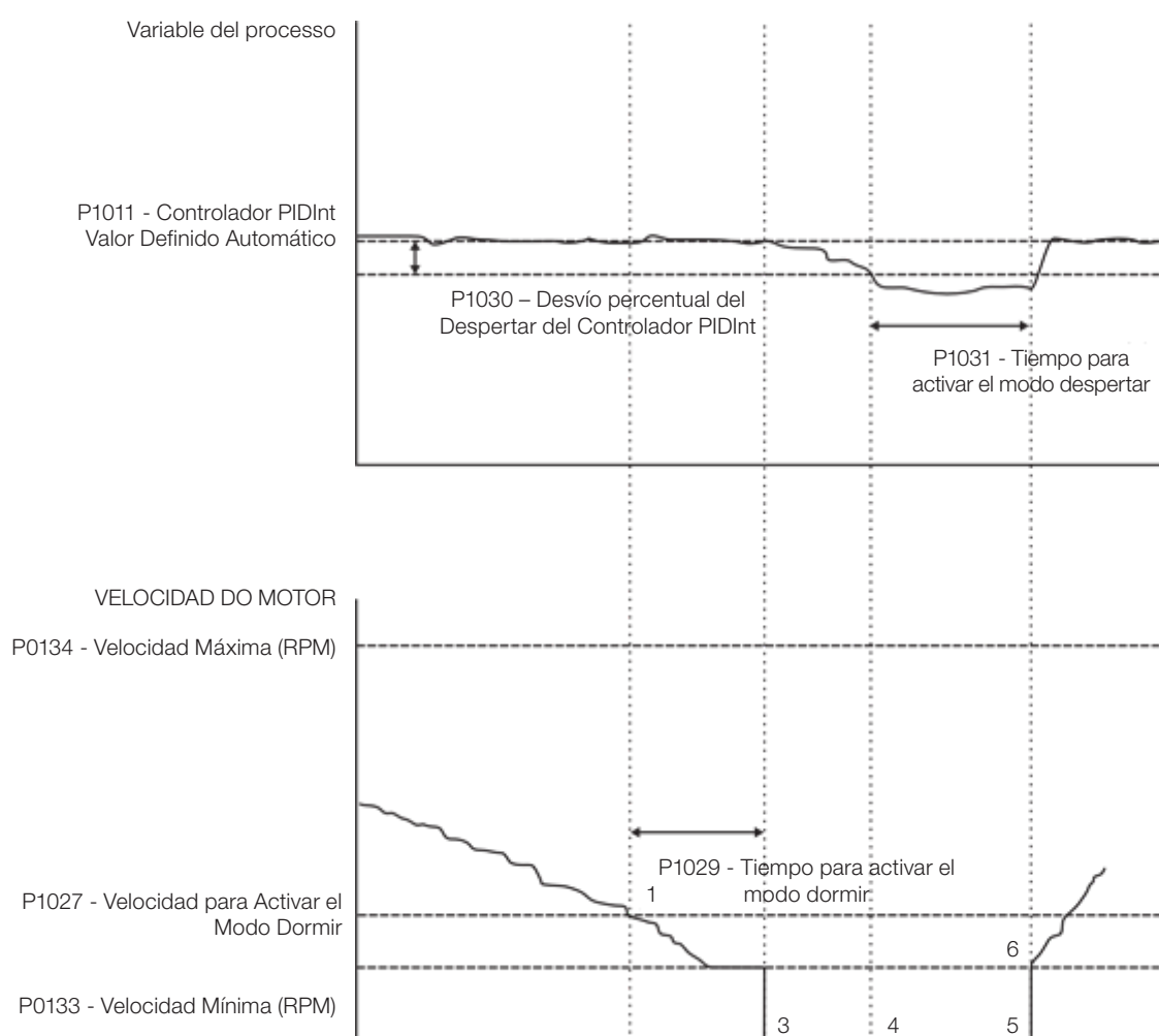
Figura 20.1: Esquema de funcionamiento para modo dormir y modo despertar
