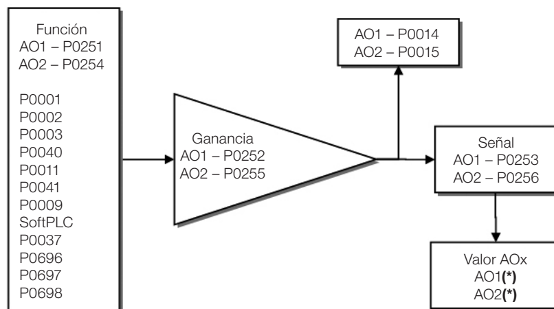
Figura 14.3: Diagrama de bloques de las salidas analógicas - AOx
