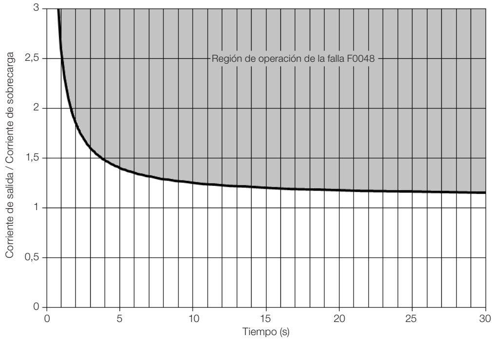
Figura 17.3: Actuación de la sobrecarga de los IGBTs (Normal Duty - ND)
