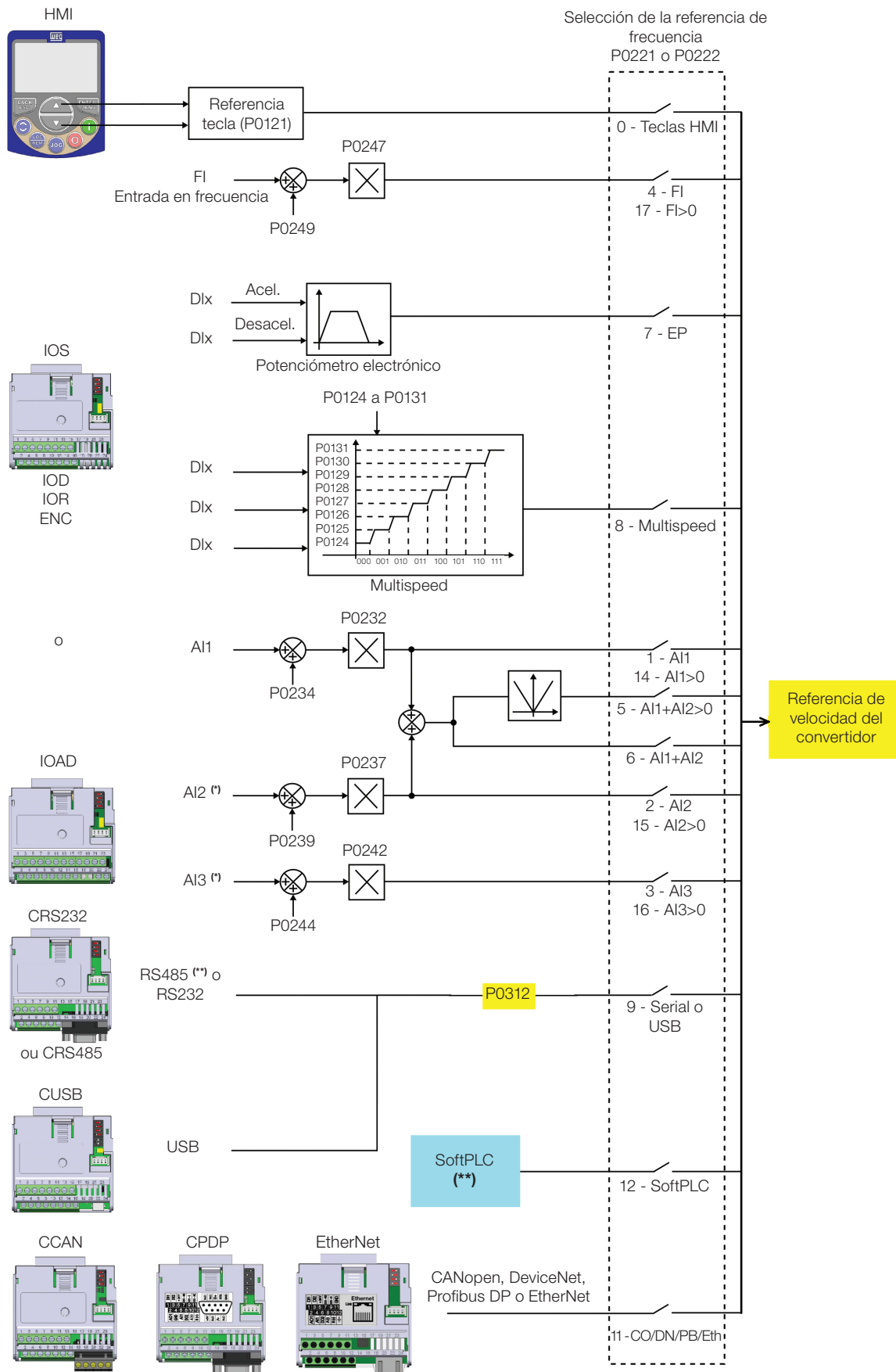
Figura 7.3: Estructura de selección de la referencia de velocidad
