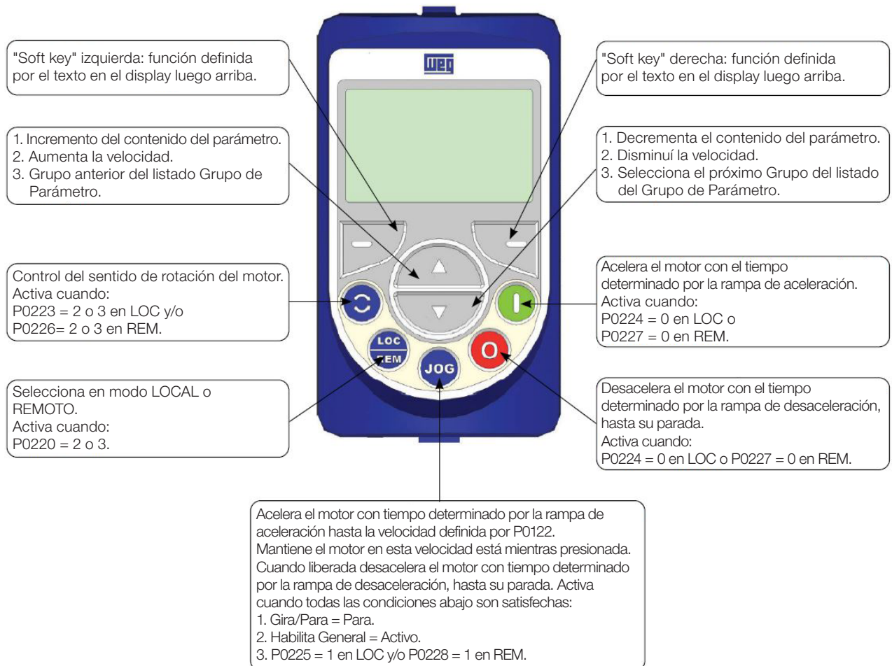
Figura 4.3: Teclas de la HMI
