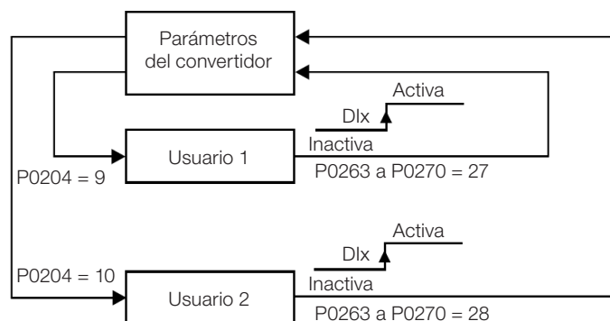
Figura 14.15: Diagrama de bloques de las funciones carga usuario 1 y usuario 2
