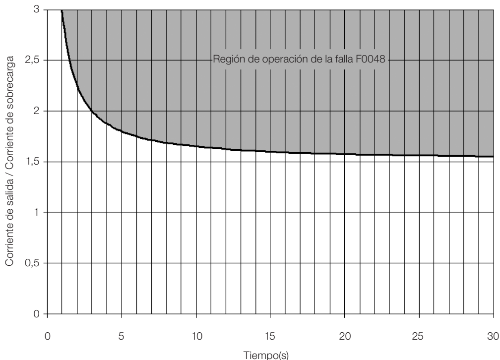
Figura 17.2: Actuación de la sobrecarga de los IGBTs (Heavy Duty - HD)
