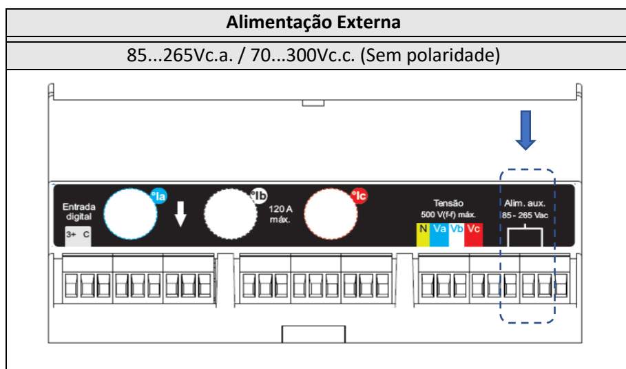
Figura 6 - Alimentação Externa
