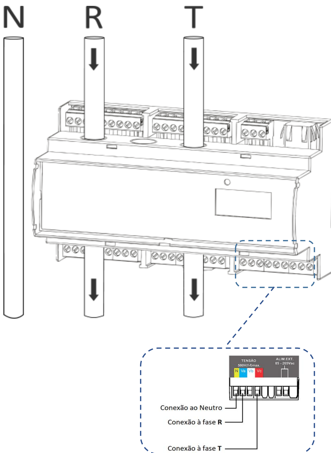
Figura 11 - TL01 Bifásico
