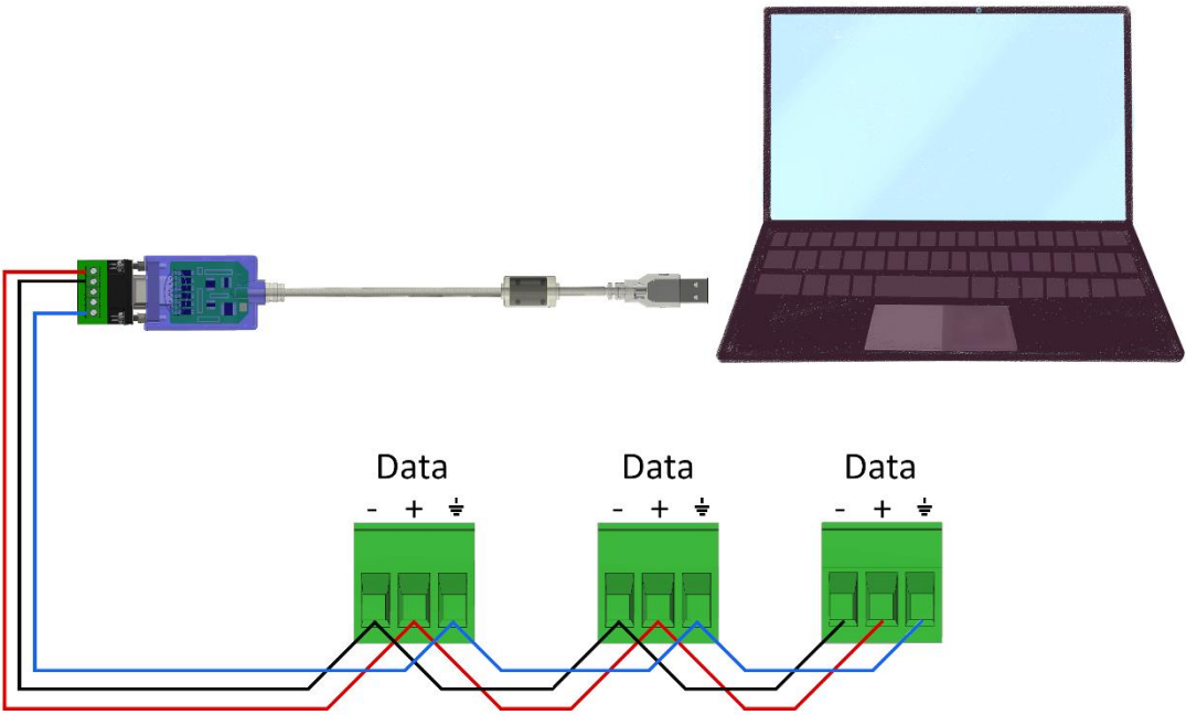
Figura 20 - Diagrama de Ligação
