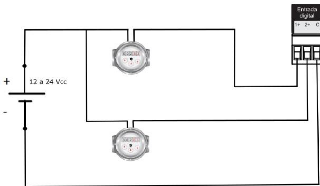
Figura 15 - Esquema de ligação Entrada Digital
