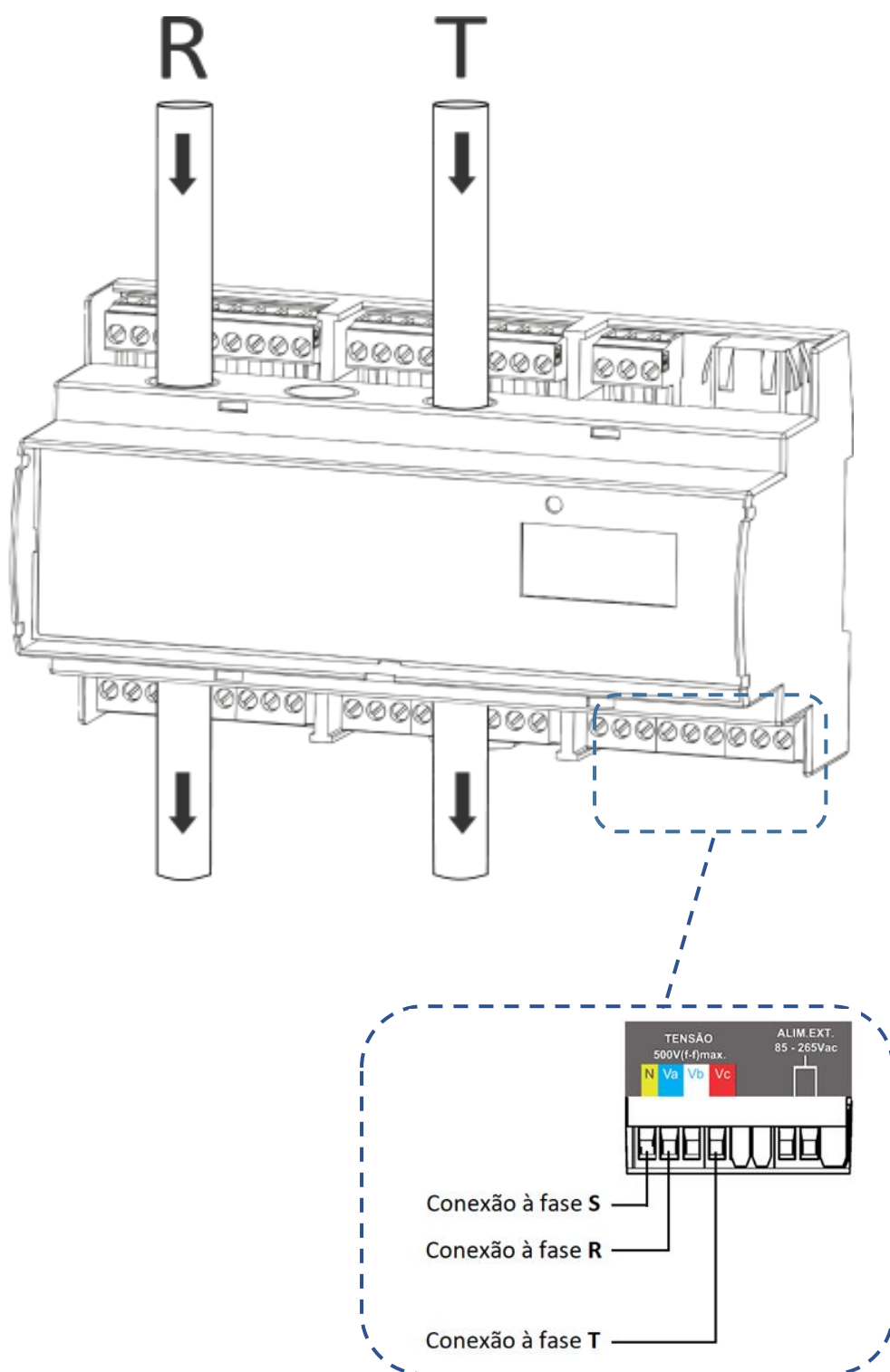
Figura 14 – TL17 Trifásico Delta
