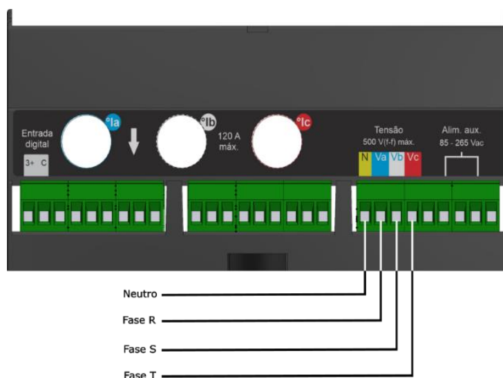
Figura 8 - Entrada de Tensão
