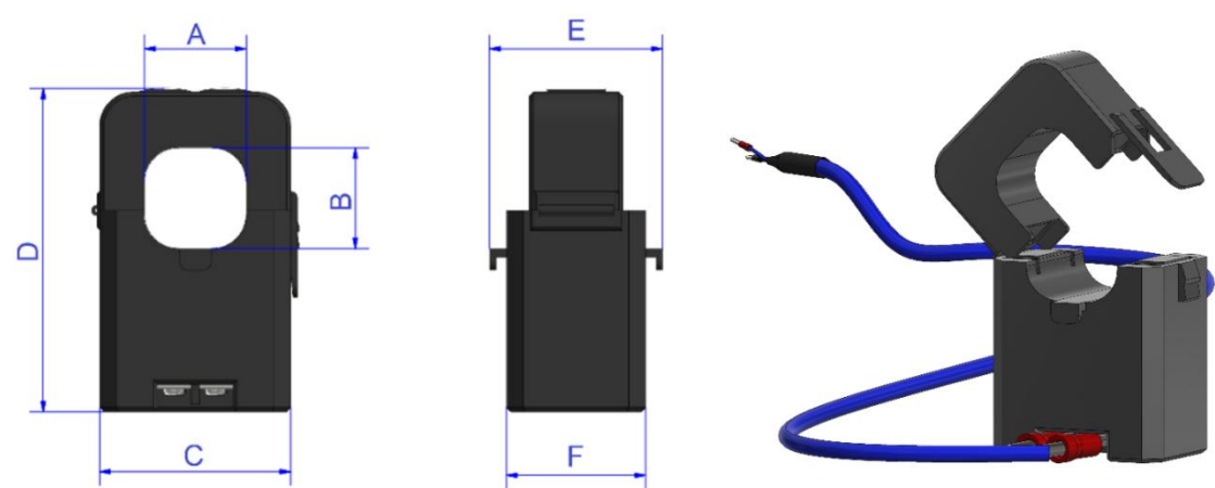
Figura 3 - Sensores Split Core
