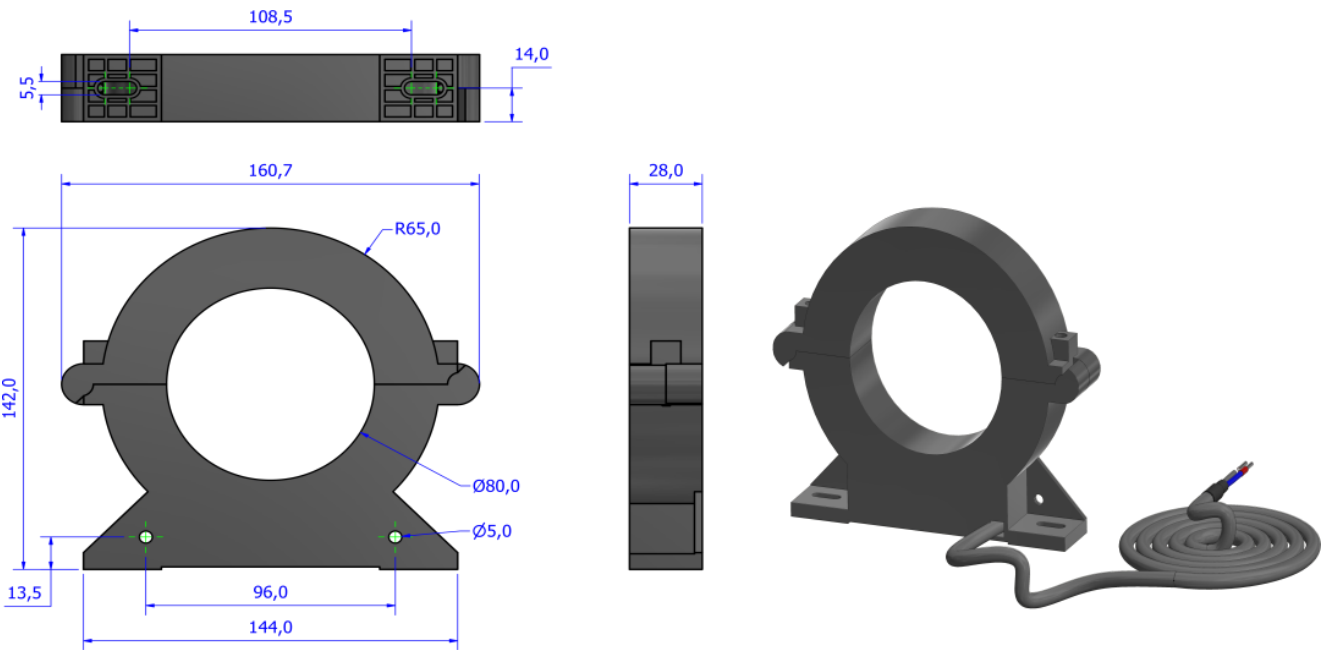
Figura 4 - Sensores Split Core de 1000 e 2000A
