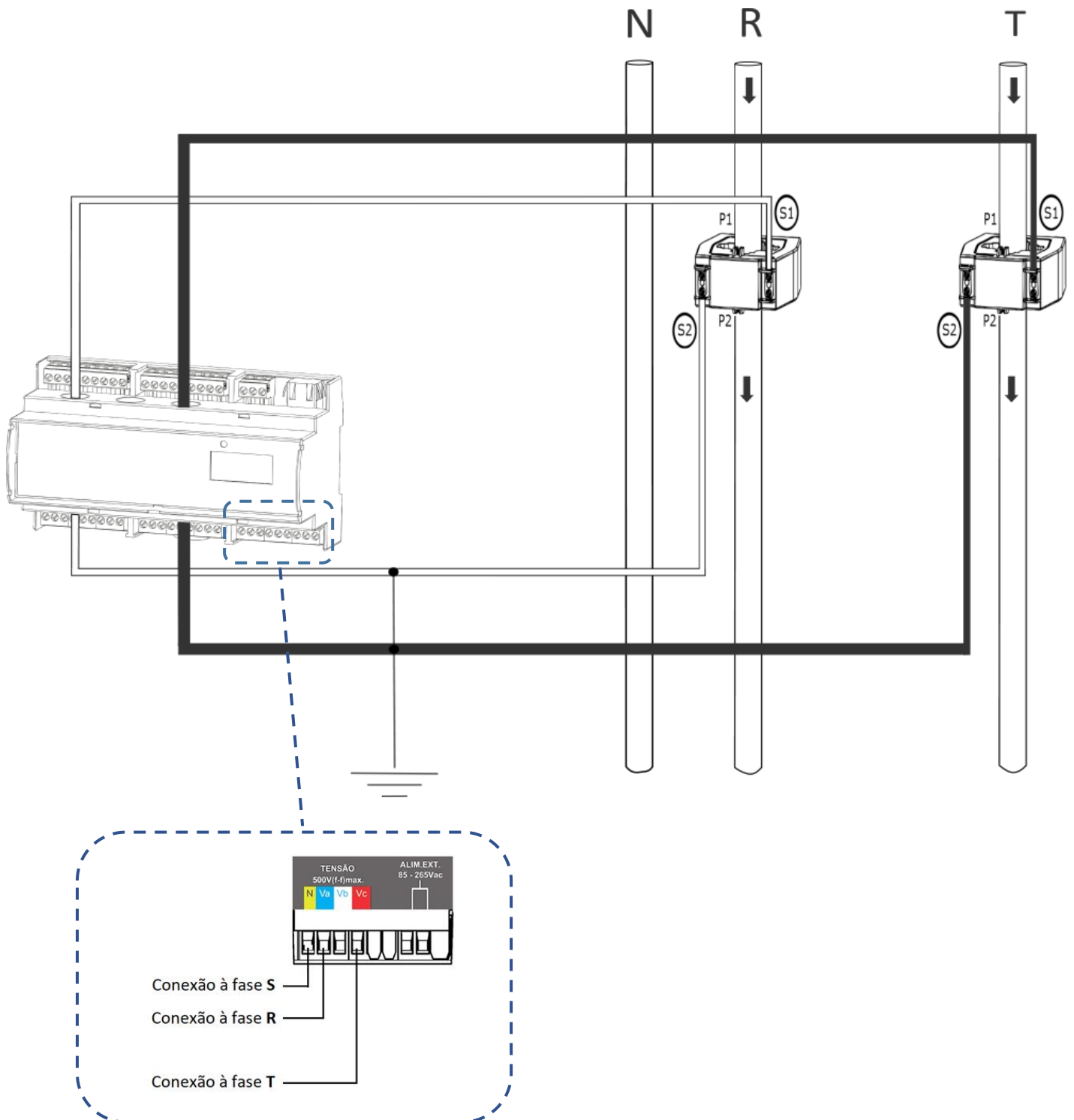
Figura 19 – TL17 Trifásico Delta
