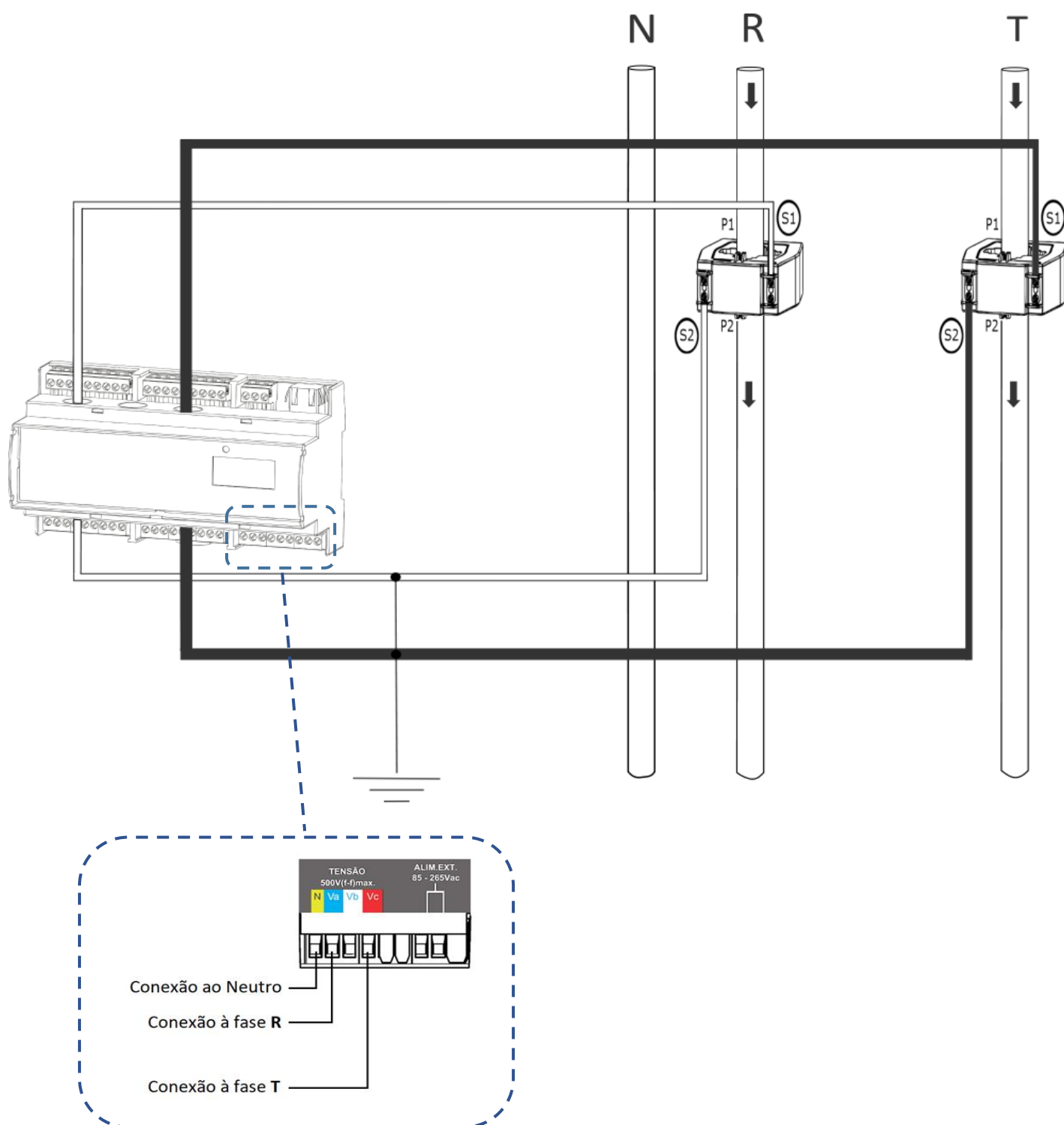
Figura 16 - TL01 Bifásico com TC
