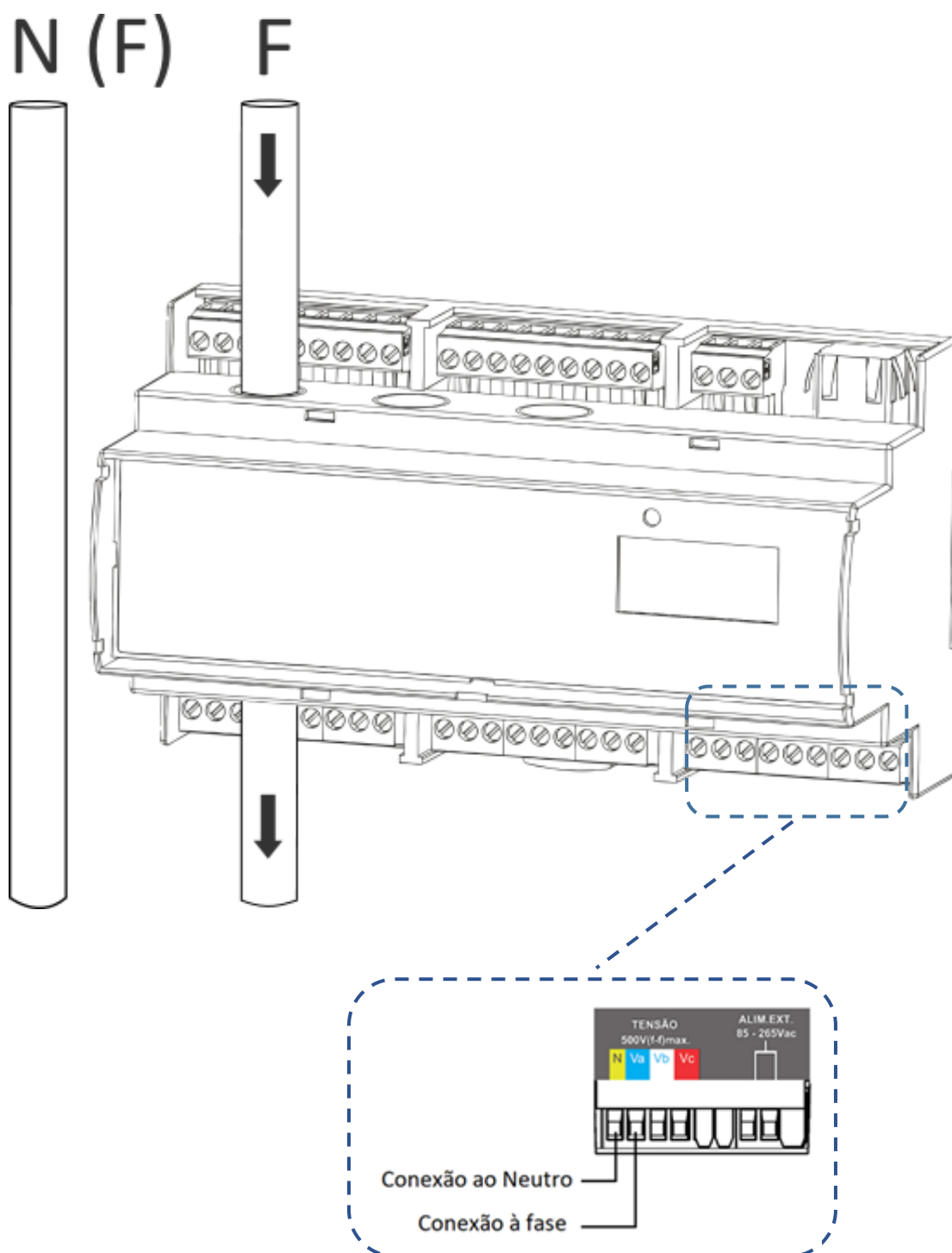
Figura 10 - TL02 Monofásico
