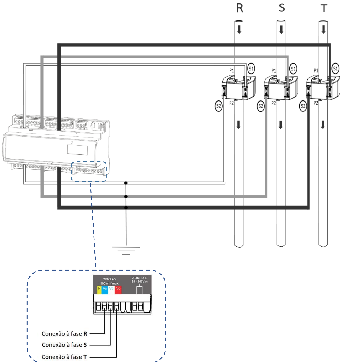
Figura 18 - TL48 Trifásico Delta com TC
