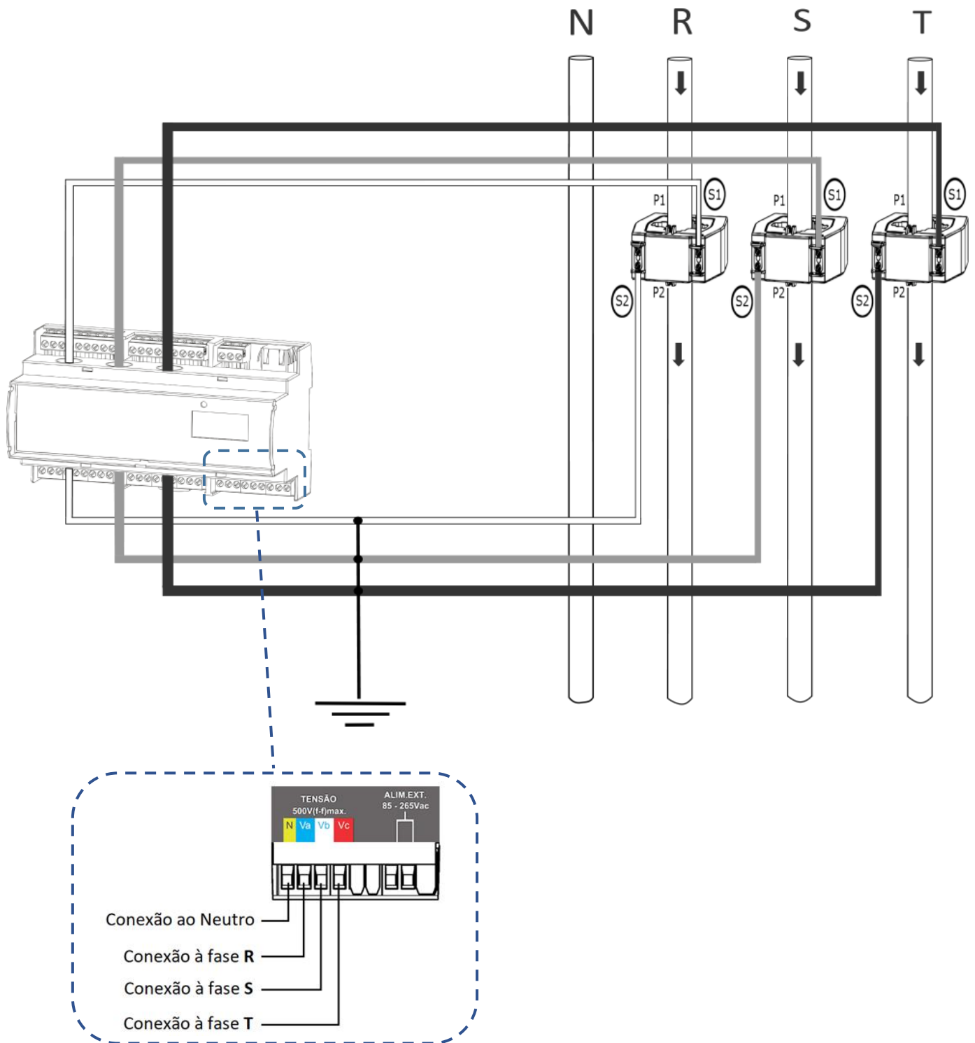
Figura 17 - TL00 Trifásico Estrela com TC
