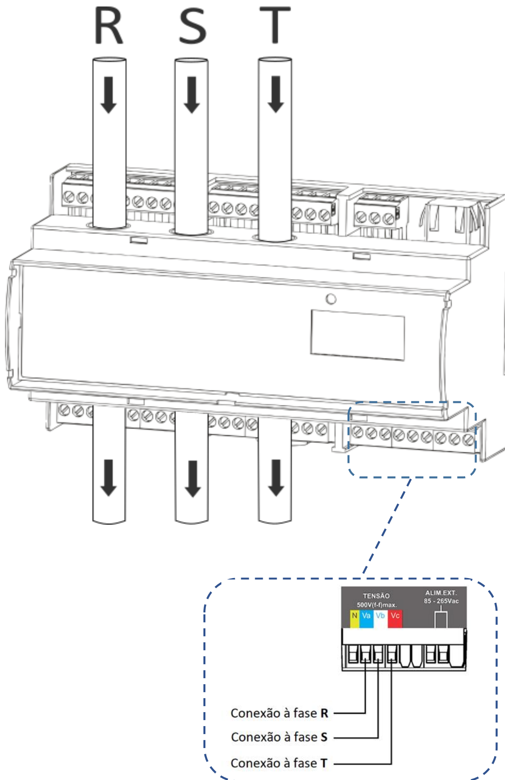
Figura 13 - TL48 Trifásico Delta
