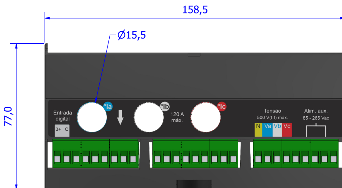
Figura 3 - Orifícios
