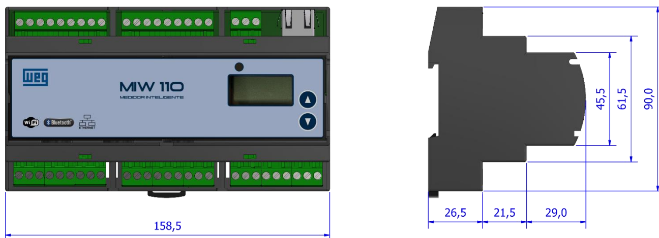
Figura 2 - Dimensionais
