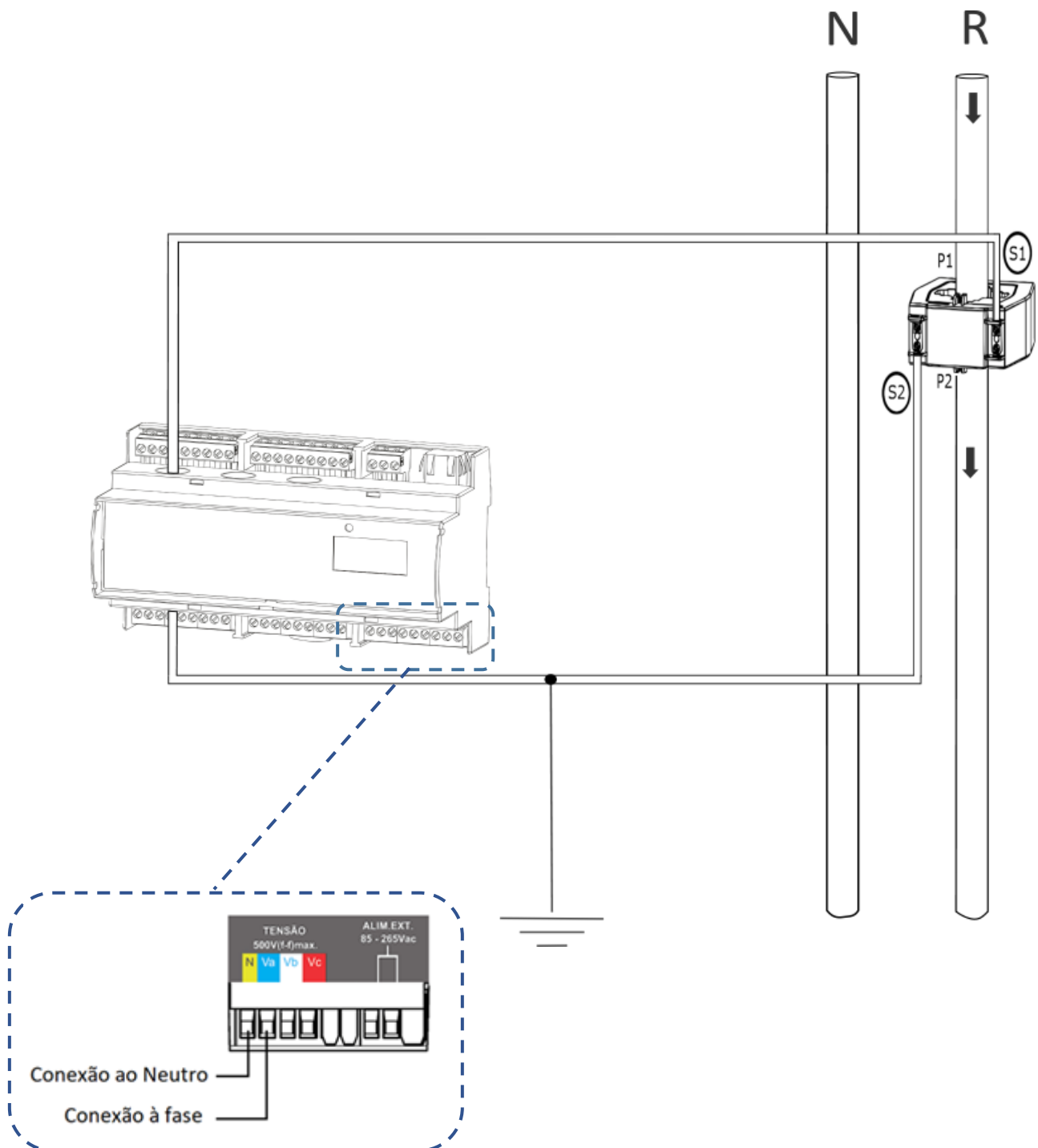
Figura 15 - TL02 Monofásico com TC
