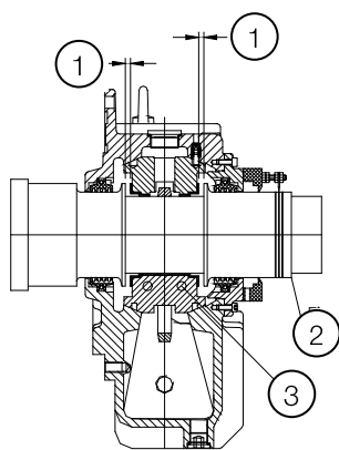
Figura 4.9: Mancal de deslizamento
