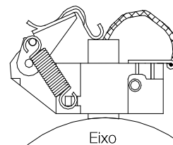
Figura 7.1: Escova para aterramento do eixo
