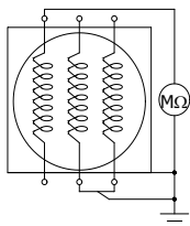
Figura 4.2: Conexão do megôhmetro em fases separadas
