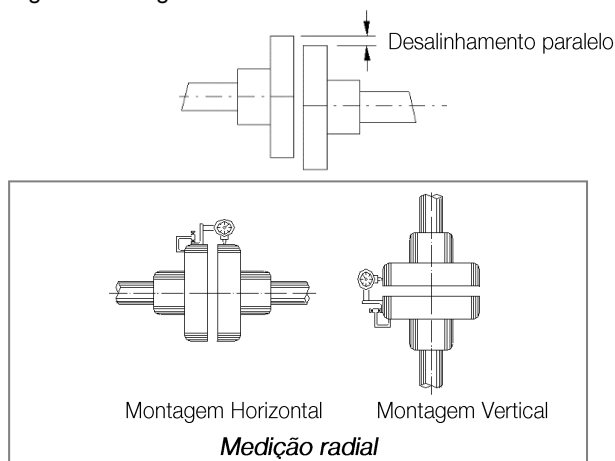
Figura 4.5: Alinhamento paralelo
