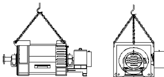
Figura 3.1: Manuseio dos geradores
