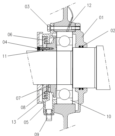
Figura 7.2: Partes do mancal de rolamento a graxa
