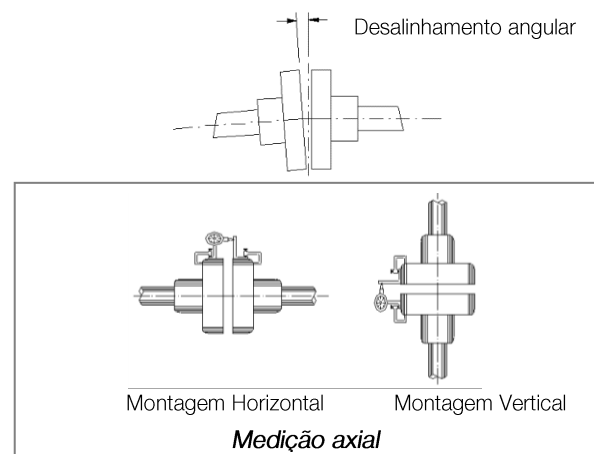
Figura 4.6: Alinhamento angular
