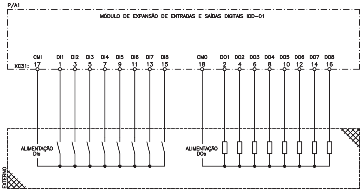
Figura 2.8: Ligação elétrica IOD-01
