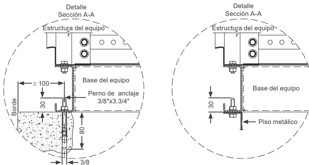
Figura 4.1: Detalles de fijación de los tableros en piso de concreto y en piso metálico
