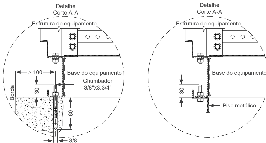
Figura 4.1: Detalhes de fixação dos painéis em piso de concreto e piso metálico
