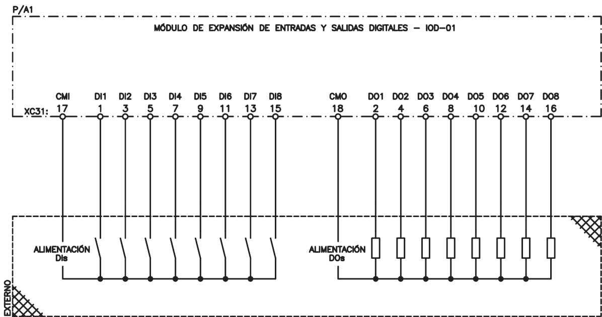
Figura 2.9: Conexión eléctrica IOD-01
