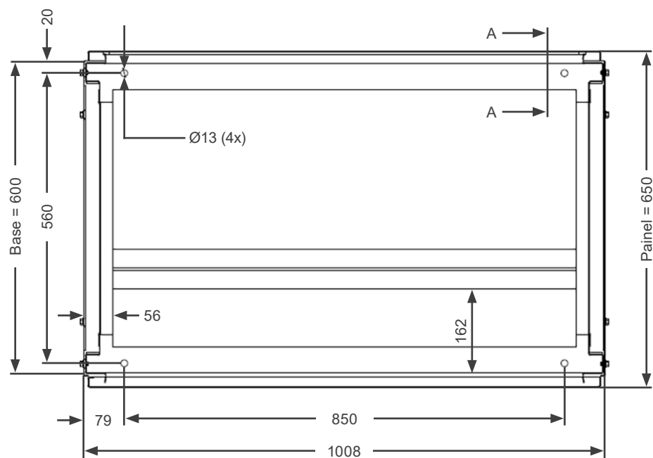
Figura 4.6: Detalhes de fixação AFW900C mecânica H
