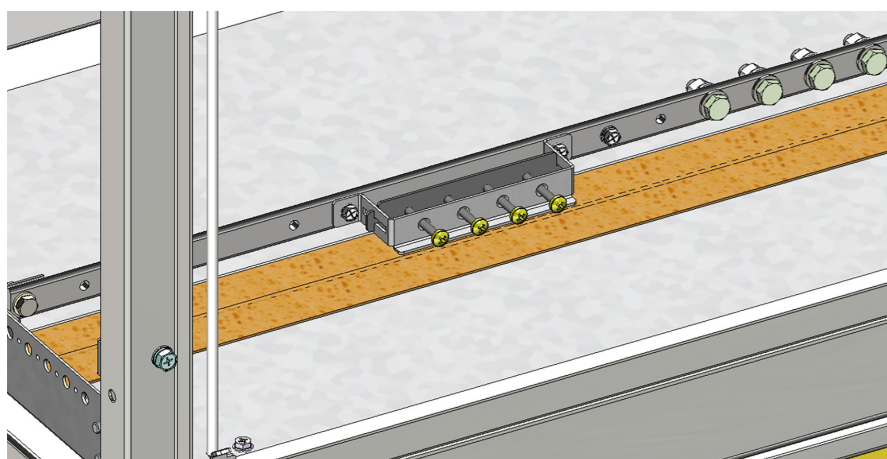
Figura 4.13: Detalhe mecânico para aterramento de cabos blindados
