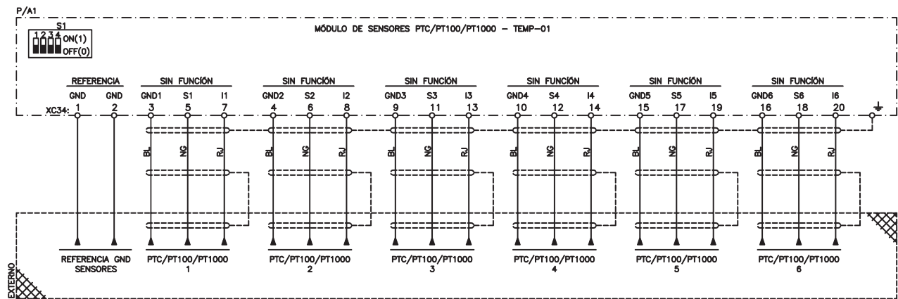
Figura 2.7: Conexión eléctrica TEMP-01
