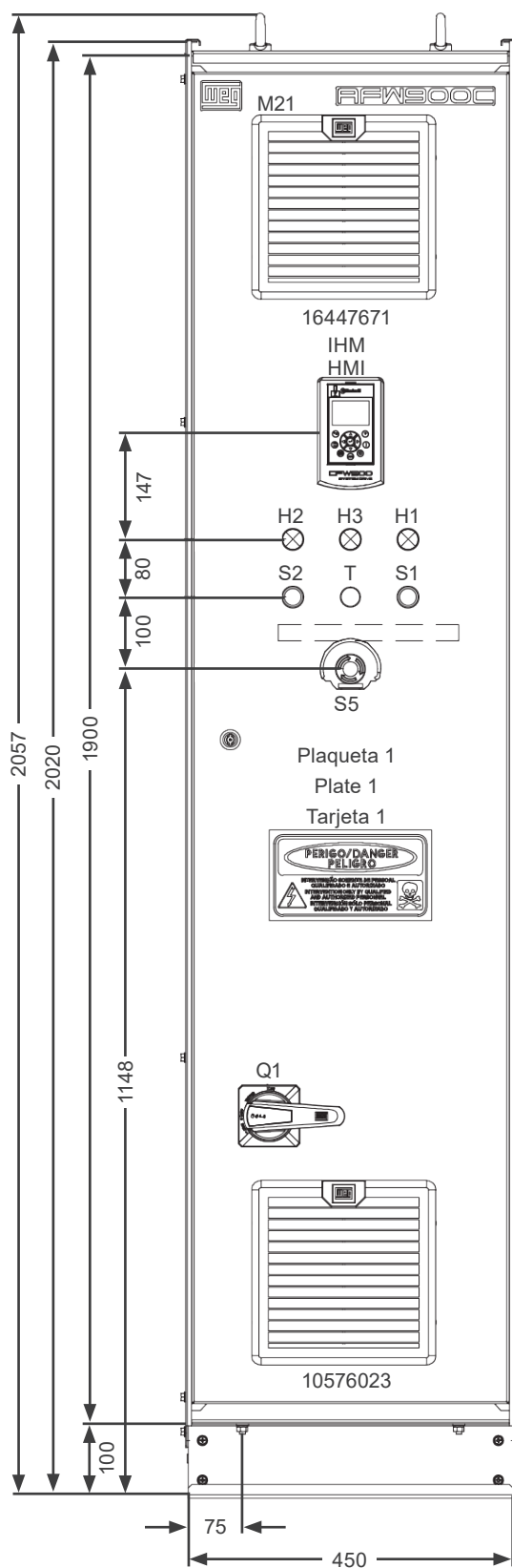
Figura 4.9: Detalles mecánicos de tamaño F
