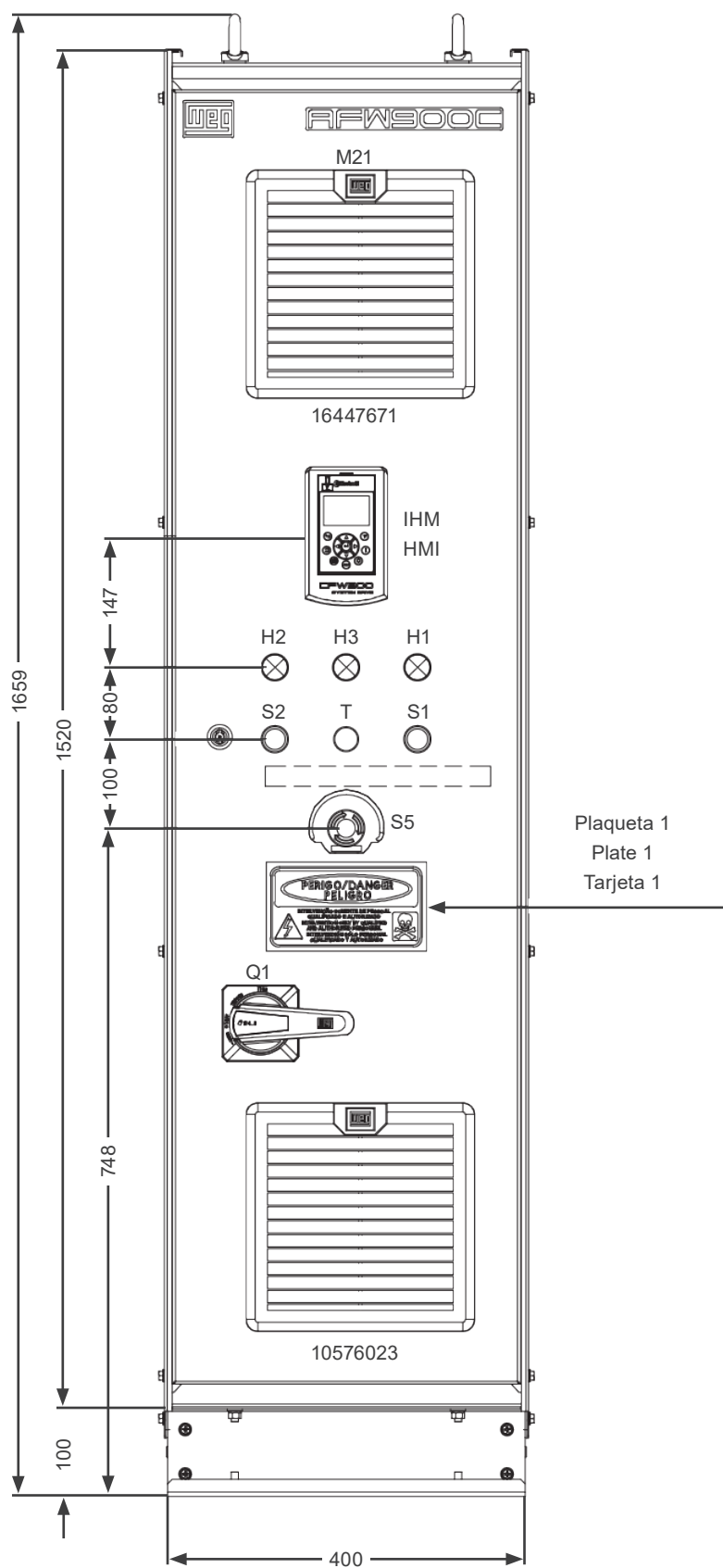
Figura 4.8: Detalles mecánicos de tamaño E
