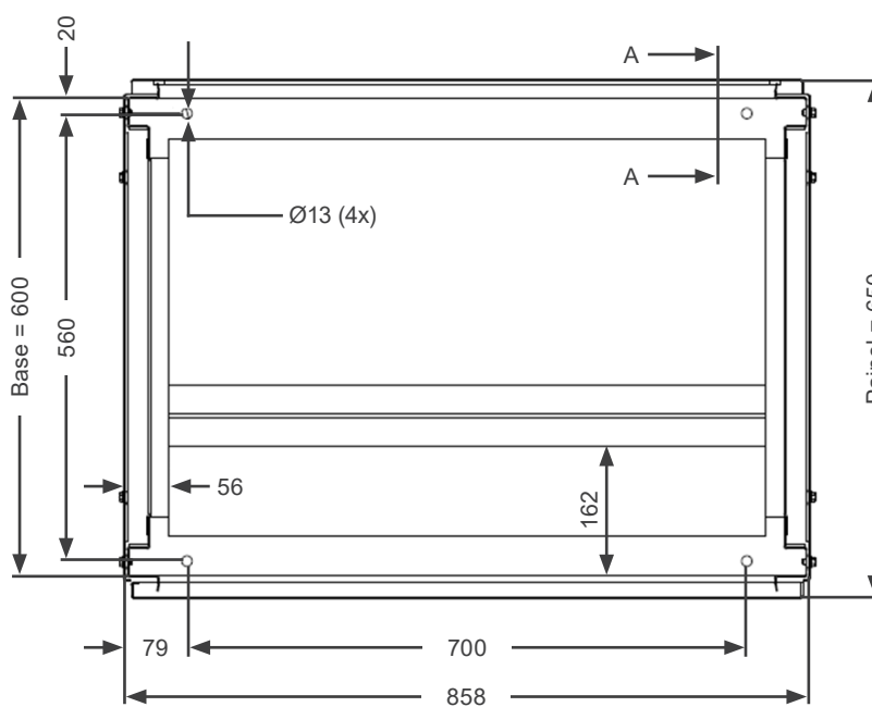
Figura 4.5: Detalles de fijación AFW900C tamaño G
