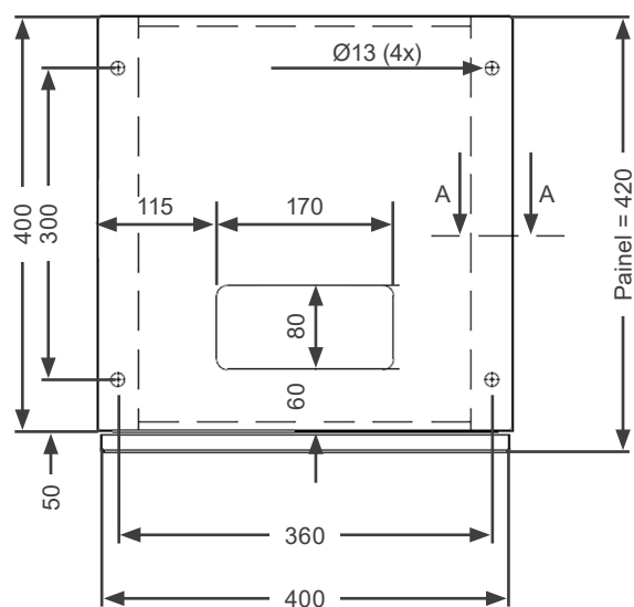
Figura 4.2: Detalles de fijación AFW900C tamaños C y D
