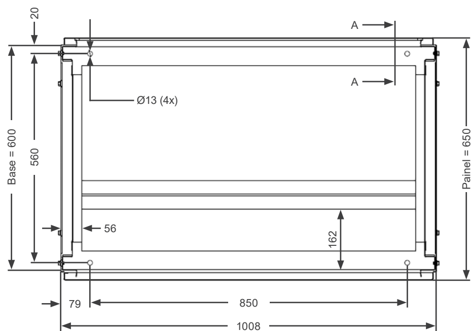
Figura 4.6: Detalles de fijación AFW900C tamaño H
