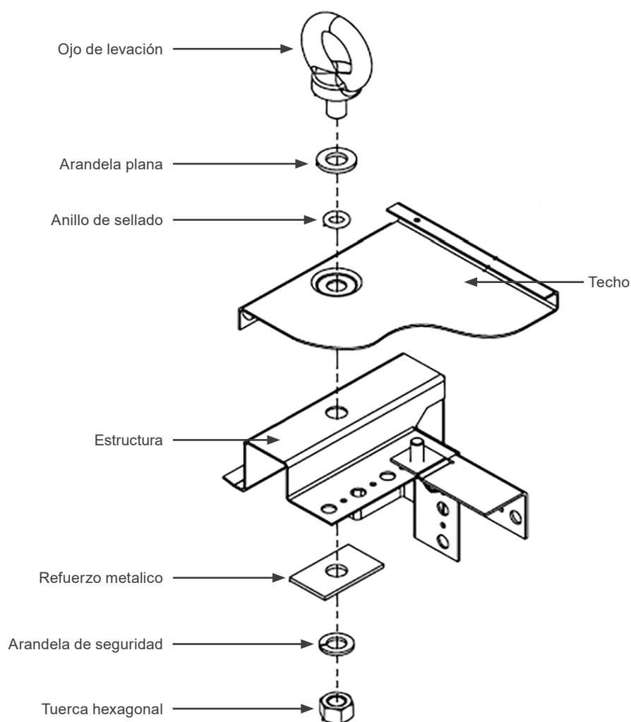
Figura 1.12: Ojal de izamiento con detalle de explosión
