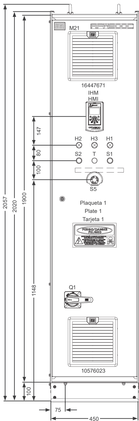
Figura 4.9: Detalhes mecânicos da mecânica F
