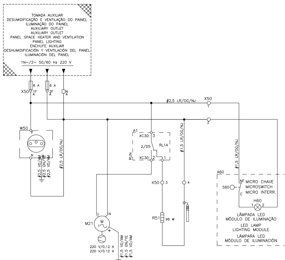
Figura 4.12: Detalhe elétrico do circuito auxiliar
