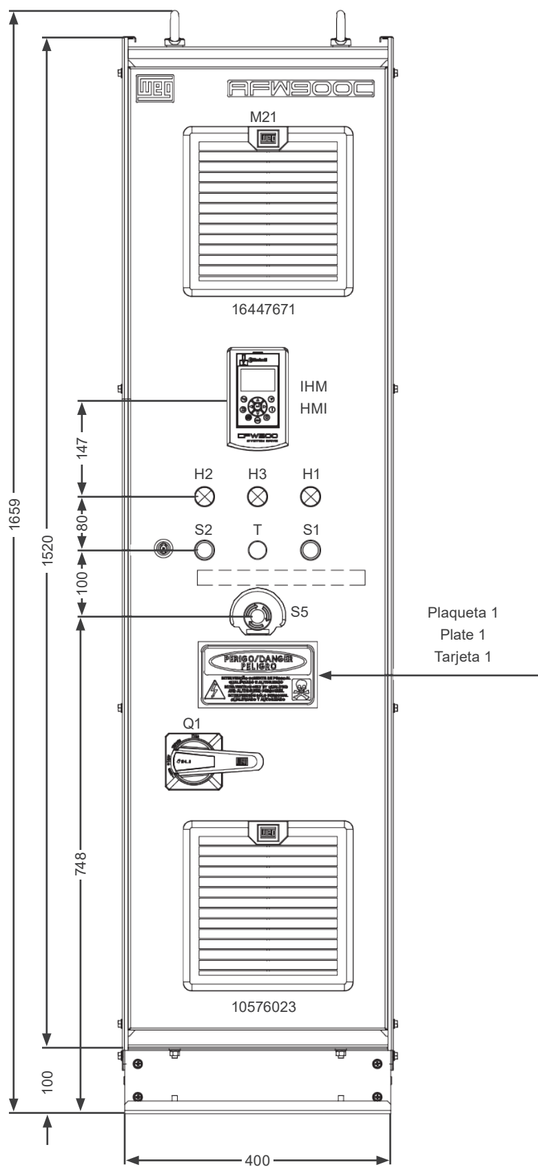
Figura 4.8: Detalhes mecânicos da mecânica E
