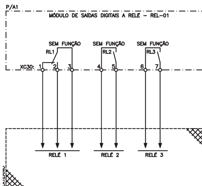
Figura 2.3: Ligação elétrica REL-01
