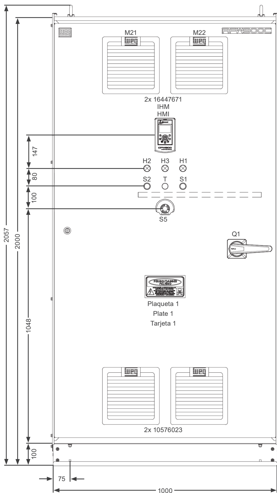
Figura 4.11: Detalhes mecânicos da mecânica H
