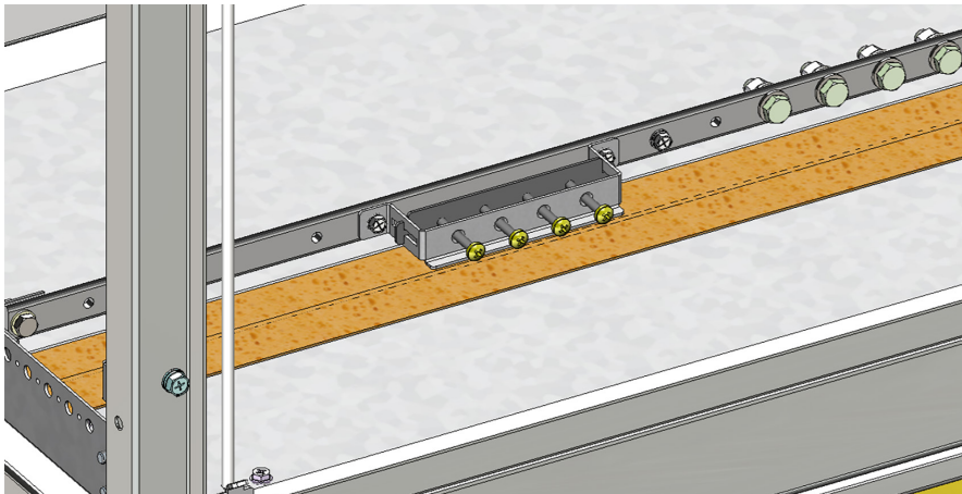
Figura 4.13: Detalle mecánico para la puesta a tierra de cables blindados
