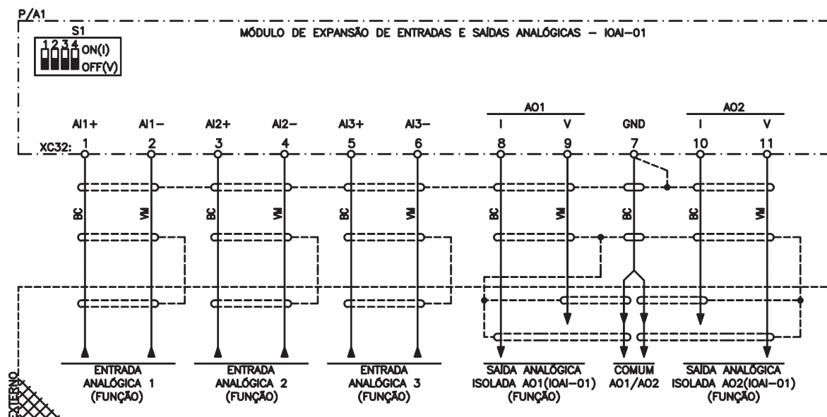
Figura 2.5: Ligação elétrica IOAI-01
