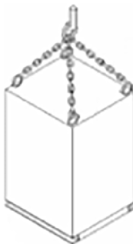
Figura 1.11: Içamento individual quatro (4) pontos
