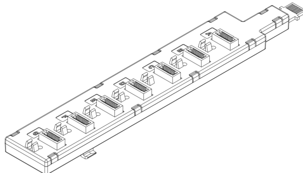
Figura 2.11: Módulo 7Slots
