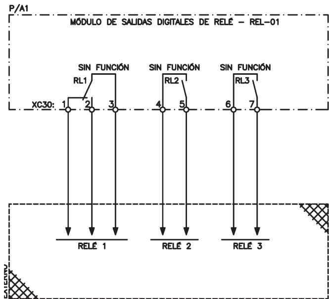
Figura 2.3: Conexión eléctrica REL-01
