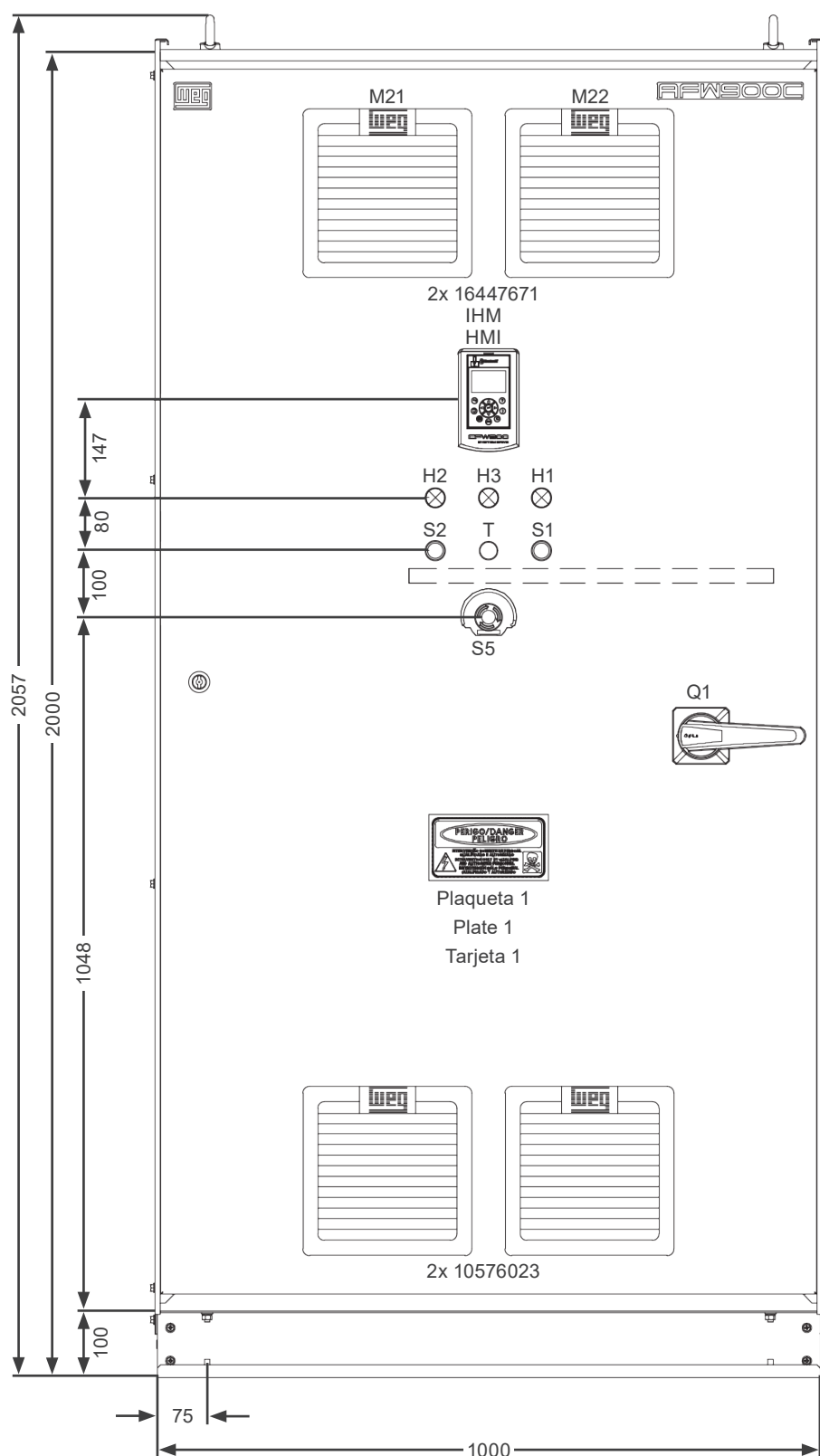
Figura 4.11: Detalles mecánicos de tamaño H
