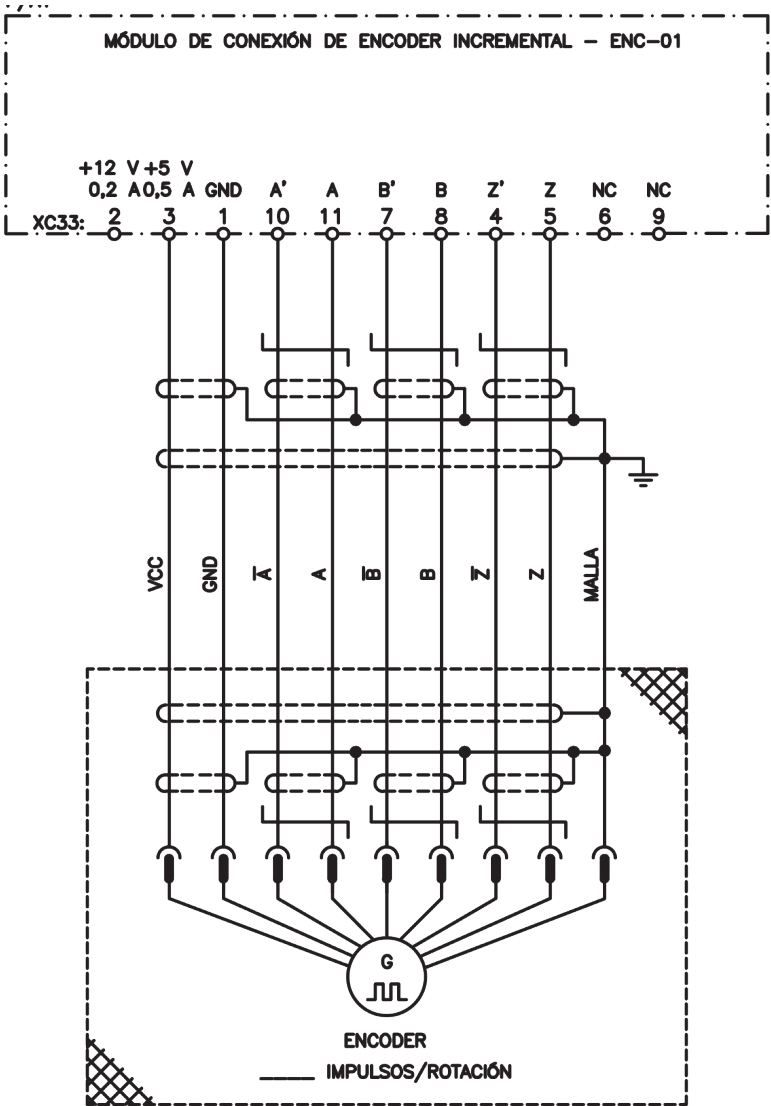
Figura 2.11: ENC-01 Conexión eléctrica
