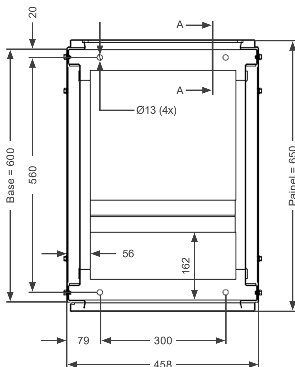
Figura 4.4: Detalhes de fixação AFW900C mecânica F
