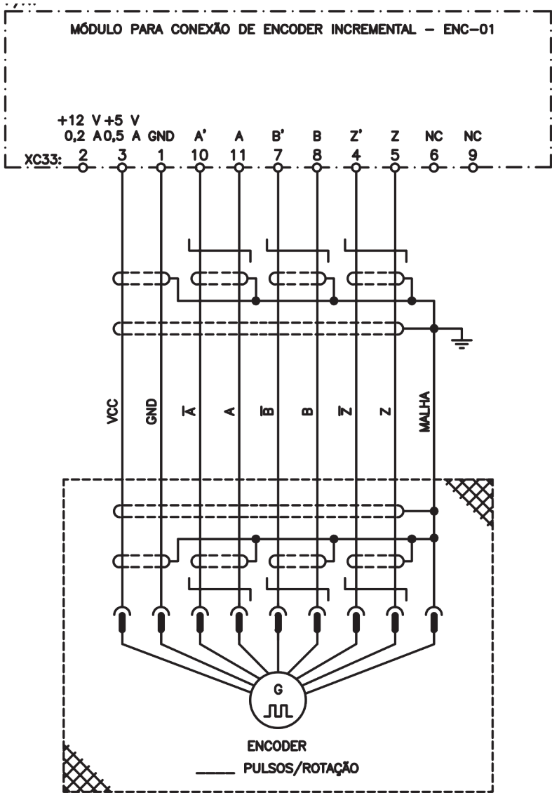
Figura 2.10: Ligação elétrica ENC-01
