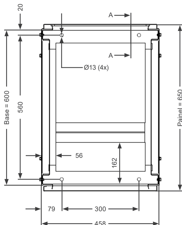
Figura 4.4: Detalles de fijación AFW900C tamaño F
