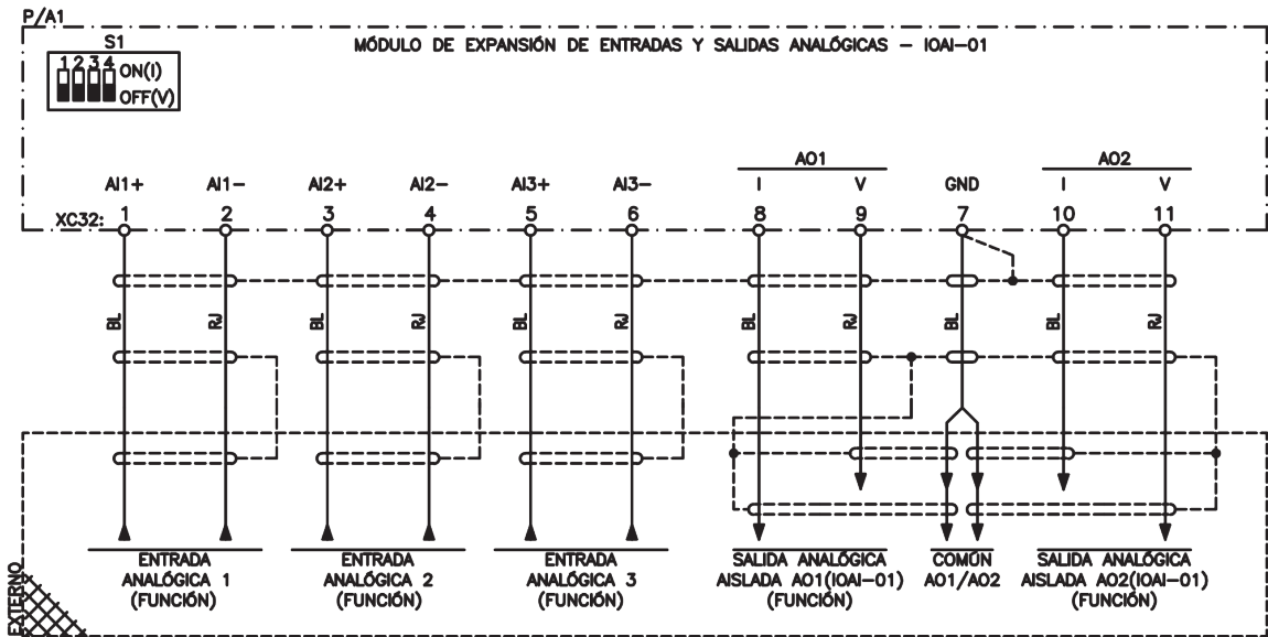
Figura 2.5: Conexión eléctrica IOAI-01
