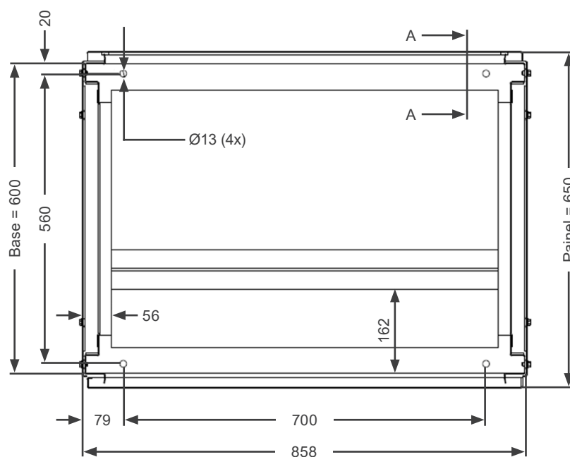
Figura 4.5: Detalhes de fixação AFW900C mecânica G
