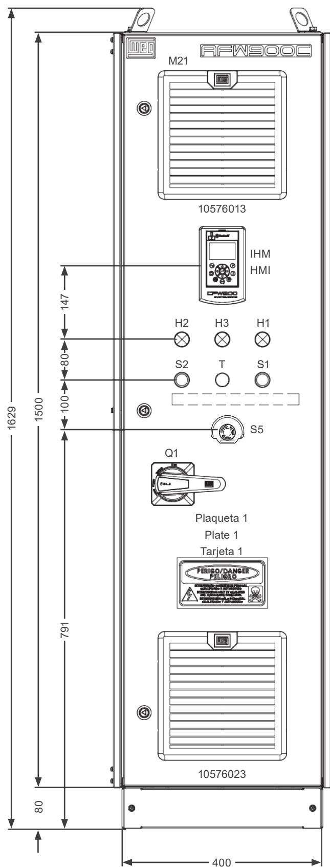
Figura 4.7: Detalhes mecânicos da mecânica C e D
