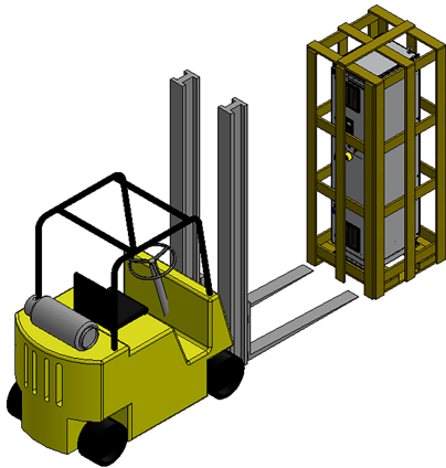
Figura 1.6: Carretilla elevadora de horquilla
