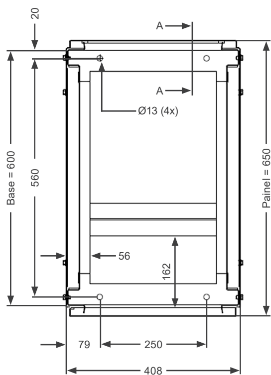
Figura 4.3: Detalles de fijación AFW900C tamaño E
