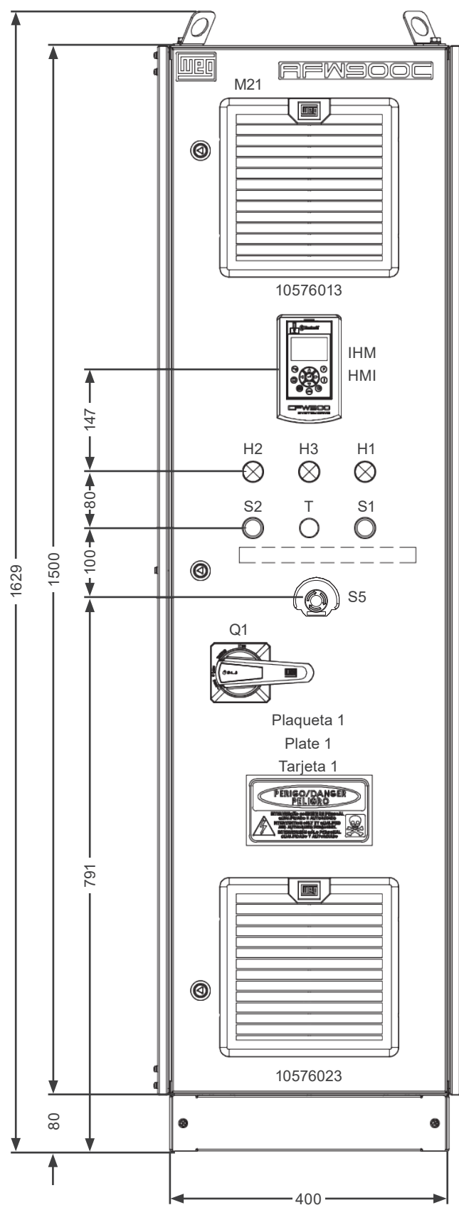
Figura 4.7: Detalles mecánicos de tamaños C y D
