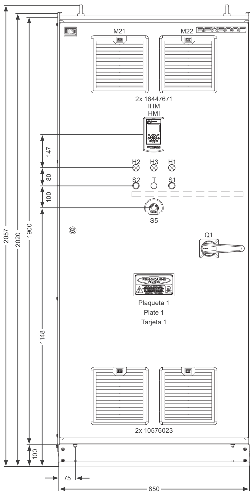
Figura 4.10: Detalhes mecânicos da mecânica G
