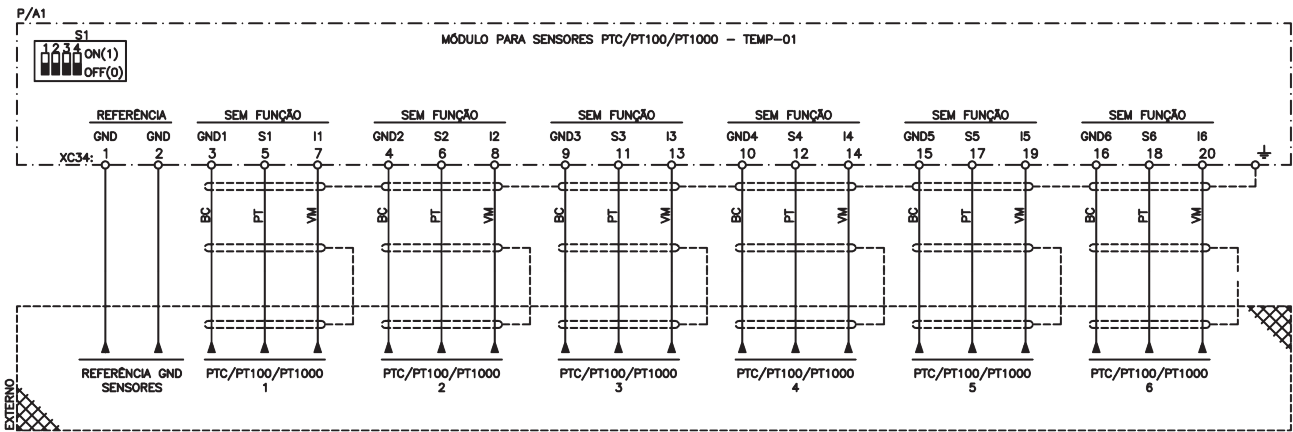
Figura 2.6: Ligação elétrica TEMP-01
