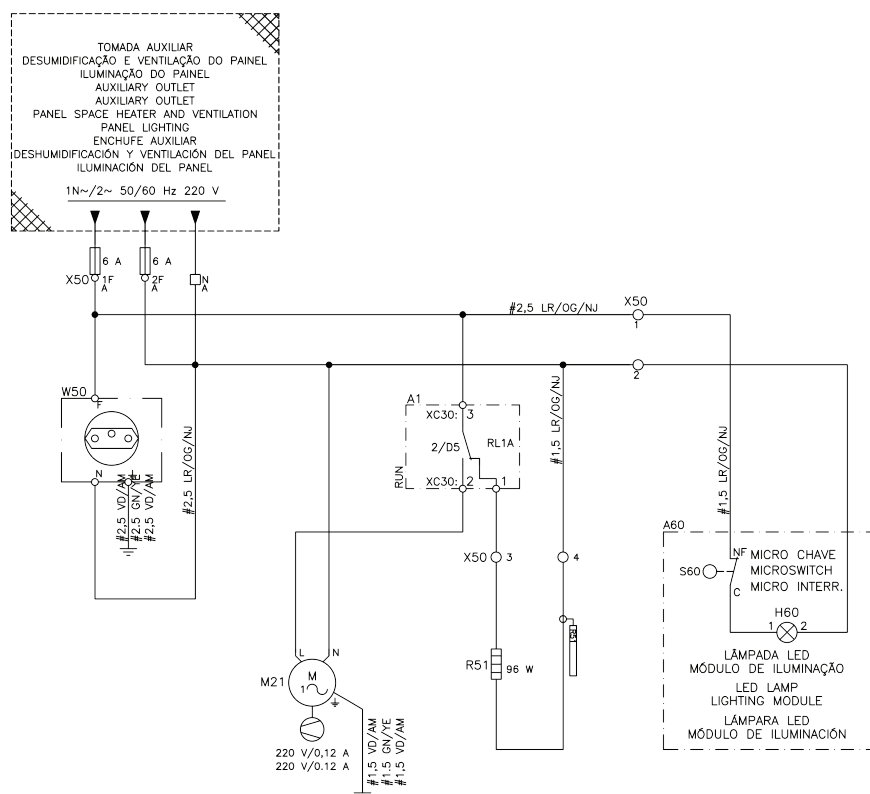
Figura 4.12: Detalle eléctrico del circuito auxiliar
