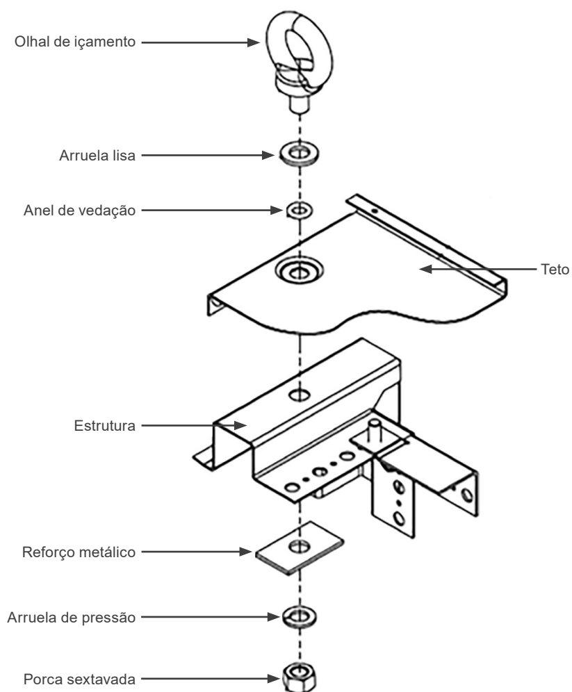
Figura 1.12: Detalhe explodido olhal de içamento
