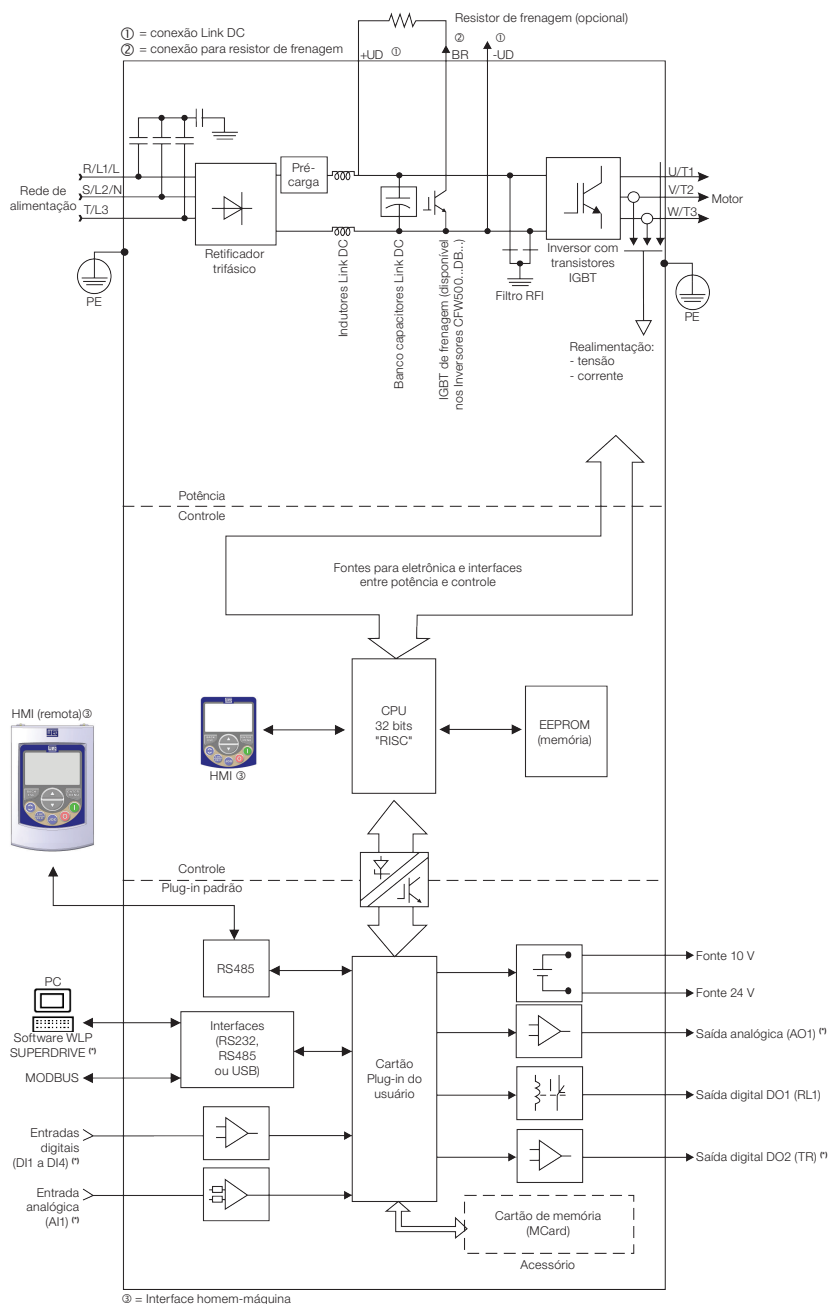
Figura 2.3: Blocodíagrama do CFW500 para mecânicas F e G
