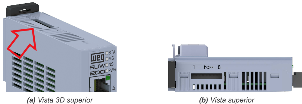
Figura 3.1: Chaves DIP.
