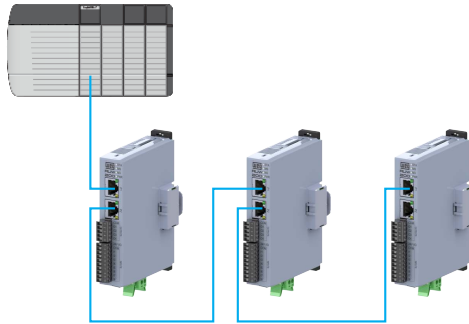
Figura 3.3: Topologia daisy chain
