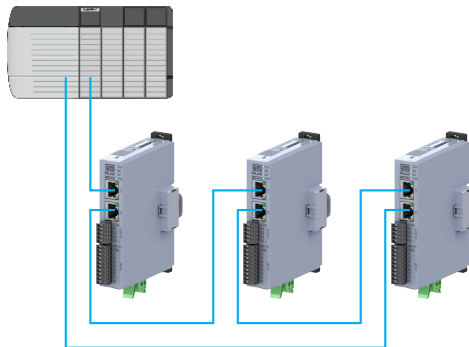
Figura 3.4: Topologia anel
