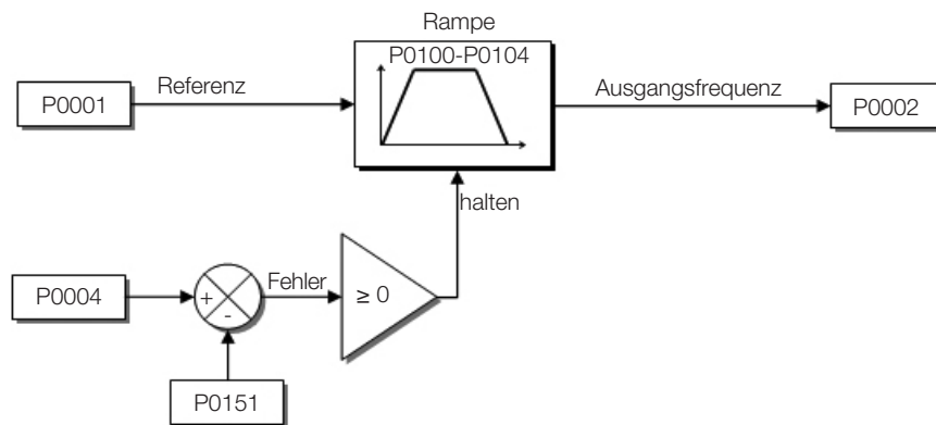
Abbildung 9.5: Blockdiagramm Zwischenkreisspannungsbegrenzung – Rampenstopp
