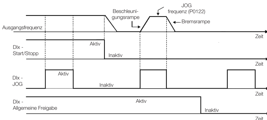
Abbildung 15.12: Beispiel der Funktion JOG
