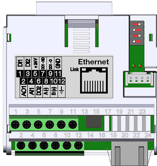
Abbildung 20.5: CFW500-CEMB-TCP / CFW500-CETH-IP / CFW500-CEPN-IO Einsteckmodul
