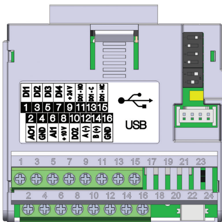
Abbildung 20.3: Steckmodul CFW500-CUSB
