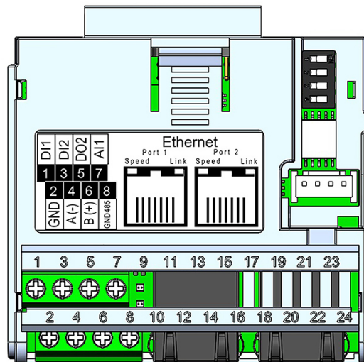
Abbildung 20.6: CFW500-CETH2 Einsteckmodul
