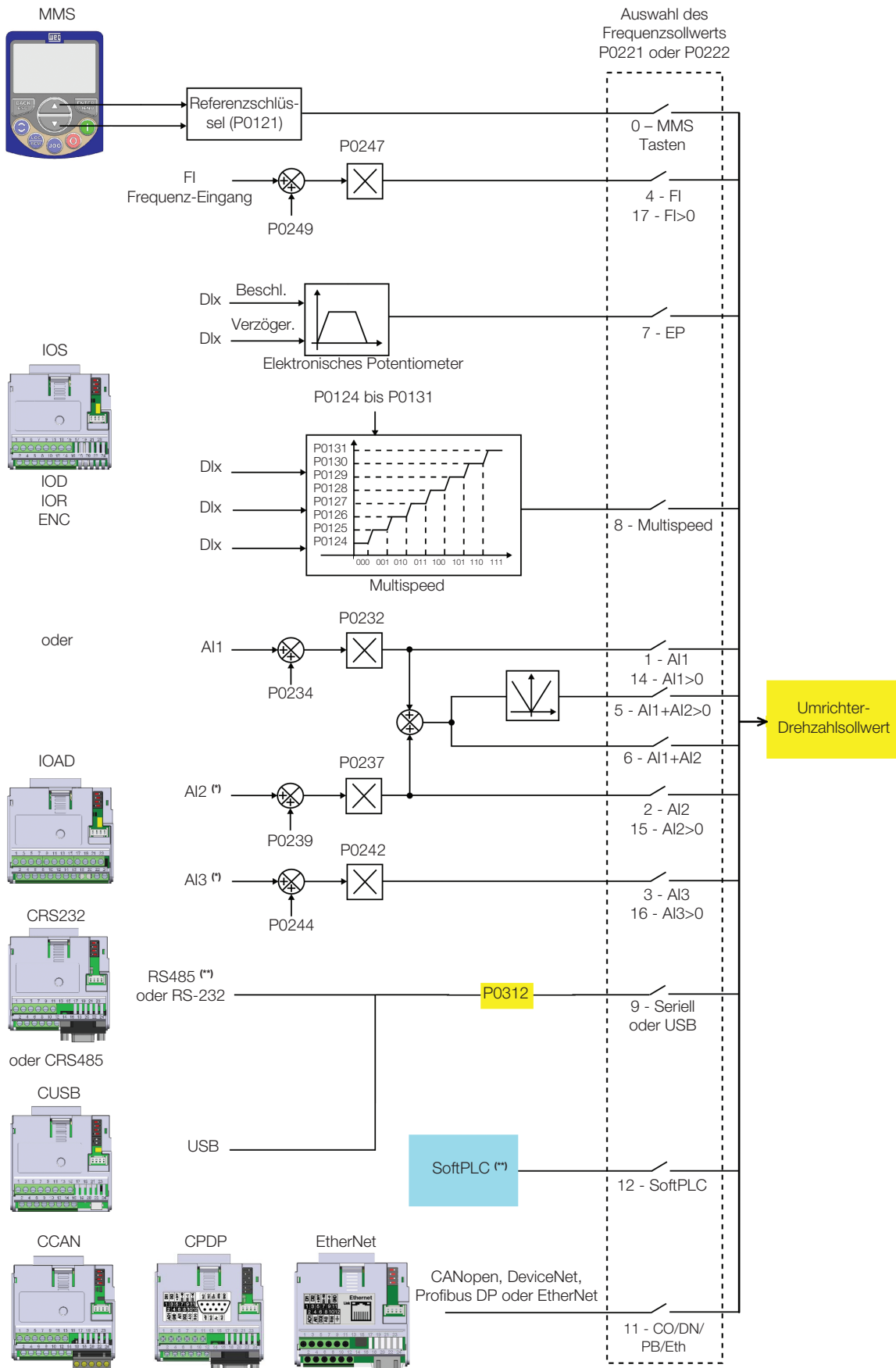
Abbildung 7.3: Struktur zur Auswahl des Drehzahlsollwerts
