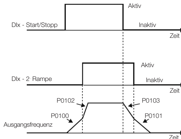
Abbildung 15.14: Beispiel der Funktion 2: Rampe
