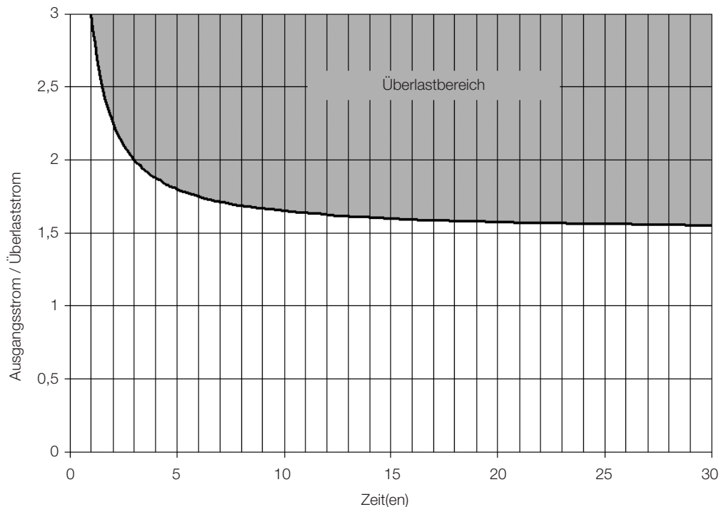
Abbildung 18.2: Auslösung der IGBT-Überlastung
