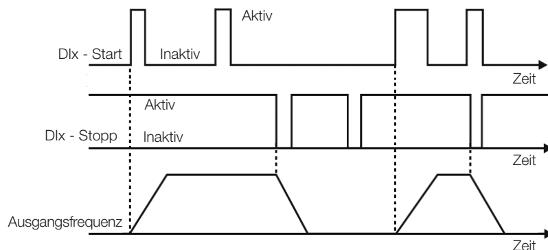
Abbildung 15.10: Beispiel für die dreiadrige Start-/Stopp-Funktion
