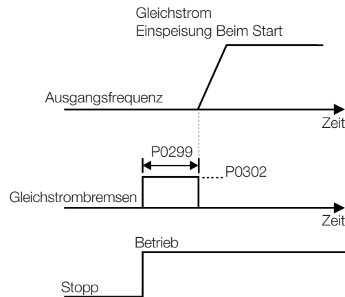
Abbildung 14.6: Betätigung der DC Bremse beim Start
