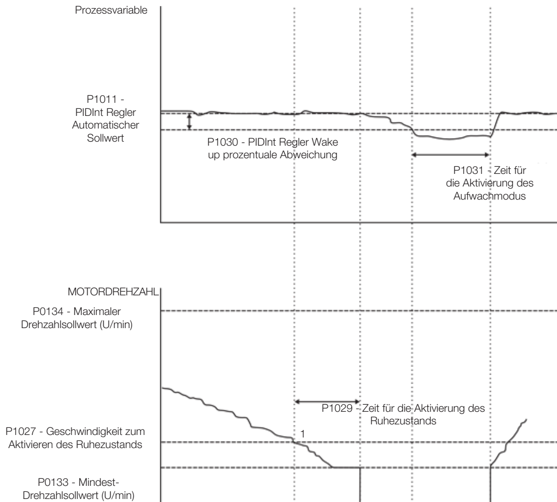
Abbildung 21.1: Funktionsschema für das Einschlafen und Aufwachen
