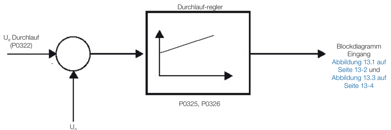
Abbildung 14.5: Durchlauf-PI-Steuerung
