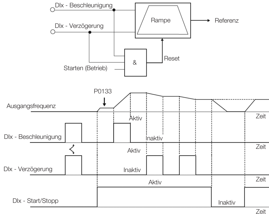
Abbildung 15.13: Beispiel der Funktion Elektronisches Potentiometer (E.P.)
