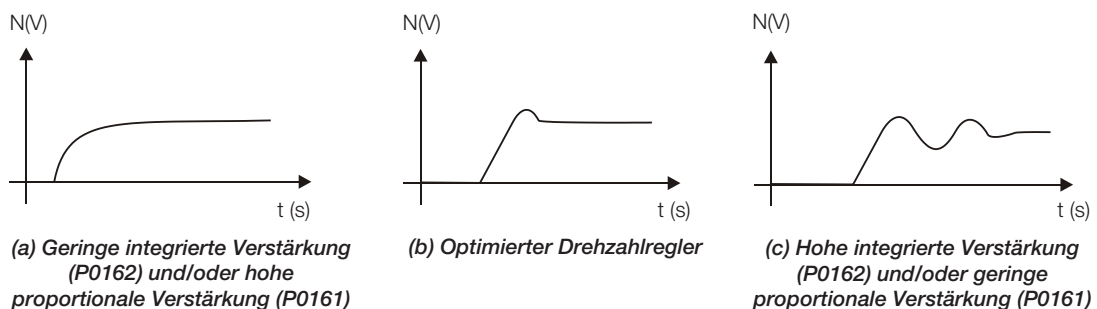
Abbildung 13.5: (a) bis (c) Ansprechtypen von Drehzahlregelungen
