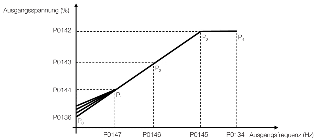
Abbildung 9.3: Bereich der Drehmomentverstärkung
