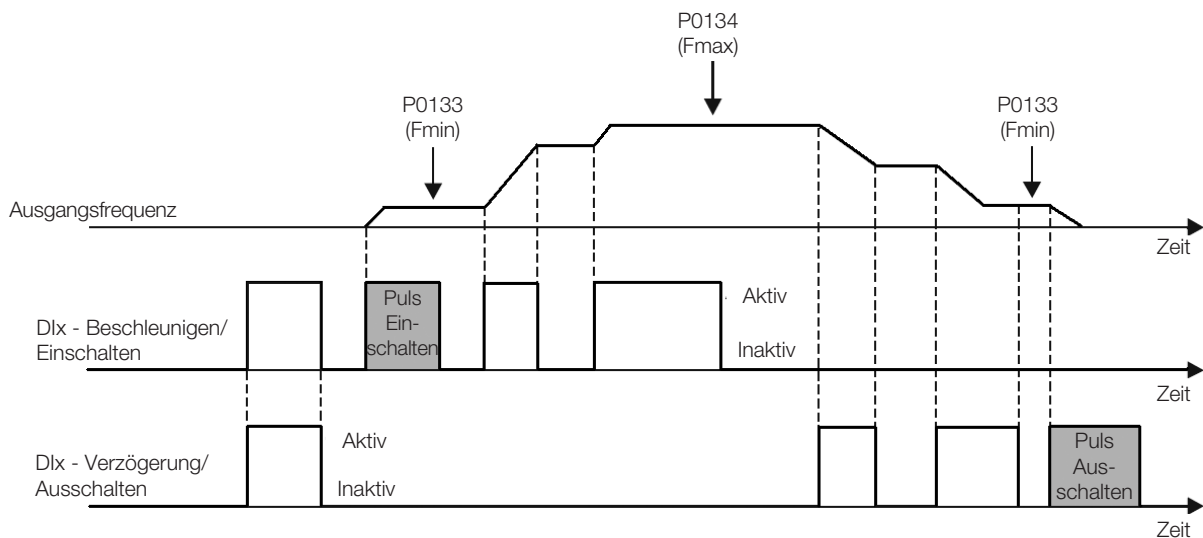
Abbildung 15.16: Beispiel von Beschleunigen Einschalten / Verzögern Ausschalten
