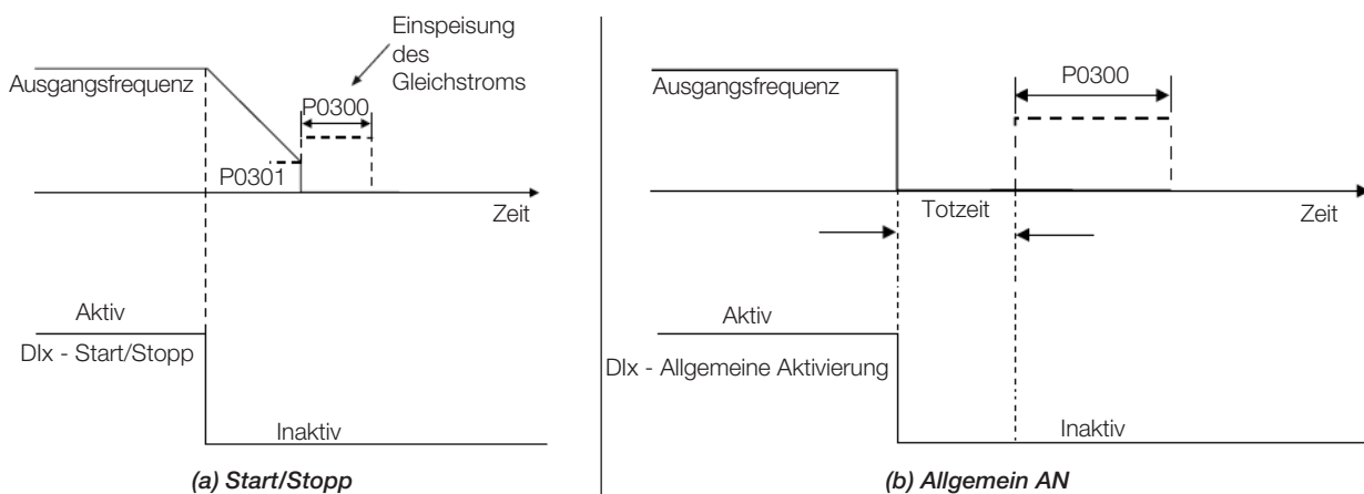
Abbildung 14.7: (a) und (b) Betätigen der DC-Bremse
