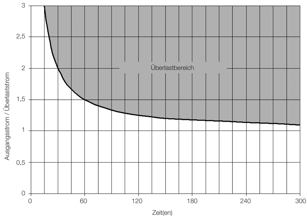
Abbildung 18.1: Aktivierung der Motorüberlastung
