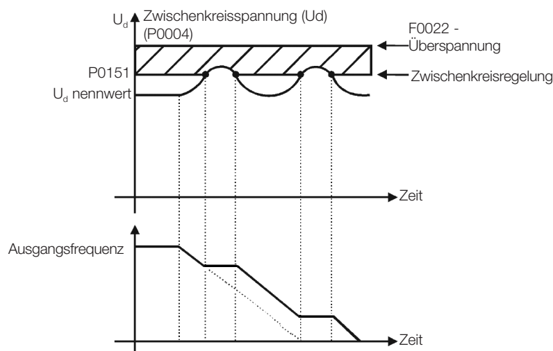
Abbildung 9.6: Beispielgrafik der Begrenzung der Zwischenkreisspannung - Rampe halten
