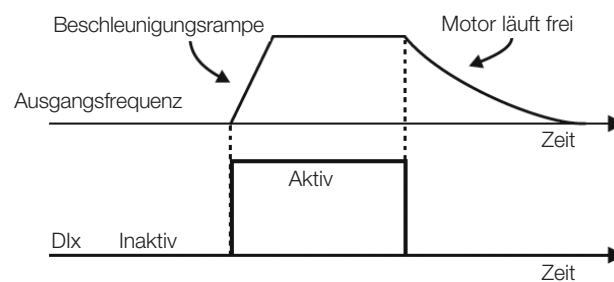
Abbildung 15.7: Beispiel der Funktion Allgemein AN
