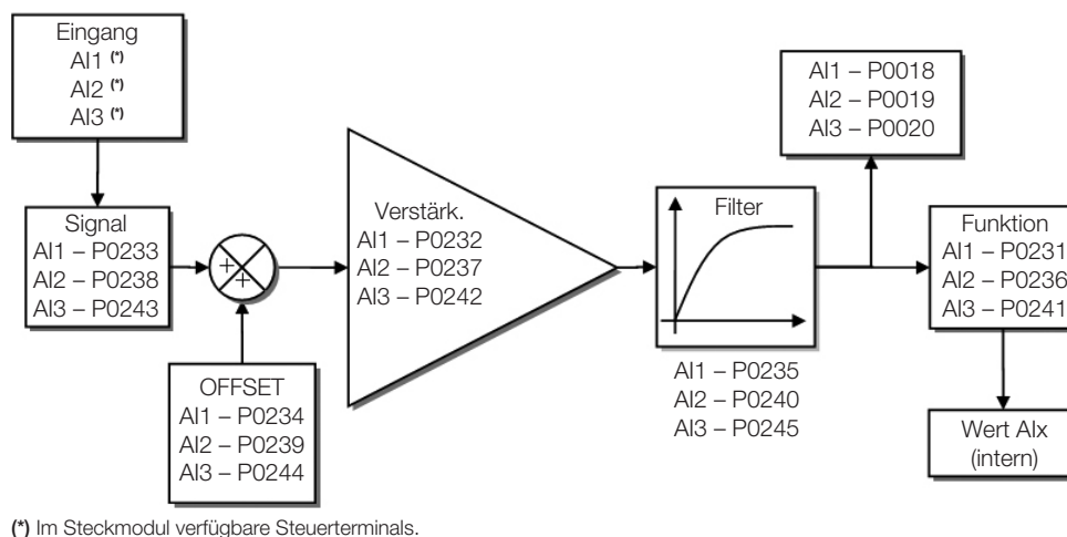
Abbildung 15.2: Blockschaltbild der analogen Eingänge - Alx
