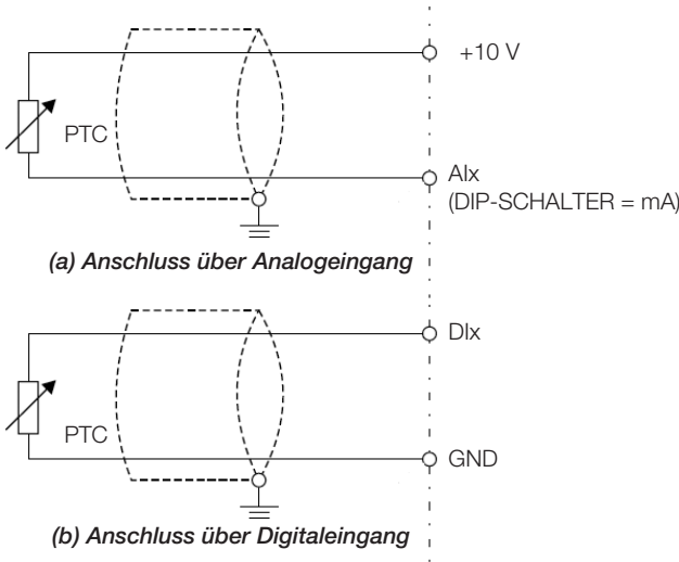
Abbildung 18.3: (a) und (b) Kaltleiter-Anschluss an den MW500
