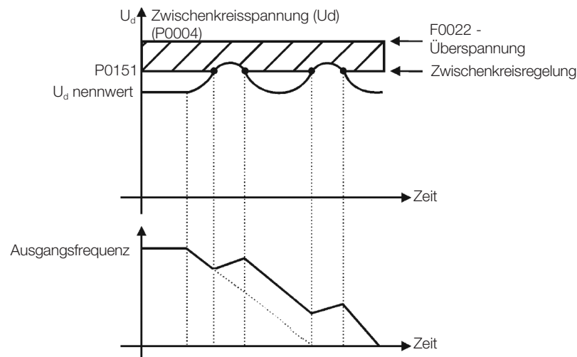
Abbildung 9.8: Beispielgrafik der Begrenzung der Zwischenkreisspannung - Rampe beschleunigen
