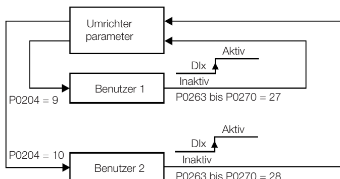
Abbildung 15.15: Blockdiagramm der Funktionen us. 1 und us. 2
