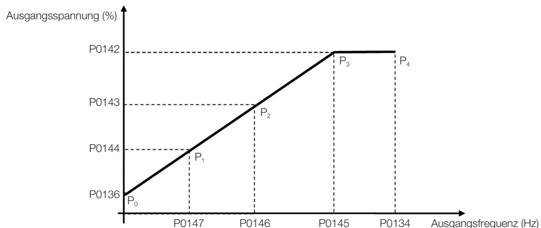
Abbildung 9.2: Kurve-U/f
