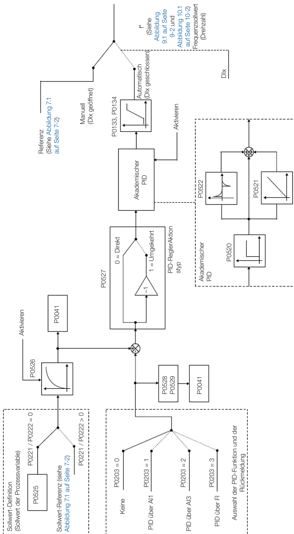
Abbildung 16.1: Blockdiagramm des PID-Reglers
