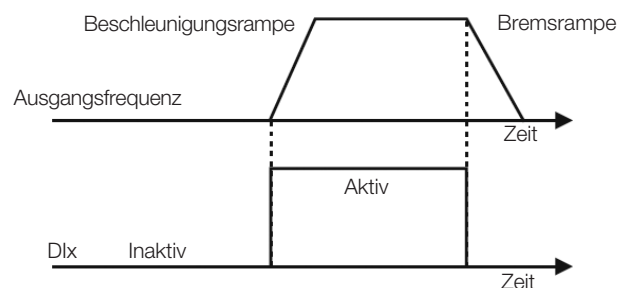
Abbildung 15.6: Beispiel der Betrieb/Stopp-Funktion
