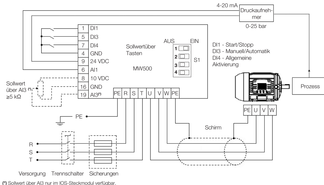
Abbildung 16.2: Beispiel für die Anwendung des MW500 PID-Reglers
