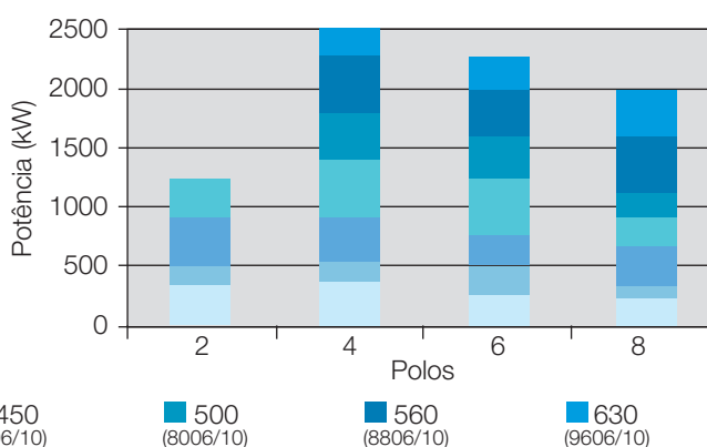
Potência x nº de polos x tamanho de carcaça (4.160 V - 60 Hz)
