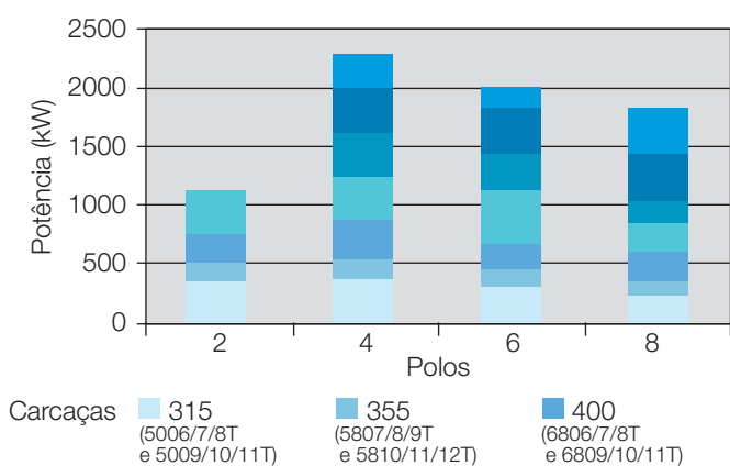
Potência x nº de polos x tamanho de carcaça (4.160 V - 50 Hz)
