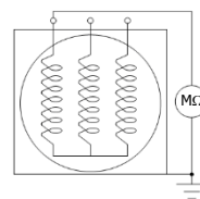
Figura 4.3: Medición en las 3 fases
