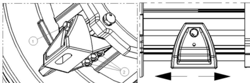
Figura 6.3- Ajuste de la posición del pie
