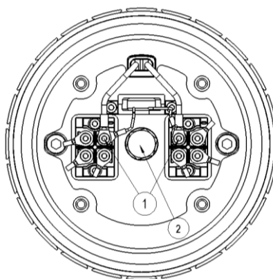
Figura 6.2- Rotor de la excitatriz AW10
