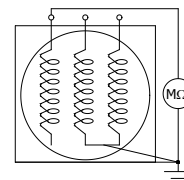
Figura 4.4: Medición en fases separadas
