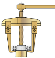
Figura 6.1: Extractor de rodamiento.
