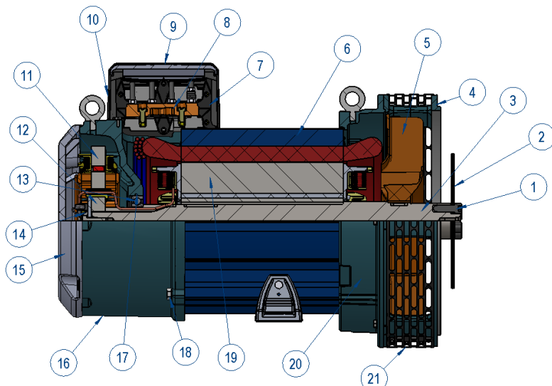
Figura 6.1- Alternador AW10
