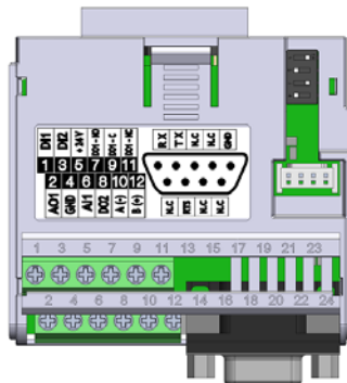
Figura 2.4: Módulo plug-in con conexión RS232
