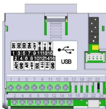
Figura 2.3: Módulo plug-in con conexión USB
