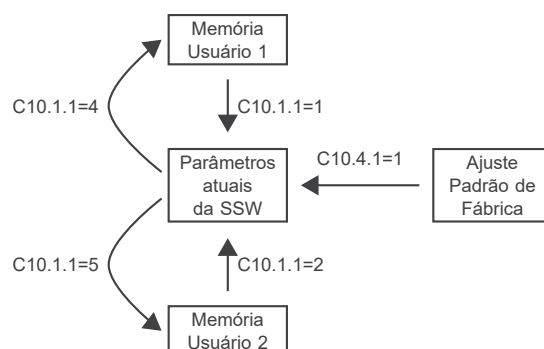
Figura 11.39: Salvamento e carregamento das configurações.
