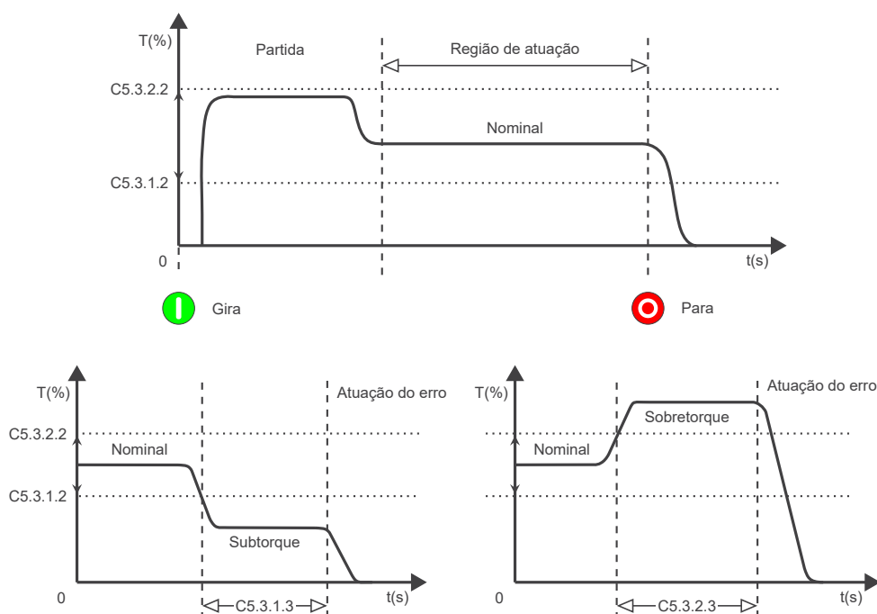
Figura 11.17: Níveis de atuação para sobre e subtorque.
