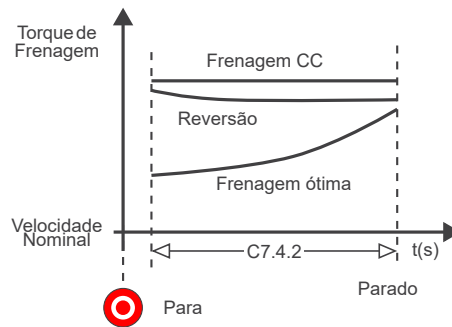
Figura 11.33: Torque de frenagem.
