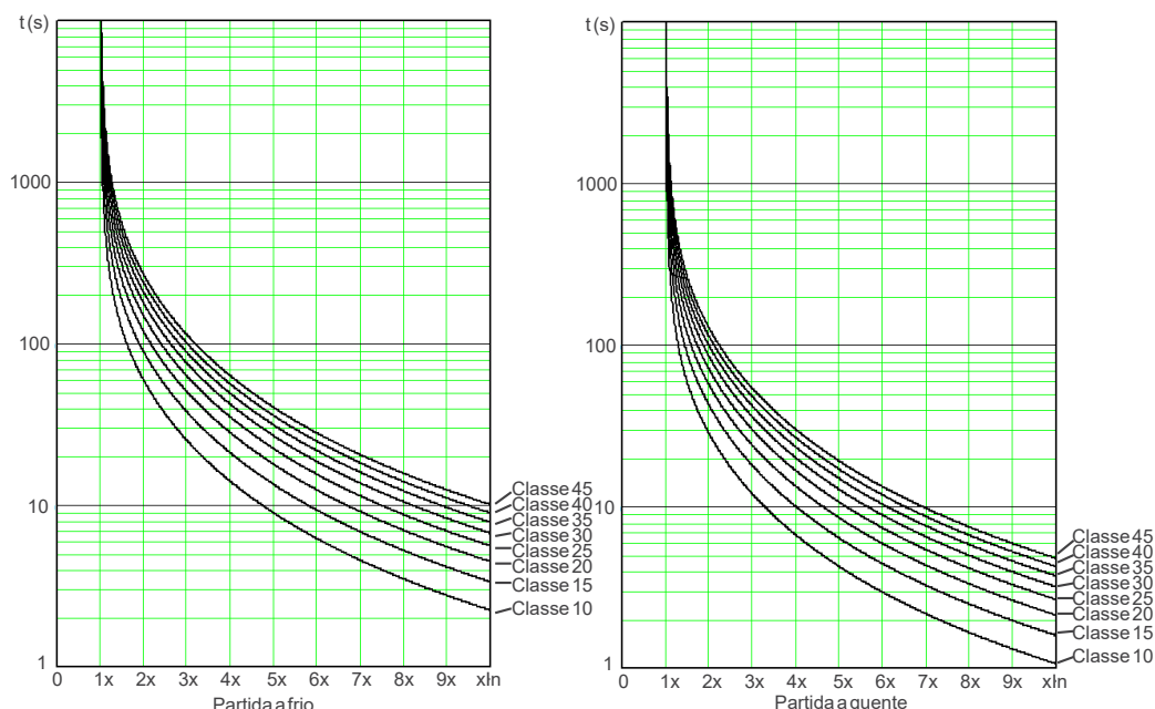
Figura 11.29: Classes Térmicas padrão de proteção do motor.
