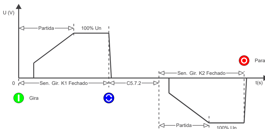
Figura 11.30: Troca do sentido de giro via contator.
