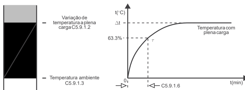
Figura 11.24: Constante de aquecimento do motor para corrente nominal.
