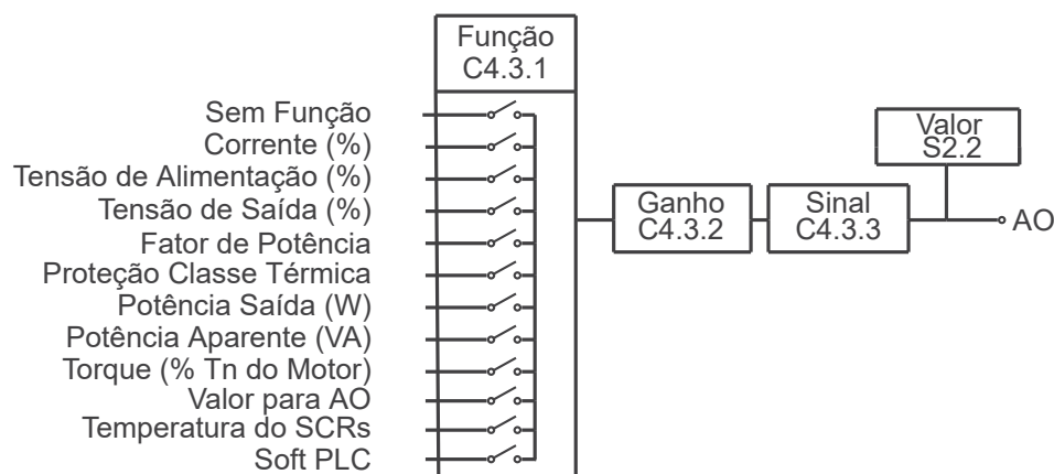
Figura 11.12: Bloco diagrama das saídas analógicas.
