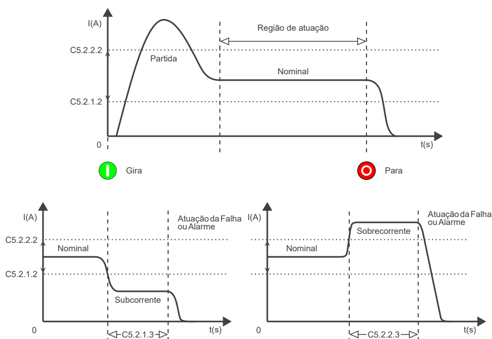
Figura 11.16: Níveis de atuação para sobre e subcorrente.
