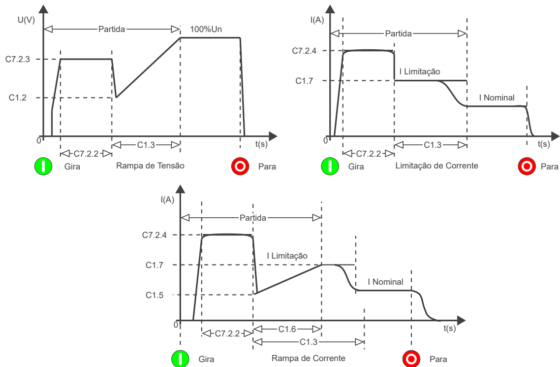
Figura 11.32: Níveis de atuação do pulso de torque na partida.
