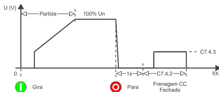
Figura 11.36: Frenagem CC.
