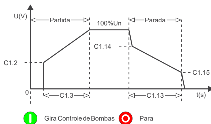
Figura 13.11: Partida com controle de bombas.
