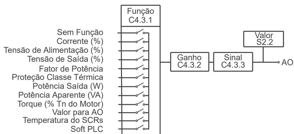
Figura 11.13: Bloco diagrama das saídas analógicas.
