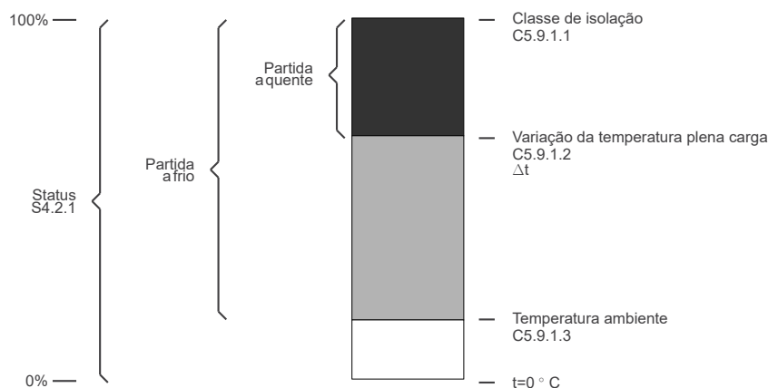
Figura 11.22: Faixas de temperaturas do motor dentro da classe de isolamento.
