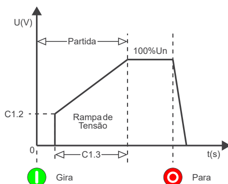
Figura 11.3: Rampa de aceleração por Rampa de Tensão.
