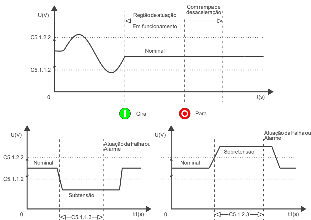
Figura 11.14: Níveis de atuação da sobre e subtensão.
