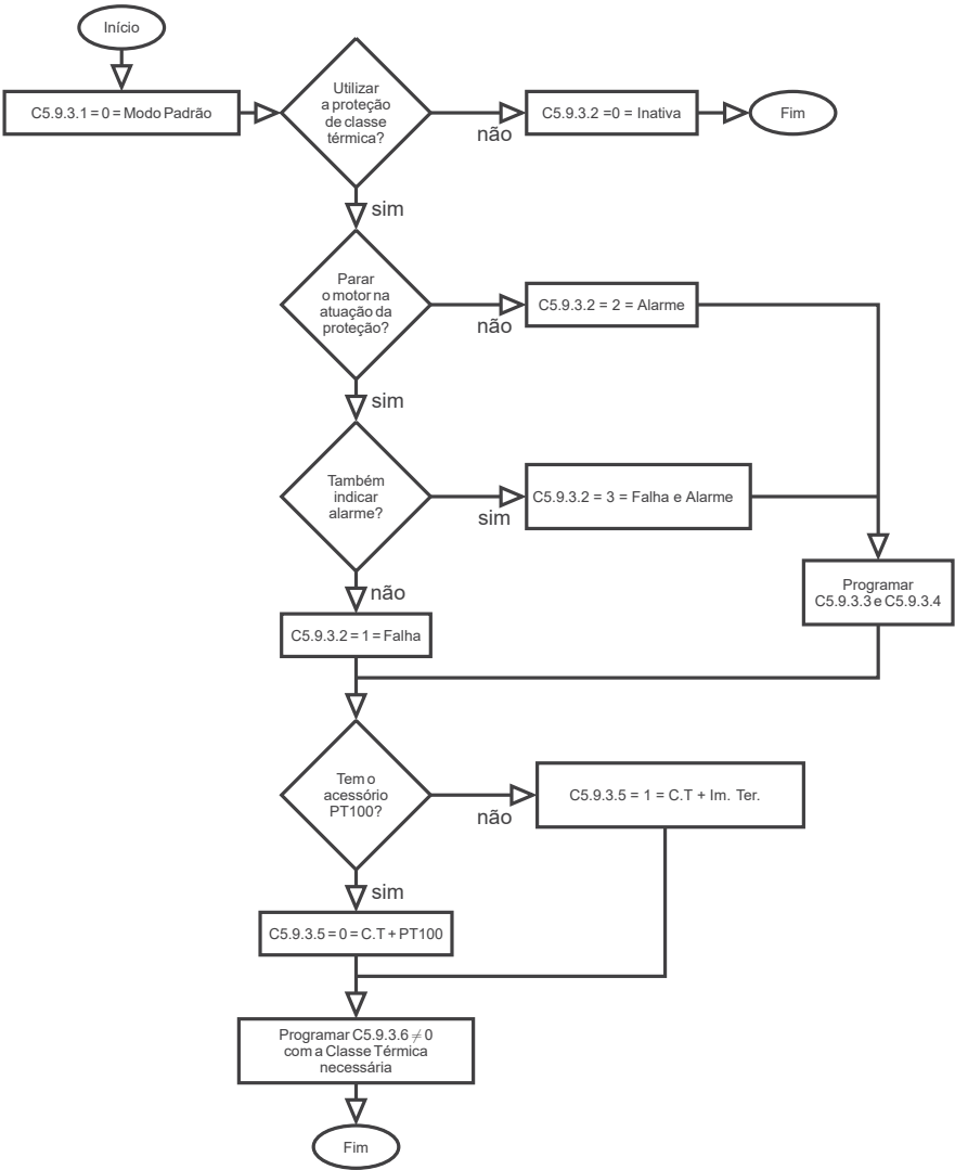
Figura 11.27: Sequência de programação da Proteção de Classe Térmica modo padrão.
