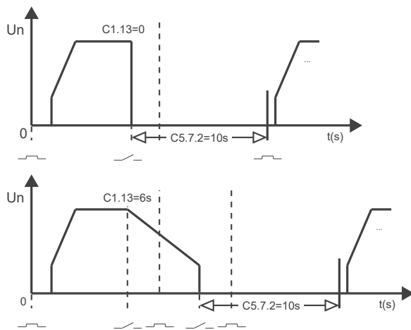
Figura 11.20: Acionamento via entrada digital (DI1).
