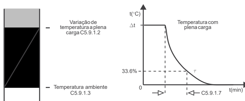
Figura 11.25: Constante de resfriamento do motor desenergizado.
