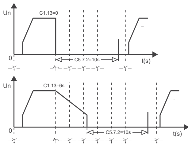
Figura 11.19: Acionamento via entradas digitais a três fios (DI1 e DI2).
