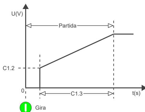
Figura 11.2: Tensão Inicial.
