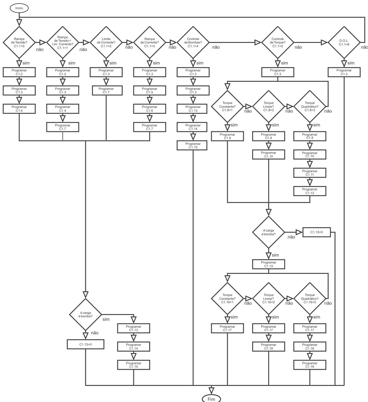
Figura 11.1: Sequência de programação dos tipos de controle.
