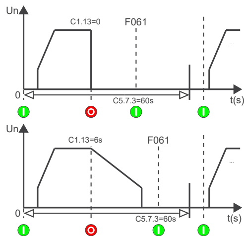
Figura 11.21: Tempo entre partidas.
