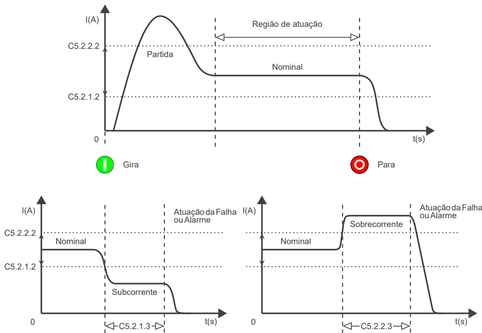
Figura 11.15: Níveis de atuação para sobre e subcorrente.
