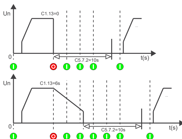
Figura 11.18: Acionamento via IHM.
