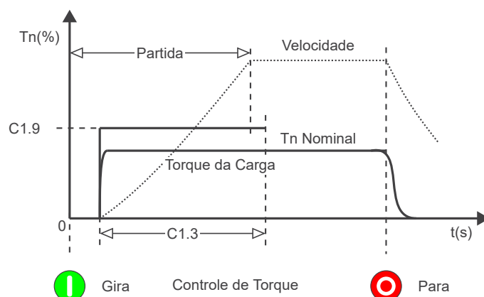
Figura 13.12: Partida com controle de torque constante, 1 ponto.
