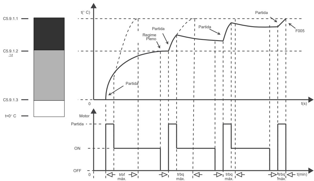
Figura 11.23: Aquecimento do motor.
