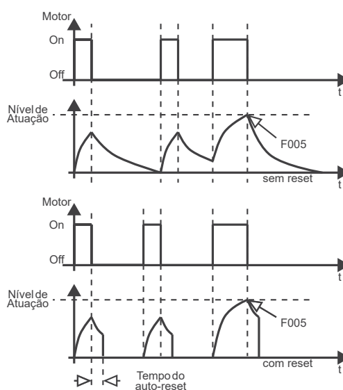
Figura 11.26: Reset da imagem térmica do motor.
