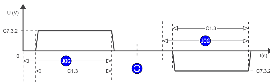
Figura 11.31: Troca de sentido de giro apenas para JOG.
