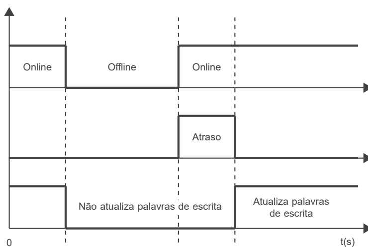
Figura 11.38: Atraso na atualização das palavras de I/O
