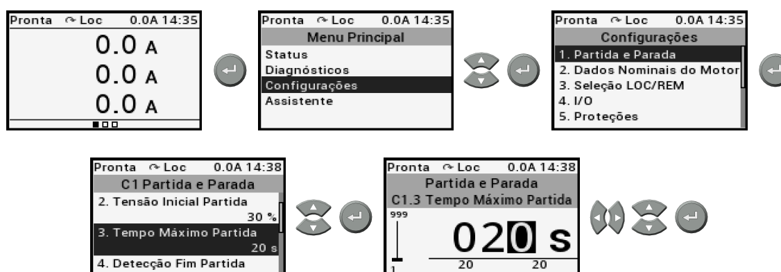
Figura 8.6: Programação do tempo máximo de partida
