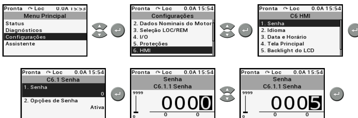
Figura 8.9: Senha para possibilitar alteração de parâmetros
