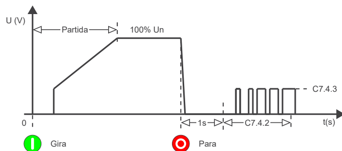
Figura 11.35: Frenagem ótima.
