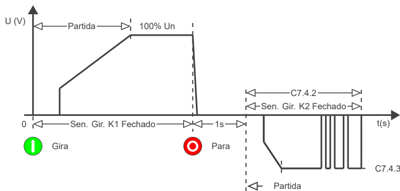
Figura 11.34: Frenagem por reversão.
