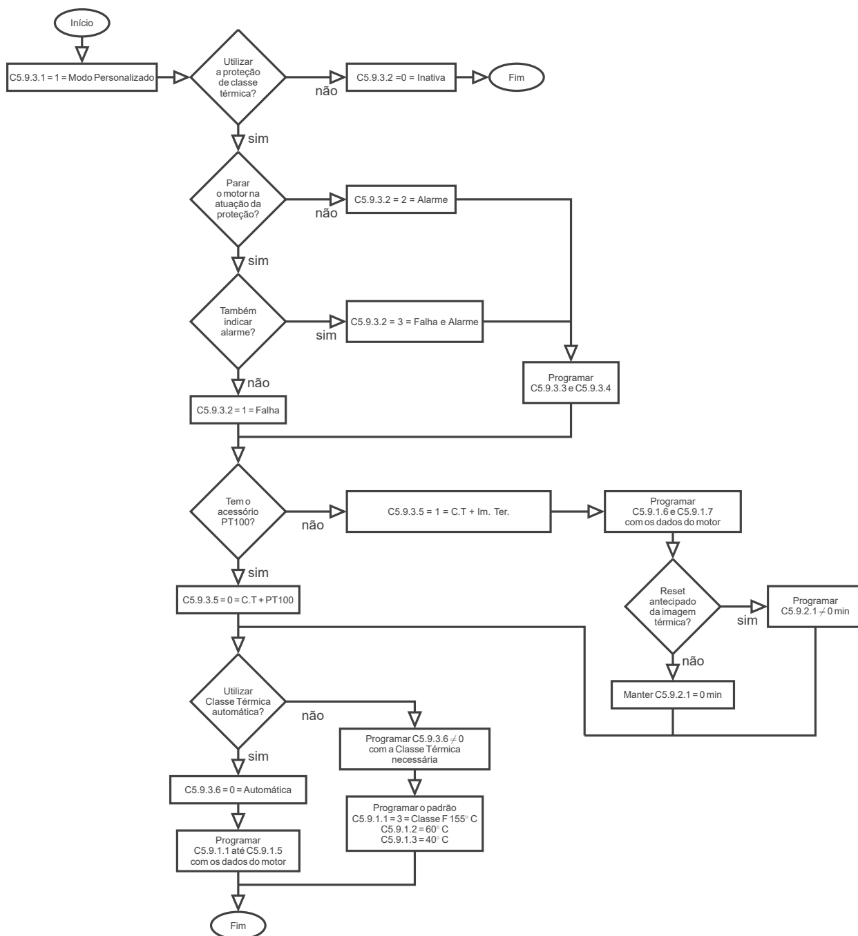
Figura 11.28: Sequência de programação da Proteção de Classe Térmica modo personalizado.
