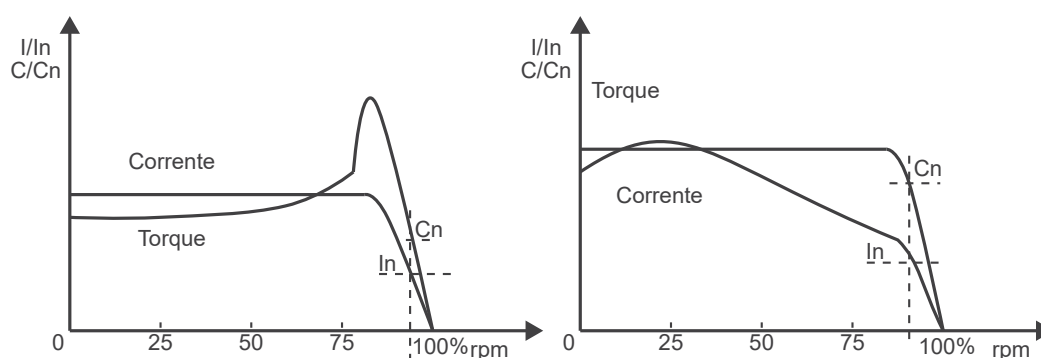
Figura 13.2: Curvas características de torque e corrente em uma partida com Limitação de Corrente e por Controle de Torque.
