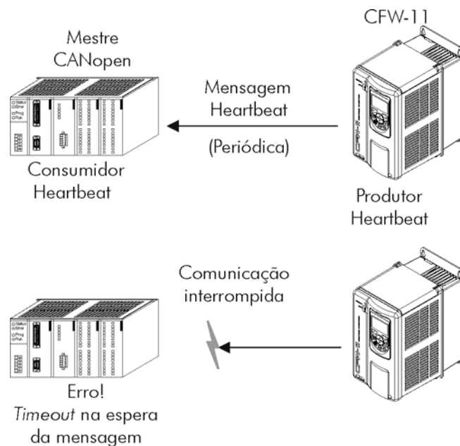
Figura 5-7 - Serviço de controle de erros – Heartbeat
