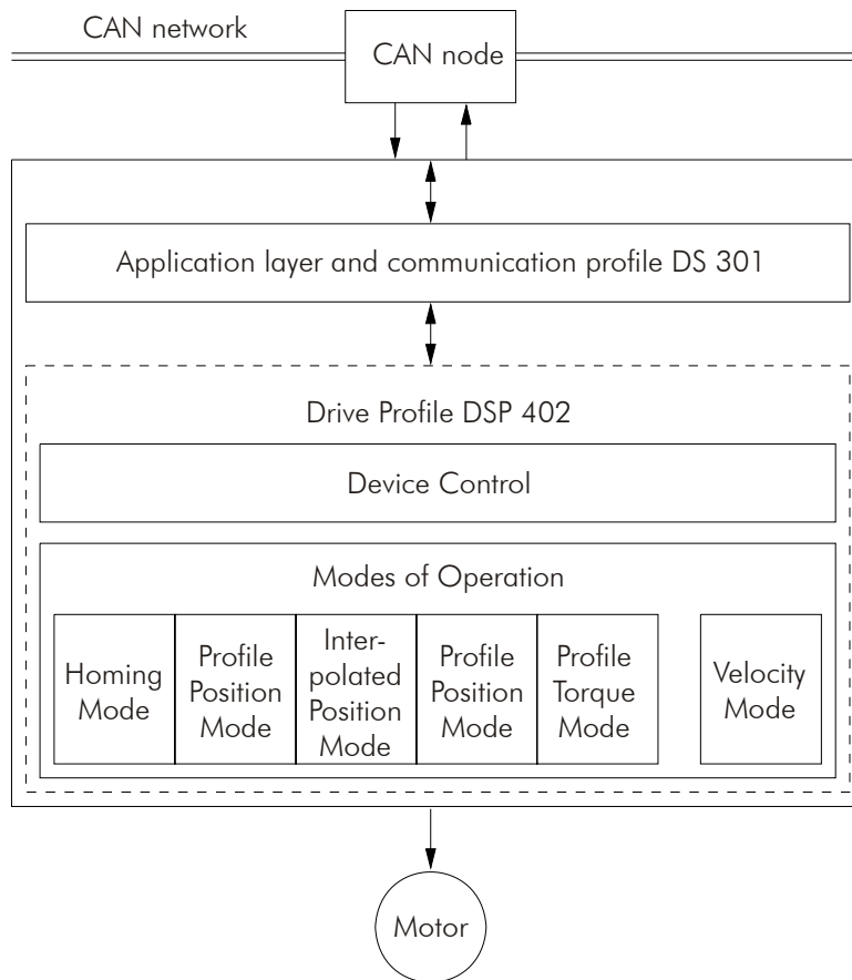
Figura 6-1 - Arquitetura de comunicação para um drive na rede CANopen
