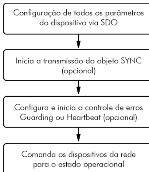
Figura 5-8 - Fluxograma do processo de inicialização
