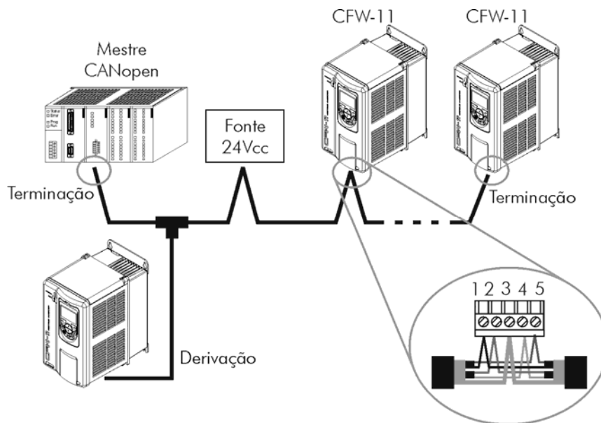
Figura 2-1 - CFW-11 em rede CANopen
