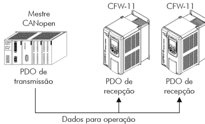
Figura 5-2 - Comunicação utilizando PDOs
