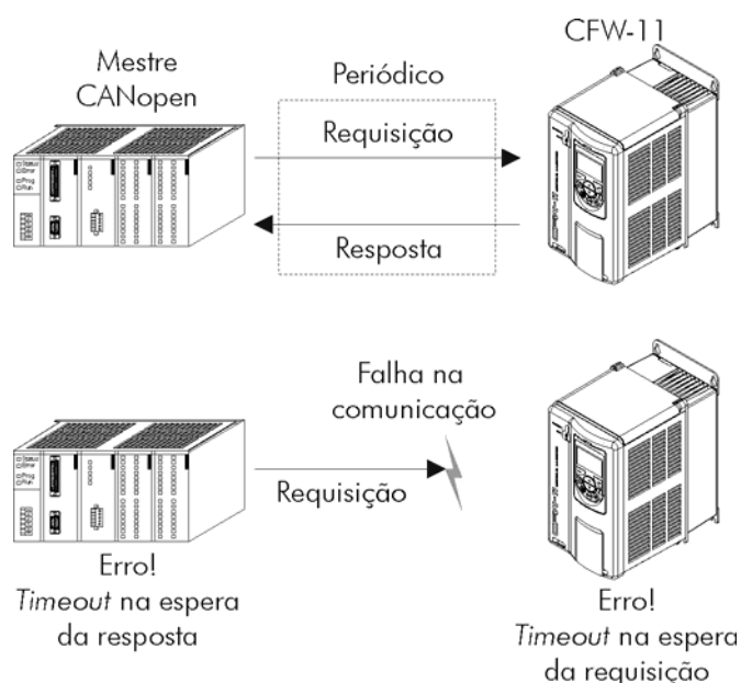
Figura 5-6 - Serviço de controle de erros – Node Guarding
