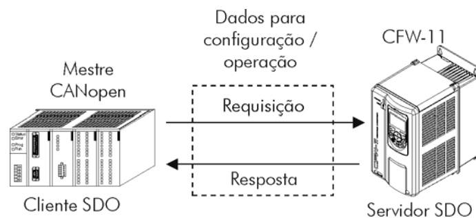
Figura 5-1 - Comunicação entre Cliente e Servidor SDO
