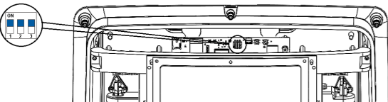
Figura 5.1: Llaves de selección de la corriente nominal
