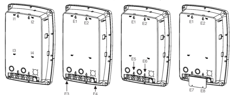
Figura 4.2: Métodos de fixação da WEMOB-PARKING
