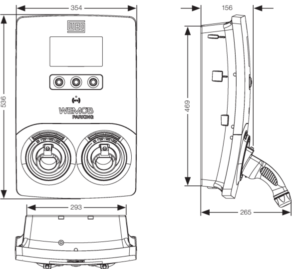
Figura 7.1: Dimensões da estação de recarga WEMOB-PARKING em mm
