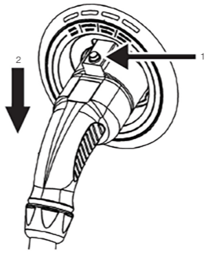
Figura 5.4: Procedimento para retirada do plugue do soquete
