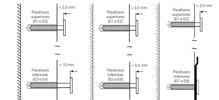
(a) Fixação 1 - sem suporte metálico (b) Fixação 2 - sem suporte metálico (c) Fixação com suporte metálico
