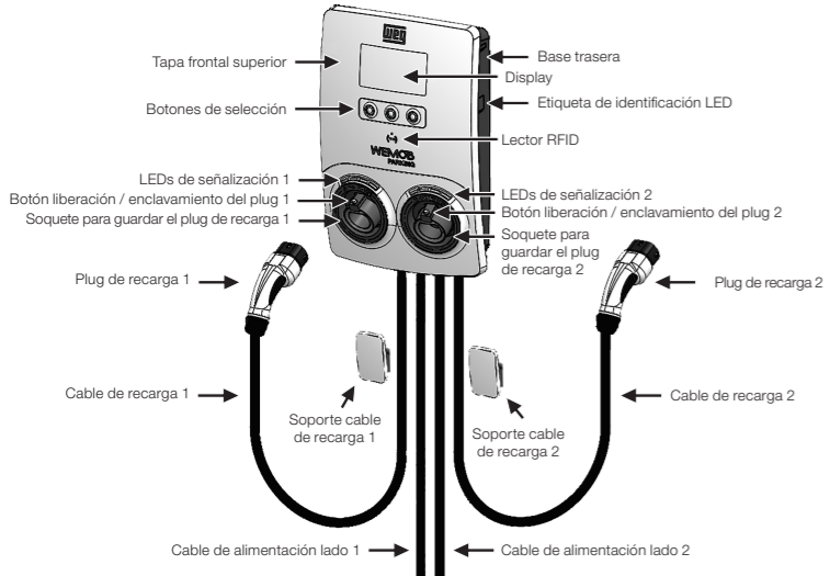
Figura 2.1: Visión general de la WEMOB-PARKING
