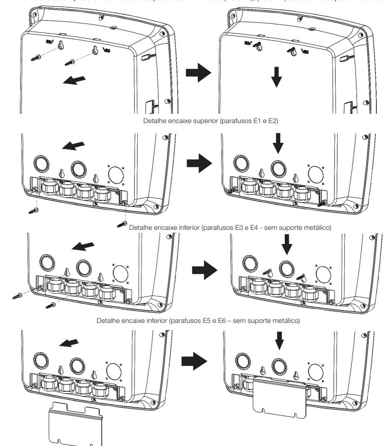
(a) Fixação 1 - sem suporte metálico (b) Fixação 2 - sem suporte metálico (c) Fixação com suporte metálico
