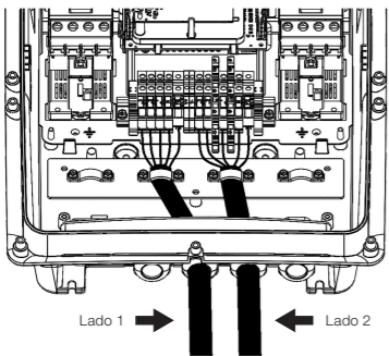
Figura 5.2: Montagem aparente dos cabos de alimentação (lado 1 e 2)
