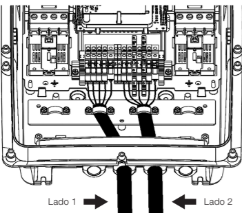
Figura 5.2: Montaje aparente de los cables de alimentación (lado 1 y 2)
