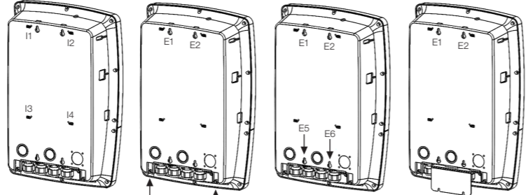
Figura 4.2: Métodos de fijación de la WEMOB-PARKING
