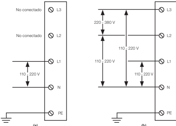
Figura 5.3: (a) y (b) Ejemplos de conexión eléctrica monofásica o bifásica y trifásica
