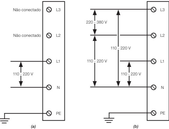
Figura 5.3: (a) e (b) Exemplos de ligação elétrica monofásica ou bifásica e trifásica
