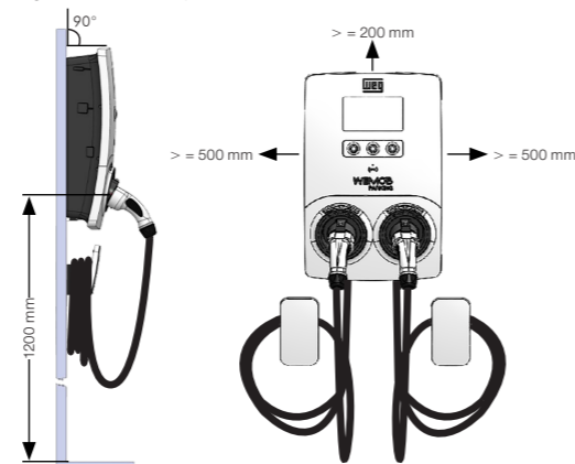
Figura 4.1: Posição de montagem e distanciamento da WEMOB-PARKING
