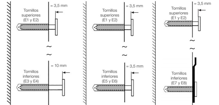
(a) Fijación 1 - sin soporte metálico (b) Fijación 2 - sin soporte metálico (c) Fijación con soporte metálico
