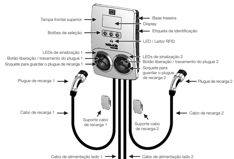
Figura 2.1: Visão geral da WEMOB-PARKING
