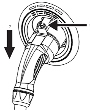
Figura 5.4: Procedimiento para retirada del plug del stecker
