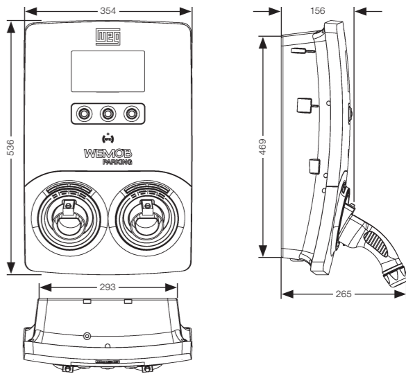
Figura 7.1: Dimensiones de la estación de recarga WEMOB-PARKING en mm
