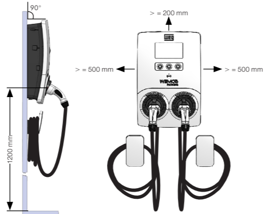
Figura 4.1: Posición de montaje y distanciamiento de la WEMOB-PARKING
