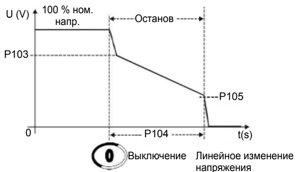
Рисунок 6.4. Линейное замедление путем декремента напряжения
