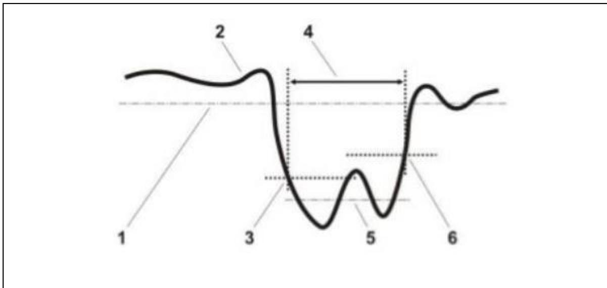
Figura 25 - Exemplo de detecção de uma interrupção de tensão - 1 - Tensão de referência, 2 - Tensão de entrada RMS, 3 - Limite de interrupção inicial, 4 - Duração de corte, 5 - Magnitude do corte, 6 - Limite de interrupção final
