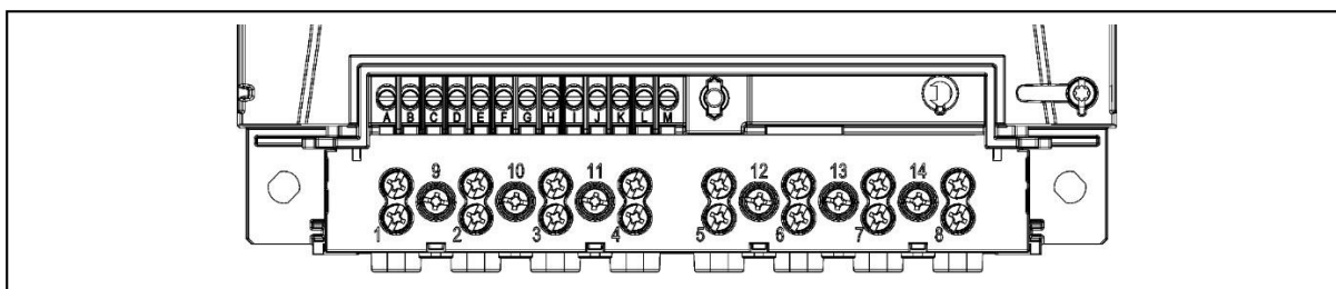
Figura 16 - Identificação dos Terminais de conexão da linha e carga e os terminais de sinal dos medidores SM W3000i
