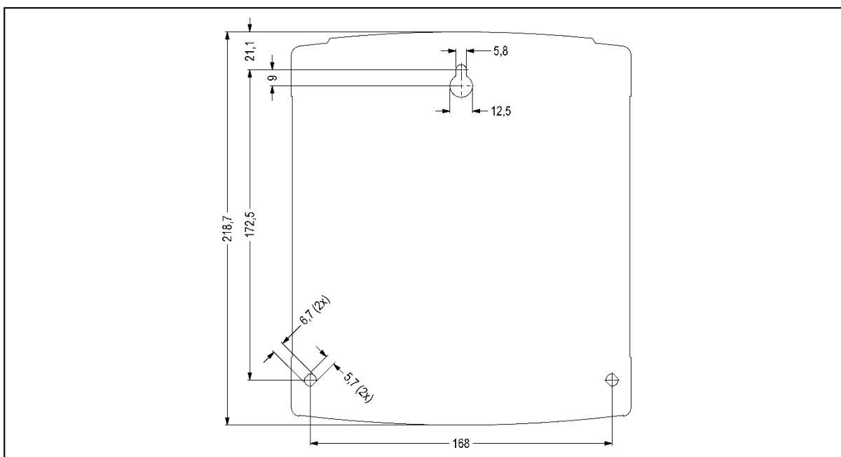
Figura 12 - Cotas para a fixação dos parafusos - medidores SM W3000i (SEM acessório de comunicação).
