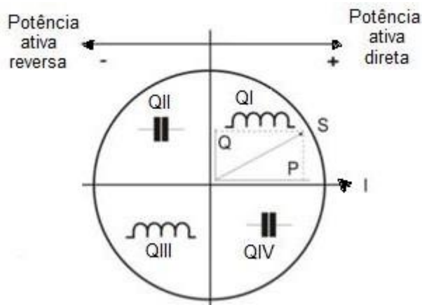
Figura 22 – Medição em 4 Quadrantes
