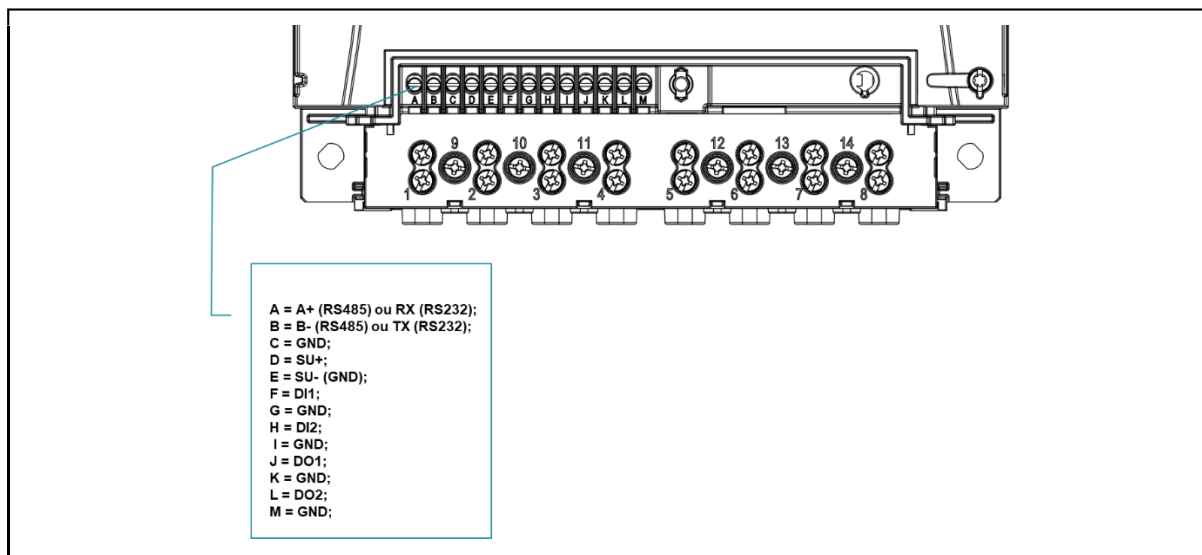
Figura 20 - Configuração dos pinos nos bornes SM W3000i.
