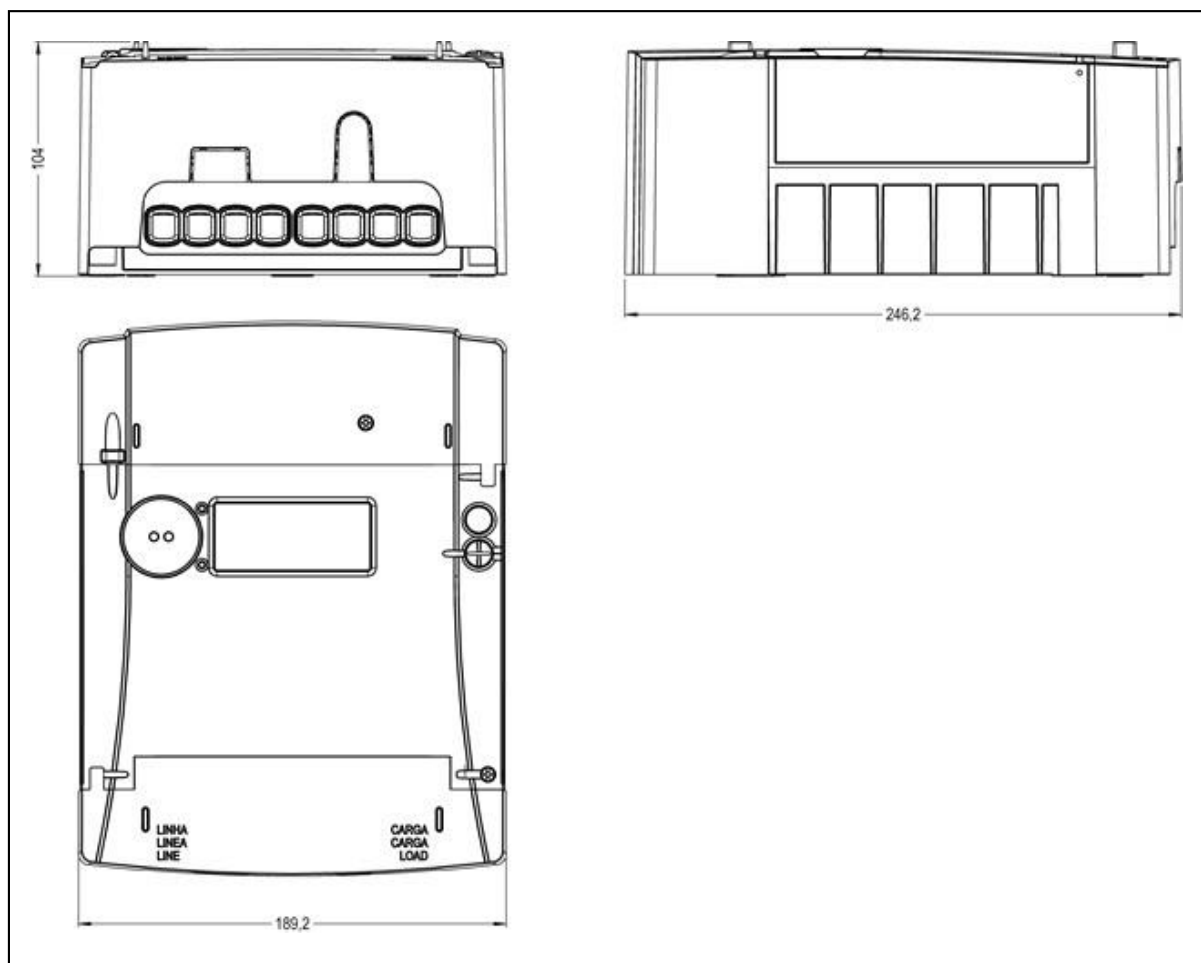
Figura 30 - Dimensões externas dos medidores SM W3000i com tampa superior longa.
