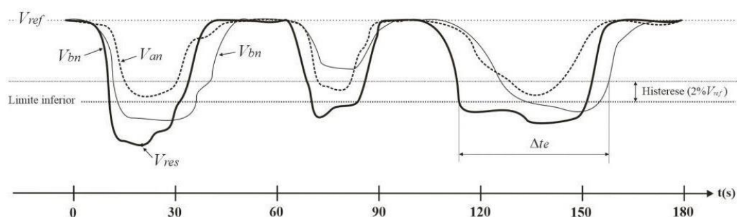
Figura 26 – Exemplo de agregação temporal do VTCD em uma janela de 180 segundos.
