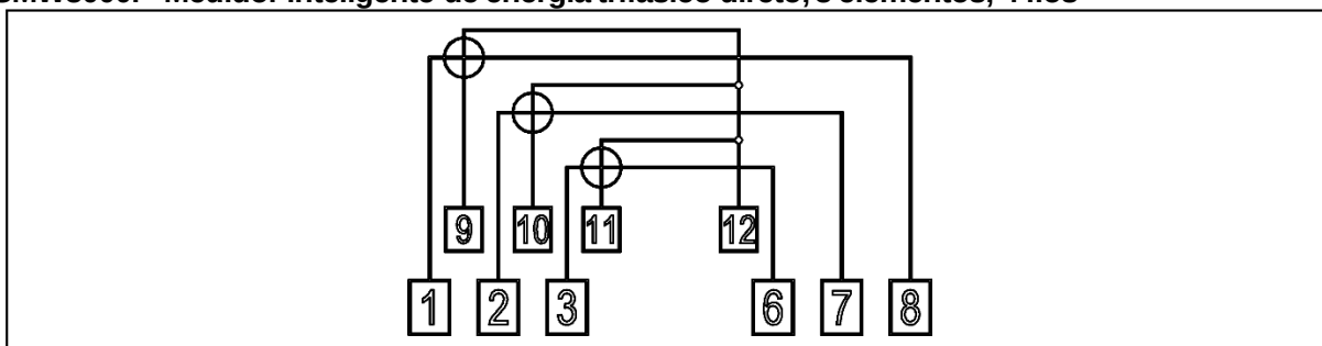
Figura 17 - Esquema de conexão Trifásico 3 Elementos 4 Fios
