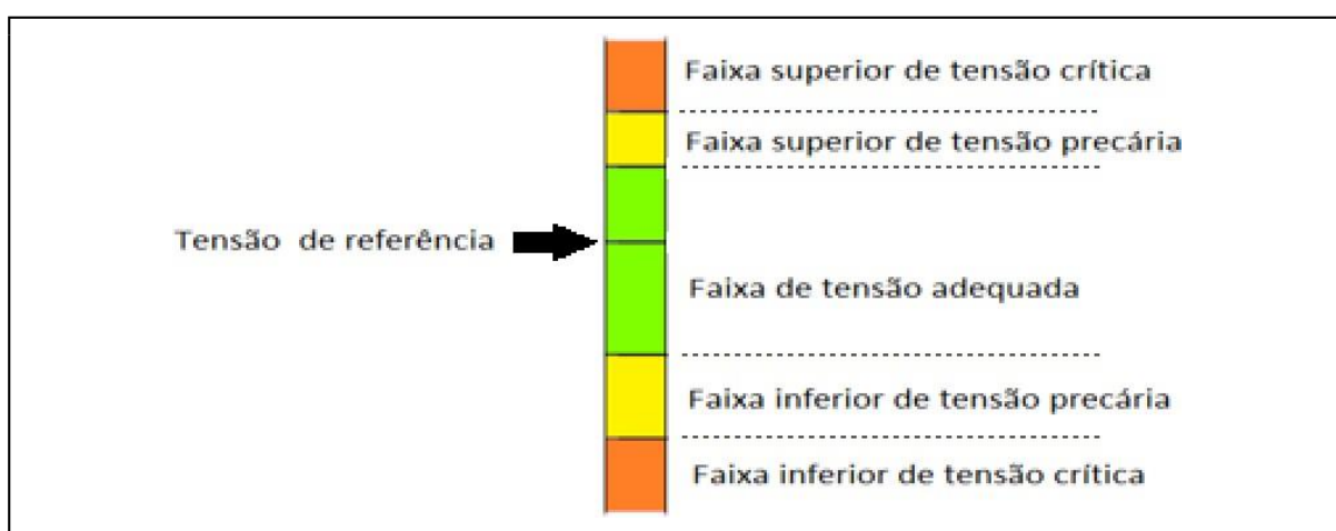
Figura 24 - Faixas de tensão em relação a tensão de referência, segundo PRODIST.
