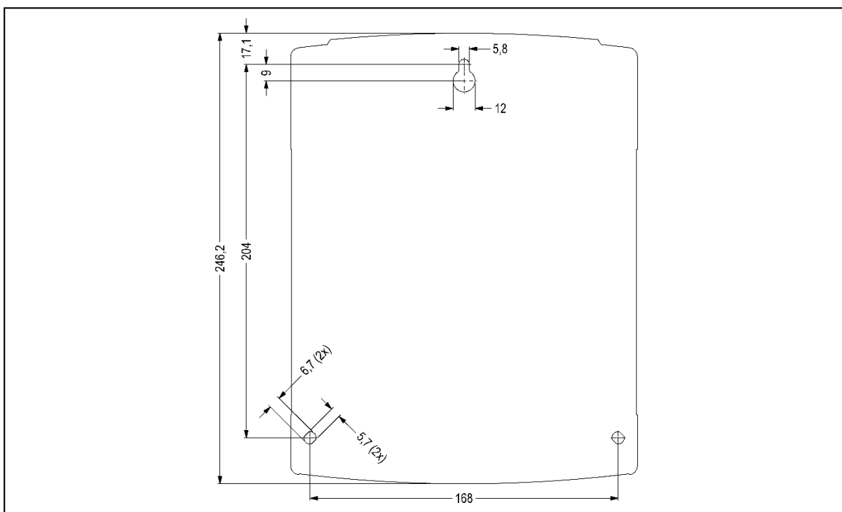
Figura 14 - Cotas para a fixação dos parafusos - medidores SM W3000i (COM acessório de comunicação).
