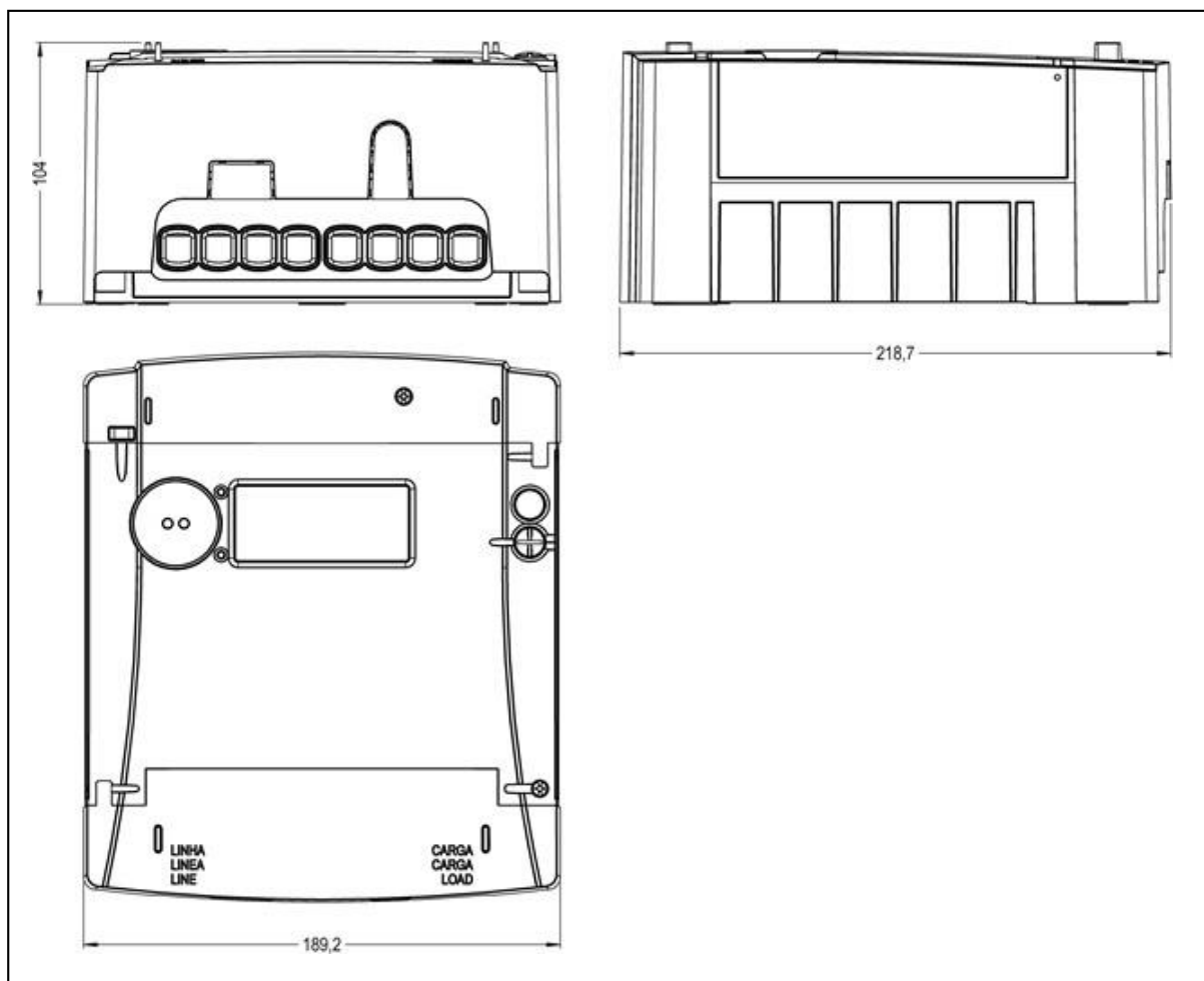
Figura 29 - Dimensões externas dos medidores SM W3000i com tampa superior curta.
