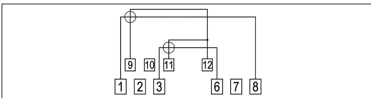
Figura 18 - Esquema de conexão Trifásico 2 Elementos 3 Fios
