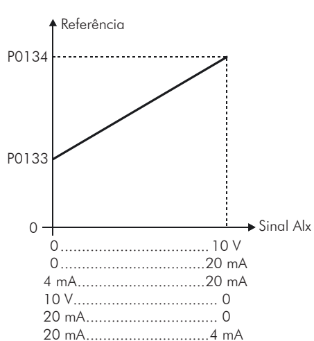
(a) Atuação das Entradas Analógicas com Zona Morta Inativa
