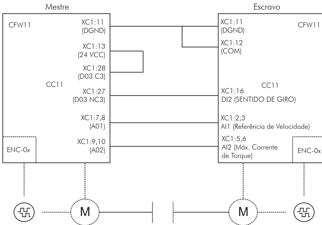
Figura 13.8 - Polaridade de torque +/-
