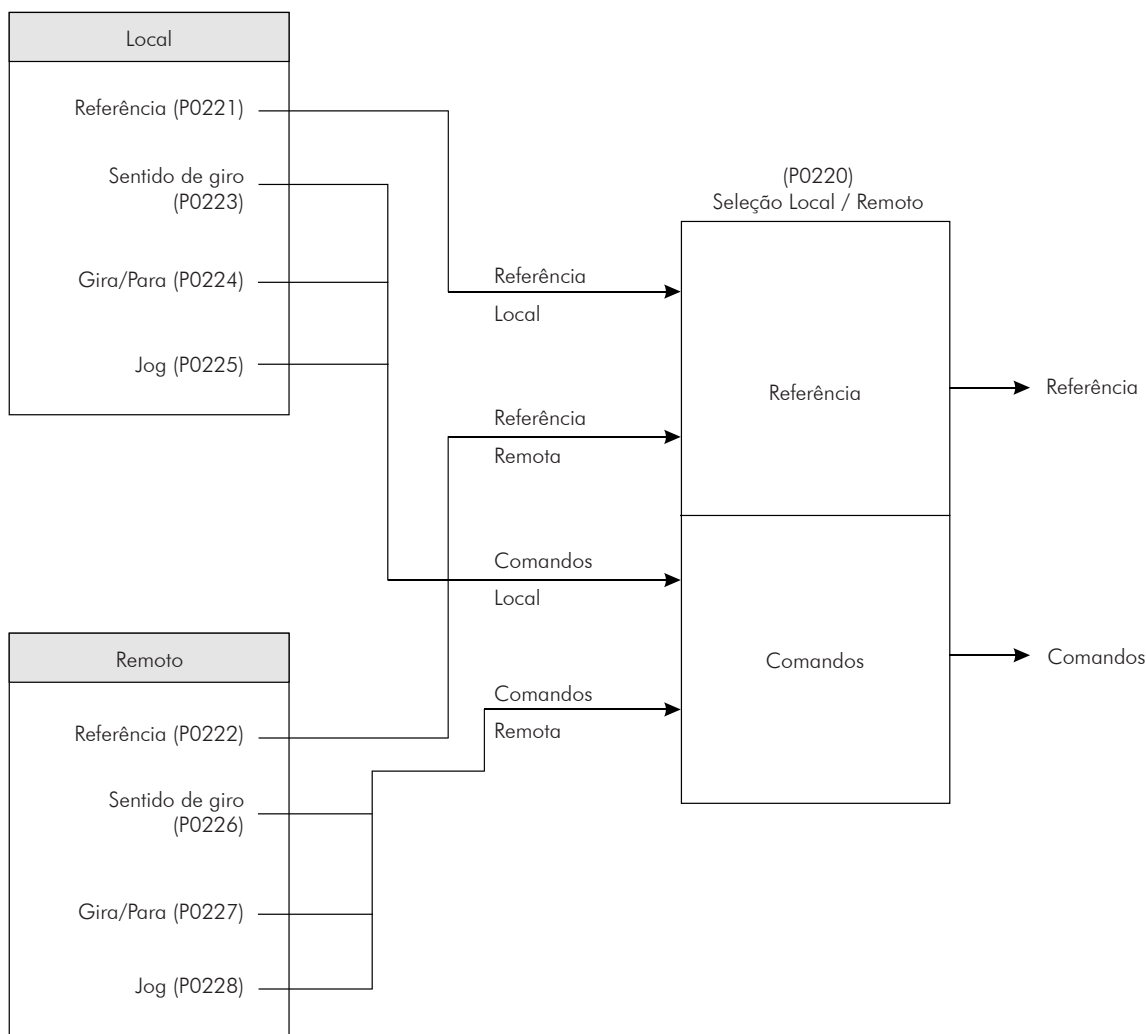
Figura 13.11 - Blocodiagrama Situação Local / Remoto
