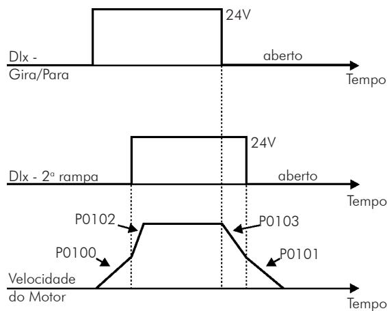
Figura 12.1 - Atuação da 2ª rampa
