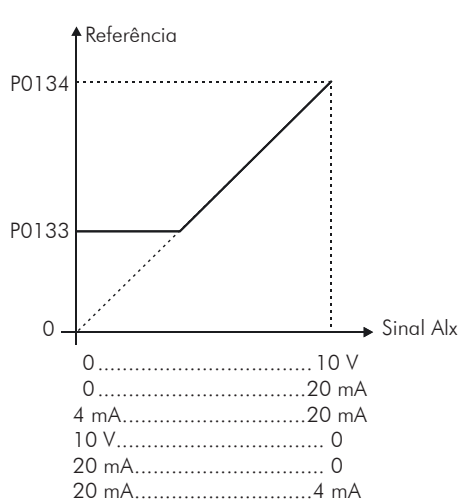
(b) Atuação das Entradas Analógicas com Zona Morta Ativa
