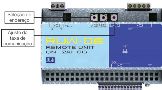
Figura 5: Chaves hexadecimal para configuração da RUW-06
