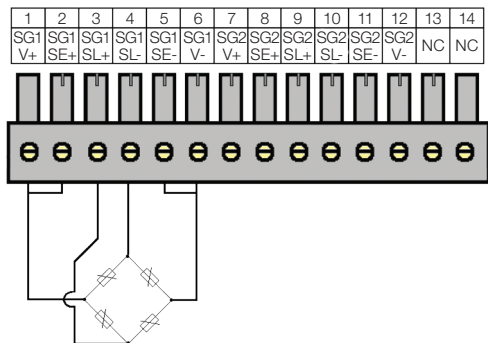
Figura 4: Esquema de ligação da entrada célula de carga a 4 fios (jumper entre V e SE)
