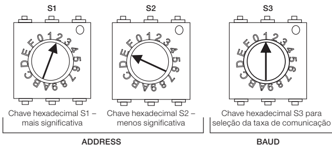
Figura 6: Chaves hexadecimal para configuração da RUW-06
