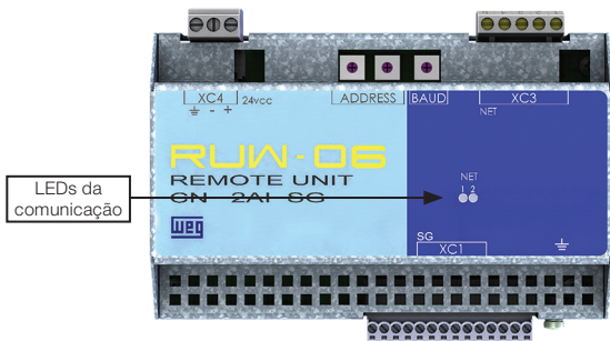
Figura 7: LED de indicação da RUW-06
