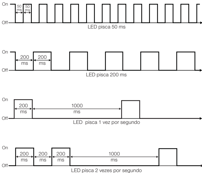
Figura 8: Diagrama de tempo para o comportamento da sinalização
