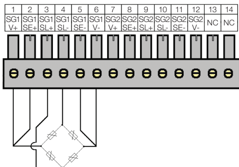
Figura 3: Esquema de ligação da entrada célula de carga a 6 fios
