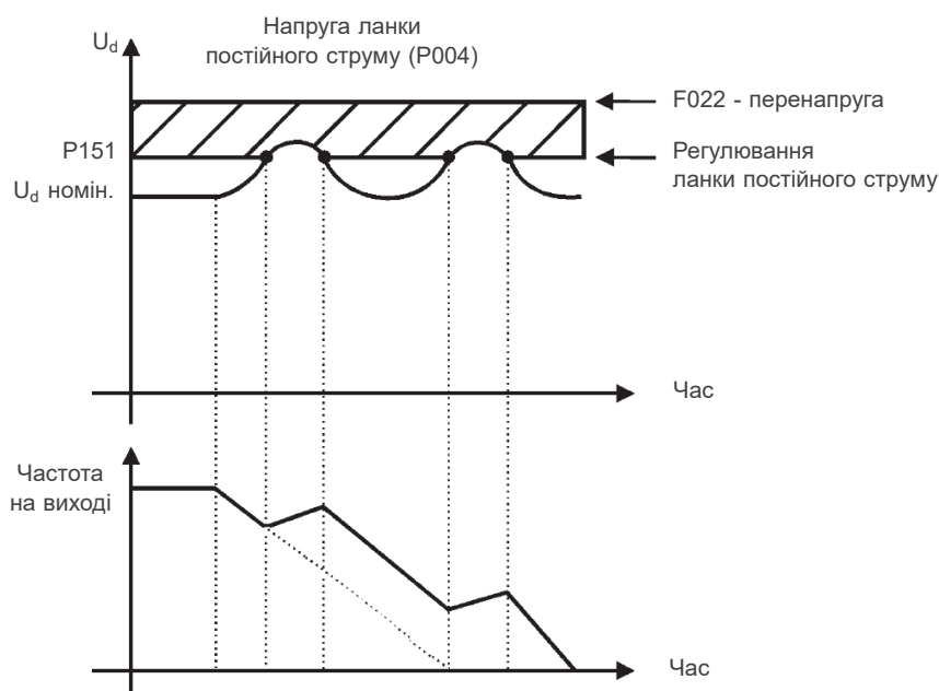
Малюнок 8.5: Приклад графіка обмеження напруги ланки постійного струму - Рампа прискорення (P150 = 0 або 1)
