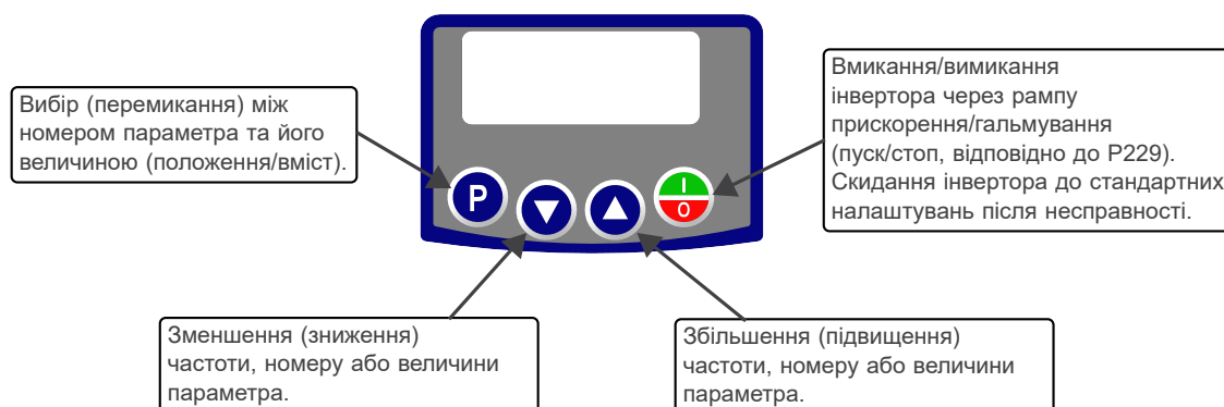
Малюнок 4.1: Кнопки інтерфейсу
