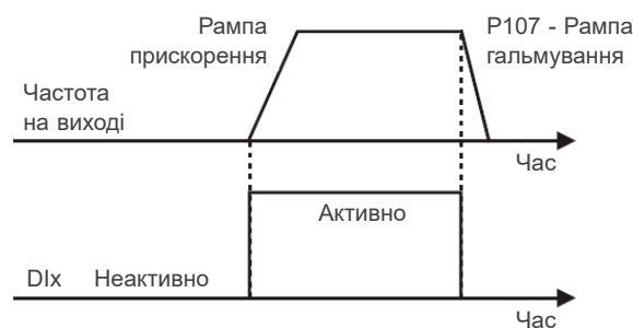
Малюнок 9.8: Приклад функції «Швидка зупинка»
