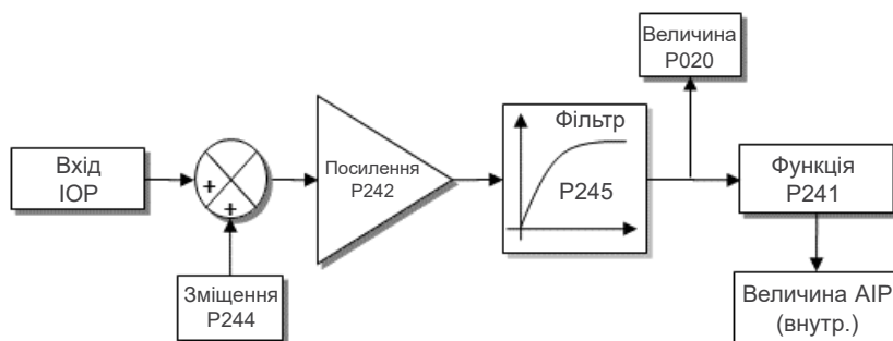
Малюнок 9.3: Блок-схема входу сигналу потенціометра AIP
