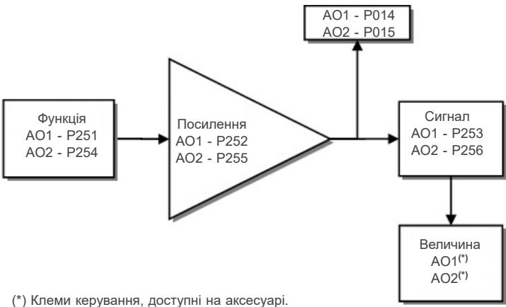
Малюнок 9.4: Блок-схема аналогового виходу (АОх)
