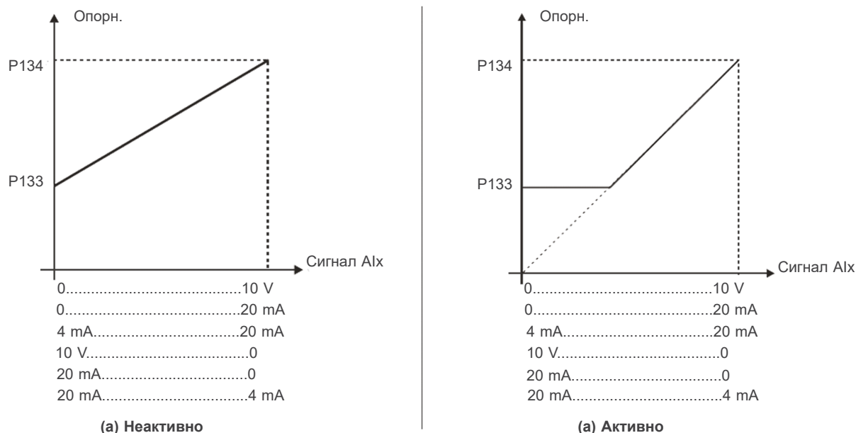
Малюнок 9.2: (а) і (б) Активація аналогових входів з мертвою зоною
