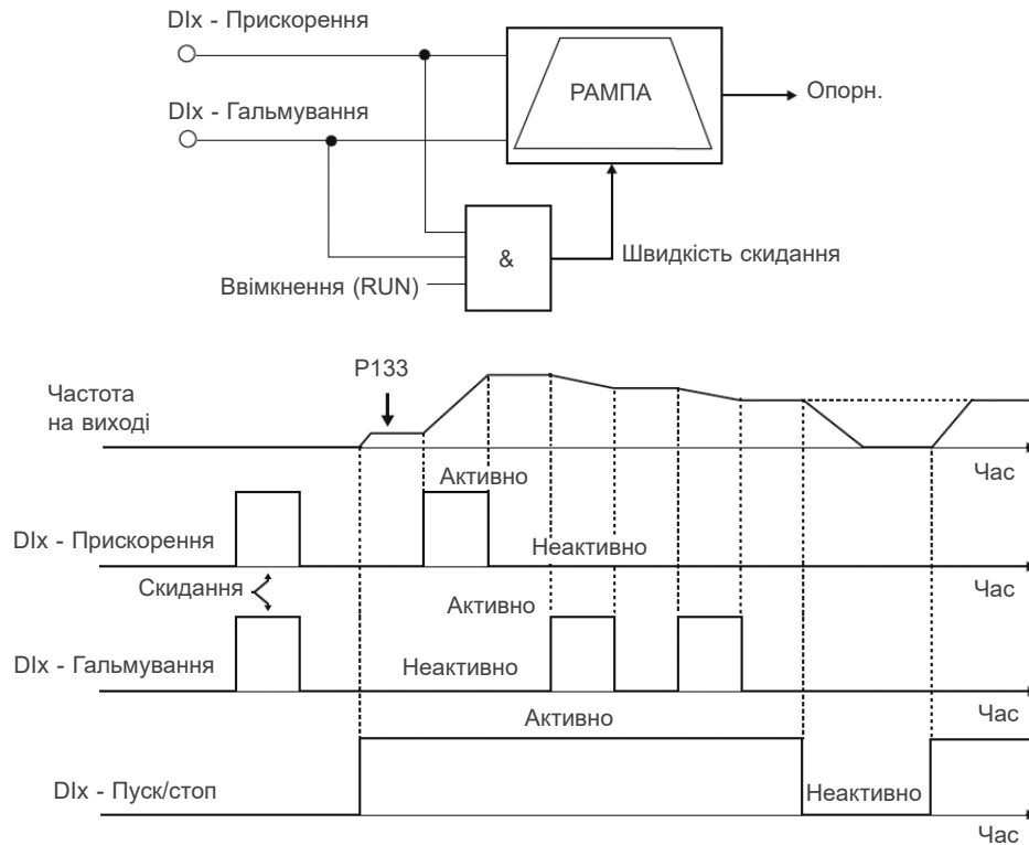
Малюнок 9.13: Приклад функції електронного потенціометра (Е.Р.)
