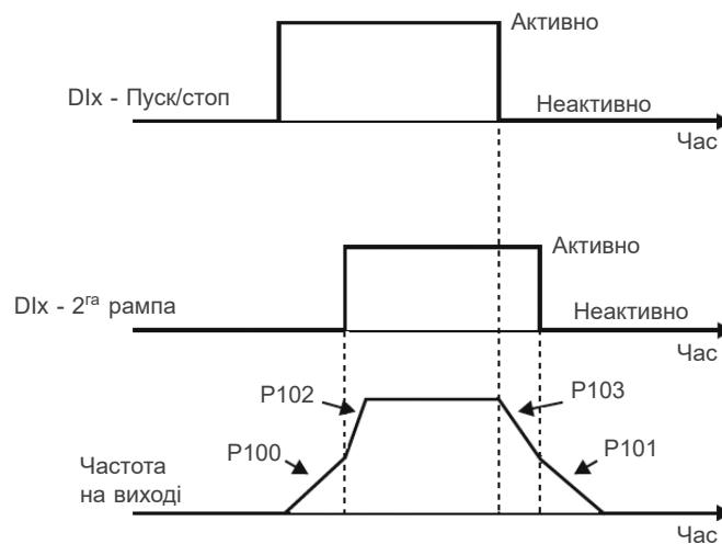
Малюнок 9.14: Приклад функції 2 ї рампи
