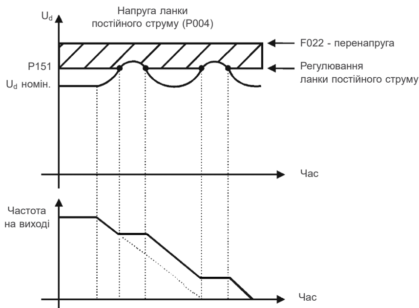
Малюнок 8.4: Приклад графіка обмеження напруги ланки постійного струму - Утримання рампи (P150 = 2 або 3)
