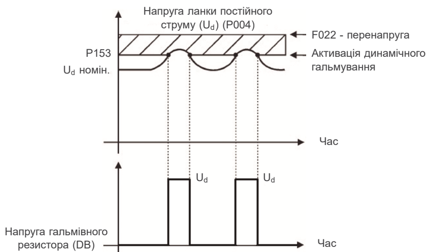
Малюнок 8.10: Крива активзації динамічного гальмування
