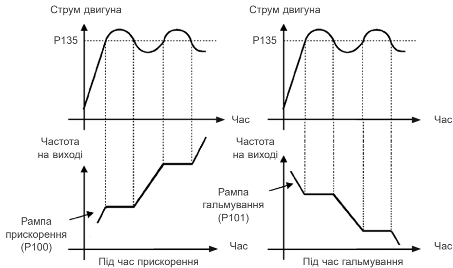
(а) "Рампа утримання"
