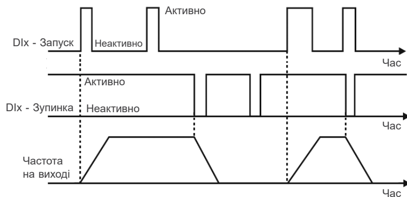
Малюнок 9.10: Приклад функції «Запуск/Зупинка»
