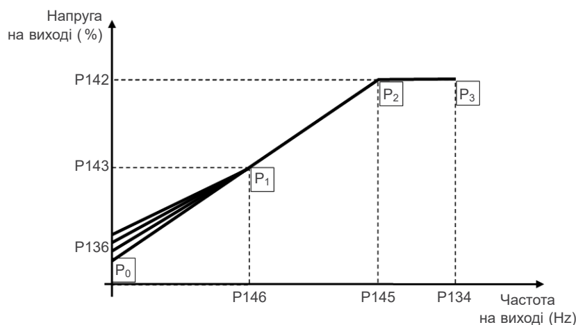
Малюнок 8.15: Регіон підсилення моменту обертання для квадратичного режиму V/f
