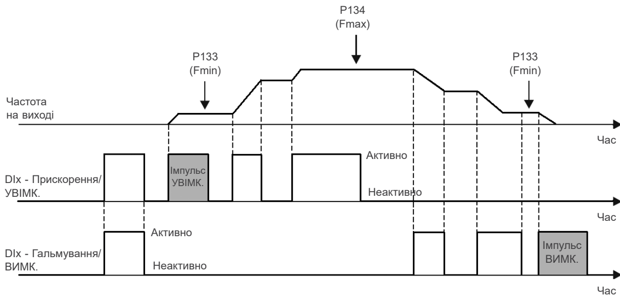
Малюнок 9.16: Приклад Прискорення УВІМК. / Гальмування ВИМК
