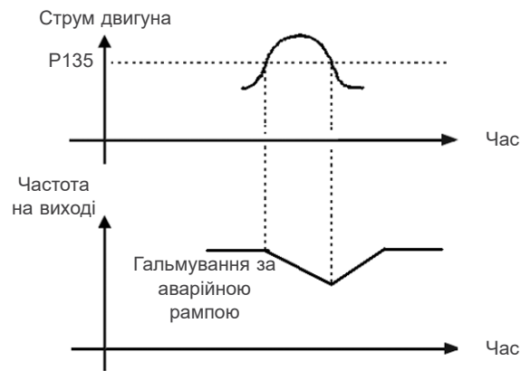
(b) "Рампа гальмування"
