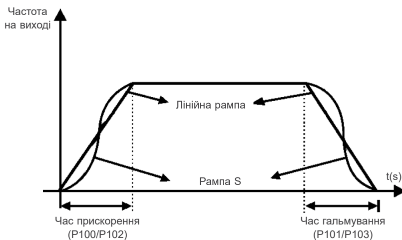
Малюнок 8.1: S або лінійна рампа
