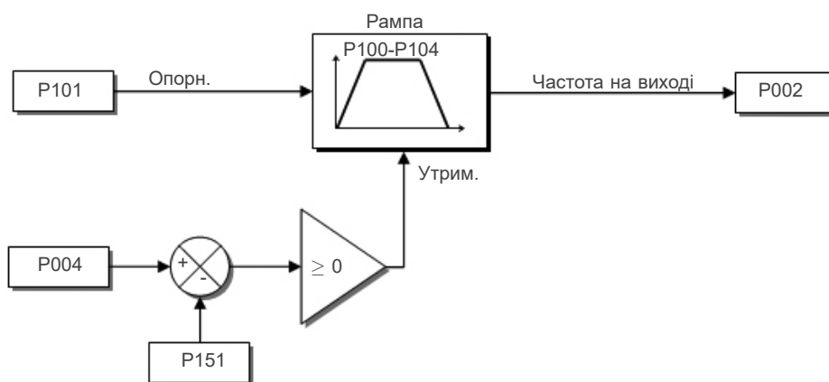
Малюнок 8.3: Блок-схема обмеження напруги ланки постійного струму
