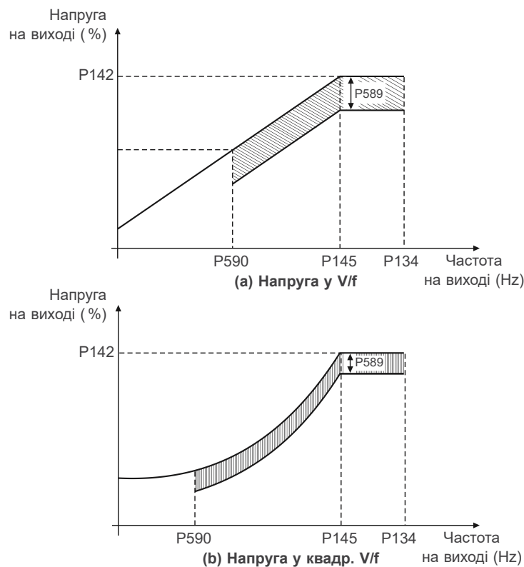
Малюнок 8.19: (a) і (b) Приклад поведінки напруги у V/f і квадратичному V/f
