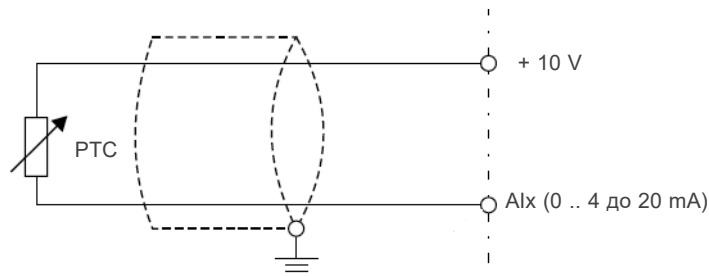
Малюнок 10.1: Підключення PTC до частотного інвертора
