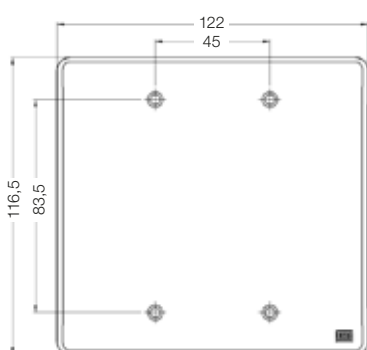
Placa 4x4 - Cega
