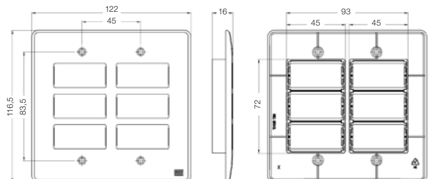
Placa 4x4 - 6 Posições
