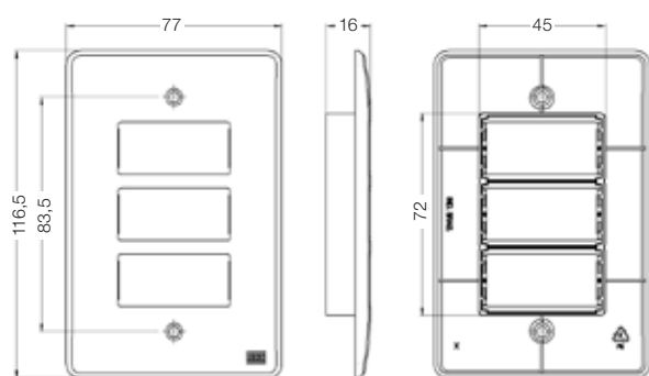
Placa 4x2 - 3 Posições
