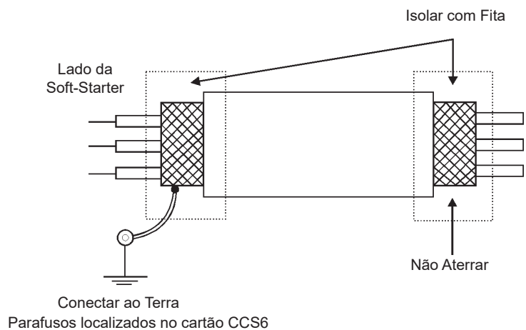
Figura 3.20 - Conexão blindagem
