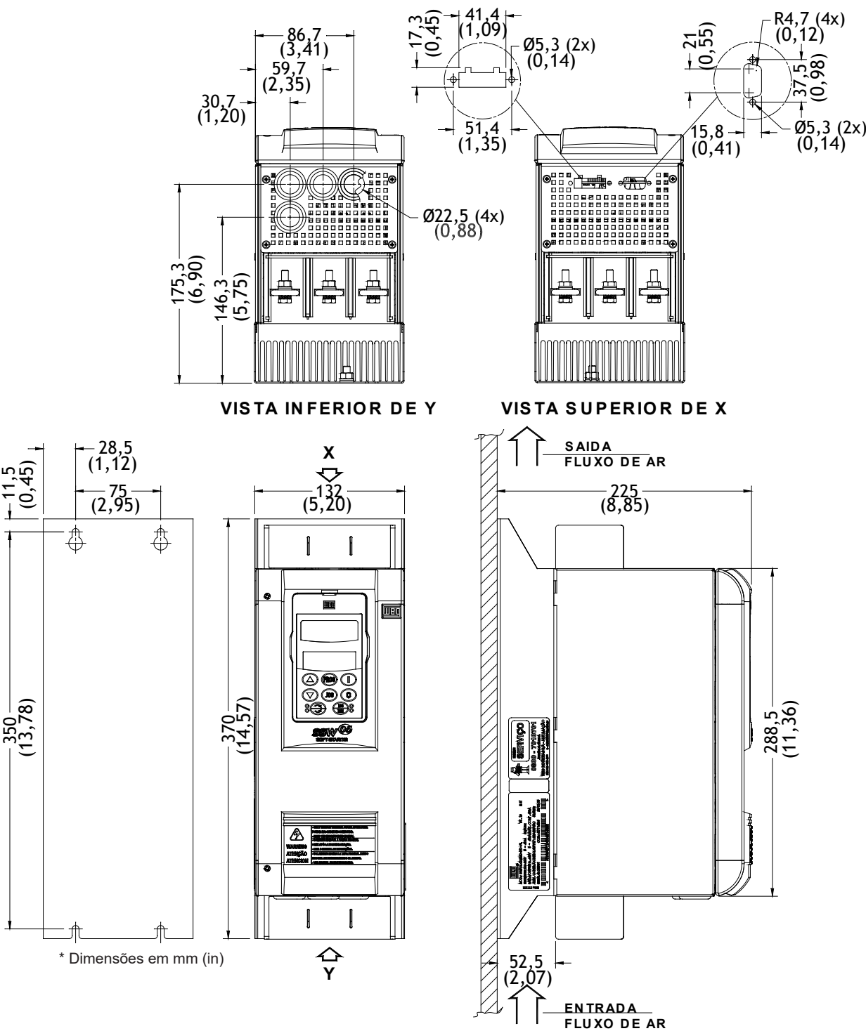
Figura 10.2 - Modelos de 45A a 130A (220-575V) ou 45A a 85A (575-690V)
