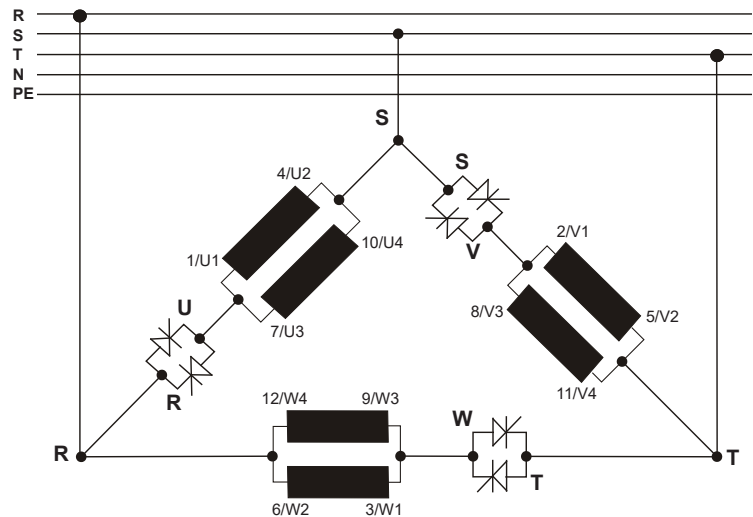
Figura 3.13 - Soft-Starter SSW-06 dentro da ligação delta do motor com motor de duplo delta em paralelo
