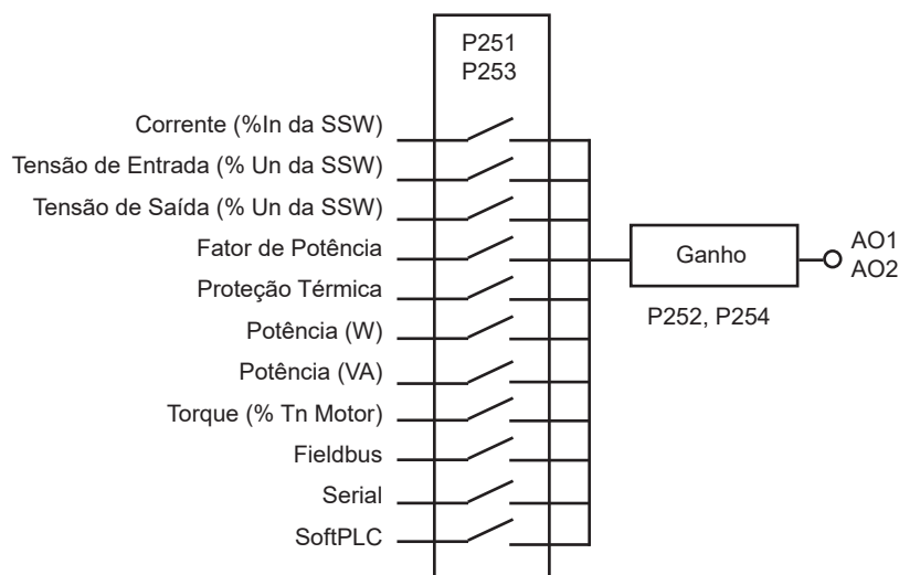
Figura 6.15 - Blocodiagrama das Saídas Analógicas
