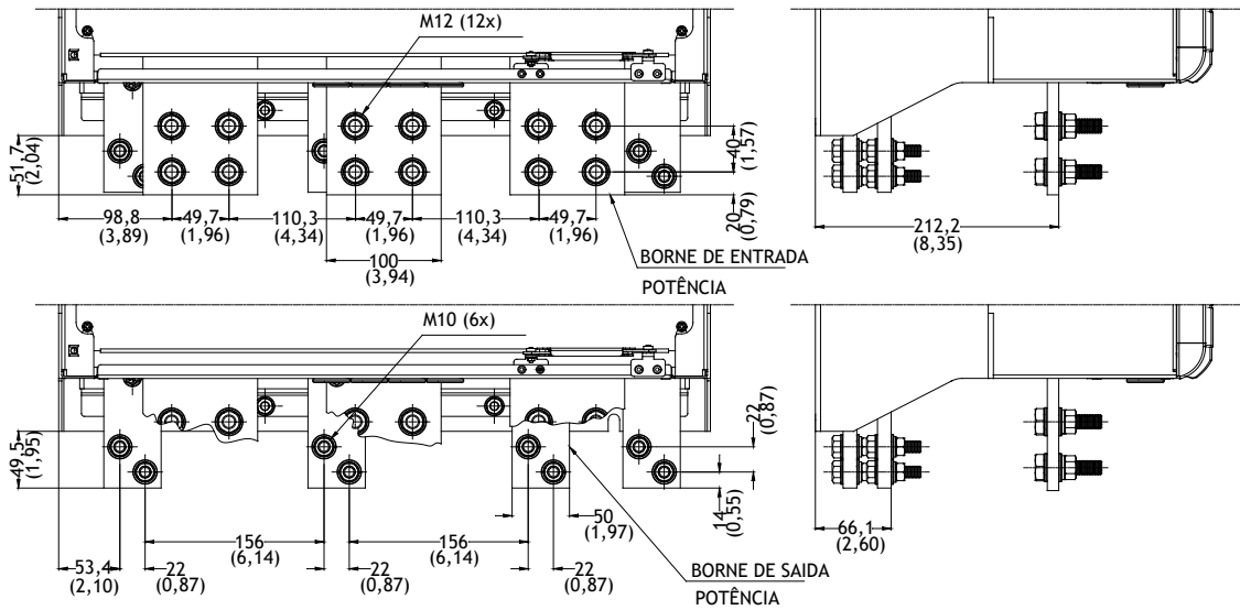
Figura 3.8 d) e) f) - Bornes de potência
