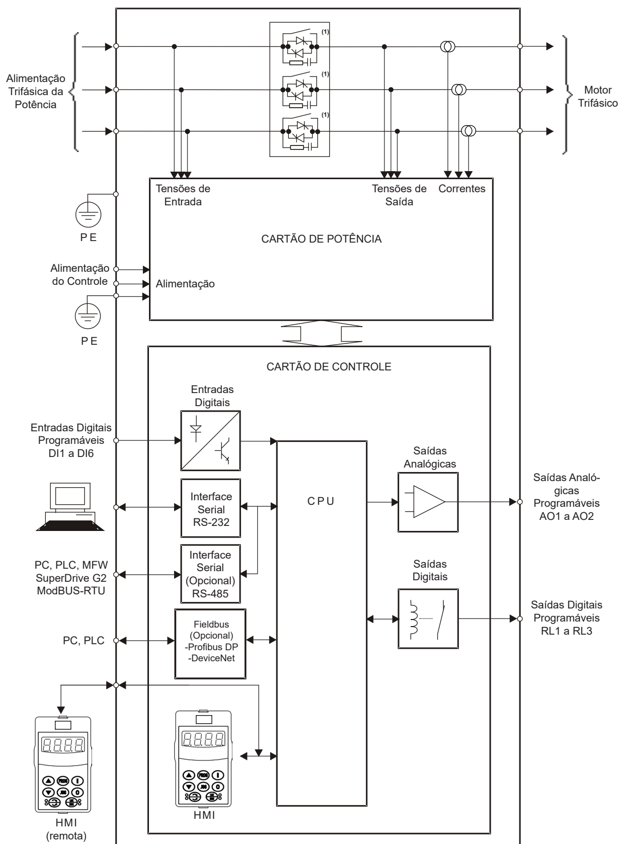
Figura 2.2 - Blocodiagrama da Soft-Starter SSW-06
