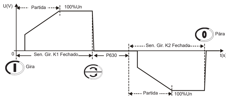
Figura 6.13 - Troca do sentido de giro via contator
