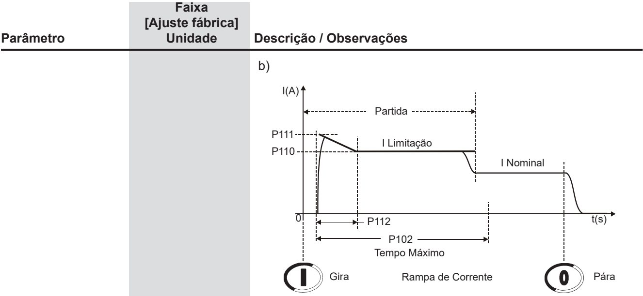
Figura 6.6 b) - Limite de corrente por Rampa de Corrente na partida
