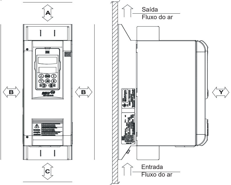
Figura 3.2 - Espaços livres para ventilação
