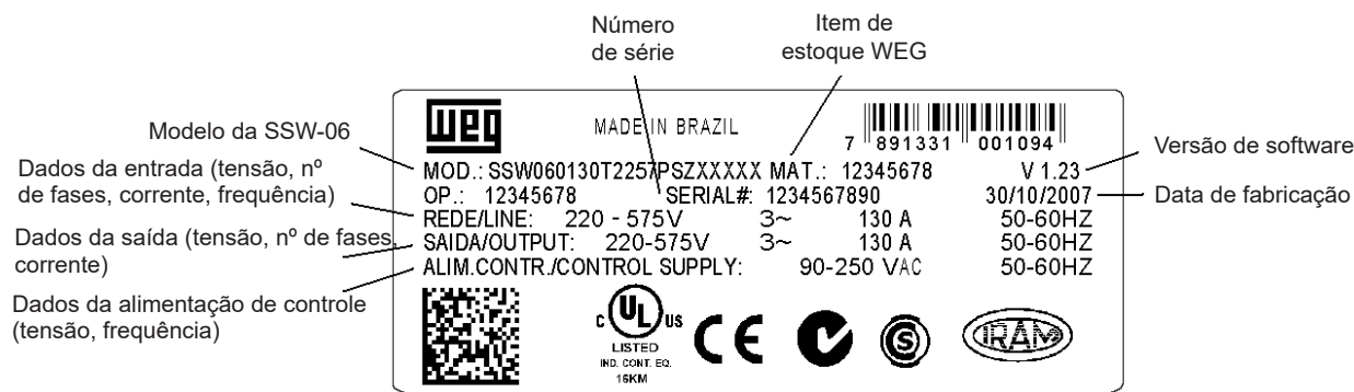
Figura 2.3 - Etiquetas de identificação da Soft-Starter SSW-06
