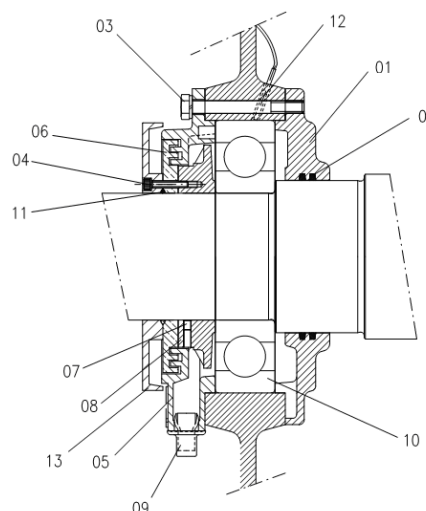
Figura 7.4: Partes do mancal de rolamento a graxa
