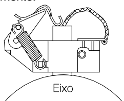
Figura 7.3: Escova para aterramento do eixo
