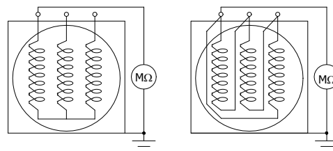
Figura 4.1: Conexão do megômetro
