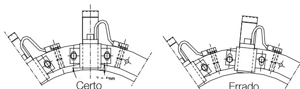
Figura 7.1: Montagem do porta-escovas.
