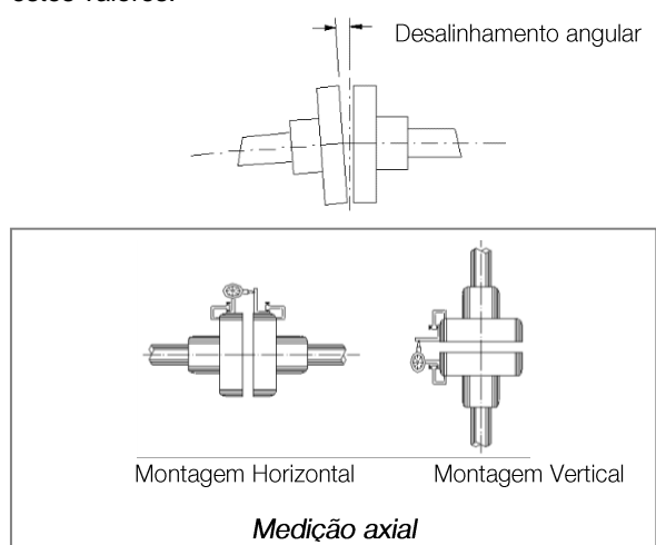
Figura 4.7: Alinhamento angular
