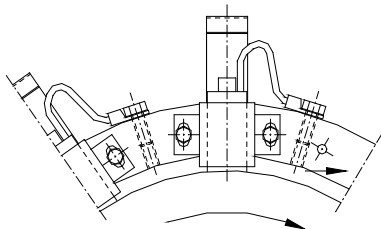
Figura 7.2: Assentamento das escovas.
