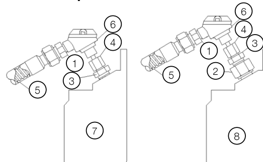
Figura 7.8: Pt100 nos mancais
