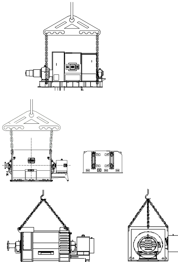
Figura 3.1: Manuseio dos motores
