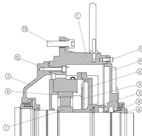
Figura 7.7: Partes do mancal de rolamento a óleo
