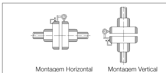
Figura 4.6: Alinhamento paralelo
