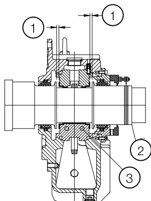
Figura 4.10: Mancais de deslizamento
