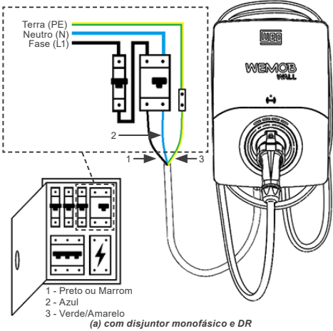
(a) com disjuntor monofásico e DR
