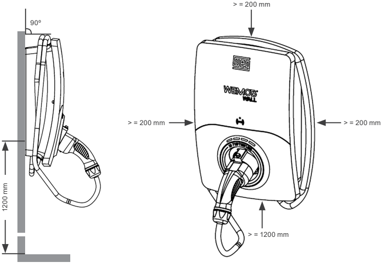
Figura 4.1: Posição de montagem e distanciamento da WEMOB-WALL
