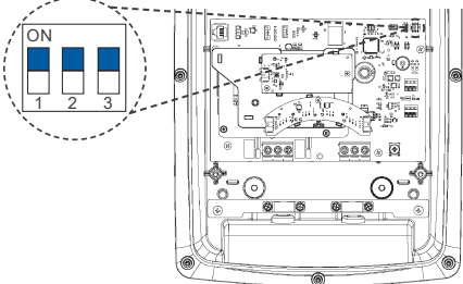
Figura 5.1: Llaves de selección de la corriente nominal
