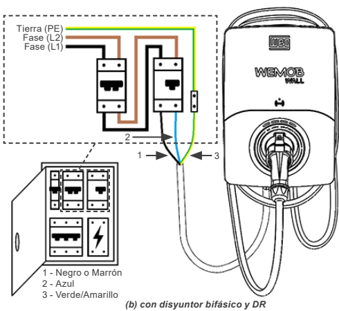
Figura 5.3: (a) y (b) ejemplos de conexión eléctrica monofásica (L1-N-PE) y bifásica (L1-L2-PE)
