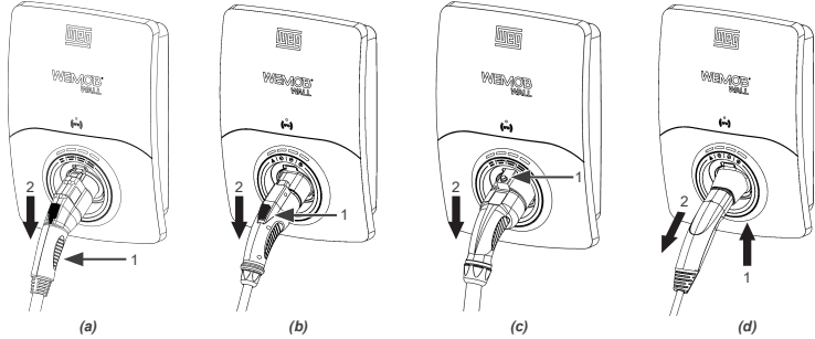
Figura 5.4: (a), (b), (c) e (d) Procedimento para retirada do plugue do soquete nas estações de recarga com cabos tipo 1, GB/T, tipo 2 e NACS
