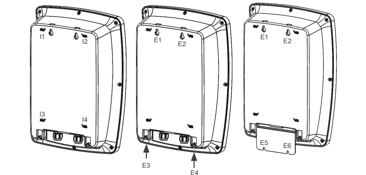
Figura 4.2: Métodos de fixação da WEMOB-WALL
