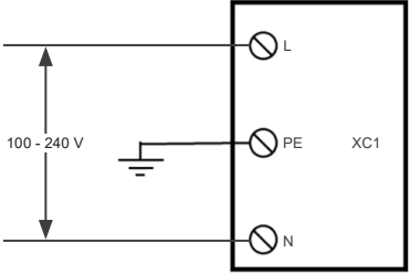
Figura 5.2: Ligação fiação interna
