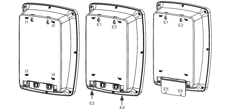
Figura 4.2: Métodos de fijación de la WEMOB-WALL
