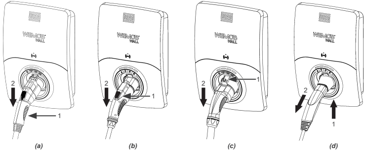
Figura 5.4: (a), (b), (c) y (d) procedimiento para retirada del plug del stecker en las estaciones de recarga con cables tipo 1, GB/T, tipo 2 y NACS
