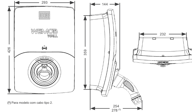
Figura 7.1: Dimensões da estação de recarga WEMOB-WALL em mm
