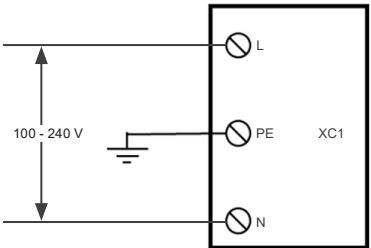
Figura 5.2: Conexión eléctrica interna
