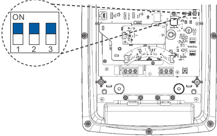
Figura 5.1: Chaves de seleção da corrente nominal
