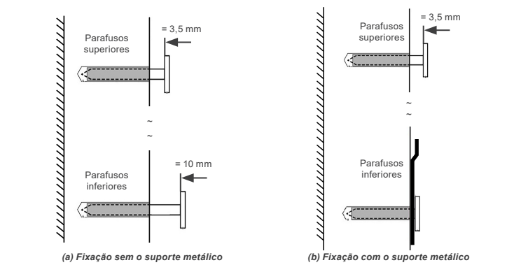
Figura 4.3: Formas de fixação externa
