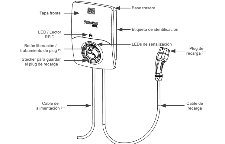
Figura 2.1: Visión general de la WEMOB-WALL
