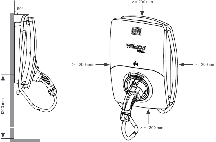
Figura 4.1: Posición de montaje y distanciamiento de la WEMOB-WALL
