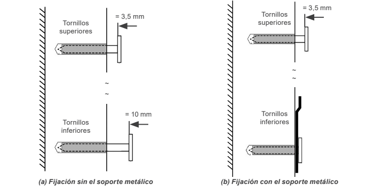
Figura 4.3: Formas de fijación externa
