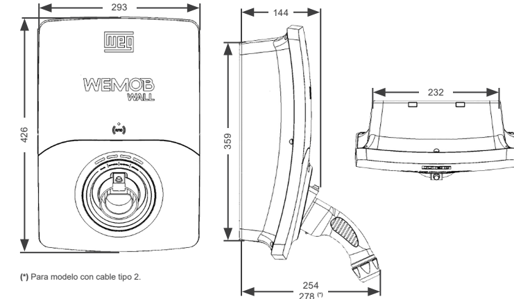
Figura 7.1: Dimensiones de la estación de recarga WEMOB-WALL en mm
