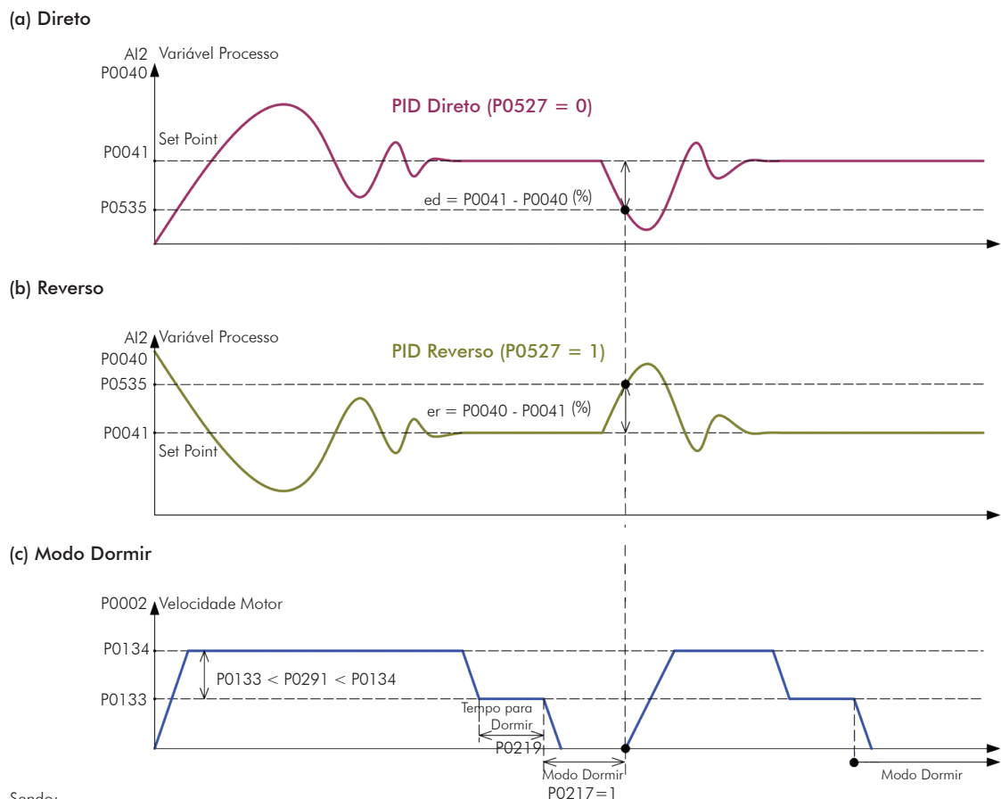
Figura 20.2 - (a) a (c) - Tipos de ação do PID
