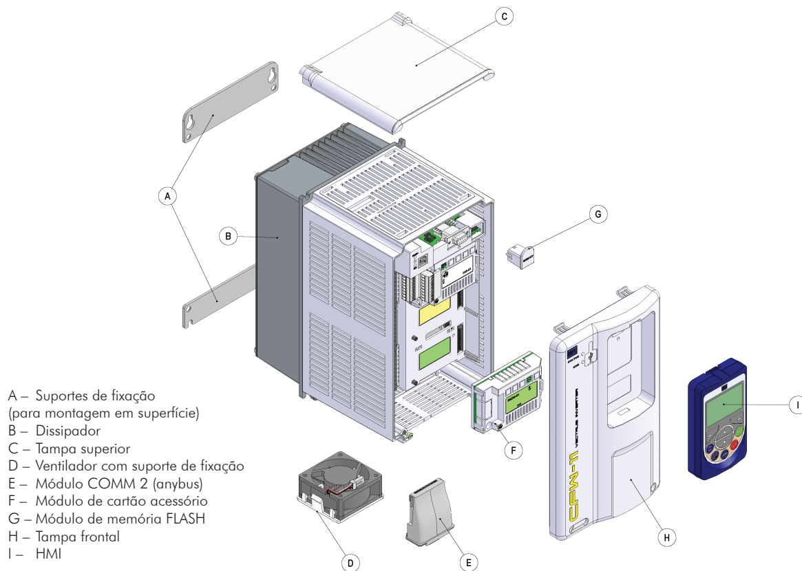
Figura 3.2 - Principais componentes do CFW-11
