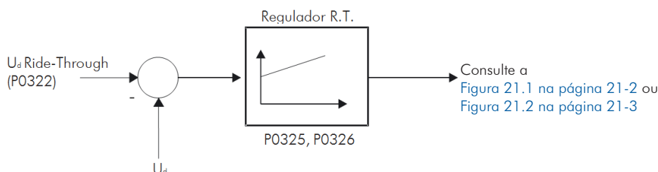
Figura 21.3 - Controlador PI do Ride-Through
