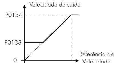
(a) Limites de velocidade considerando "Zona Morta" inativa (P0230 = 0)
