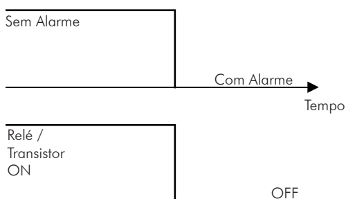
Figura 13.8 - (a) a (s) - Detalhes do funcionamento das funções das saídas digitais e a relé
