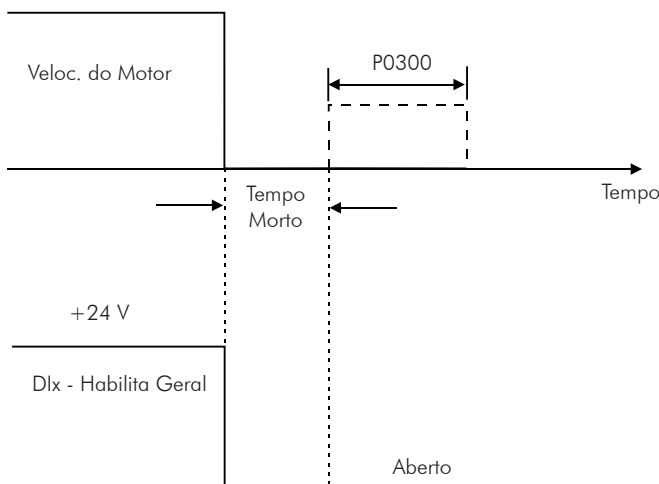
Figura 12.12 - Atuação da frenagem CC via Desabilita Geral - Modo V/f
