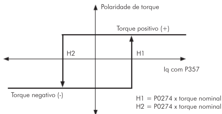
Figura 13.7 - Histerese para Corrente de Torque - Iq
