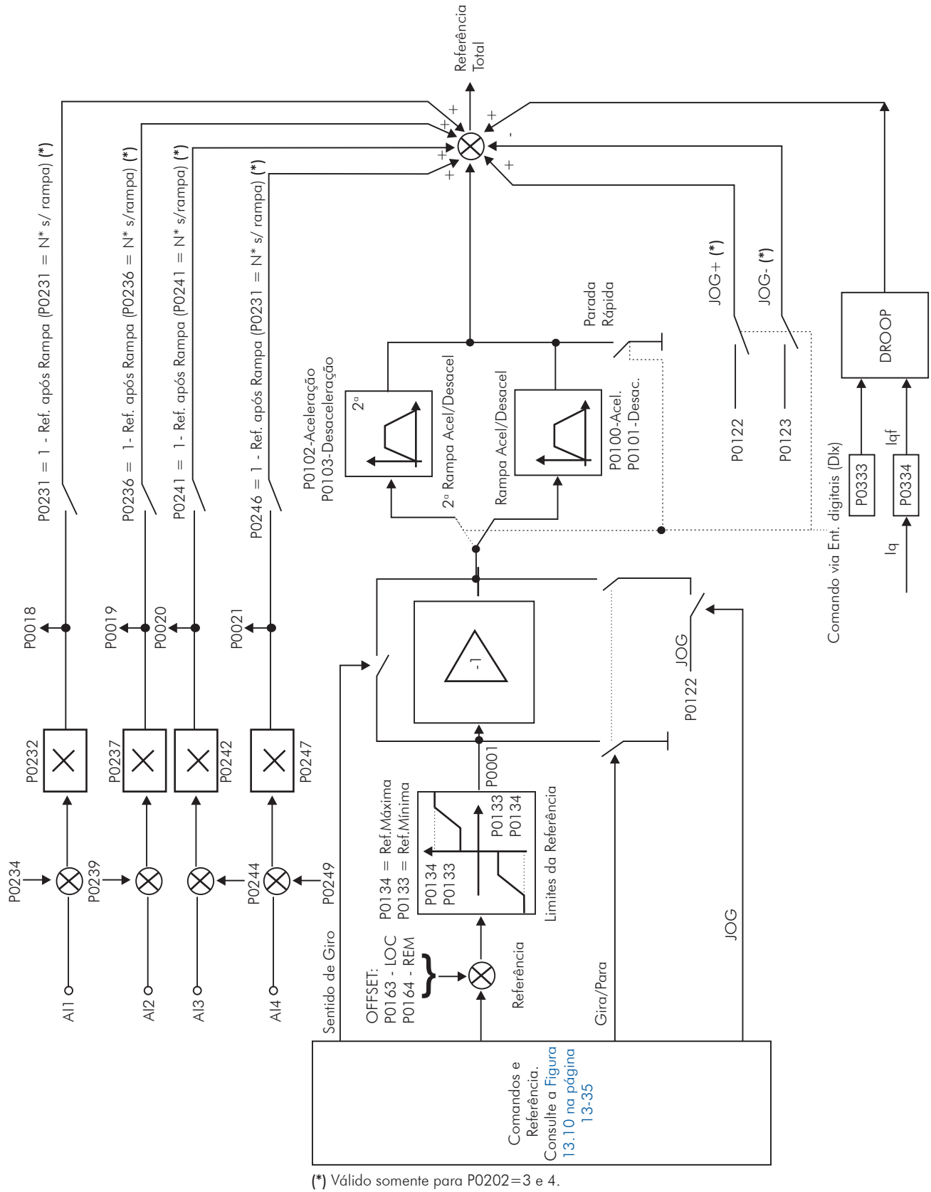
Figura 13.9 - Blocodiagrama da Referência de Velocidade
