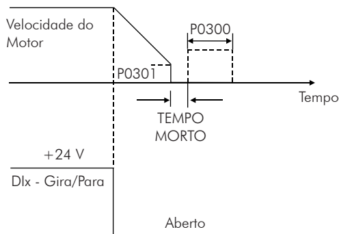
(a) Atuação da frenagem CC no bloqueio por rampa (via desabilita rampa)
