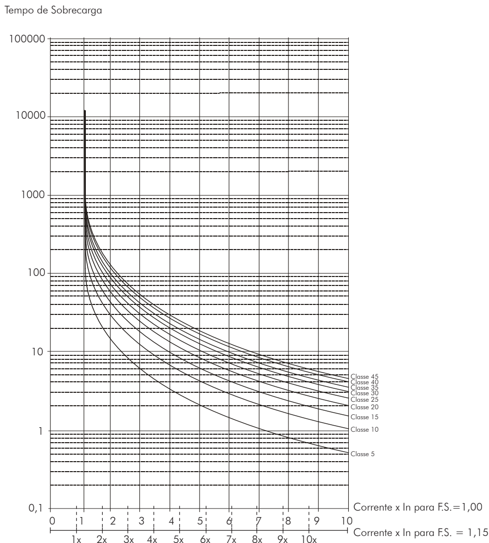
(b) Curvas de sobrecarga com o motor a quente para cargas do tipo HD e ND
