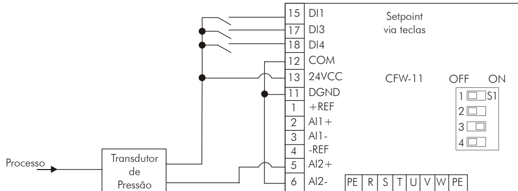
Figura 20.5 - Ligação de transdutor ao CFW-11 com 2 fios
