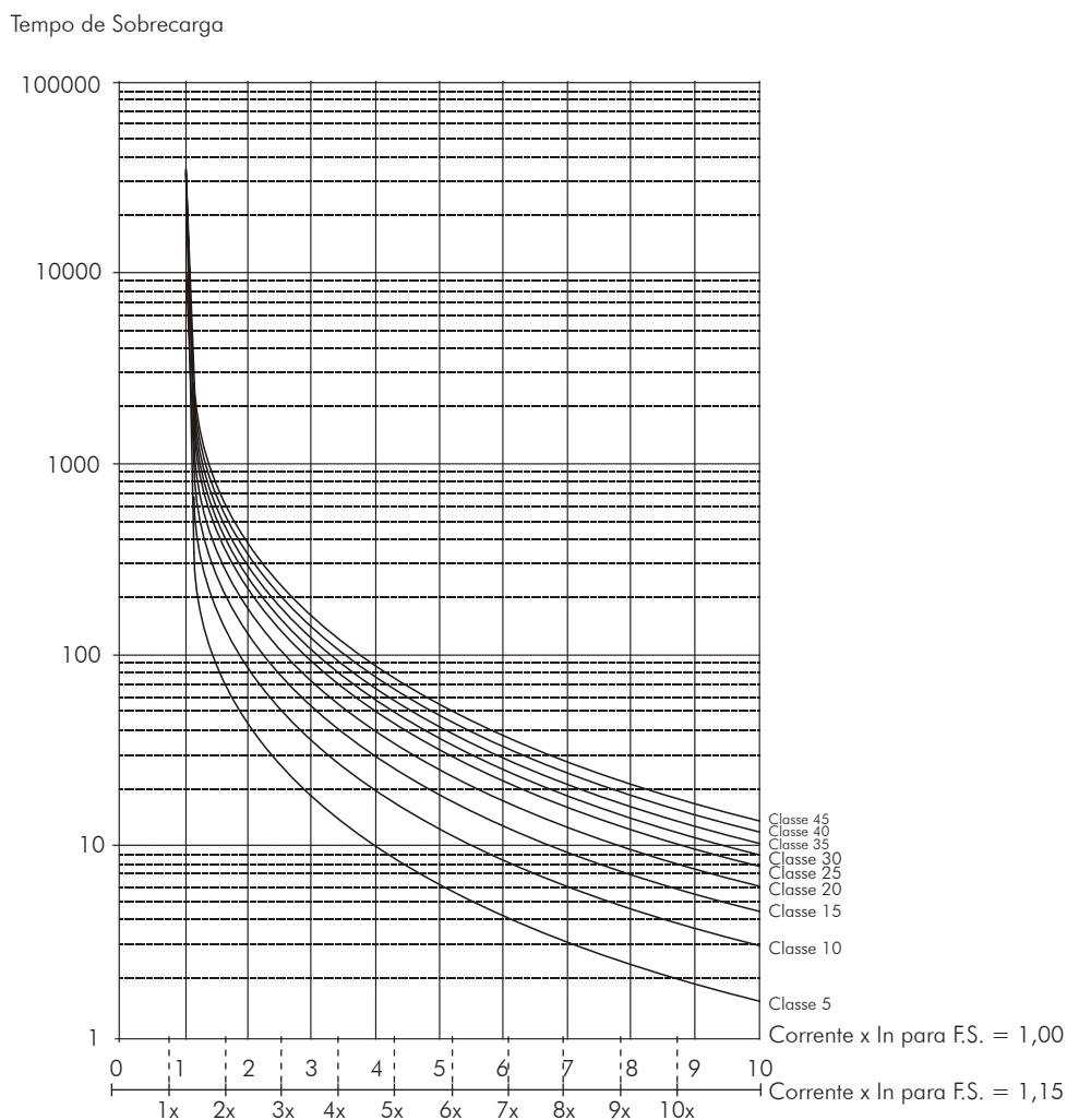
(a) Curvas de sobrecarga com o motor a frio para cargas do tipo HD e ND
