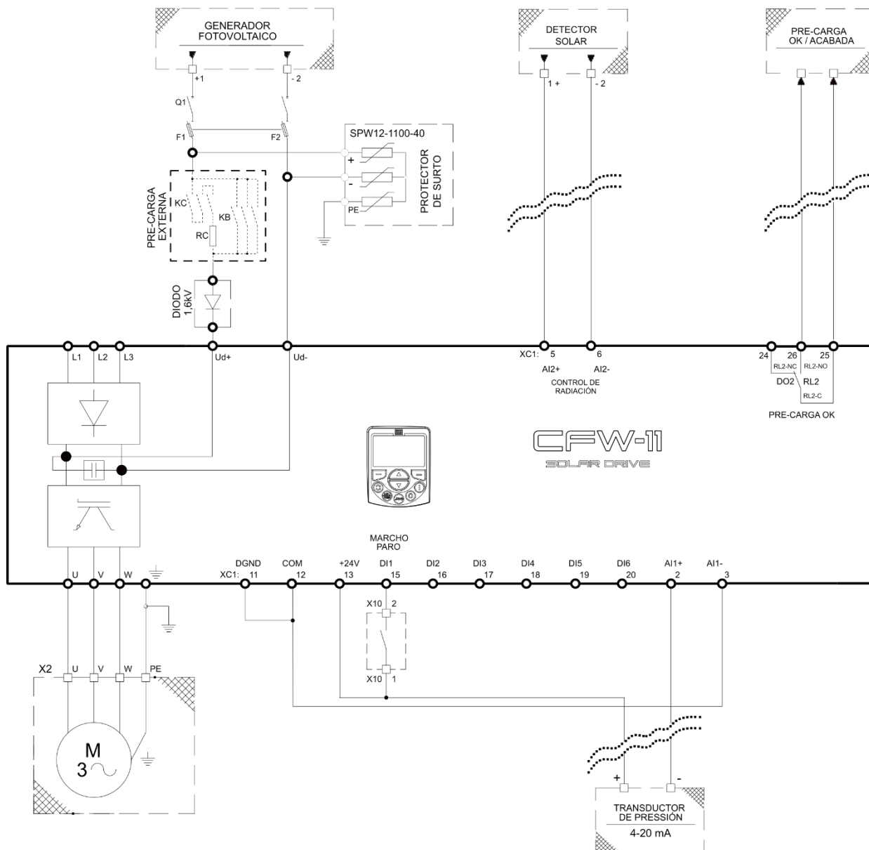
Figura 3.4 – Ejemplo de conexión del sistema fotovoltaico de bombeo de agua para CFW11 modelo T4
