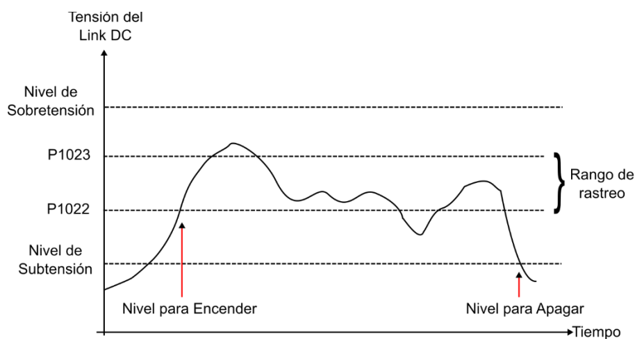
Figura 4.2 – Ajuste del rango de valores mínimos y máximos de rastreo del MPPT
