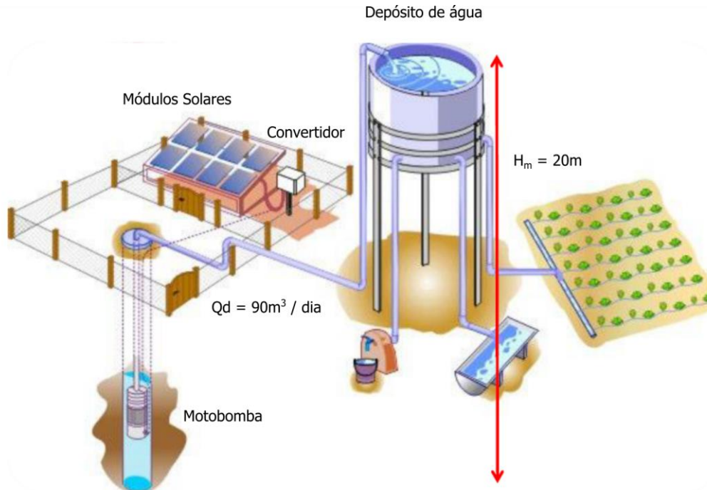
Figura 3.1 – Ejemplo de un sistema de bombeo solar
