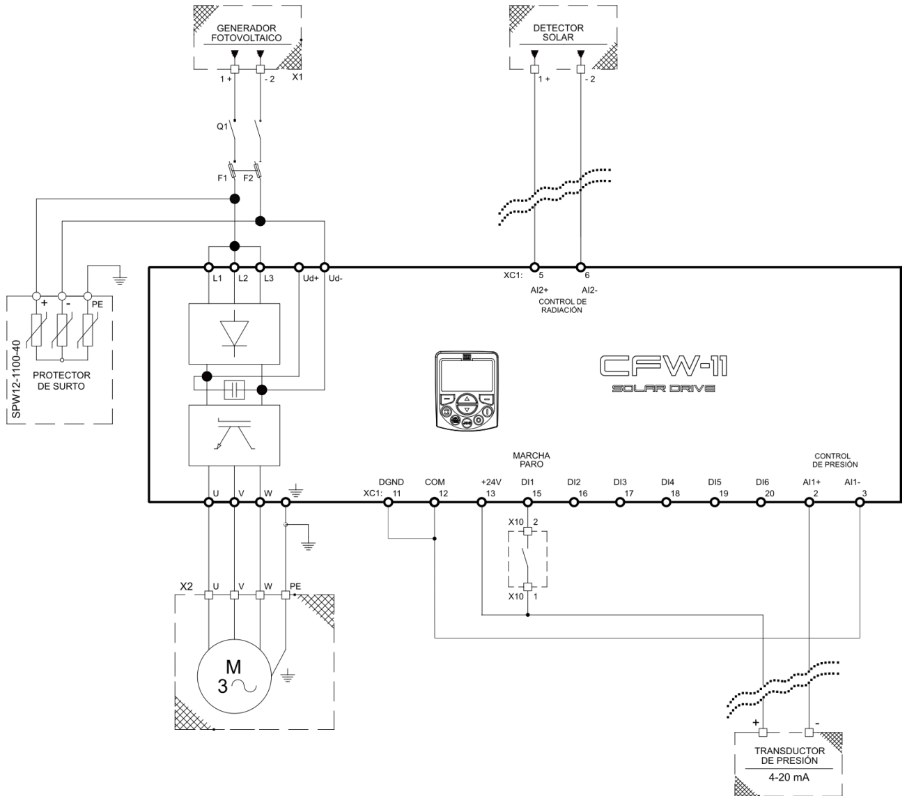
Figura 3.3 – Ejemplo de conexión del sistema fotovoltaico de bombeo de agua para CFW11 modelo T4
