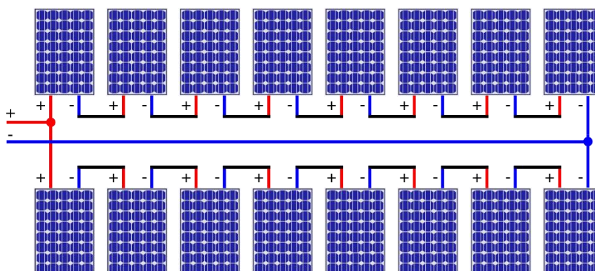
Figura 3.2 – Conexión de los módulos solares
