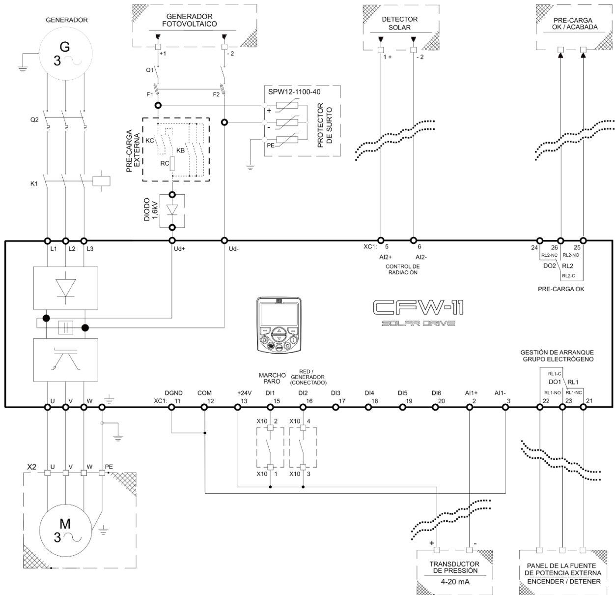
Figura 3.5 – Ejemplo de conexión del sistema fotovoltaico de bombeo de agua para CFW11 Modelo T4 con alimentación externa
