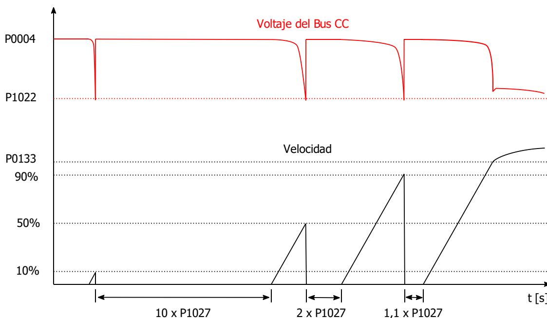
Figura 5.1 - Ejemplo: Ajuste automático del tiempo entre arranques
