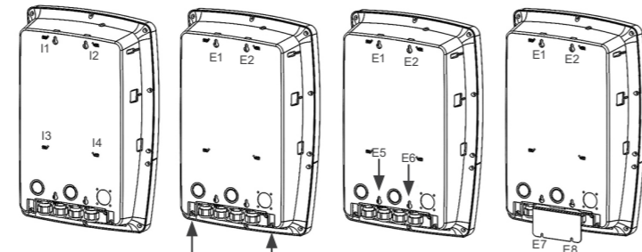
Figura 4.2: Métodos de fixação da WEMOB-PARKING
