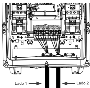
Figura 5.2: Montaje aparente de los cables de alimentación (lado 1 y 2)
