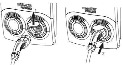
Figura 5.4: Procedimento para inserir o plugue no soquete
