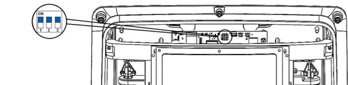
Figura 5.1: Chaves de seleção da corrente nominal
