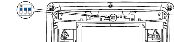
Figura 5.1: Llaves de selección de la corriente nominal
