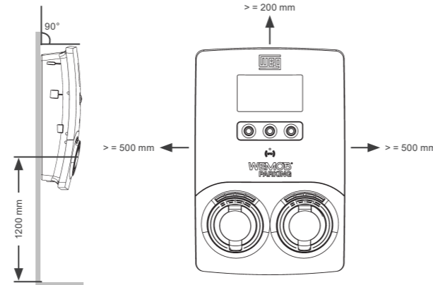
Figura 4.1: Posição de montagem e distanciamento da WEMOB-PARKING 2S2
