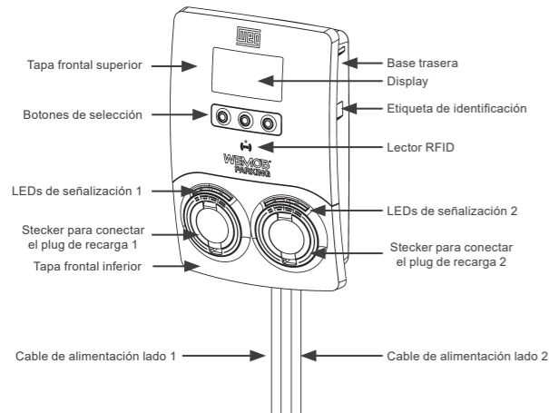
Figura 2.1: Visión general de la WEMOB-PARKING
