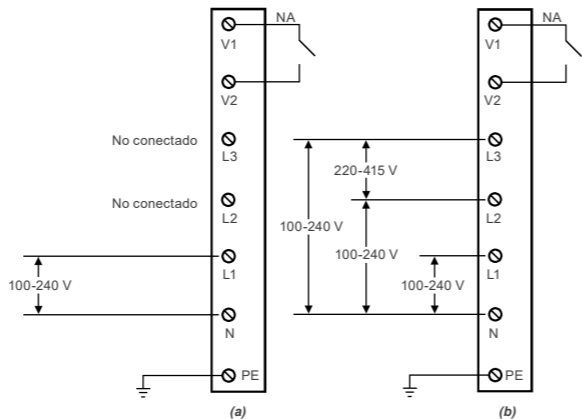
Figura 5.3: Ejemplos de conexión eléctrica: (a) monofásica o bifásica, (b) trifásica
