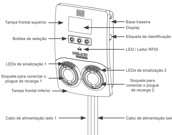
Figura 2.1: Visão geral da WEMOB-PARKING
