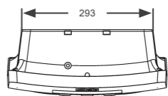
Figura 7.1: Dimensiones de la estación de recarga WEMOB-PARKING en mm
