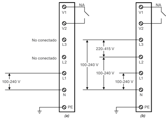
Figura 5.3: Exemplos de ligação elétrica: (a) monofásica ou bifásica, (b) trifásica
