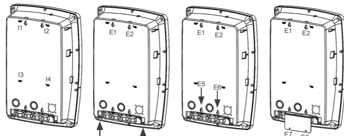
Figura 4.2: Métodos de fijación de la WEMOB-PARKING
