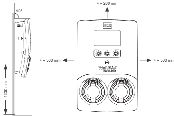
Figura 4.1: Posición de montaje y distanciamiento de la WEMOB-PARKING 2S2
