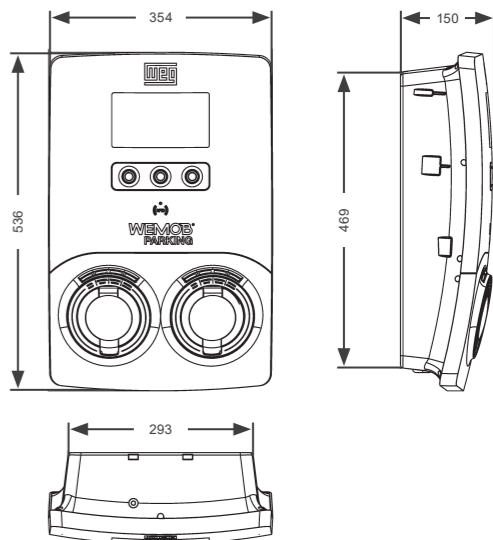
Figura 7.1: Dimensões da estação de recarga WEMOB-PARKING em mm
