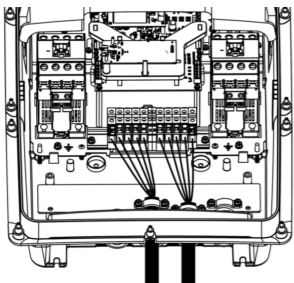
Figura 5.2: Montagem aparente dos cabos de alimentação (lado 1 e 2)
