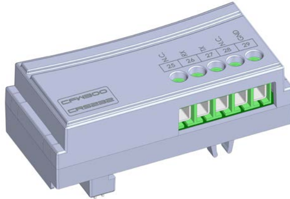
Figura 2.3: Módulo com conexão RS232
