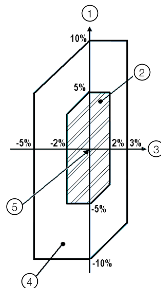
Figura 2.1: Limites das variações da tensão e frequência
