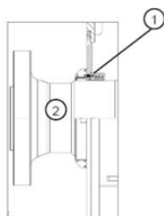
Figura 8.1: Medição entreferro
