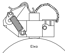
Figura 7.1: Escova para aterramento do eixo
