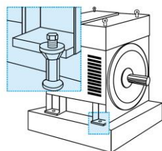
Figura 4.9: Chumbadores
