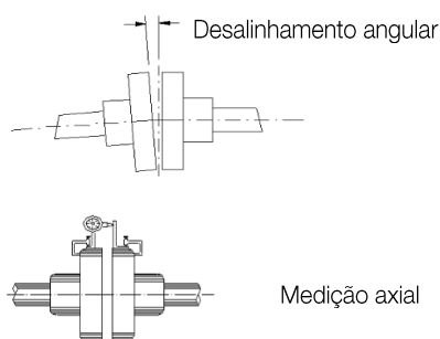
Figura 4.11: Alinhamento angular
