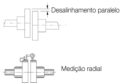
Figura 4.10: Alinhamento paralelo
