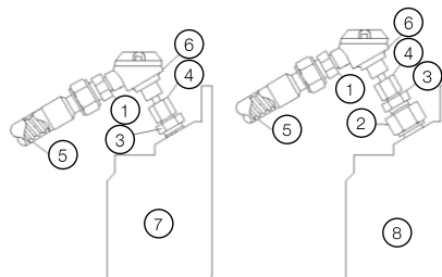
Figura 7.8: Pt100 nos mancais
