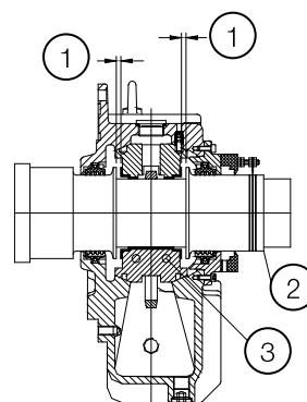
Figura 4.15: Mancal de deslizamento
