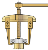
Figura 7.6: Dispositivo para sacar o rolamento
