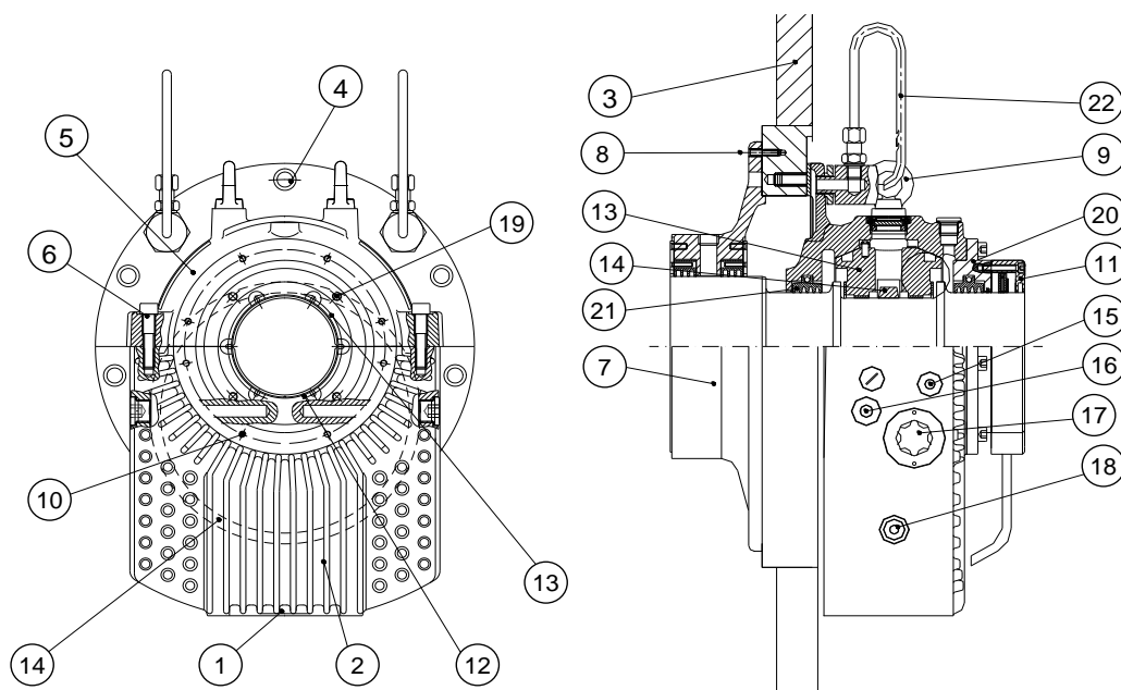
Figura 7.7: Partes do mancal de deslizamento
