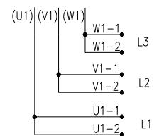
Figura 4.5: Conexões paralelas
