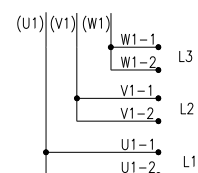
Figura 4.6: Conexões paralelas
