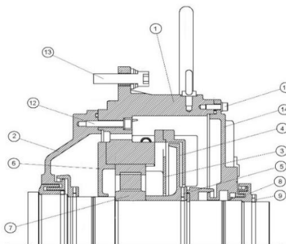
Figura 7.5: Partes do mancal de rolamento a óleo
