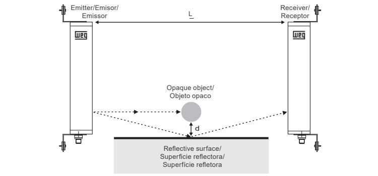
Figura A.5: Exemplos de aplicações usando espelhos
