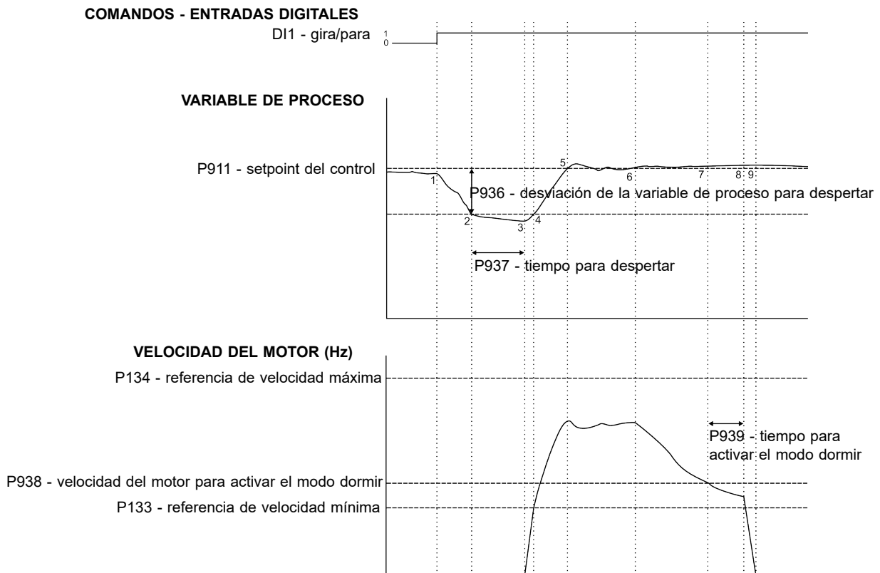
Figura 14.4: Funcionamiento del controlador PID con modo dormir habilitado
