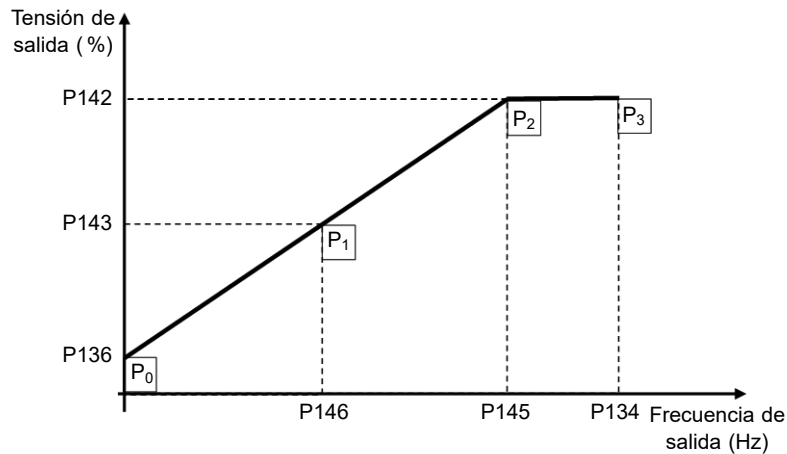
Figura 8.13: Curva V/f
