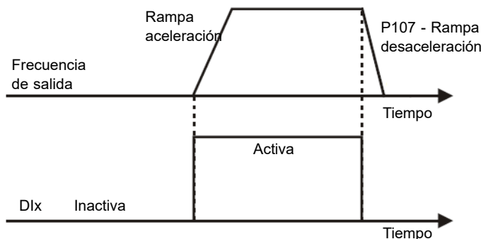
Figura 9.8: Ejemplo de la función Parada Rápida
