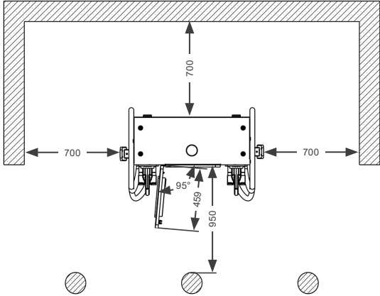
Figura 4.5: Distanciamento mínimos recomendados para fixação da WEMOB-STATION no totem - mm
