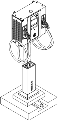
Figura 4.10: Exemplo fixação da estação WEMOB-STATION (60/80 kW) no totem
