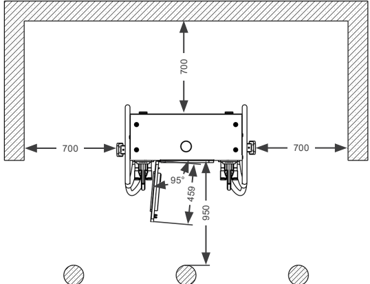
Figura 4.5: Distancia mínima recomendada para fijación de la WEMOB-STATION al tótem - mm
