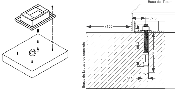
Figura 4.8: Detalles de los puntos de fijación - mm
