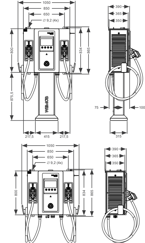
Figura 7.1: Dimensões da estação de recarga WEMOB-STATION – mm
