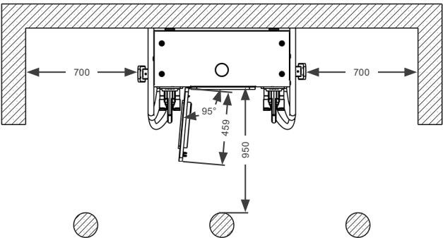
Figura 4.4: Distancia mínima para fijación de la WEMOB-STATION a la estructura de concreto - mm
