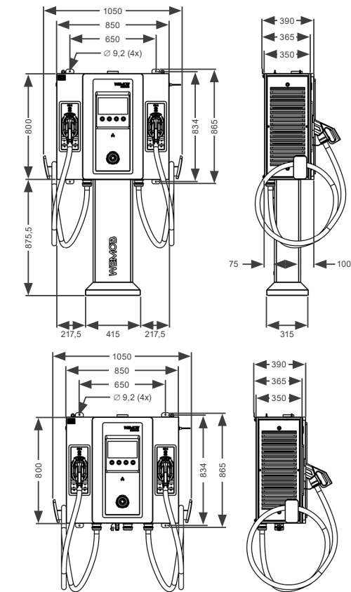
Figura 7.1: Dimensiones de la WEMOB-STATION en mm
