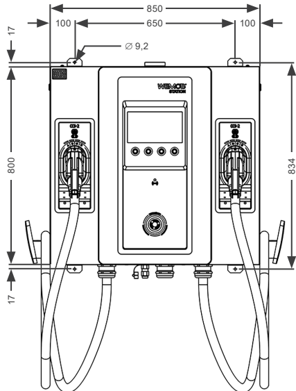
Figura 4.6: Dimensões da WEMOB-STATION (60/80 kW) para a fixação à estrutura de concreto - mm
