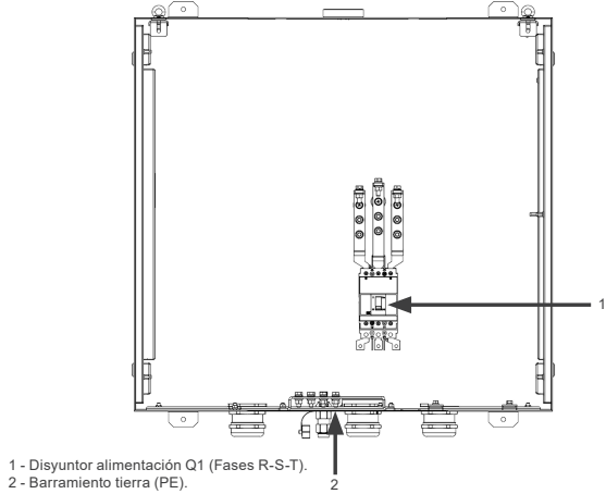
Figura 5.2: Conexiones de los cables de alimentación - Fases (R-S-T) y puesta a tierra (PE)
