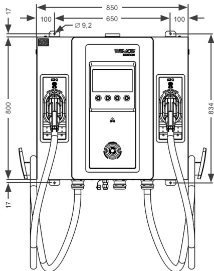
Figura 4.6: Dimensiones de la WEMOB-STATION (60/80 kW) para la fijación en la estructura de concreto - mm
