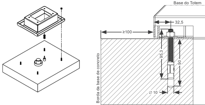
Figura 4.8: Detalhes dos pontos de fixação - mm
