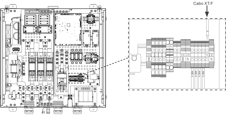
Figura 5.3: Ajuste de la tensión de la red de alimentación
