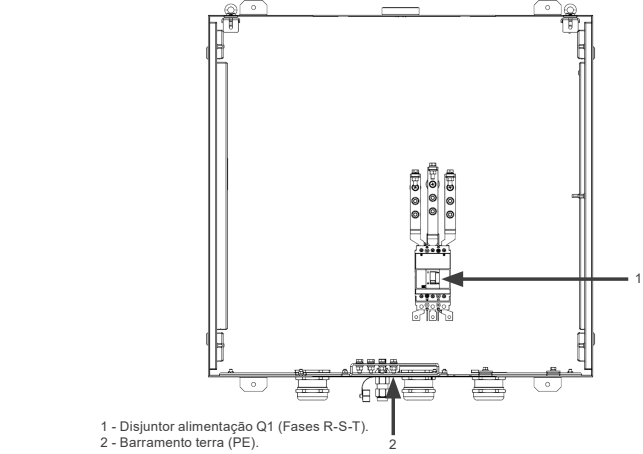
Figura 5.2: Conexões dos cabos de alimentação - Fases (R-S-T) e aterramento (PE)
