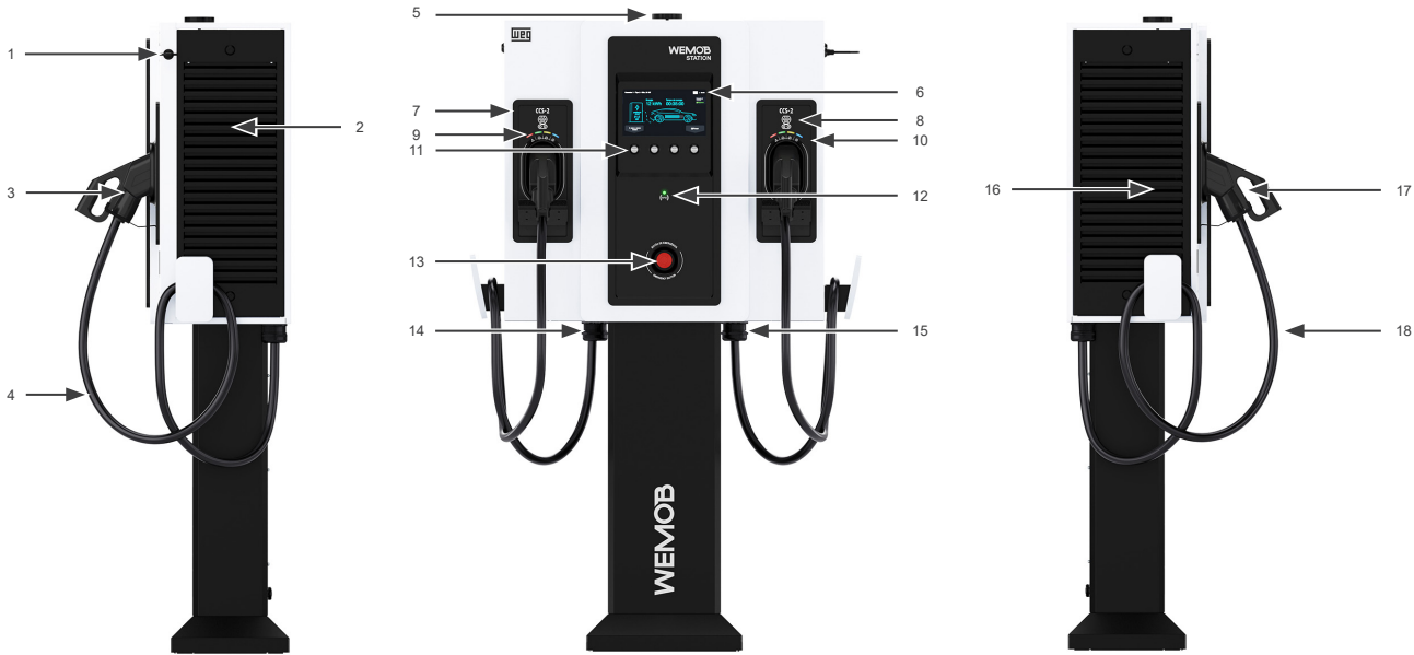
Figura 2.1: Visão geral da estação de recarga WEMOB-STATION (60/80 kW)
