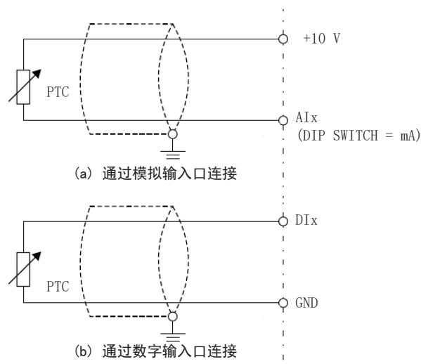
图18.3: (a) 和 (b) - PTC与MW500的接线
