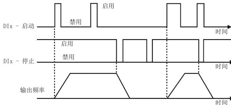
图15.10: 三线启动/停止功能示例
