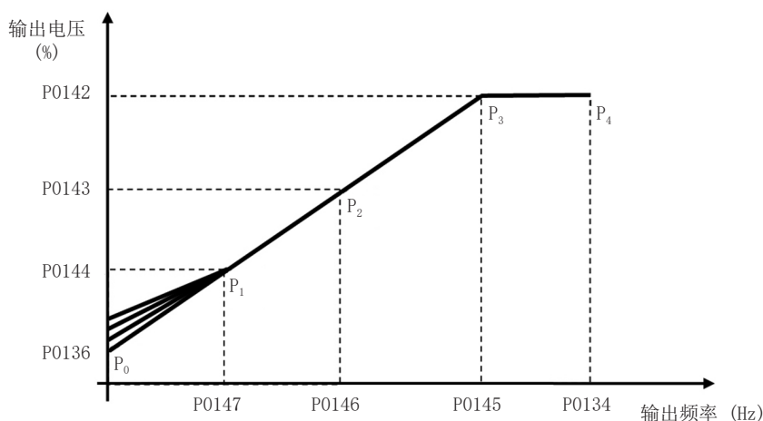
图9.3: 转矩提升区
