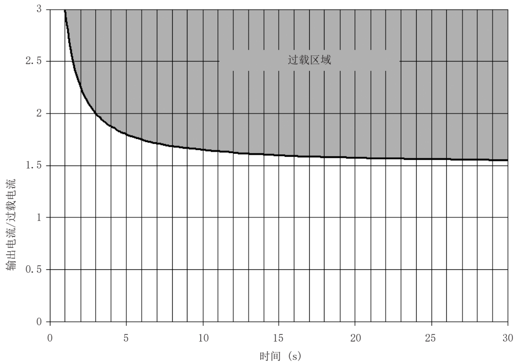
图18.2: IGBT过载的致动
