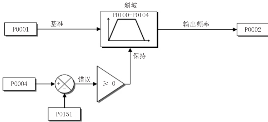
图9.5: DC Link限压框图 - 斜坡保持
