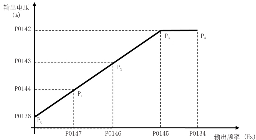
图9.2: V/f曲线
