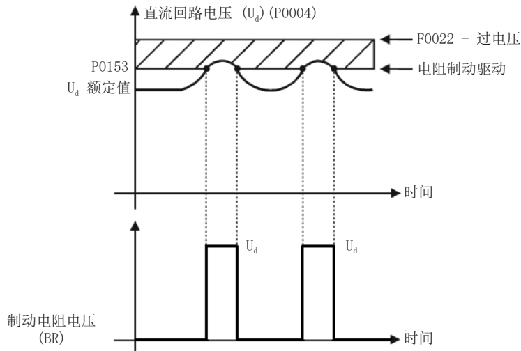
图17.1: 变频制动的动作曲线
