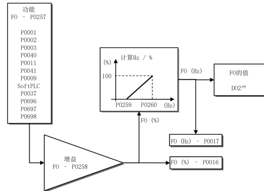
图15.5: 频率输出FO (DO2) 的框图
