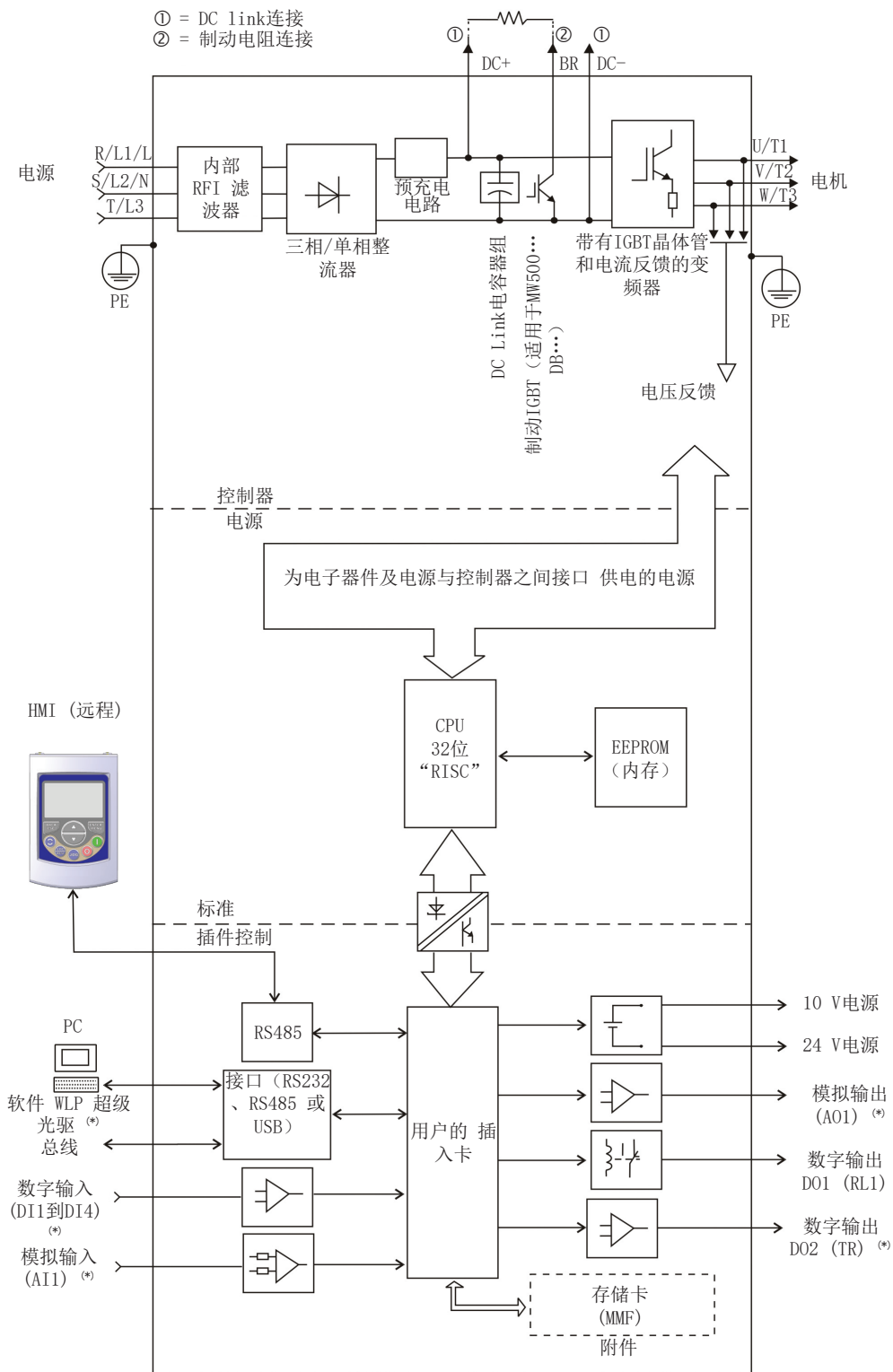
图3.1: MW500框图
