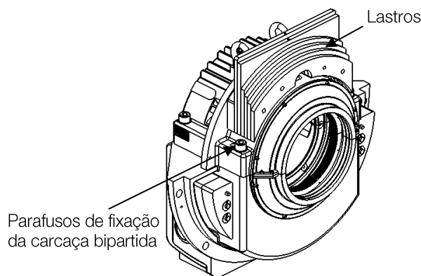
Figura 8.4: Mancal dianteiro com lastros
