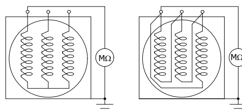
Figura 4.1: Conexão do megômetro
