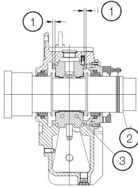
Figura 4.9: Mancal de deslizamento
