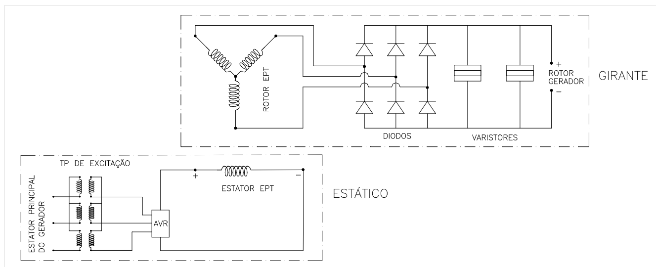
Figura 5.2: Circuitos elétricos internos do gerador sem PMG
