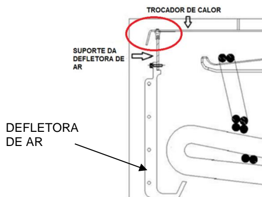
Figura 8.2: Montagem correta do trocador de calor
