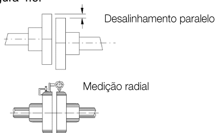
Figura 4.5: Alinhamento paralelo
