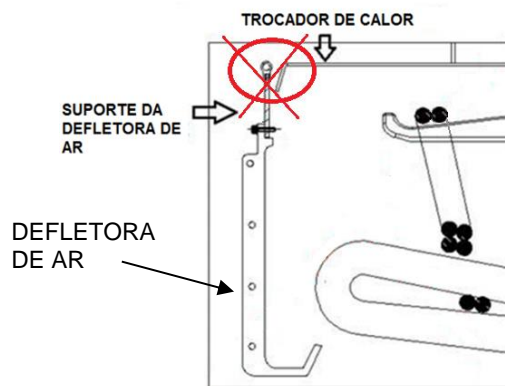
Figura 8.3: Montagem incorreta do trocador de calor
