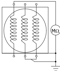
Figura 4.2: Conexão do megômetro em fases separadas
