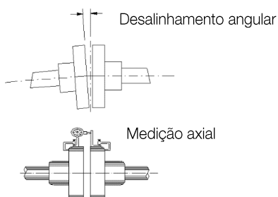
Figura 4.6: Alinhamento angular
