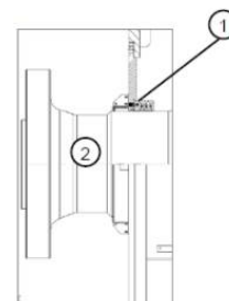
Figura 8.5: Medição entreferro
