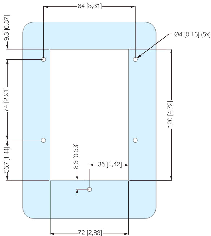
Dimensions/Dimensiones/Dimensões mm [in]
