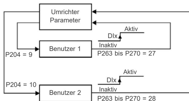
Abbildung 9.15: Das Blockdiagramm der Funktionen lädt Benutzer 1 und Benutzer 2
