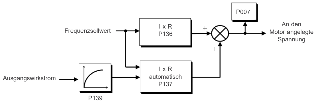
Abbildung 8.17: Blockschaltbild der automatischen Drehmomentanhebung
