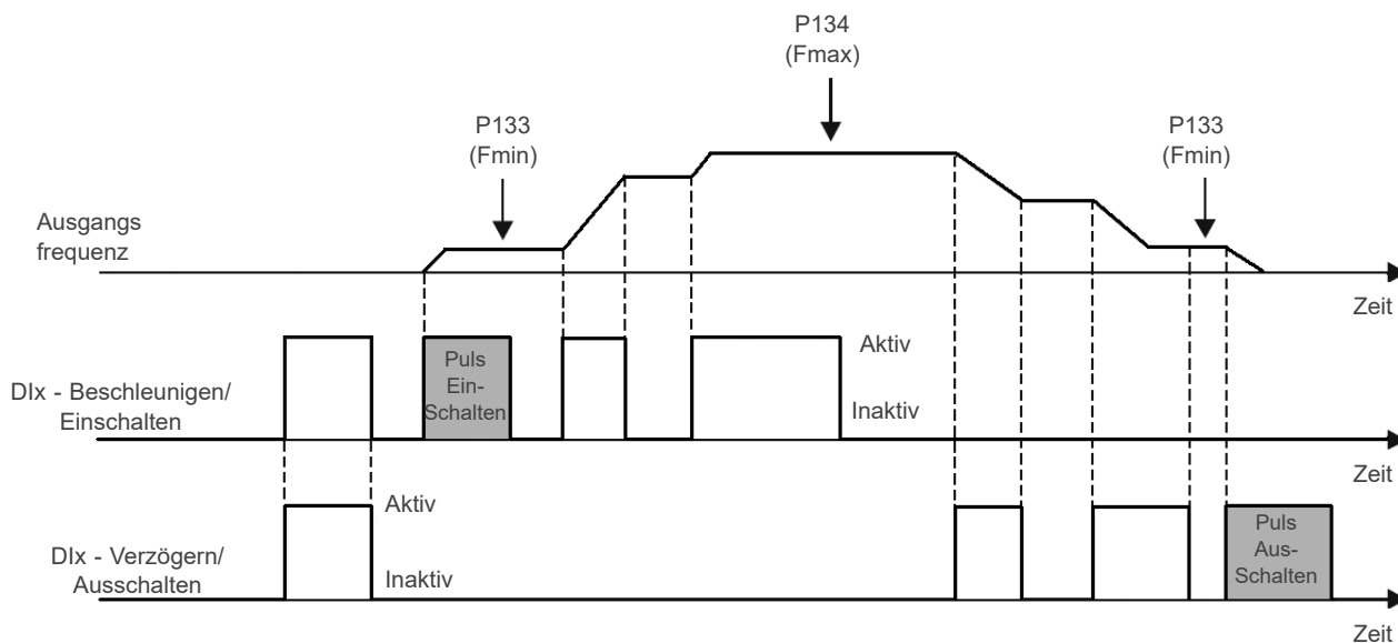
Abbildung 9.16: Beispiel von Beschleunigen Einschalten / Verzögern Ausschalten
