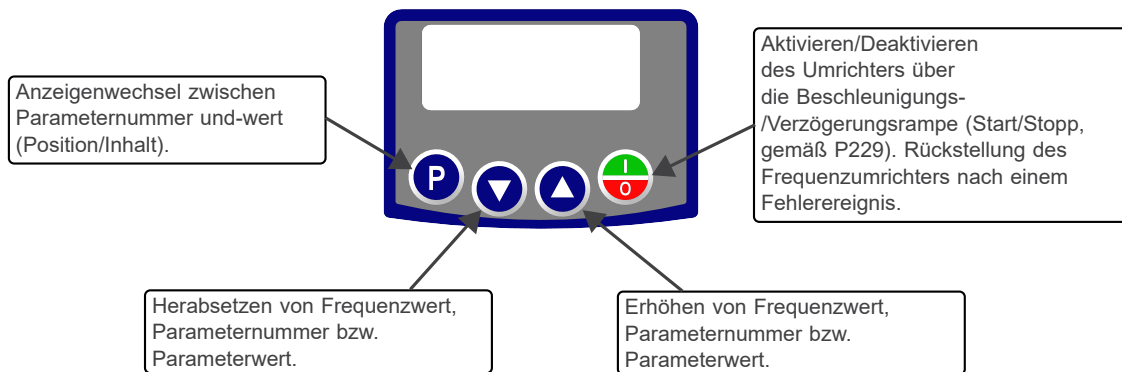
Abbildung 4.1: MMS-Tasten
