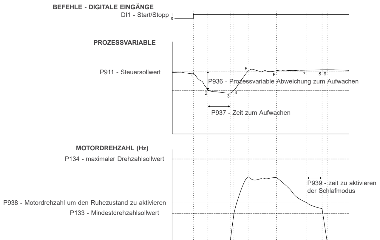
Abbildung 14.4: Betrieb des PID-Reglers mit aktiviertem Ruhezustand
