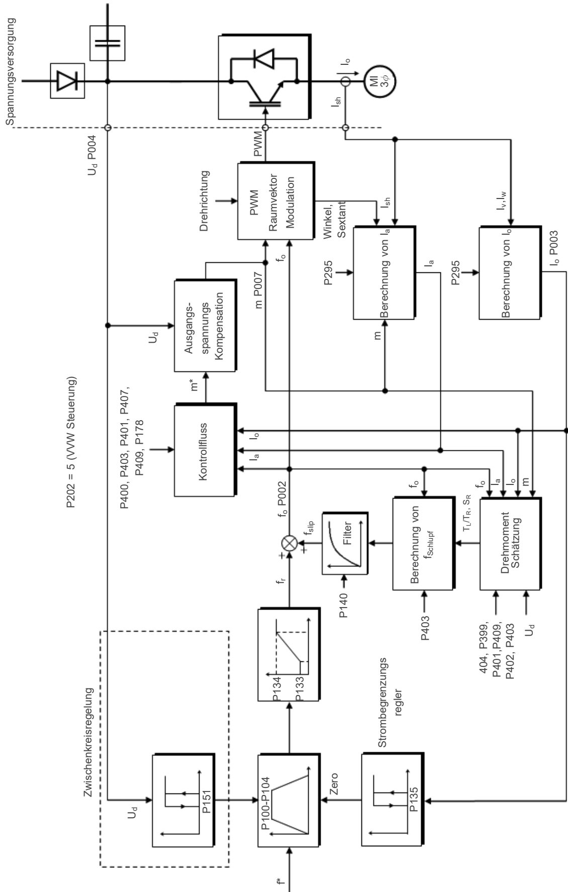
Abbildung 8.20: VVW-Kontrollfluss
