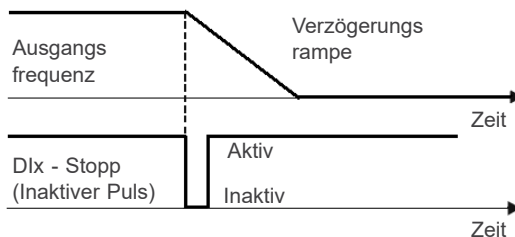
Abbildung 9.18: Beispiel für die Stopp-Funktion mit inaktivem puls
