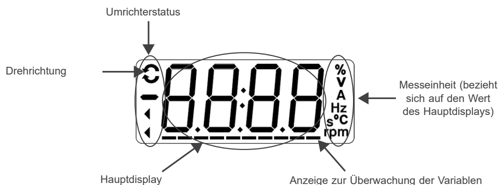
Abbildung 4.2: Anzeigefelder
