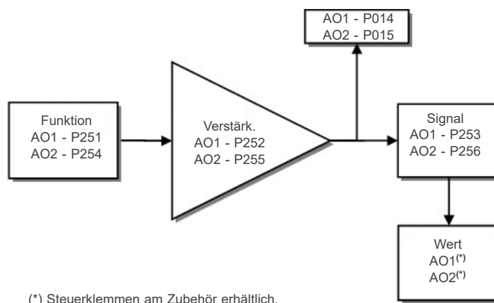
Abbildung 9.4: Blockschaltbild des analogen Ausgangs (AOx)
