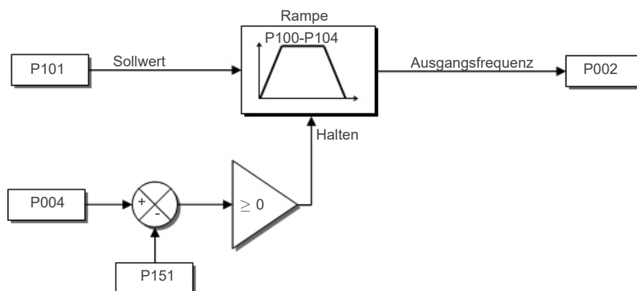
Abbildung 8.3: Blockschaltbild der Begrenzung der Zwischenkreisspannung
