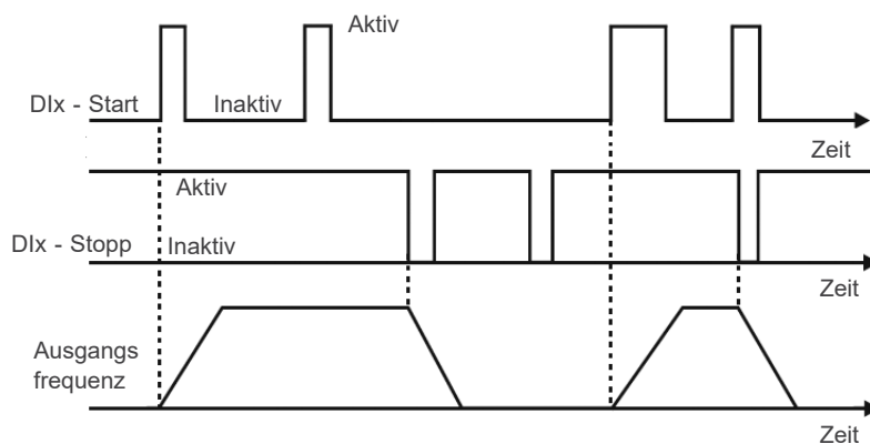
Abbildung 9.10: Beispiel der Funktion Start/Stopp
