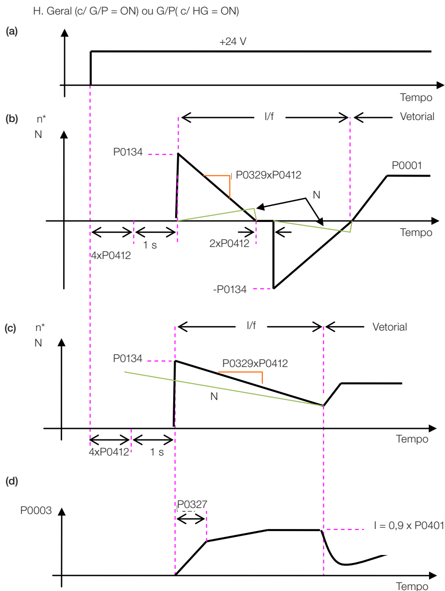
Figura 14.3: (a) a (d) - Influencia de P0327 y P0329 durante el Flying Start (P0202 = 4)
