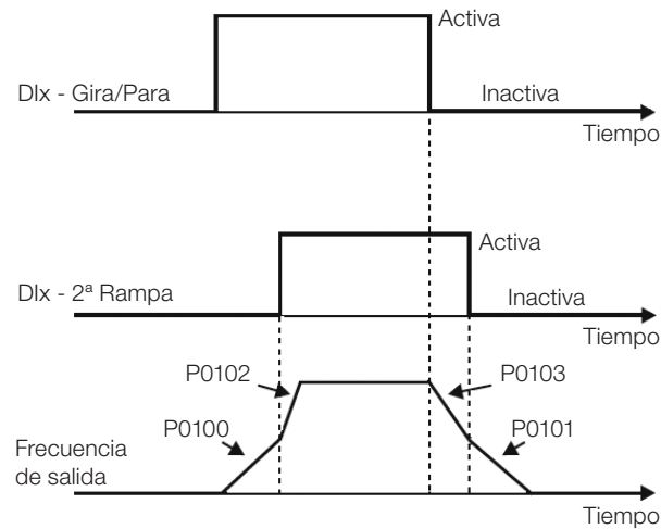
Figura 15.14: Ejemplo de la función 2ª Rampa
