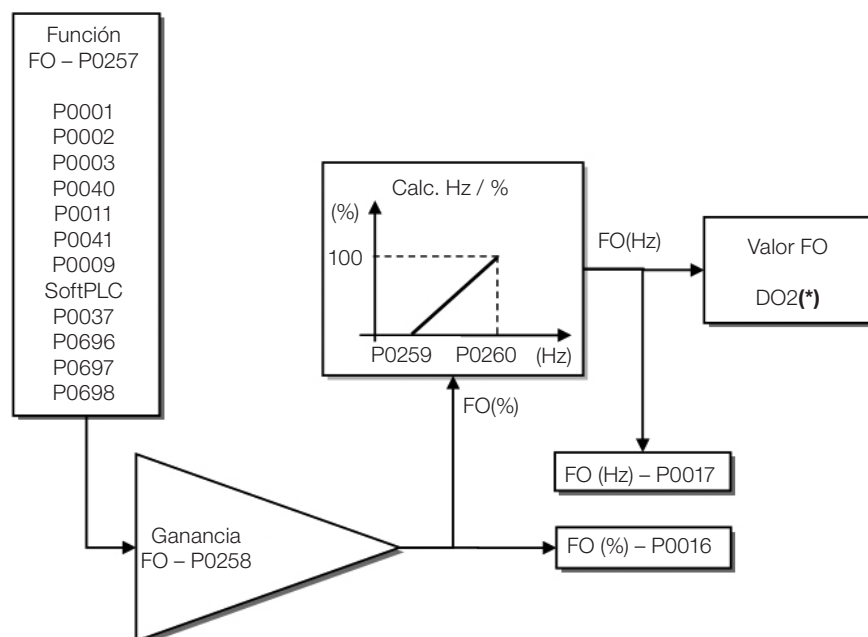
Figura 15.5: Diagrama de bloques de la salida en frecuencia FO (DO2)
