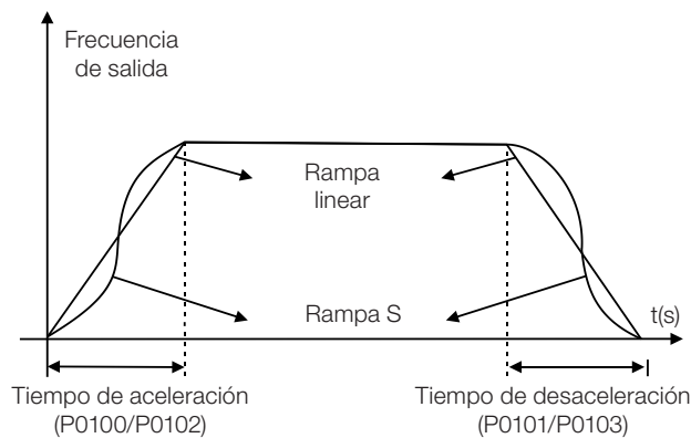
Figura 14.1: Rampa S o Linear
