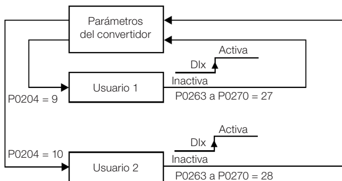
Figura 15.15: Diagrama de bloques de las funciones carga us. 1 y us. 2
