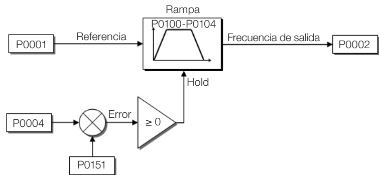
Figura 9.5: Bloque-diagrama de la limitación de la tensión de el Link DC - Hold de Rampa
