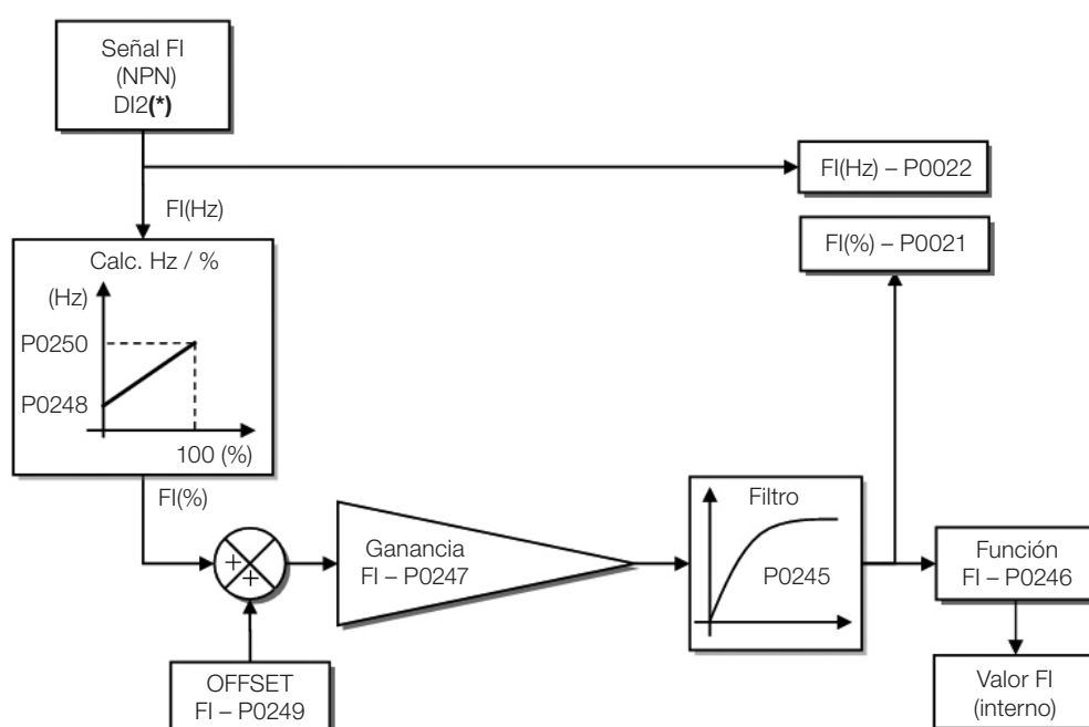
Figura 15.4: Diagrama de bloques de la entrada en frecuencia – FI (DI2)
