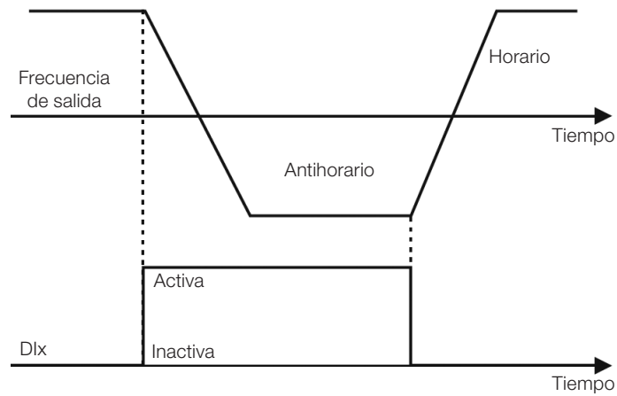
Figura 15.11: Ejemplo de la función Sentido de Giro
