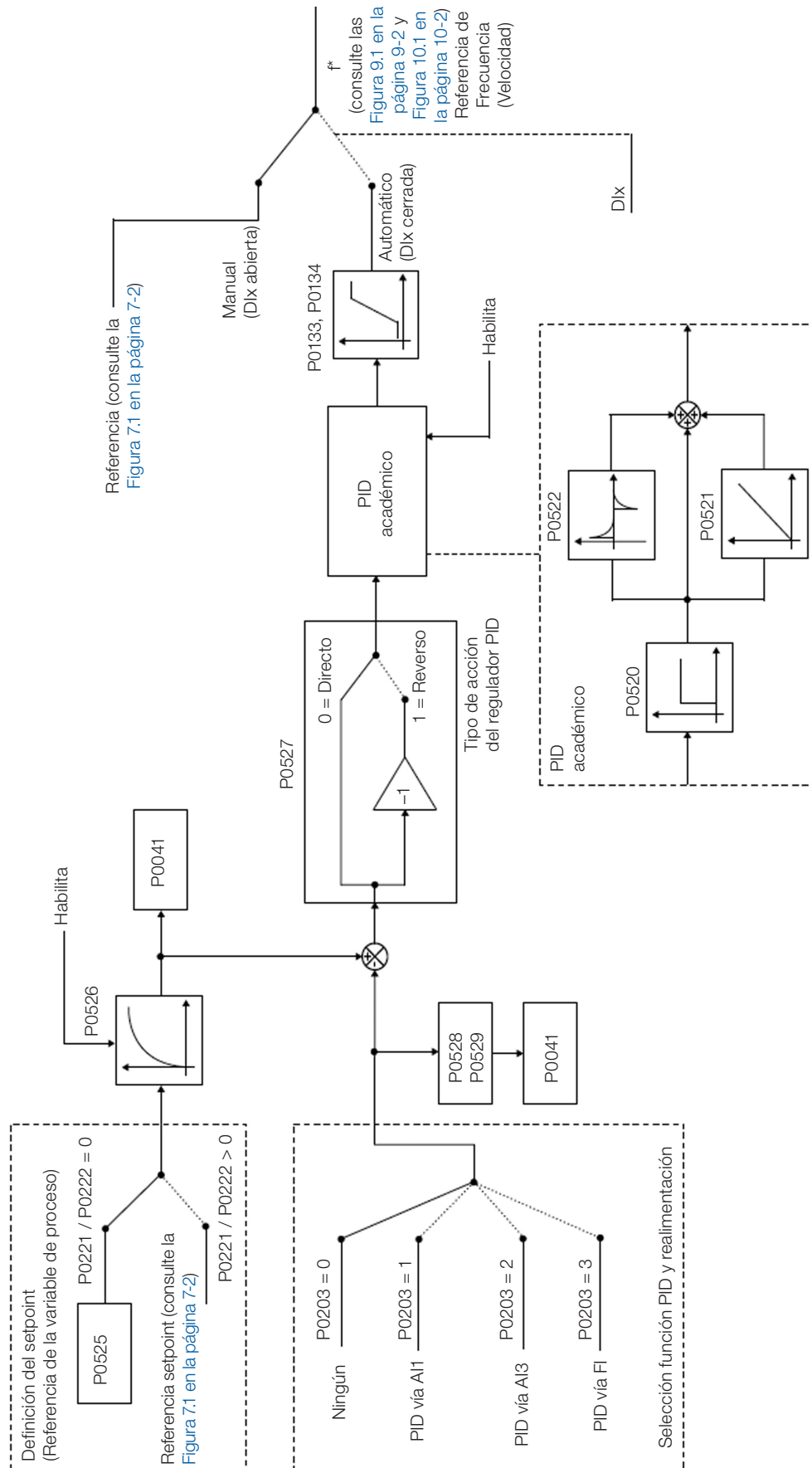
Figura 16.1: Diagrama de bloques del regulador PID
