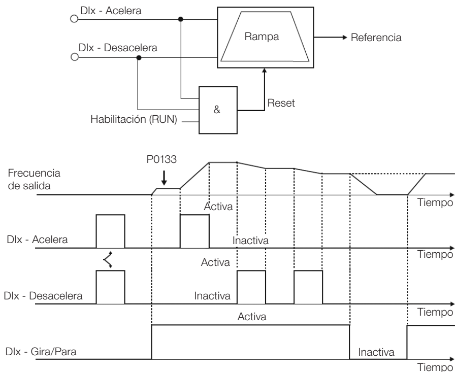
Figura 15.13: Ejemplo de la función Potenciómetro Electrónico (E.P.)
