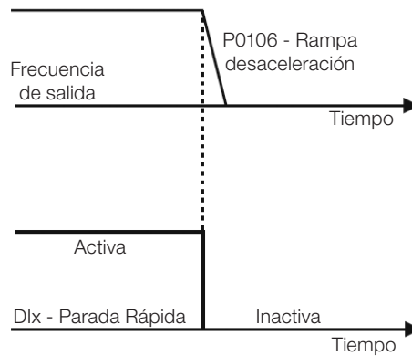
Figura 15.8: Ejemplo de la función Parada Rápida
