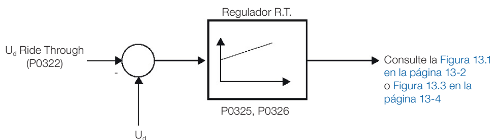
Figura 14.5: Controlador PI del "Ride Through"
