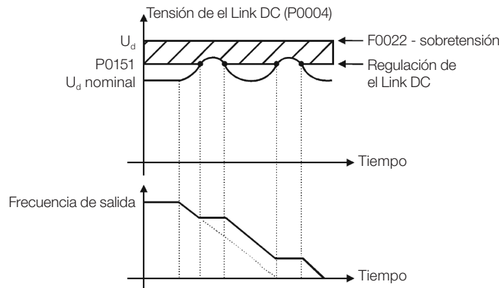
Figura 9.6: Gráfico ejemplo de la limitación de la tensión de el Link DC - Hold de Rampa
