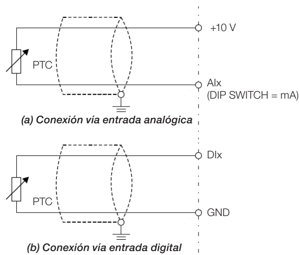
Figura 18.3: (a) y (b) Conexión del PTC al MW500
