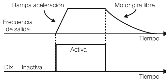
Figura 15.7: Ejemplo de la función Habilita General
