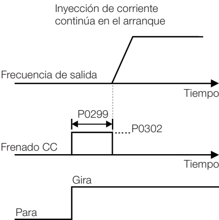
Figura 14.6: Actuación del Frenado CC en el arranque
