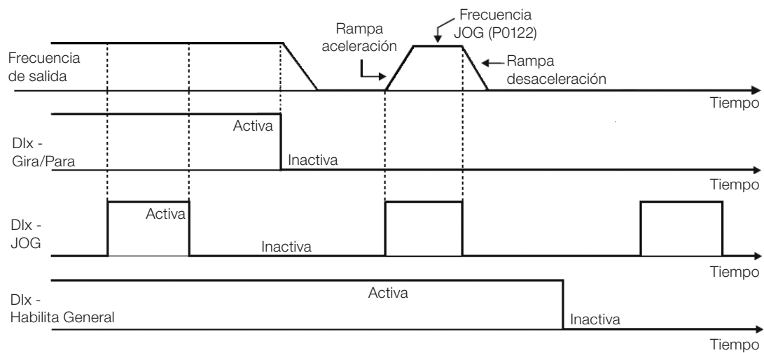
Figura 15.12: Ejemplo de la función JOG
