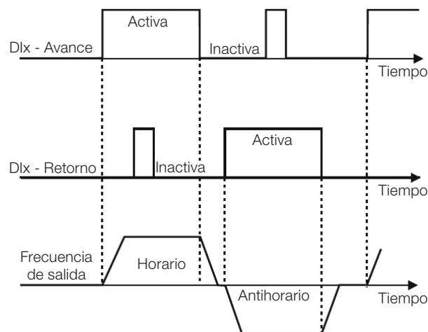
Figura 15.9: Ejemplo de la función Avance/Retorno
