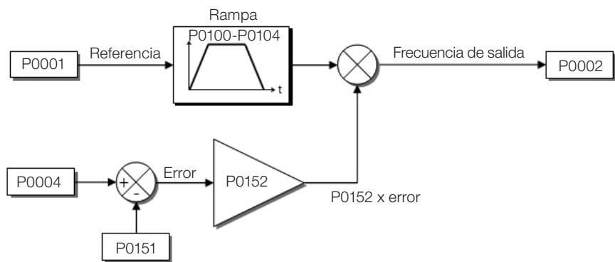
Figura 9.7: Bloque-diagrama de la limitación de la tensión de el Link DC - Acelera Rampa
