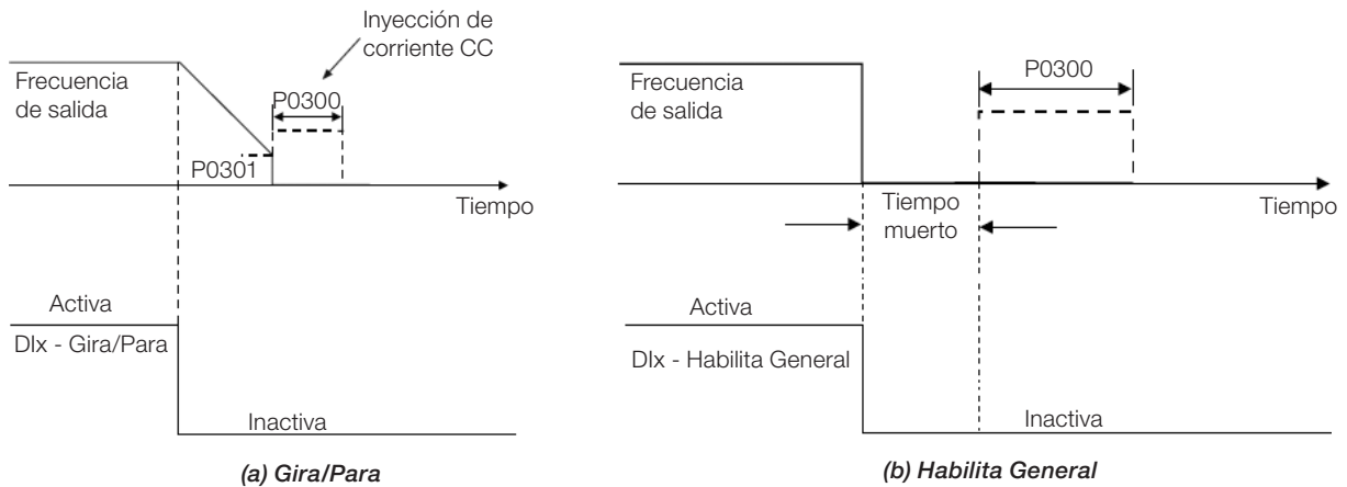
Figura 14.7: (a) y (b) Actuación del Frenado CC
