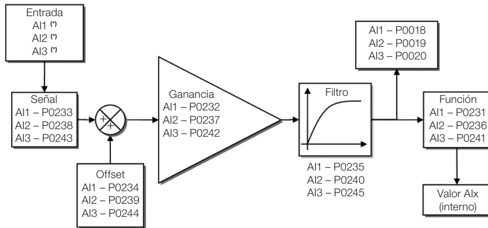
Figura 15.2: Diagrama de bloques de las entradas analógicas - Alx
