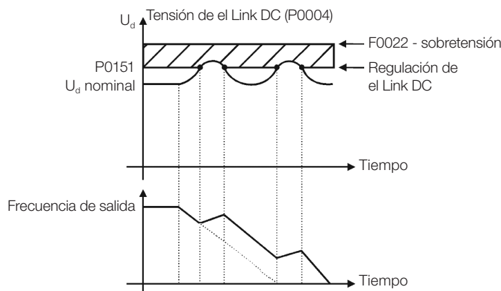
Figura 9.8: Gráfico ejemplo de la limitación de la tensión de el Link DC - Acelera Rampa
