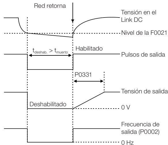
Figura 14.2: Actuación de la función Ride Through
