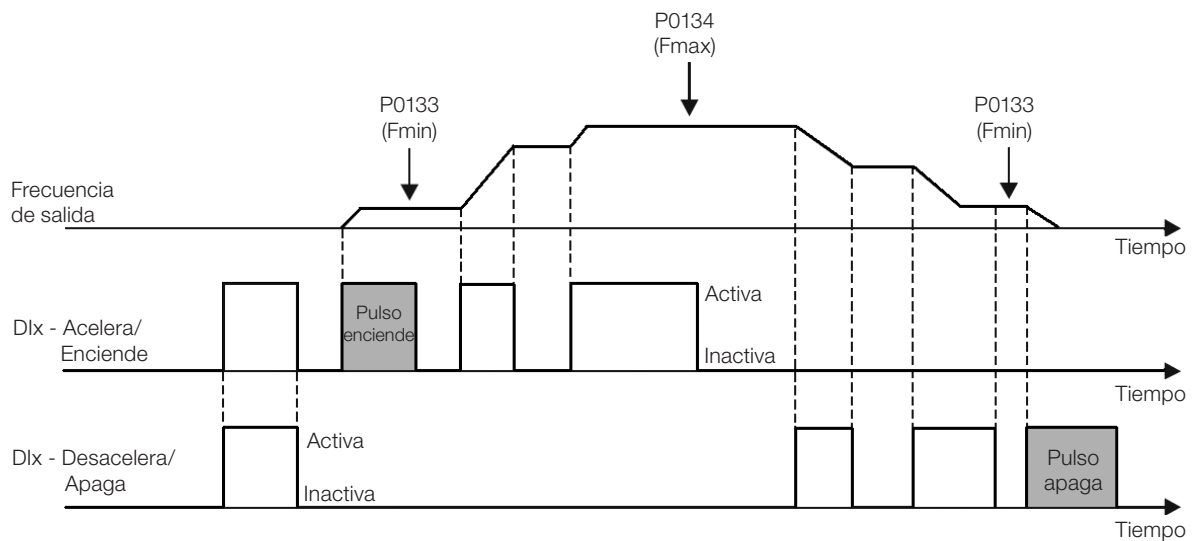
Figura 15.16: Ejemplo de la función Acelera enciende / Desacelera apaga
