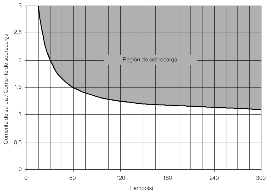
Figura 18.1: Actuación de la sobrecarga del motor
