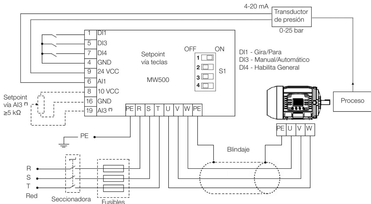
Figura 16.2: Ejemplo de aplicación del regulador PID del MW500
