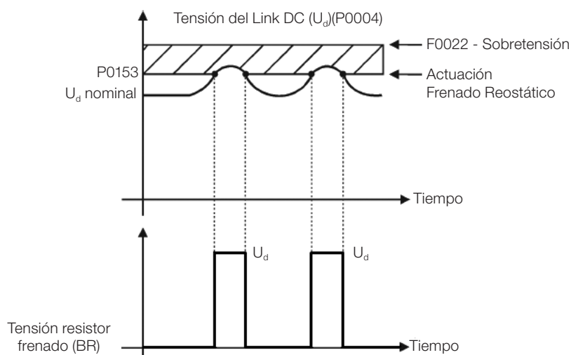
Figura 17.1: Curva de actuación del Frenado Reostático
