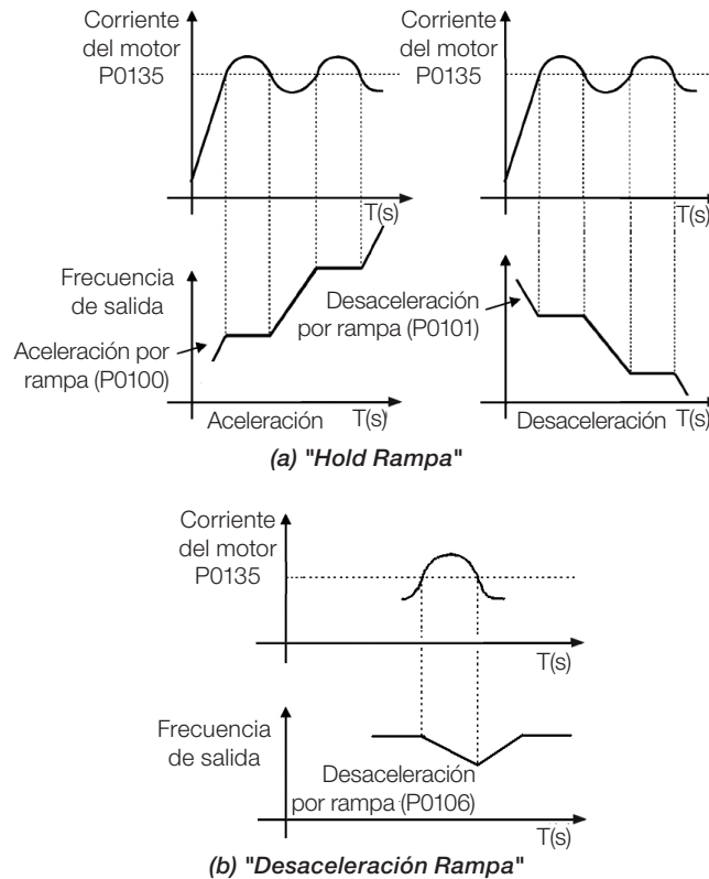
Figura 9.9: (a) y (b) Modos de actuación de la Limitación de Corriente vía P0135
