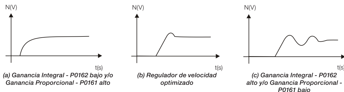
Figura 13.5: (a) a (c) - Tipo de respuestas del regulador de velocidad
