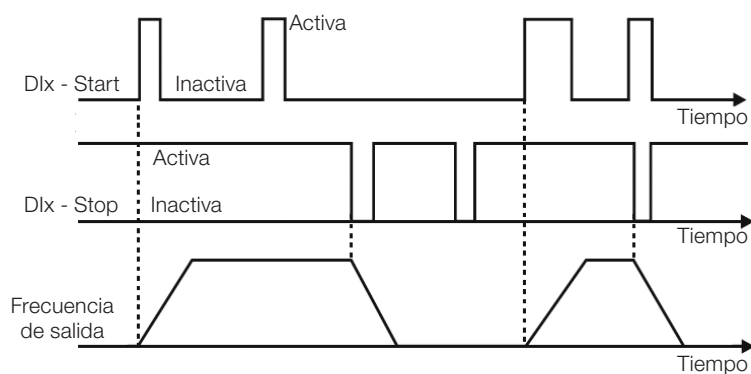
Figura 15.10: Ejemplo de la función Start/Stop tres hilos
