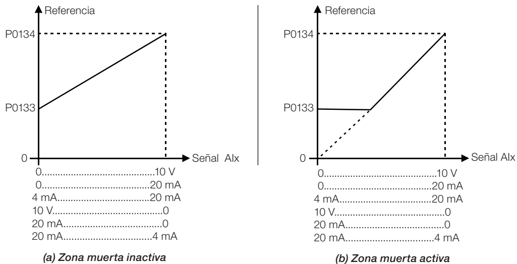
Figura 15.1: (a) y (b) Actuación de las entradas analógicas
