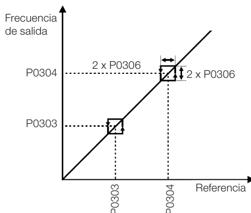
Figura 14.8: Actuación de la frecuencia evitada
