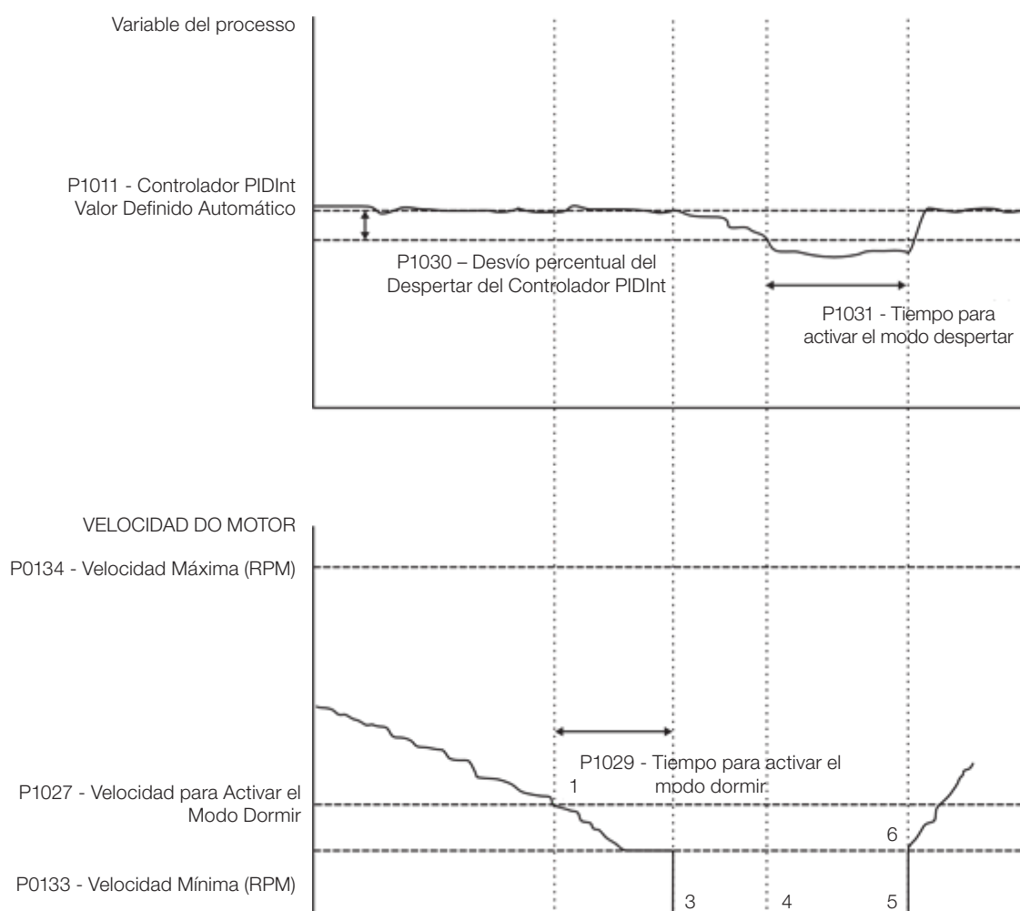
Figura 21.1: Esquema de funcionamiento para modo dormir y modo despertar
