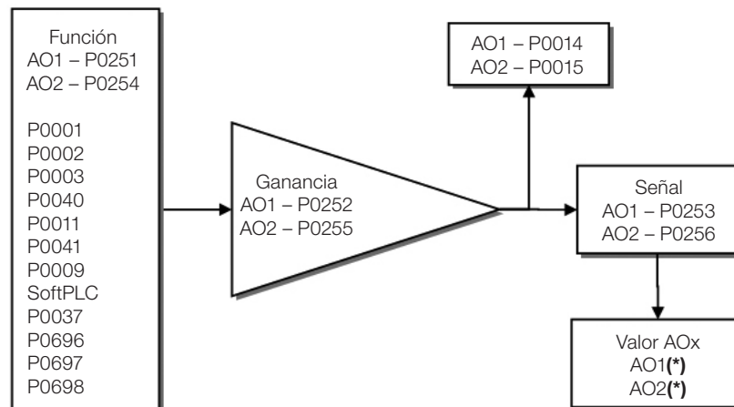
Figura 15.3: Diagrama de bloques de las salidas analógicas – AOx
