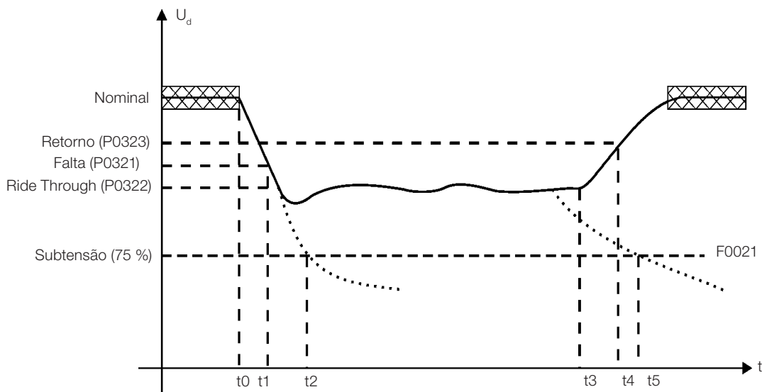
Figura 14.4: Actuación de la función Ride Through en el modo vectorial
