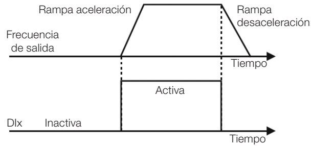
Figura 15.6: Ejemplo de la función Gira/Para
