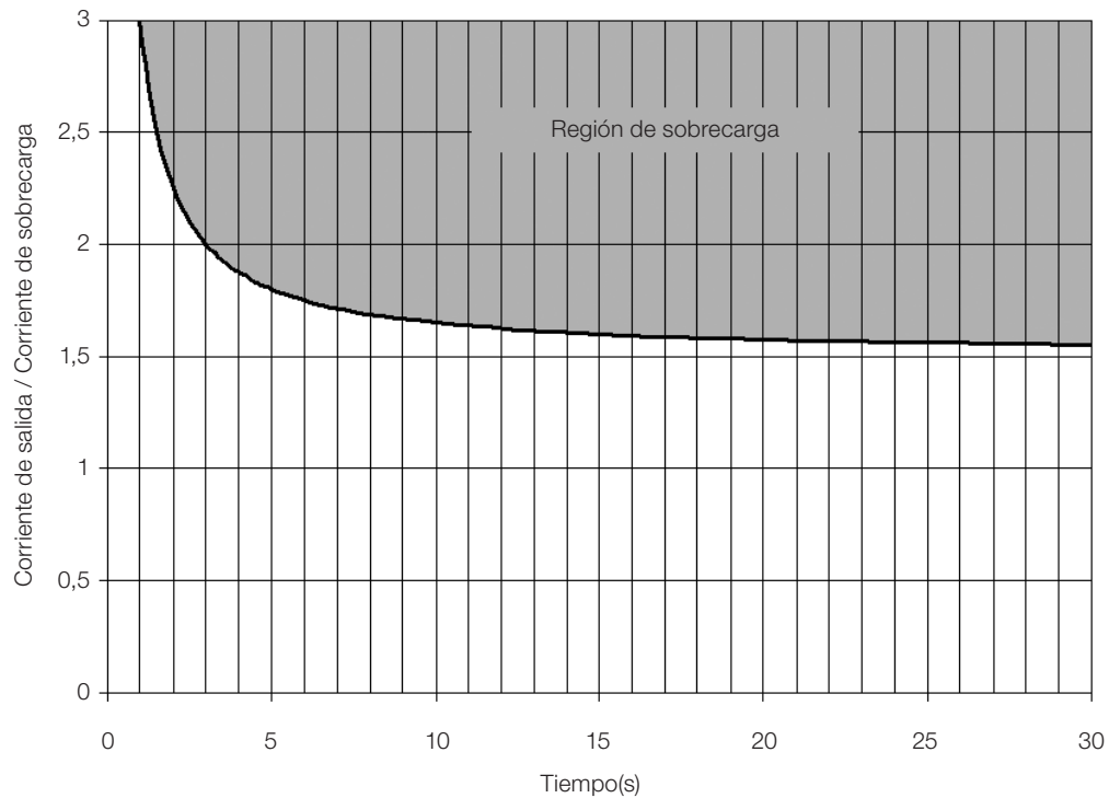
Figura 18.2: Actuación de la sobrecarga de los IGBTs
