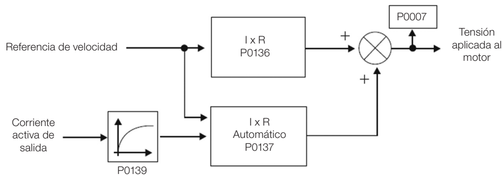
Figura 9.4: Bloque-diagrama del boost de torque automático
