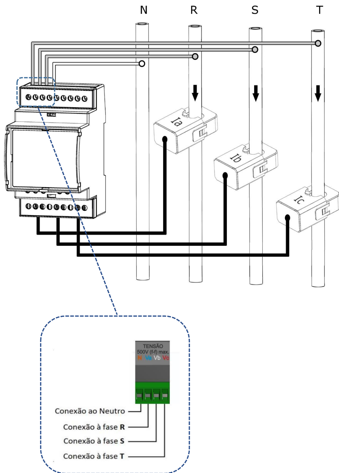
Figura 10 - TL00 Trifásico Estrela
