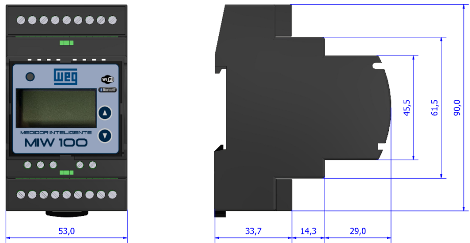
Figura 2 - Dimensionais
