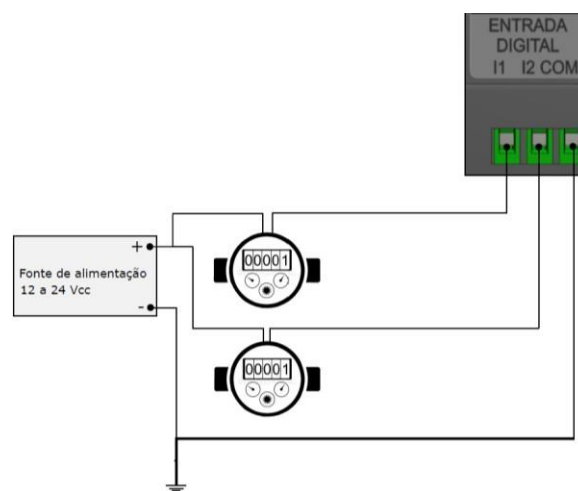
Figura 13 - Esquema de ligação Entrada Digital
