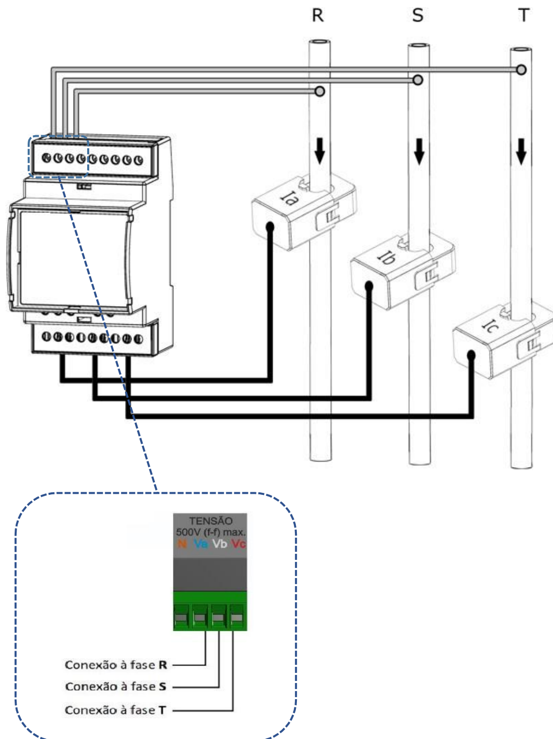
Figura 12 - TL17 Trifásico Delta 2TC's
