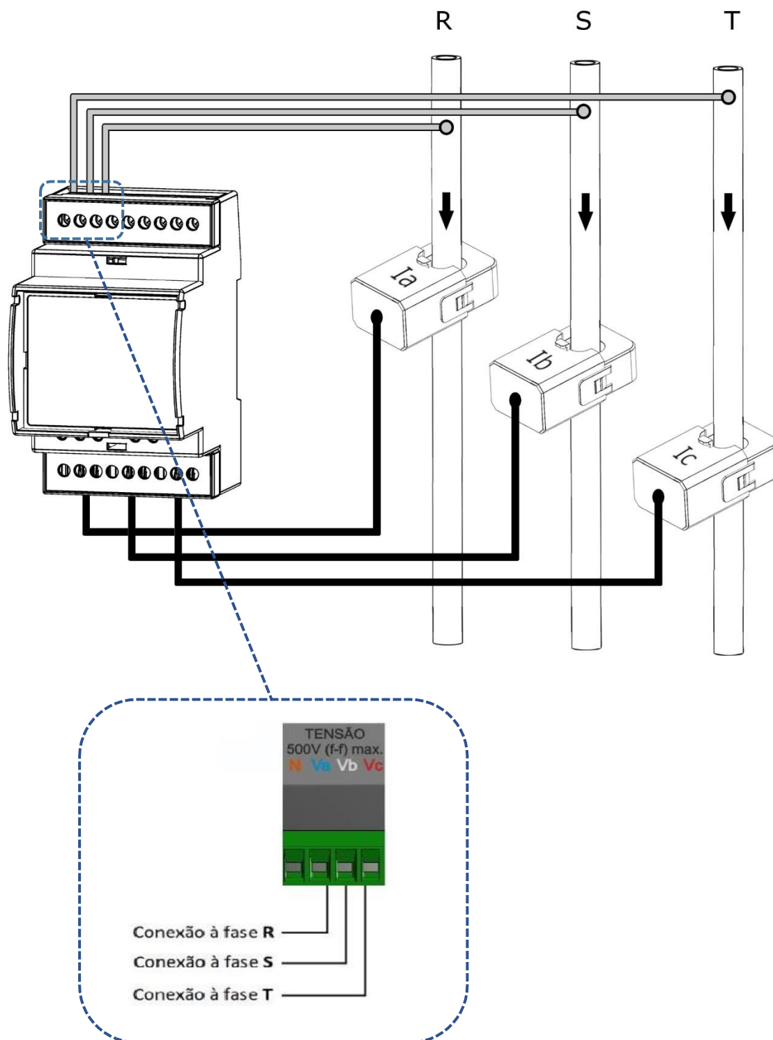
Figura 11 - TL48 Trifásico Delta
