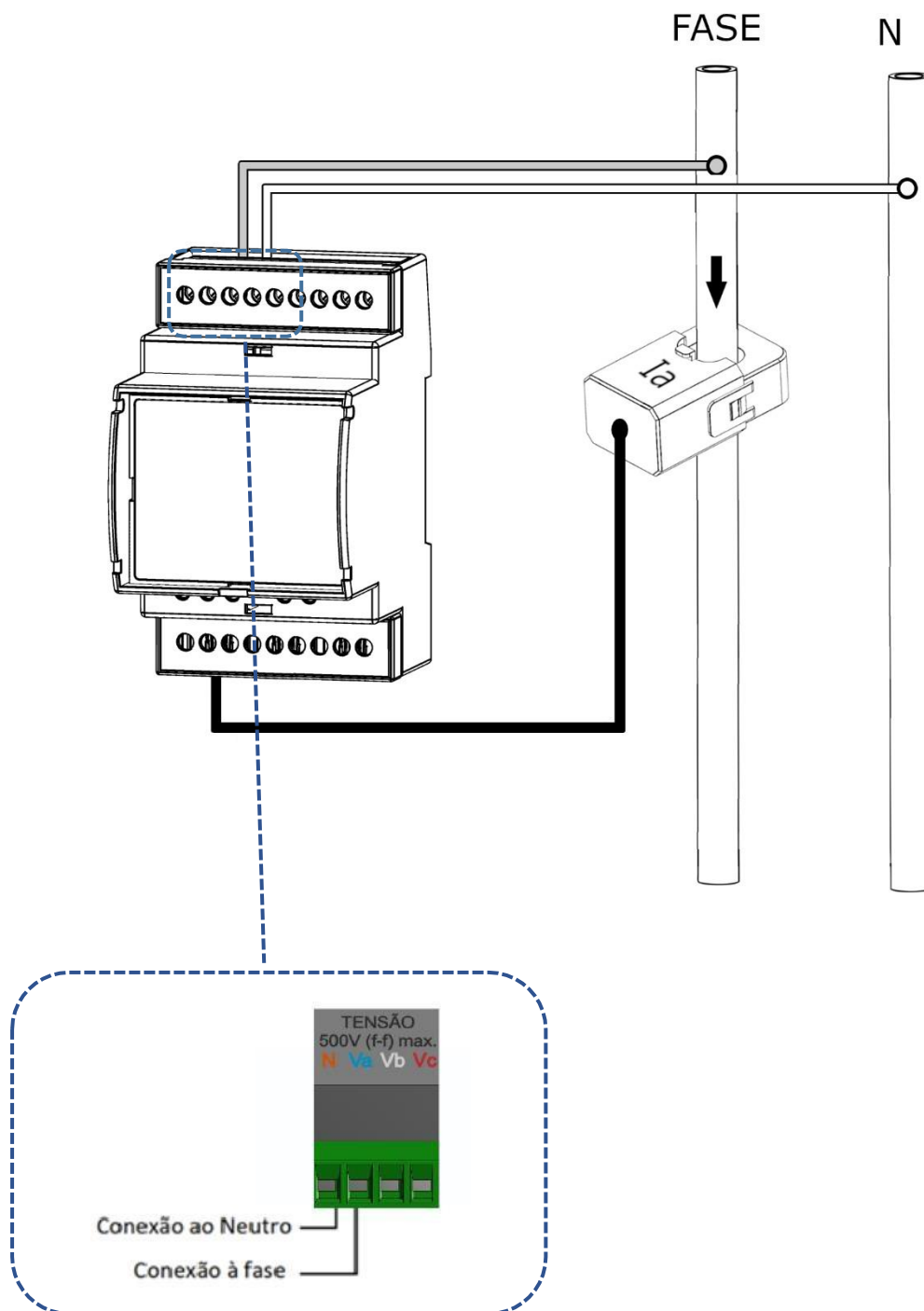
Figura 8 - TL02 Monofásico
