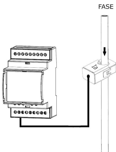
Figura 7 - Entrada de Corrente
