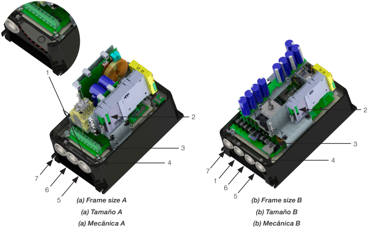
Figura A.4: (a) a (c) Procedimento de remoção do fechamento frontal do CFW500 IP66
