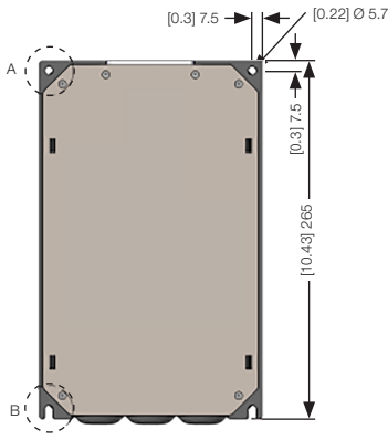
Figure A.1: Dimensions of the CFW500 IP66 frame size A Figura A.1: Dimensiones CFW500 IP66 tamaño A Figura A.1: Dimensões CFW500 IP66 mecânica A
