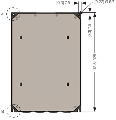
Figure A.2: Dimensions of the CFW500 IP66 frame size B Figura A.2: Dimensiones CFW500 IP66 tamaño B Figura A.2: Dimensões CFW500 IP66 mecânica B
