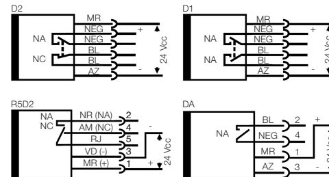
Figura 1: Diagrama eléctrico
