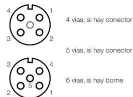
Figura 1: Diagrama eléctrico
