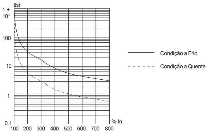
Figura 15.2 - Curva de sobrecarga eletrônica dos tiristores.
