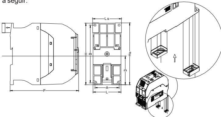
Figura 10.1 - Dimensiones de la SSW-05 Plus
