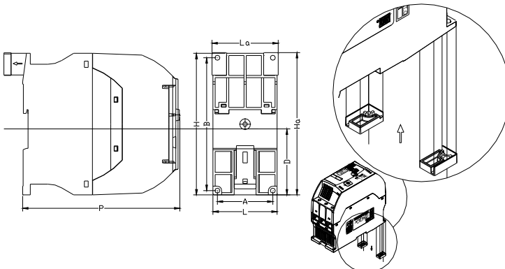
Figura 10 - Dimensões da SSW-05 Plus
