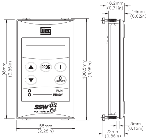
Figura 19.3 – Dimensiones del HMI-SSW05-RS
