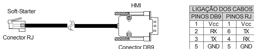
Figura 19.1- Cabo CAB-RS para HMI-SSW05-RS
