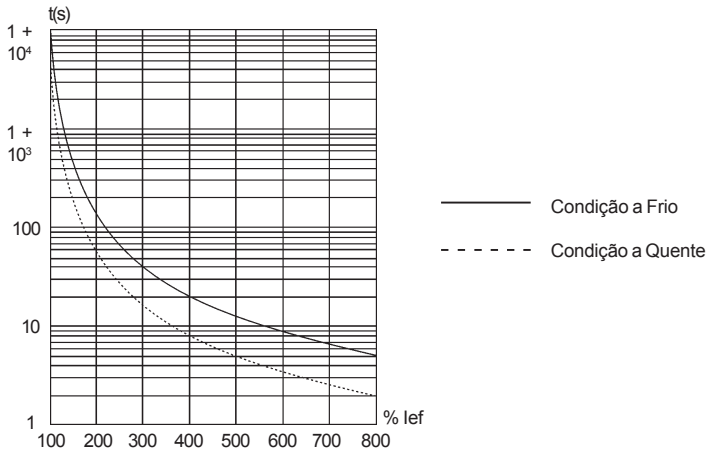
Figura 15.1 - Curva de sobrecarga eletrônica do motor.
