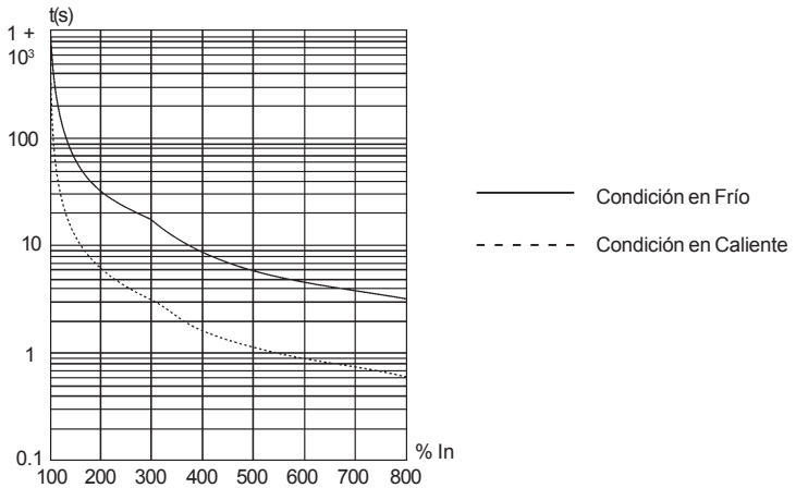
Figura 15.2 - Curva de sobrecarga electrónica de los tiristores.
