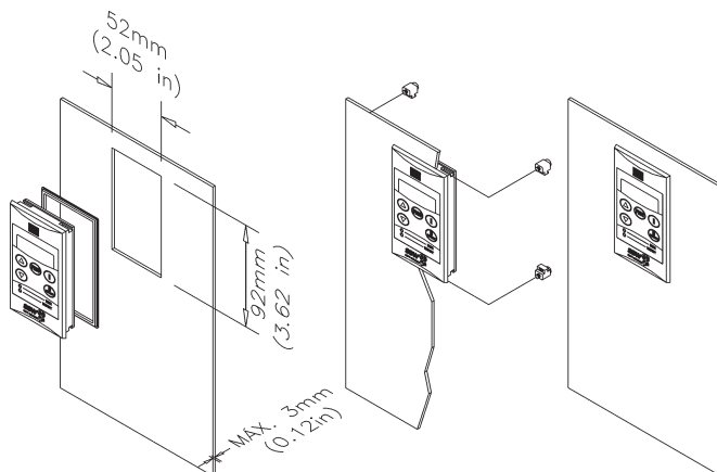
Figura 19.5 - Instalación del HMI-SSW05-RS
