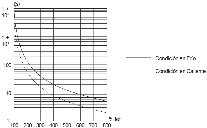
Figura 15.1 - Curva de sobrecarga electrónica del motor.
