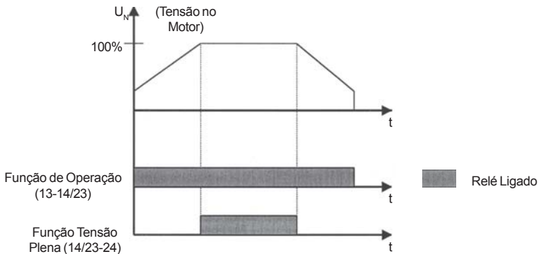
Figura 13 - Funcionamento das saídas digitais a relé
