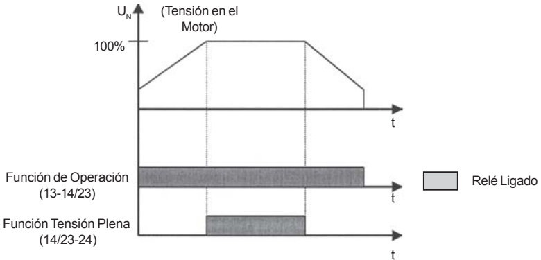
Figura 13 - Funcionamiento de las salidas digitales al relé
