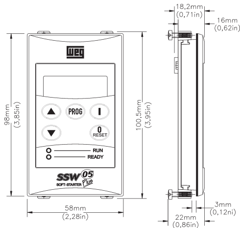
Figura 19.3 - Dimensões da HMI-SSW05-RS.
