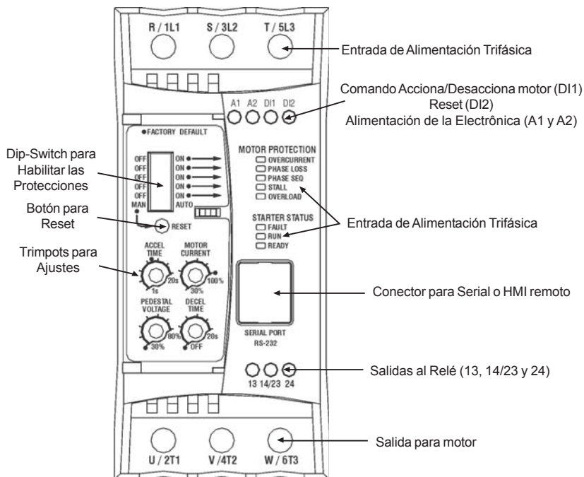
Figura 5.1 - Vista frontal de la SSW05 Plus
