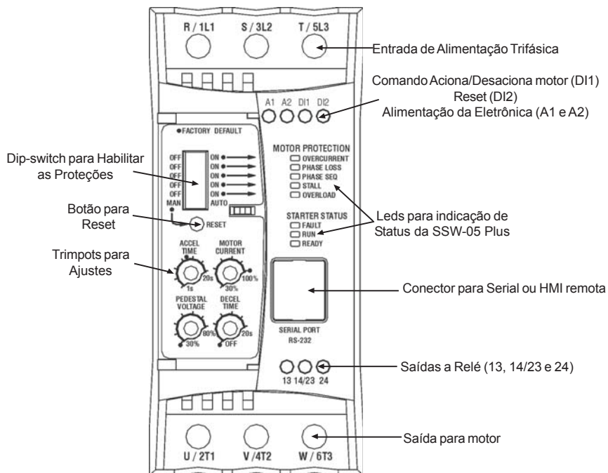
Figura 5.1 - Vista frontal da SSW05 Plus
