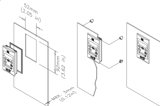
Figura 19.5 - Instalação da HMI-SSW05-RS.
