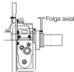
Figura 4.10: Marcação do centro magnético
