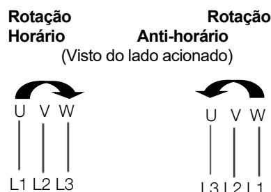
Figura 6.1: Sequência de fases (IEC60034-8)
