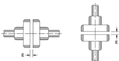
Figura 4.8: Folga axial do acoplamento (E)
