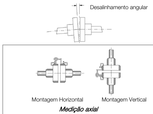
Figura 4.6: Alinhamento angular
