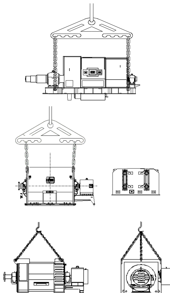
Figura 3.1: Manuseio dos geradores
