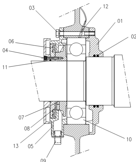
Figura 7.2: Partes do mancal de rolamento a graxa
