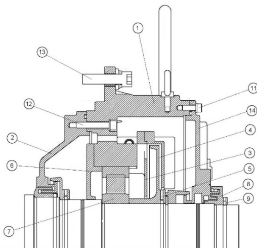
Figura 7.5: Partes do mancal de rolamento a óleo
