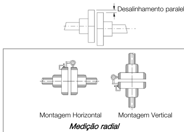
Figura 4.5: Alinhamento paralelo
