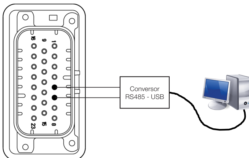
Figura 3.20: Conexão da interface RS-485 com o PC disponível no conector XC9
