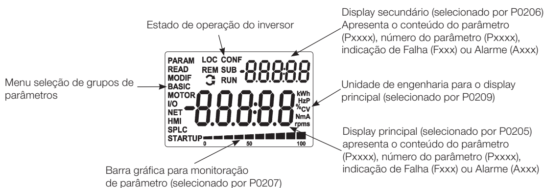
Figura 5.2: Tela na inicialização e campos do display
