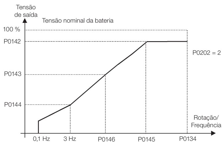
Figura 10.7: Curva V/f em função de P0142 a P0146
