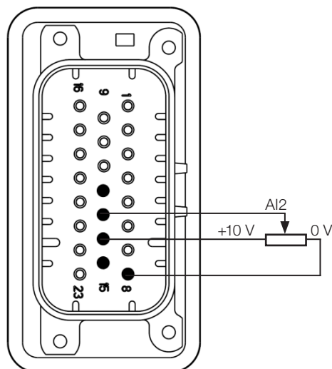
Figura 3.11: Conexões da AI2 (0...10 V e +10...0 V) em XC10
