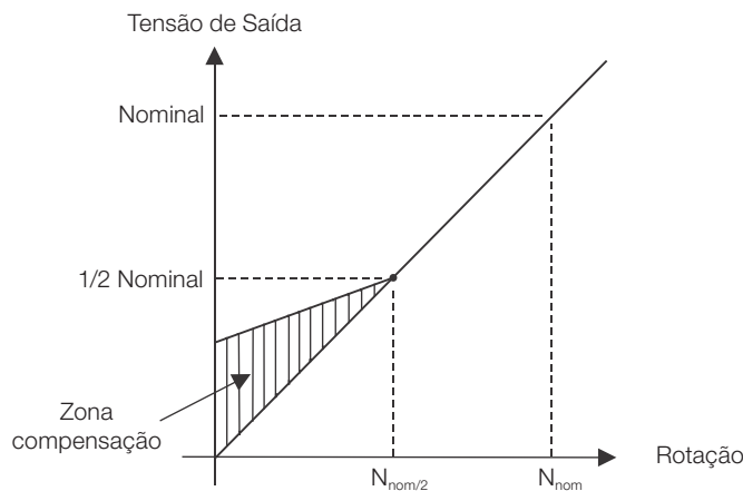
Figura 10.4: Efeito de P0137 na curva V/f (P0202 = 0)
