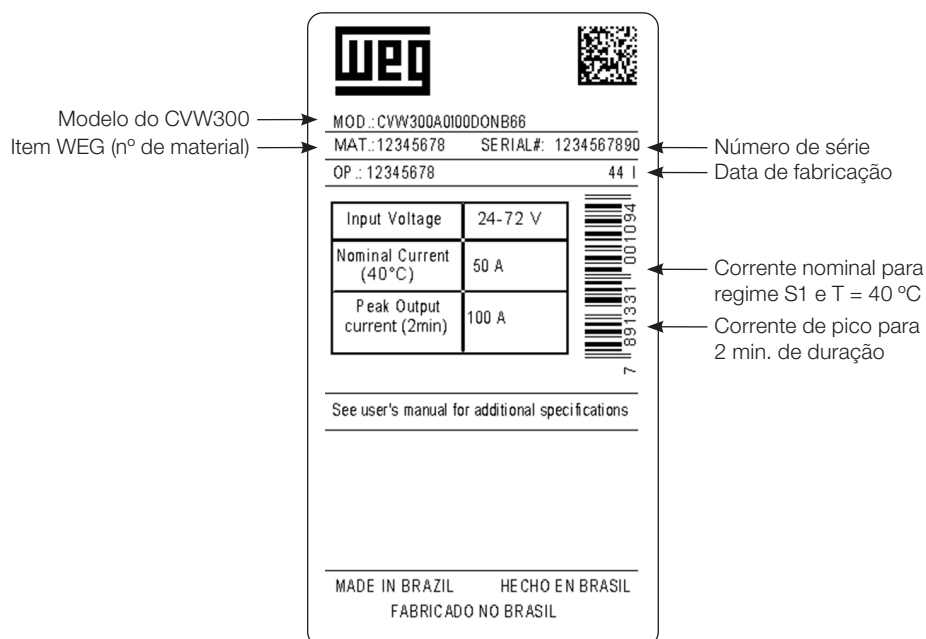
Figura 2.2: Etiqueta de identificação
