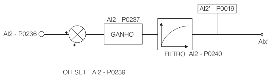
Figura 12.2: Blocodiagrama da entrada analógica AI2
