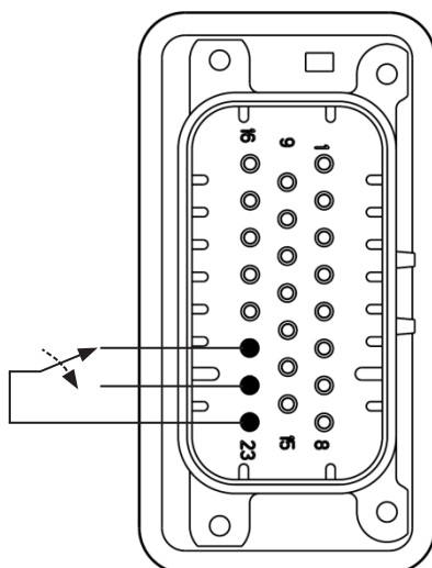
Figura 3.16: Saída digital a relé, disponibilizada no conector XC10
