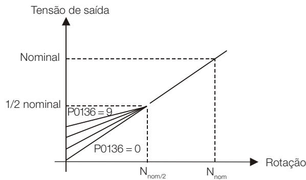
Figura 10.2: Efeito de P0136 na curva V/f (P0202 = 0 ou 1)
