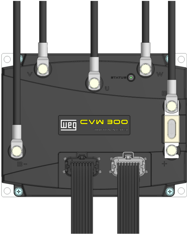
Figura 3.2: Conexões dos cabos de potência e sinal do CVW300
