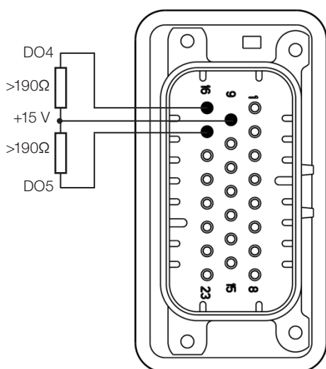
Figura 3.14: Conexões das saídas digitais DO4 e DO5, disponíveis em XC9
