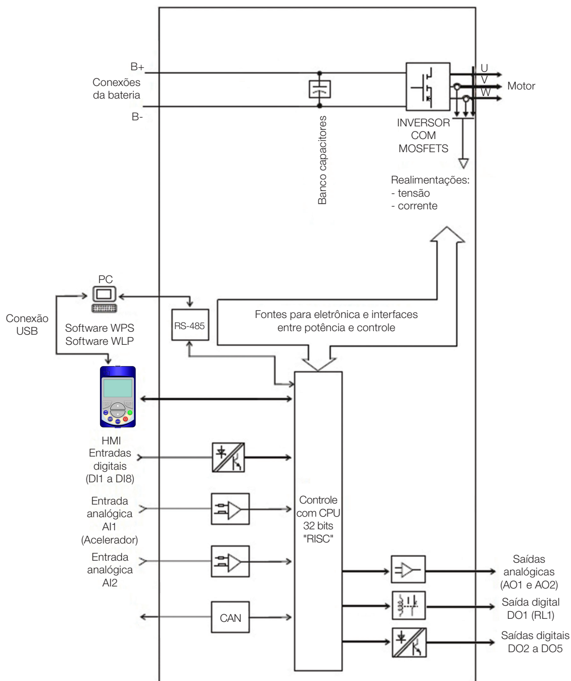
Figura 2.1: Blocodiagrama do CVW300
