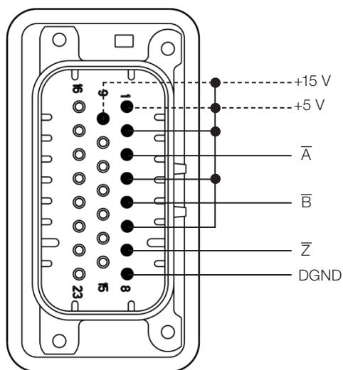
Figura 3.26: Conexões para encoder tipo coletor aberto
