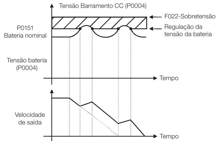
Figura 10.12: Gráfico exemplo de atuação da limitação da tensão da bateria com a função acelera rampa
