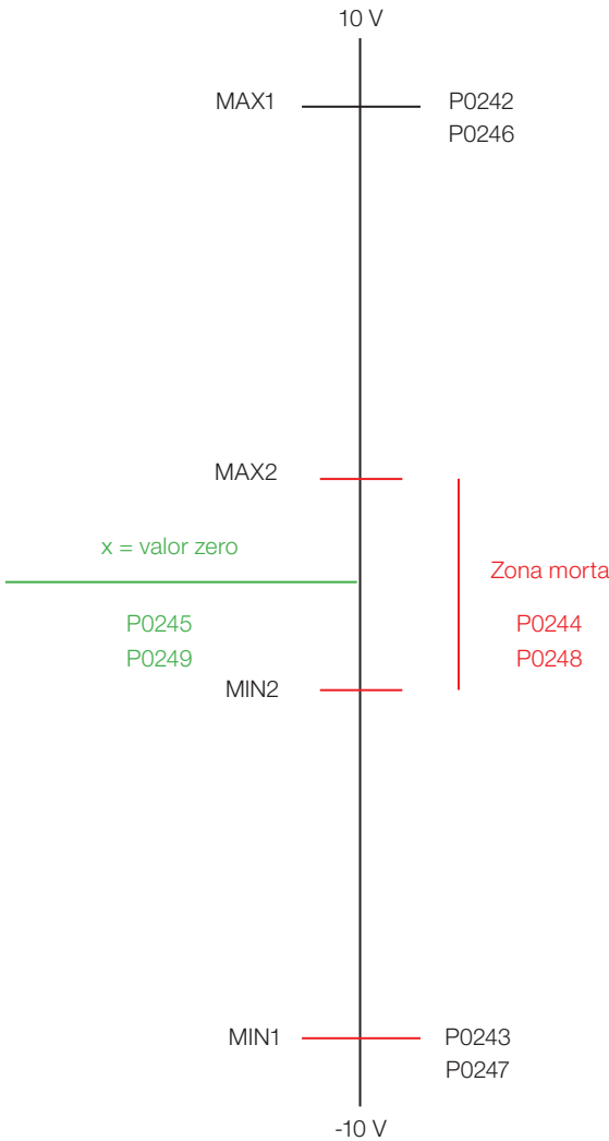
Figura 12.4: Representação da escala de leitura da AI1
