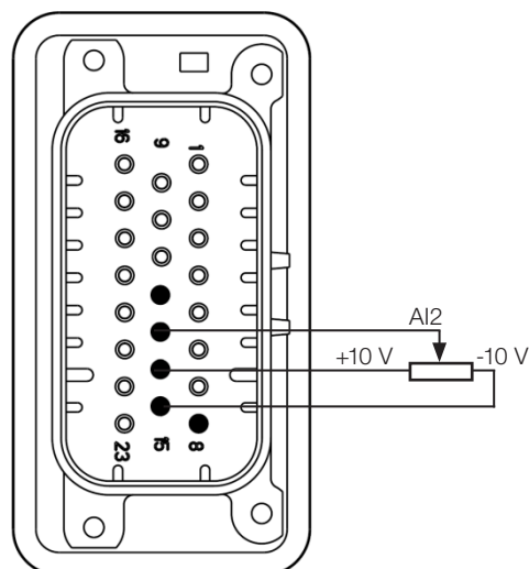
Figura 3.13: Conexões da AI2 (-10...10 V), em XC10
