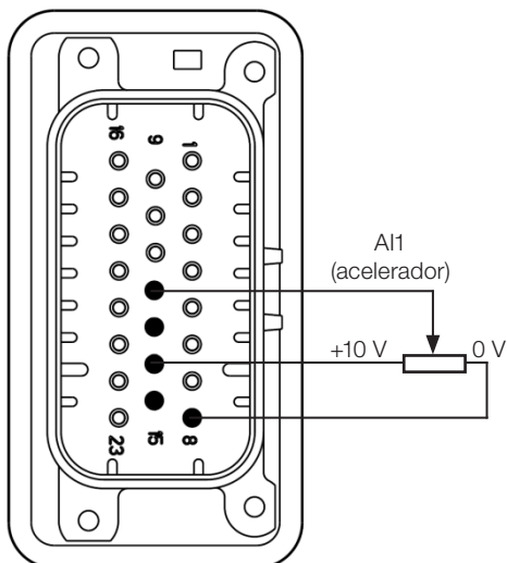
Figura 3.10: Conexão do acelerador (0...10 V e +10...0 V) em XC10
