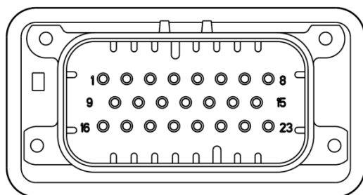
Figura 3.6: Conector XC9 (PRETO)
