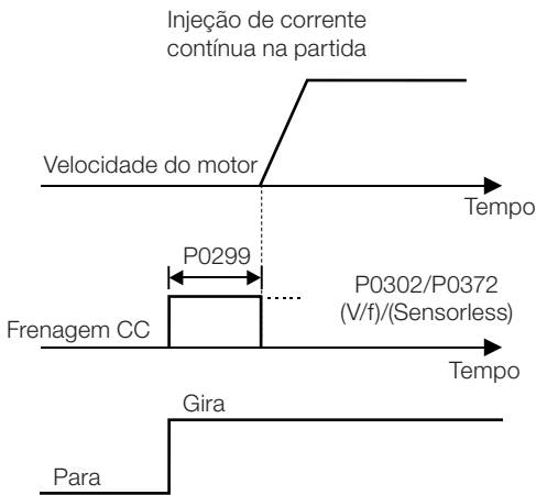
Figura 11.5: Atuação de frenagem CC na partida
