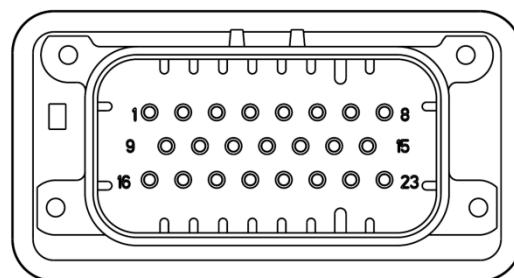
Figura 3.7: Conector XC10 (CINZA)
