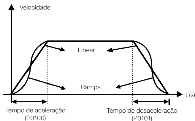
Figura 11.1: Rampa S ou linear
