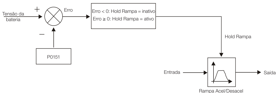
Figura 10.9: Blocodiagrama da função de limitação da tensão da bateria utilizando Hold de Rampa
