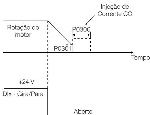
Figura 11.6: (a) e (b) Atuação da frenagem CC no bloqueio por rampa (via desabilita rampa)
