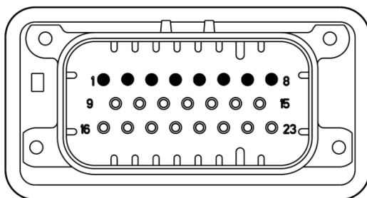
Figura 3.24: Terminais para conexão do encoder disponível no conector XC10
