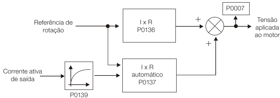
Figura 10.3: Blocodograma boost de torque
