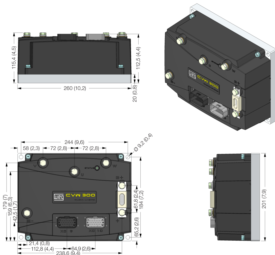
Figura 3.1: Dimensionais do CVW300
