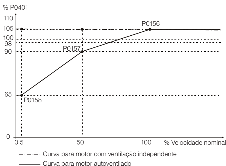
Figura 13.2: Níveis de proteção de sobrecarga
