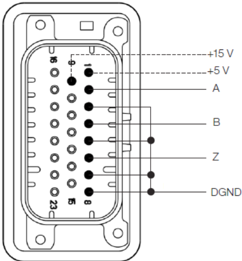
Figura 3.27: Conexões para encoder tipo linedrive e ou push-pull sem canais diferenciais
