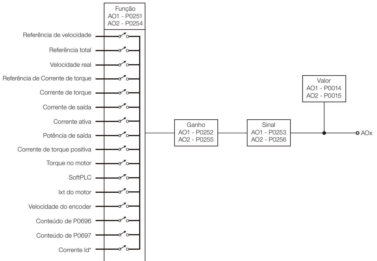
Figura 12.9: Blocodiagrama das saídas analógicas
