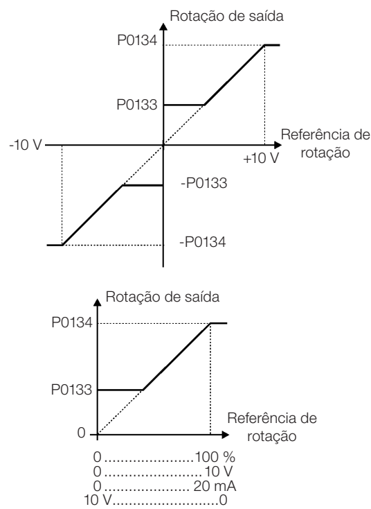
Figura 11.3: Limites de rotação considerando "Zona Morta" ativa (P0230 = 1)
