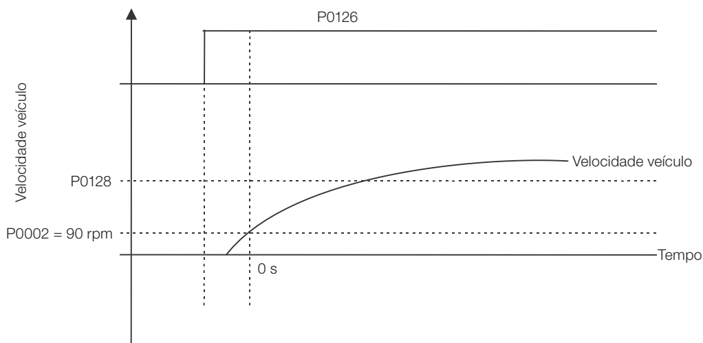
Figura 11.2: Atuação da função de tempo para atingir uma velocidade específica
