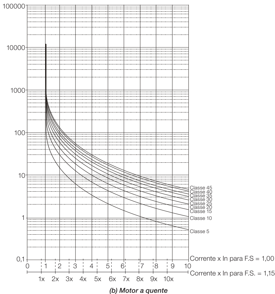
Figura 13.3: (a) e (b) Curvas de sobrecarga
