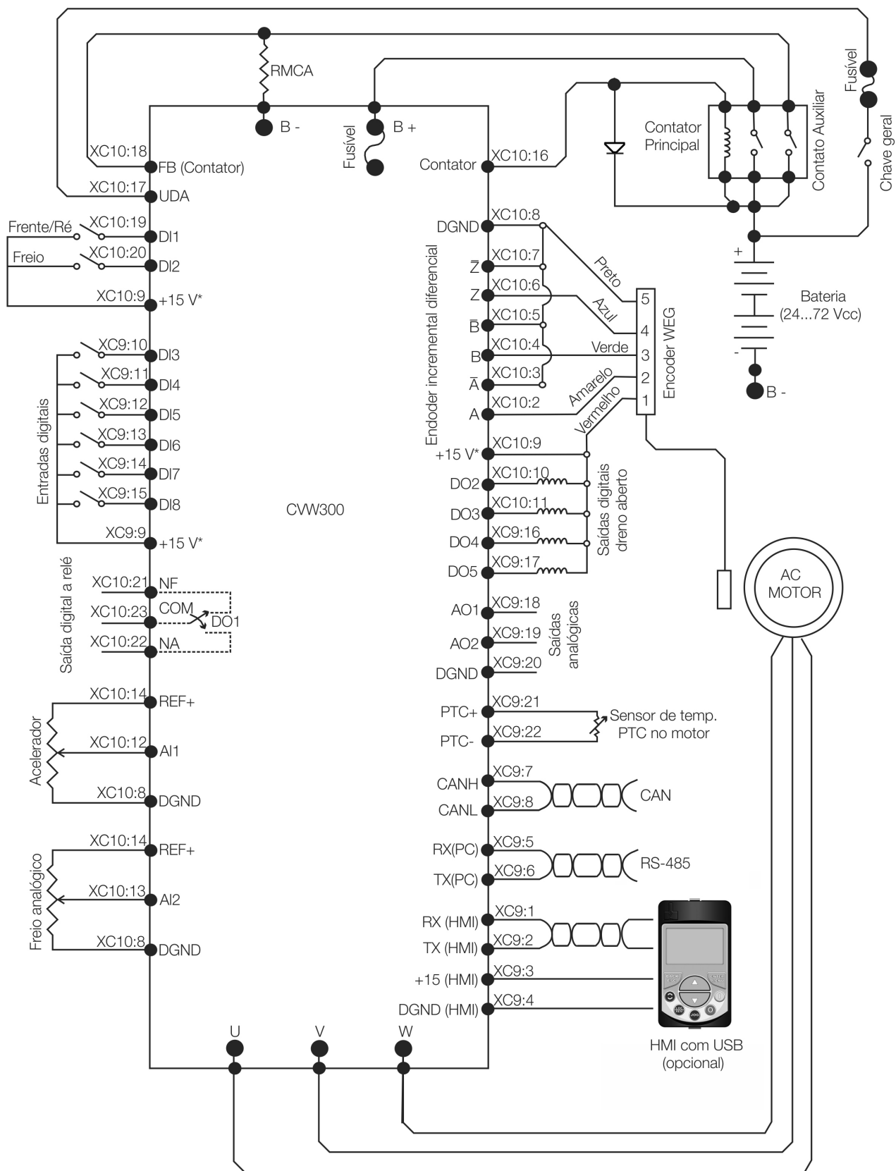
Figura 3.4: Diagrama de conexões
