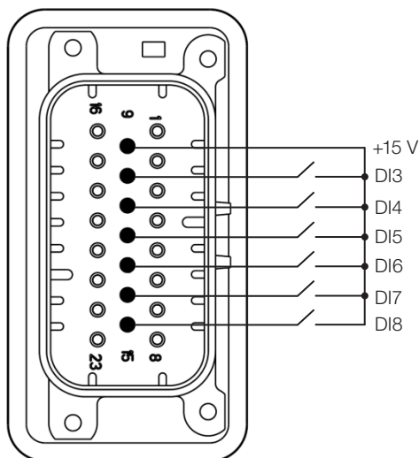
Figura 3.8: Conexões das entradas digitais em XC9
