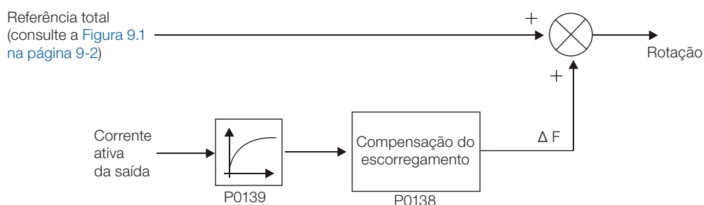
Figura 10.5: Blocodograma da compensação de escorregamento
