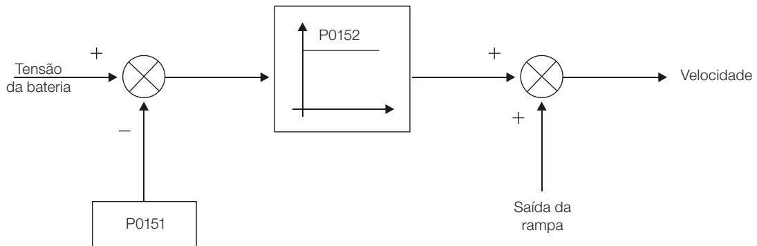
Figura 10.11: Blocodigrama da função de limitação da tensão da bateria via acelera rampa
