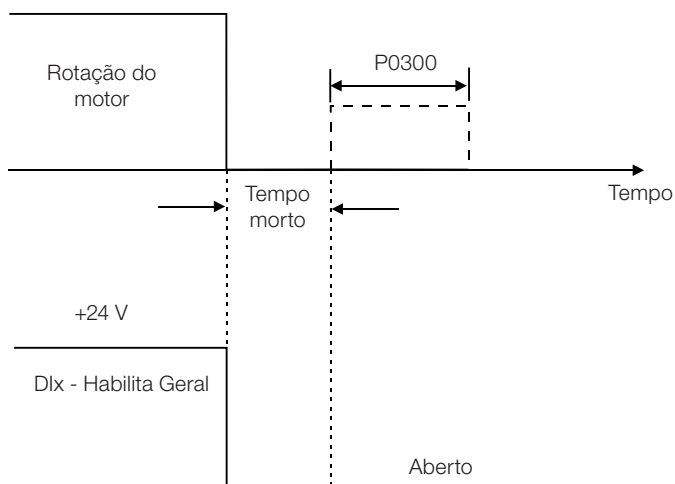
Figura 11.7: Atuação da frenagem CC via Desabilita Geral - Modo V/f
