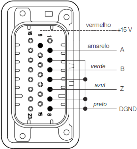
Figura 3.28: Conexões para encoder do motor de tração WEG tipo linedrive e ou push-pull sem canais diferenciais
