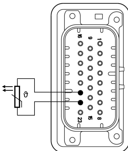
Figura 3.18: Conexão do PTC disponível no conector XC9
