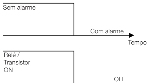
Figura 12.12: (a) a (q) Detalhes do funcionamento das funções das saídas digitais e a relé
