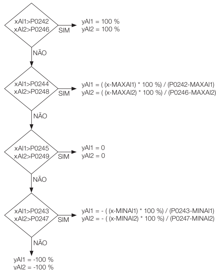
Figura 12.7: Fluxograma da rotina de calibração de AI1 e AI2
