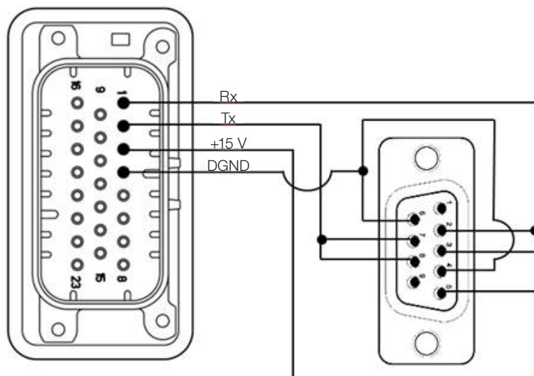
Figura 3.23: Conexões entre conector XC9 e DB9 (fêmea – Vista traseira)
