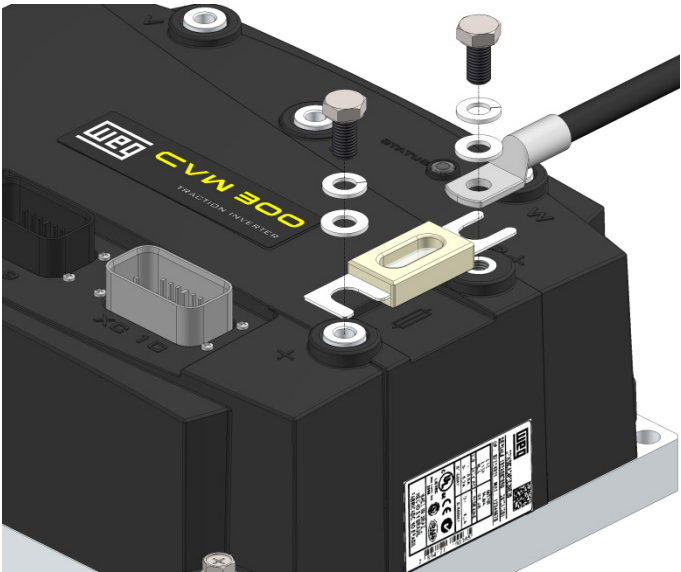
Figura 3.5: Detalhe da conexão do fusível
