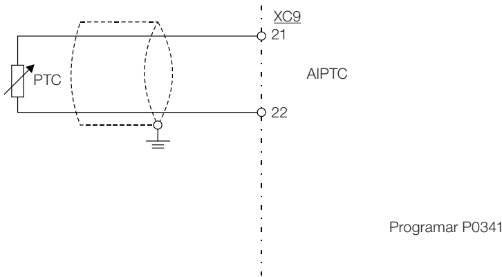
Figura 13.1: Exemplo de conexão do AIPTC
