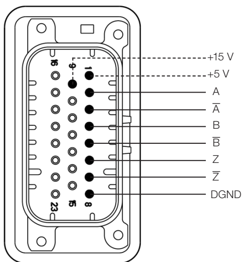
Figura 3.25: Conexões para encoder tipo linedrive ou push-pull
