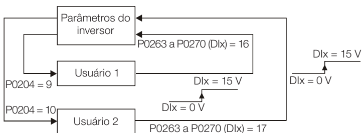
Figura 12.10: Detalhes sobre o funcionamento da função Carrega Usuário 1 ou 2
