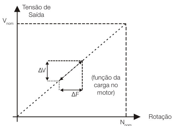
Figura 10.6: Curva V/f com compensação de escorregamento
