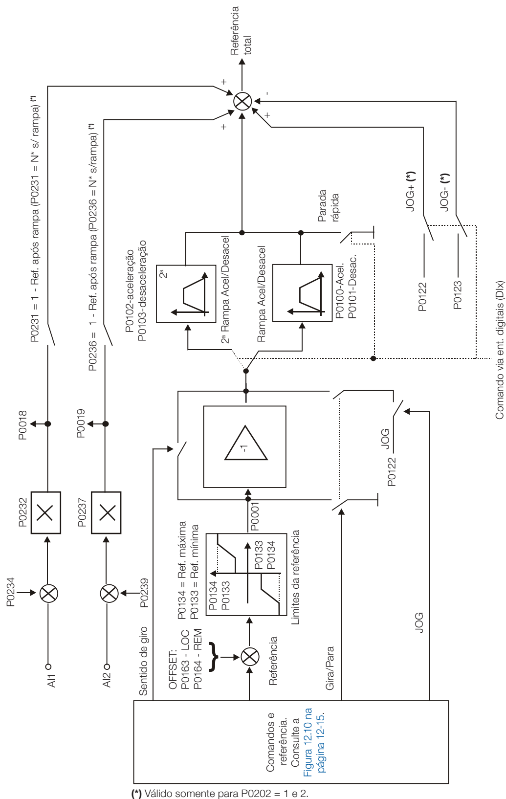
Figura 12.13: Blocodiagrama da referência de velocidade
