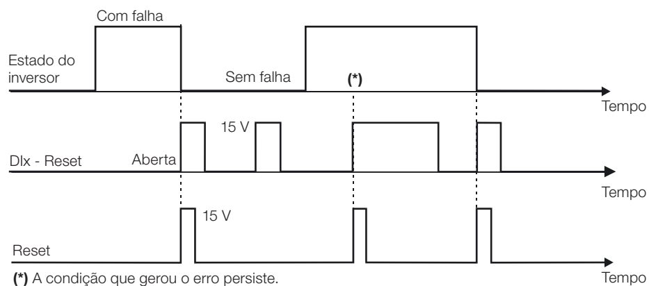
Figura 12.11: (a) a (j) Detalhes sobre funcionamento das funções das entradas digitais
