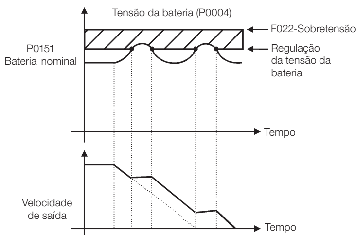
Figura 10.10: Gráfico exemplo de atuação da limitação da tensão da bateria com a função Hold de Rampa
