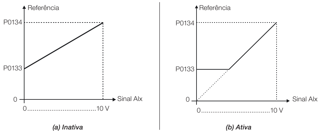
Figura 12.1: (a) e (b) Atuação das Entradas Analógicas com Zona Morta
