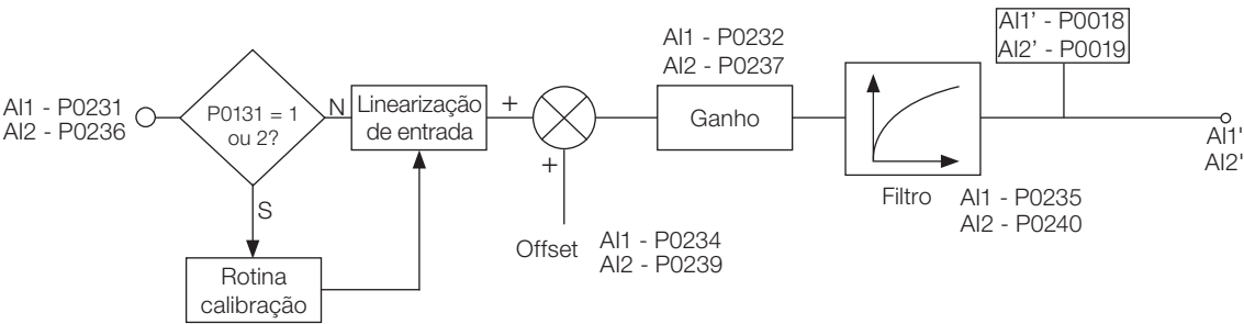
Figura 12.8: Blocodiagrama da entrada analógica AI1 (acelerador) e entrada analógica AI2
