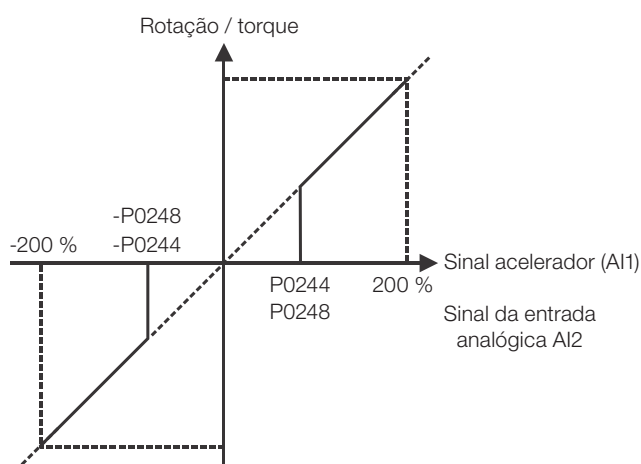
Figura 12.3: Percentual de zona morta em AI1 ou AI2
