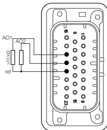
Figura 3.17: Saídas analógicas, disponíveis em XC10
