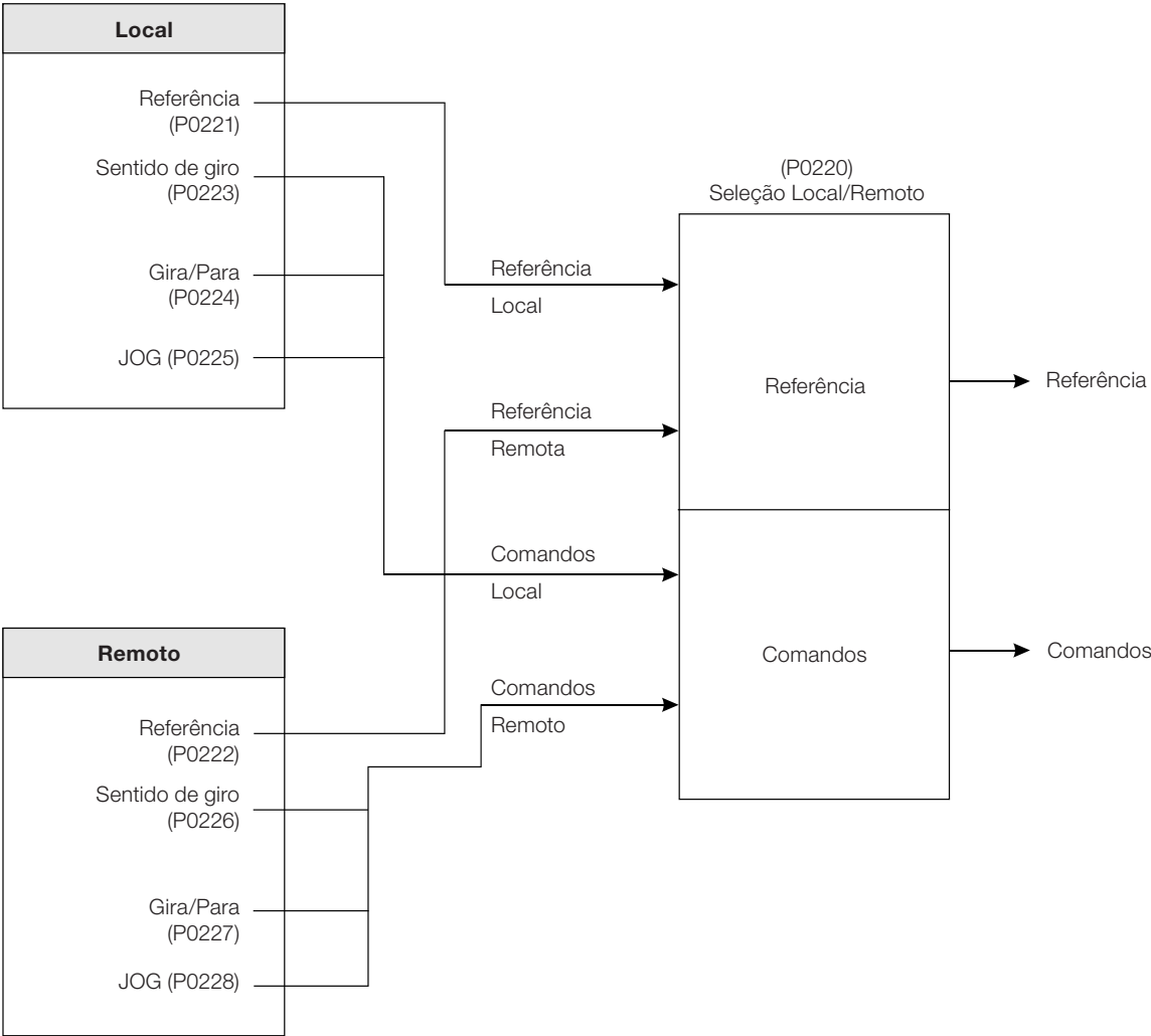
Figura 12.14: Blocodigrama situação Local/Remoto
