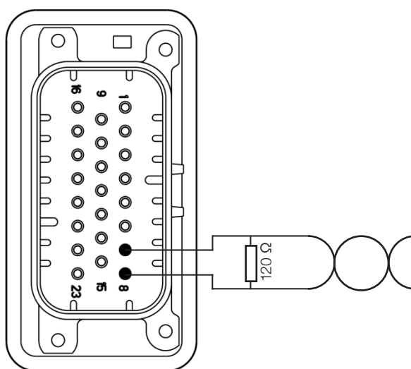
Figura 3.19: Conexão recomendada da CAN, disponível em XC9
