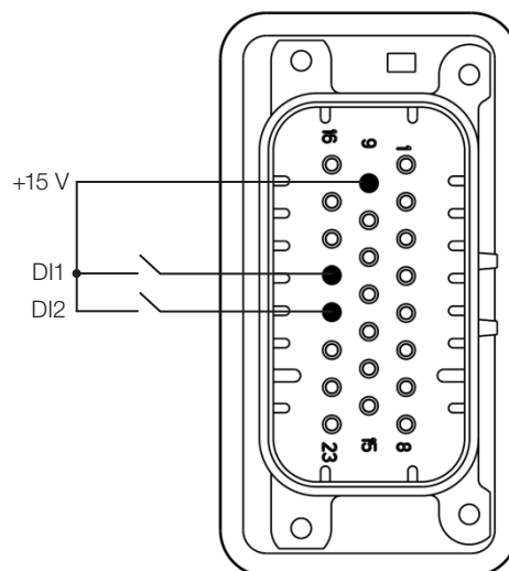
Figura 3.9: Conexões das entradas analógicas em XC10
