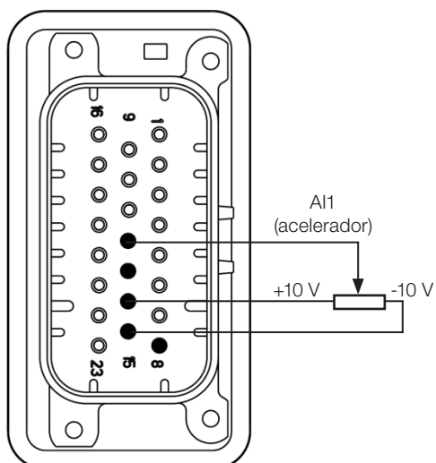
Figura 3.12: Conexão do acelerador (-10...10 V) - tipo wig-wag, em XC10
