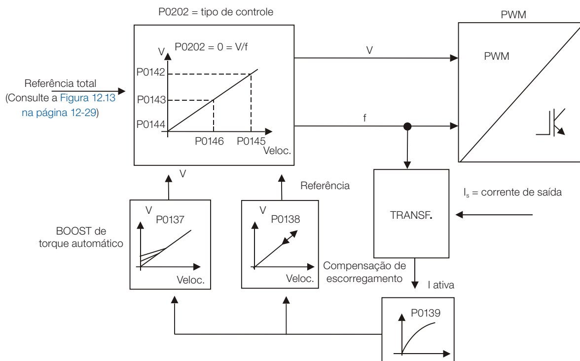
Figura 10.1: Blocodiagrama controle V/f
