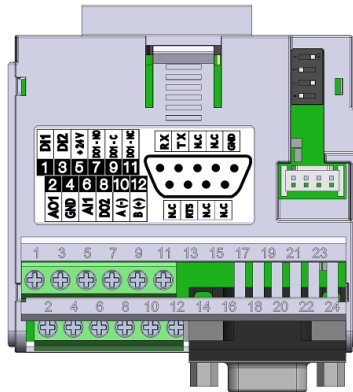
Figura 2.4: Módulo plug-in con conexión RS232
