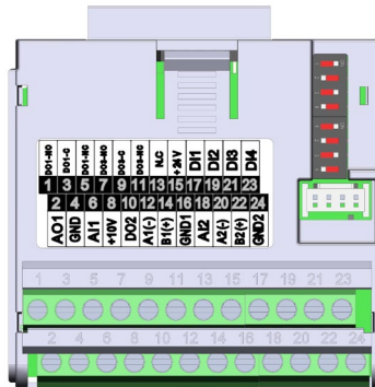
Figura 2.2: Módulo plug-in con RS485 adicional
