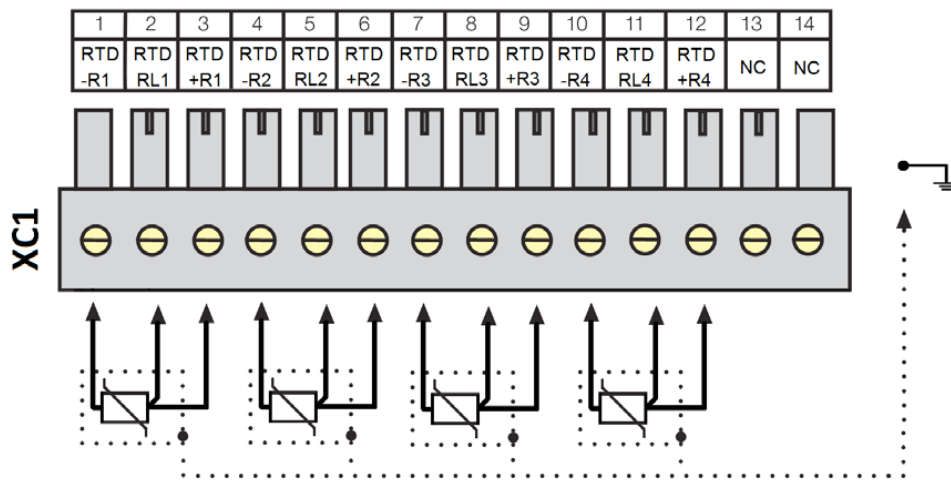
Figura 1.4: Esquema de ligação dos RTDs
