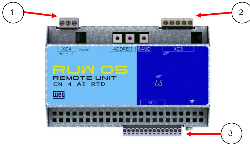
Figura 1.2: Conexões da RUW05
