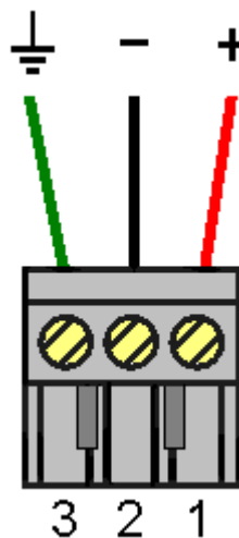
Figura 1.3: Conector de alimentação da remotaRUW05
