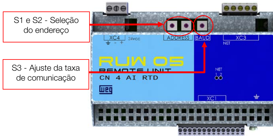
Figura 5.1: Chaves hexadecimal para configuração da RUW05
