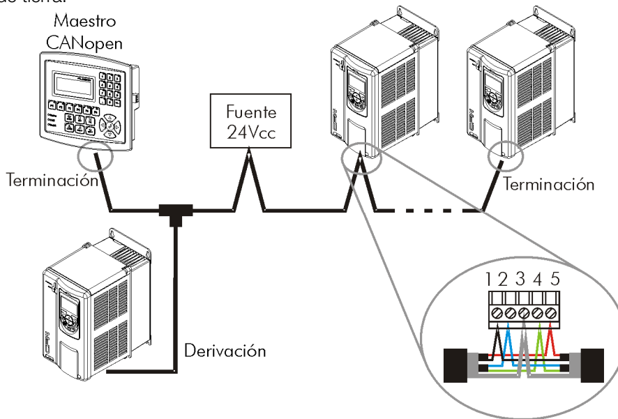
Figura 3.2: Ejemplo de instalación en red CANopen
