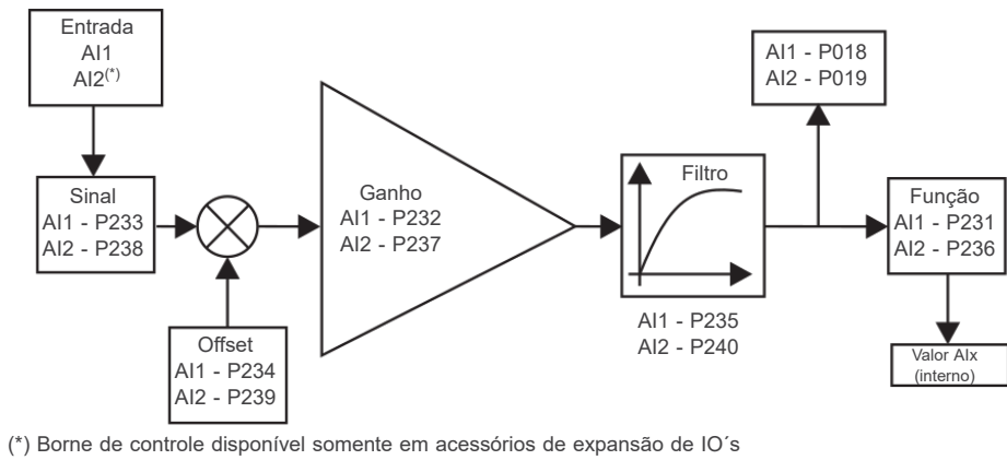
Figura 9.1: Diagrama de blocos das entradas analógicas (Alx)
