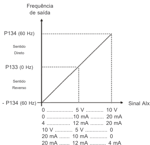
Figura 15.4: Resultado para aplicação 3
