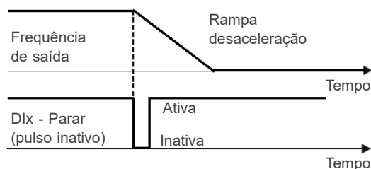
Figura 9.18: Exemplo da função Parar com pulso inativo
