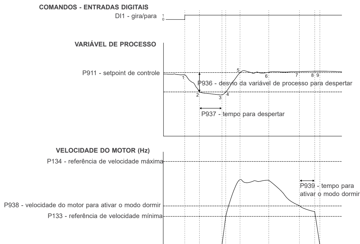
Figura 14.4: Funcionamento do controlador PID com modo dormir habilitado
