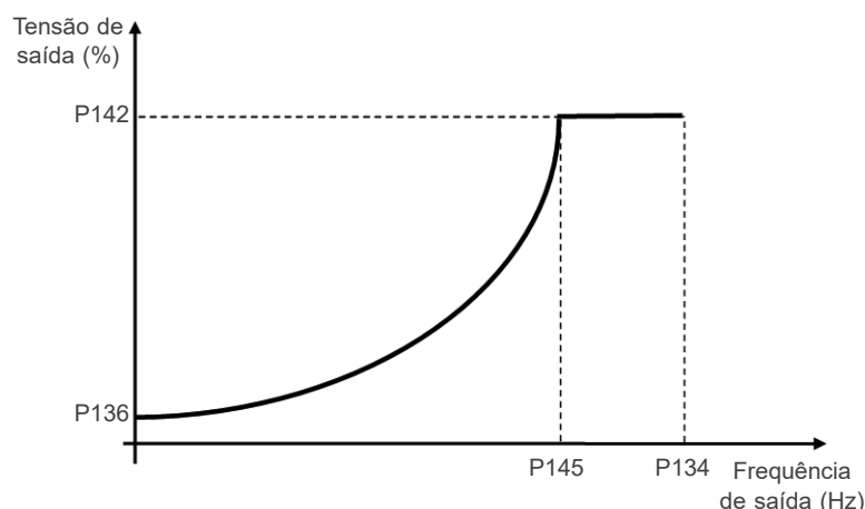
Figura 8.14: Curva V/f Quadrática
