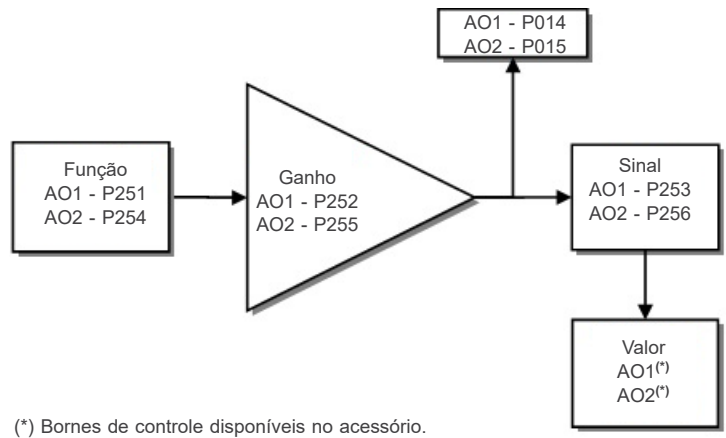
Figura 9.4: Diagrama de blocos da saída analógica (AOx)
