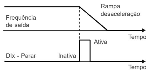
Figura 9.17: Exemplo da função Parar
