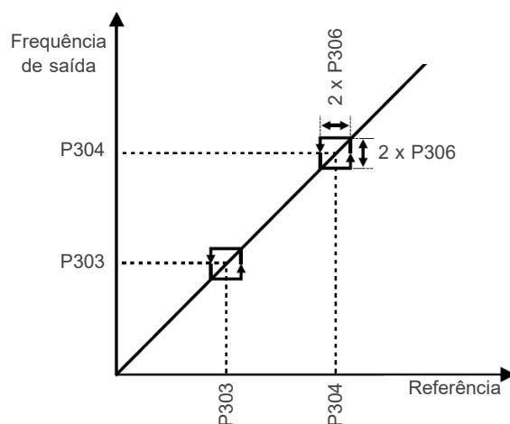
Figura 8.11: Atuação da frequência evitada
