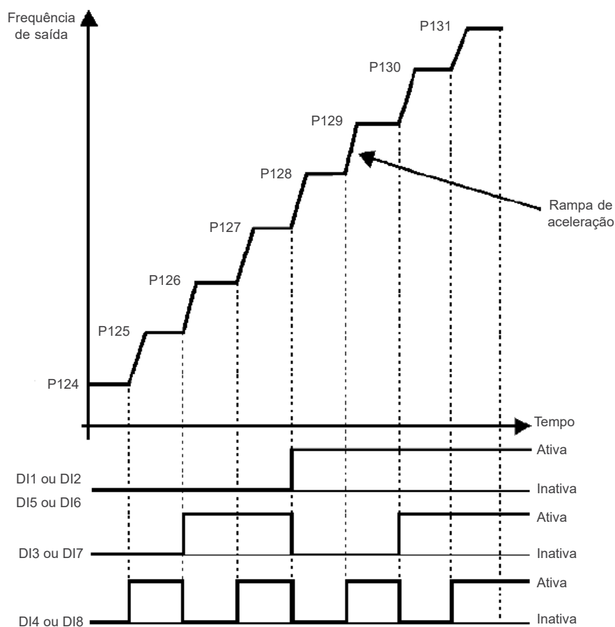
Figura 7.3: Gráfico de funcionamento da função Multispeed
