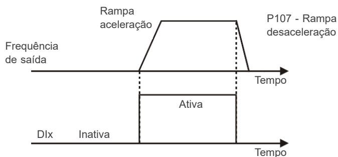
Figura 9.8: Exemplo da função Parada Rápida
