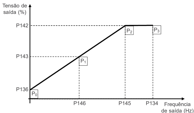
Figura 8.13: Curva V/f
