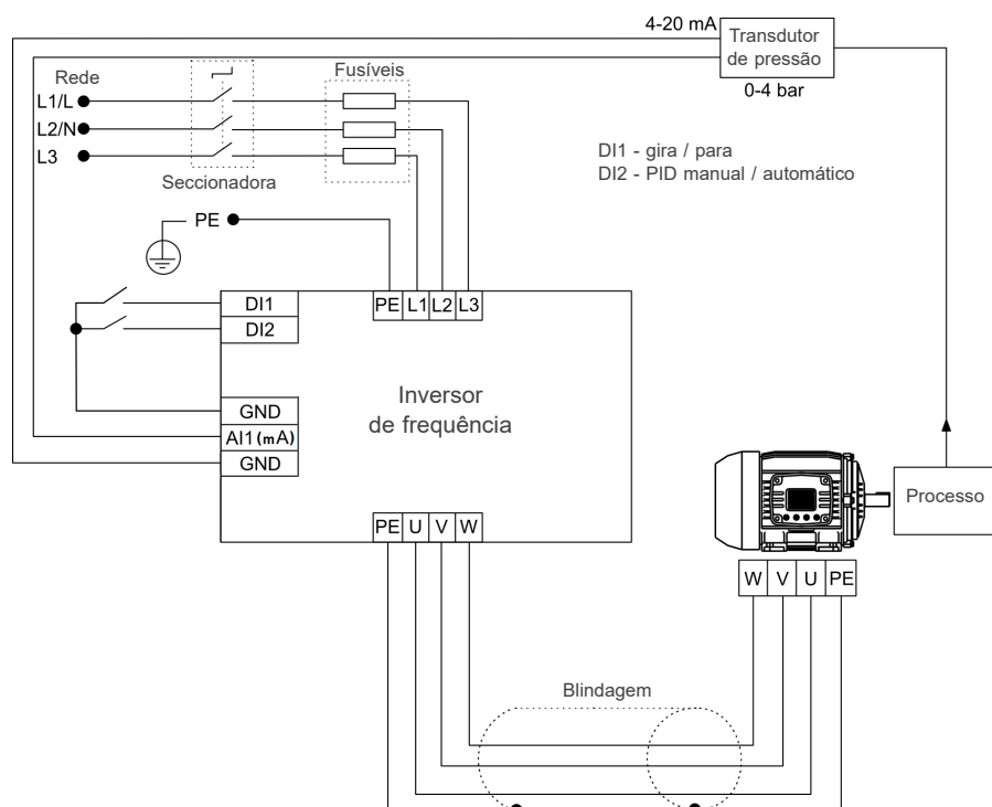
Figura 14.2: Exemplo da aplicação controlador PID
