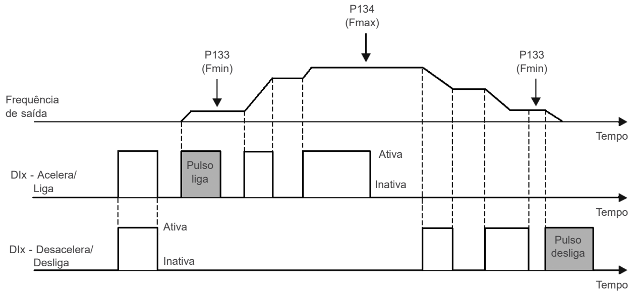
Figura 9.16: Exemplo da função Acelera-Liga / Desacelera-Desliga
