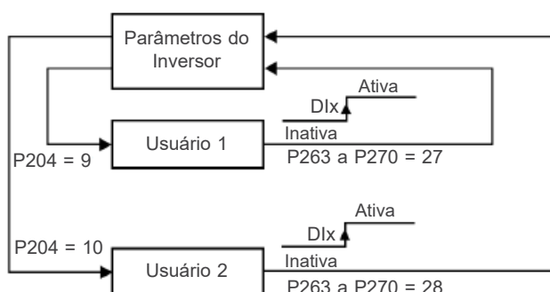
Figura 9.15: Diagrama de blocos das funções carga usuário 1 e usuário 2
