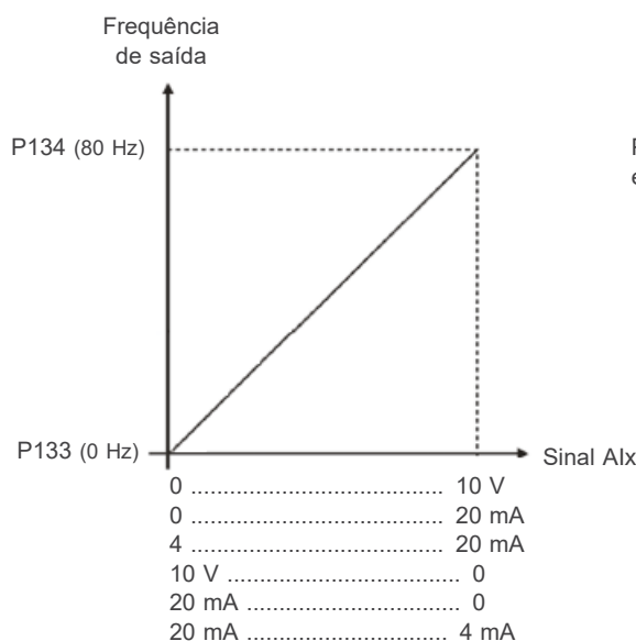
Figura 15.3: Resultado para aplicação 2
