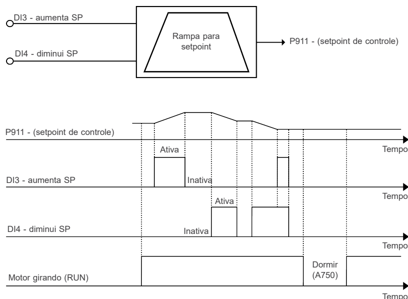
Figura 14.3: Gráfico de funcionamento da função E.P.
