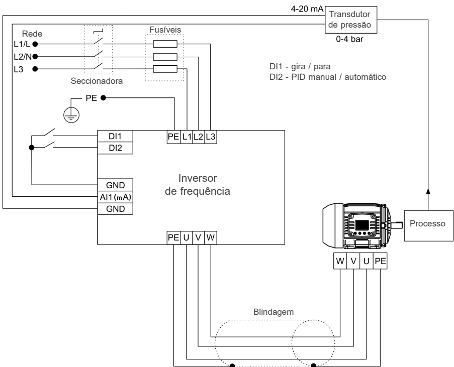
Figura 15.7: Exemplo de aplicação com controlador PID
