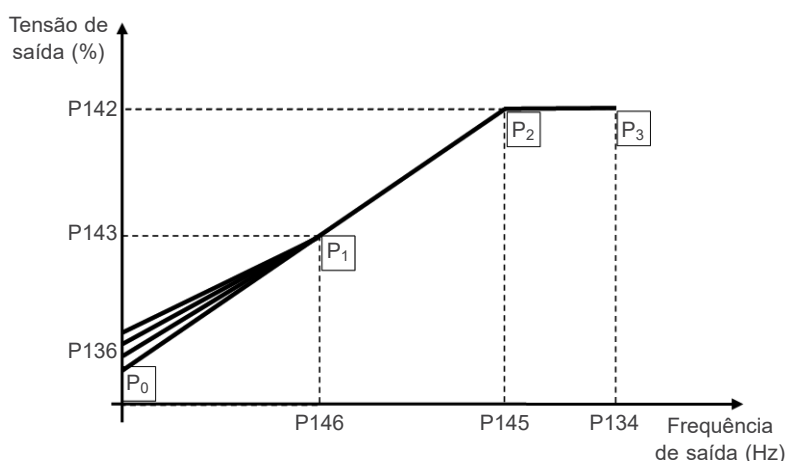
Figura 8.15: Região do boost de torque para modo de controle V/f
