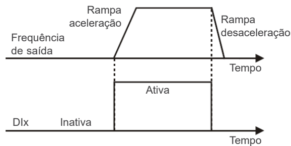
Figura 9.6: Exemplo da função Gira/Para
