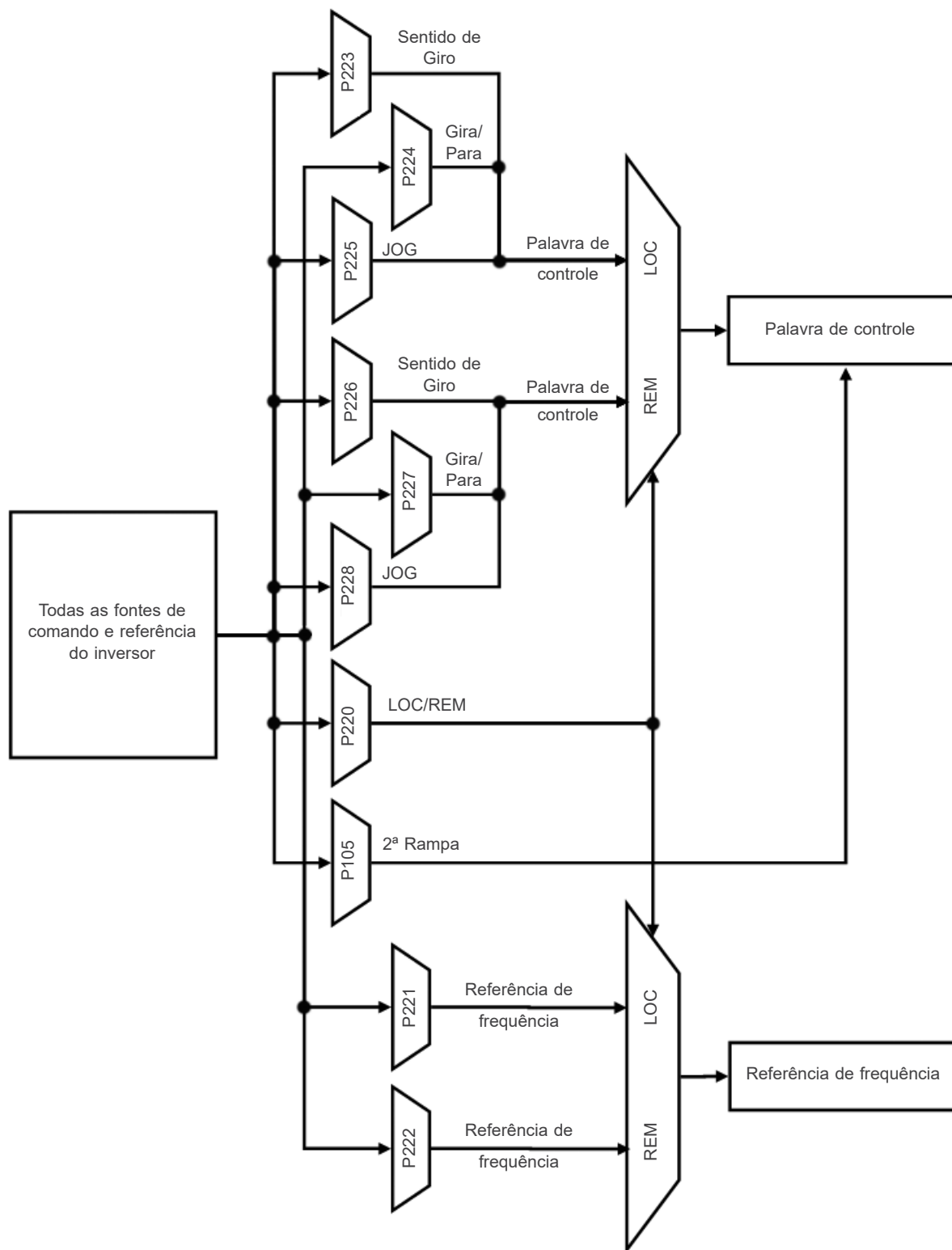
Figura 7.1: Blocodograma para comandos e referências
