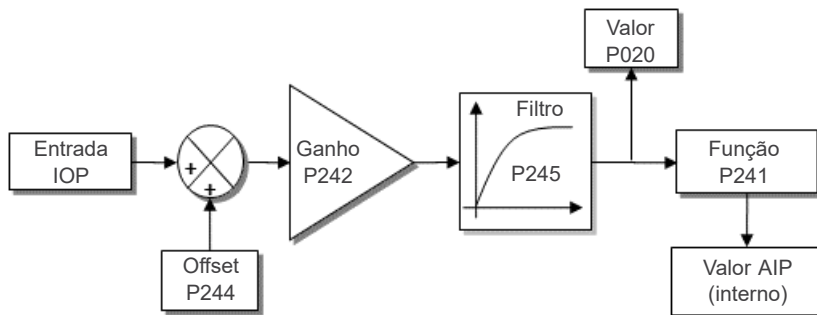
Figura 9.3: Diagrama de blocos da entrada sinal potenciômetro AIP
