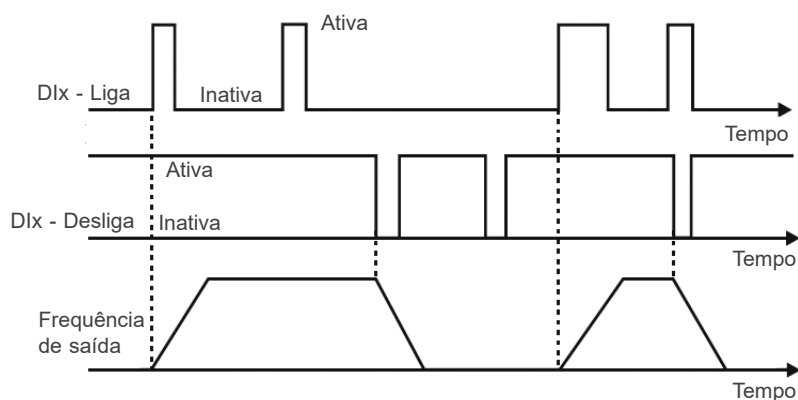
Figura 9.10: Exemplo da função Liga/Desliga
