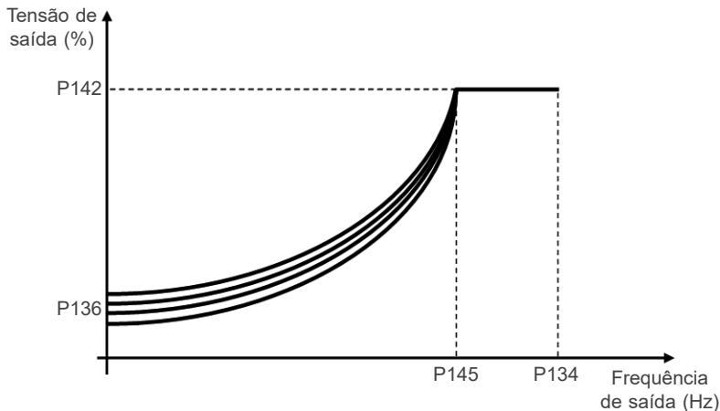
Figura 8.16: Região do boost de torque para modo de controle V/f Quadrático
