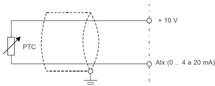
Figura 10.1: Conexão do PTC ao inversor de frequência
