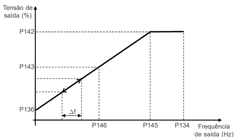
Figura 8.18: Compensação de escorregamento em um ponto de operação da curva V/f
