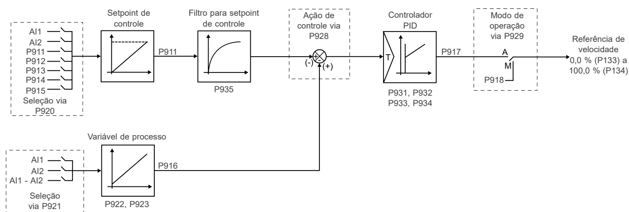
Figura 14.1: Blocodiagrama do controlador PID
