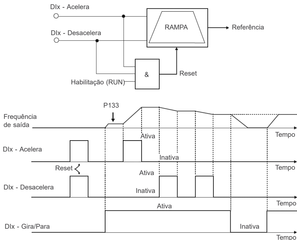
Figura 9.13: Exemplo da função Potenciômetro Eletrônico (E.P.)
