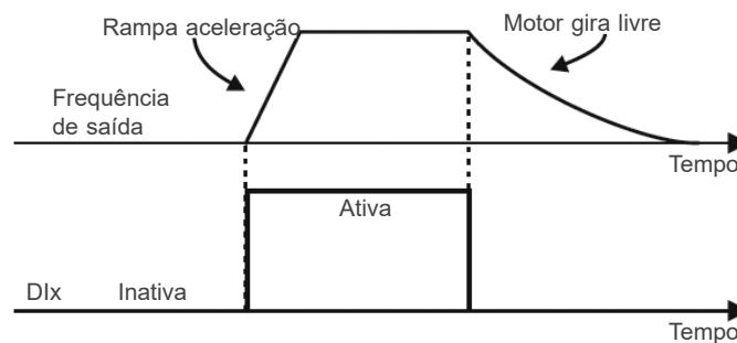
Figura 9.7: Exemplo da função Habilita Geral
