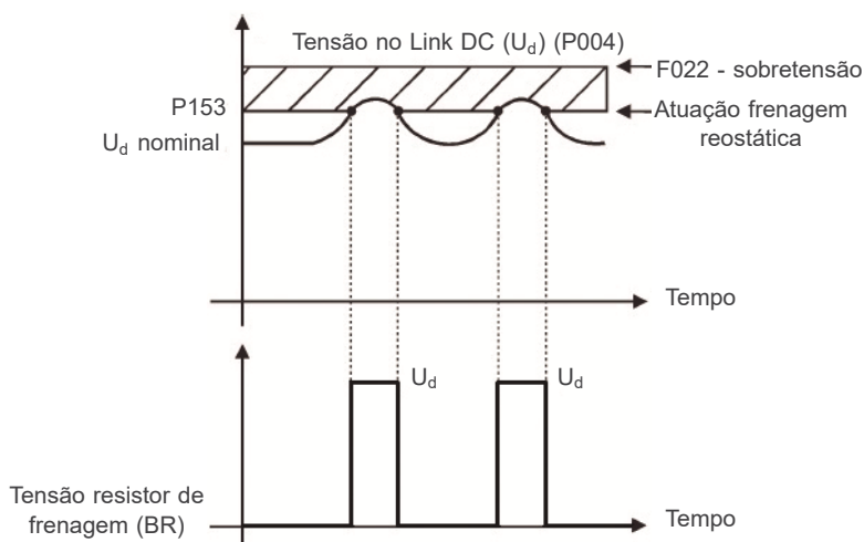
Figura 8.10: Curva de atuação da frenagem reostática
