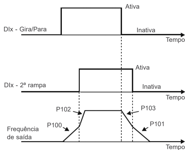
Figura 9.14: Exemplo da função 2ª Rampa
