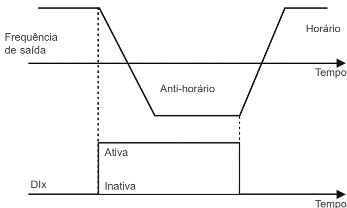
Figura 9.11: Exemplo da função Sentido de Giro
