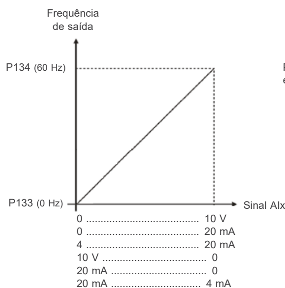
Figura 15.2: Resultado para aplicação 1
