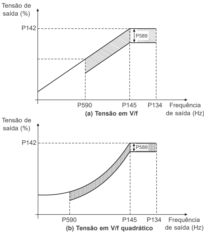
Figura 8.19: (a) e (b) Exemplo de comportamento da tensão em V/f e V/f quadrático
