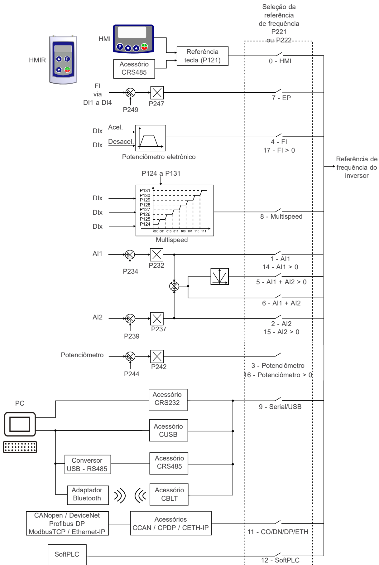
Figura 7.2: Estrutura de seleção da referência de frequência
