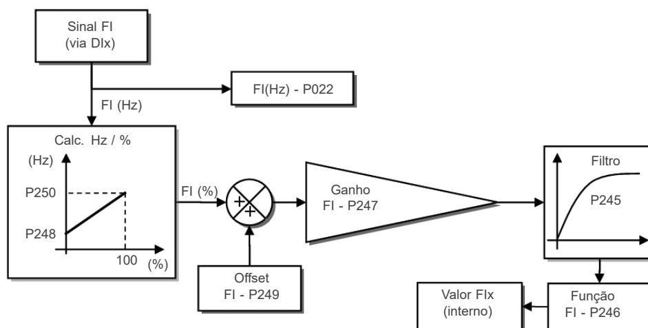
Figura 9.5: Diagrama de blocos da entrada em frequência - FI (Dlx)
