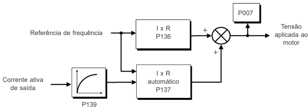
Figura 8.17: Blocodiagrama do boost de torque automático
