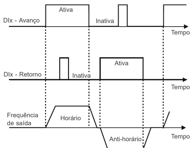
Figura 9.9: Exemplo da função Avanço/Retorno
