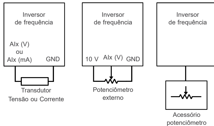
Figura 15.1: Conexões genéricas para entradas analógicas
