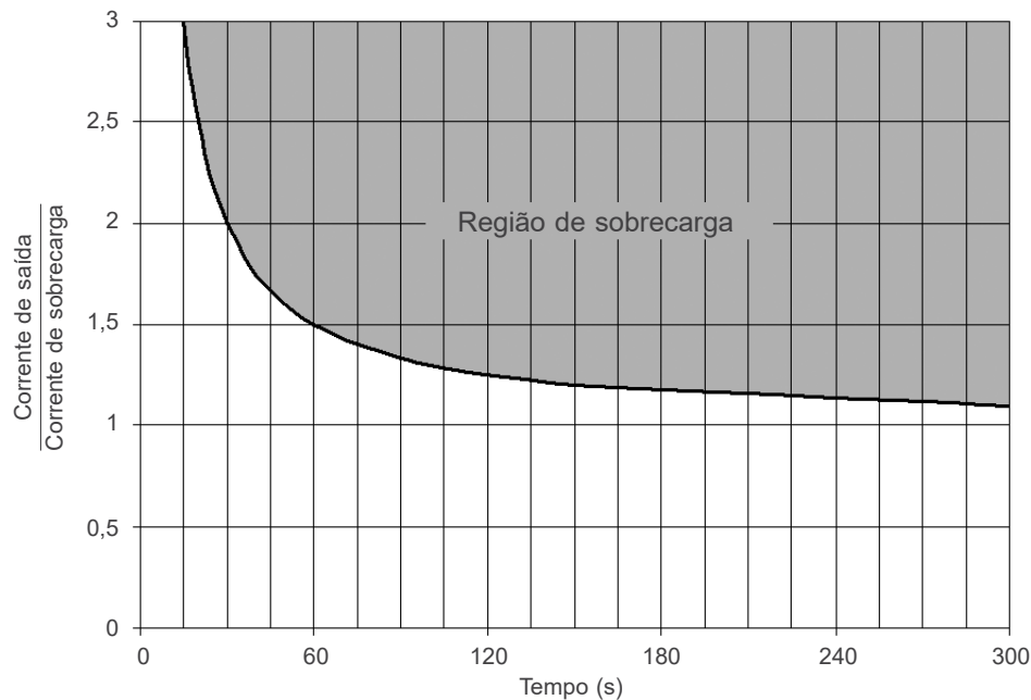
Figura 10.2: Atuação da sobrecarga do motor
