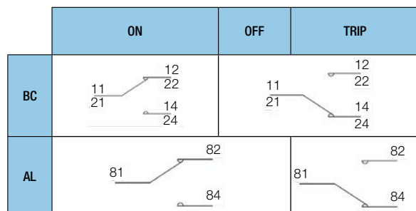
Diagrama Esquemático dos Blocos de Contatos BC e AL (Disjuntores DWB)
