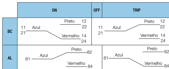
Diagrama Esquemático dos Blocos de Contatos BC e AL (Disjuntores DWA1600)
