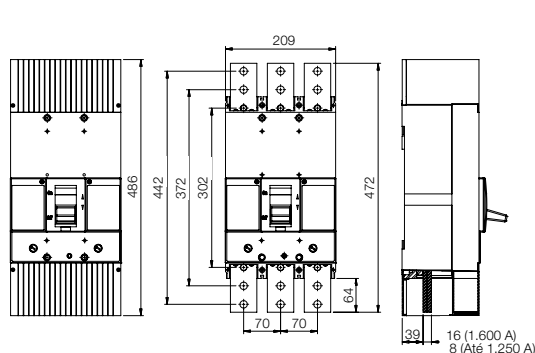
Mecânica 1600 3P + BE DWA1600
