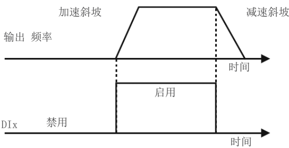
图 14.6: 启动/停止功能示例
