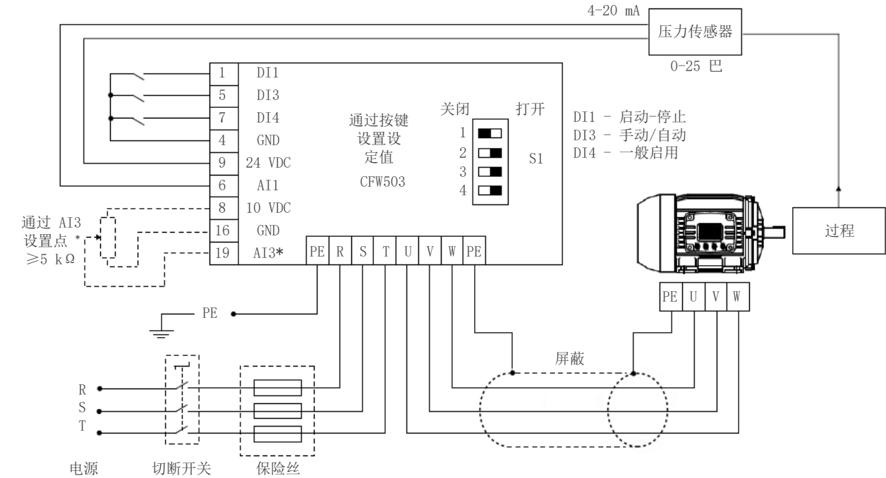
图 15.2: CFW503 PID控制器的应用示例
