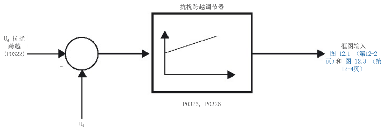
图 13.5: 抗扰跨越PI控制器
