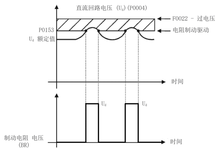
图 16.1：变阻制动的动作曲线
