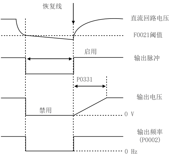
图 13.2: 执行抗扰跨越功能
