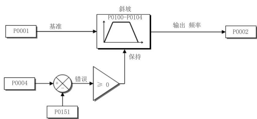
图 9.6: DC Link限压框图 - 斜坡保持
