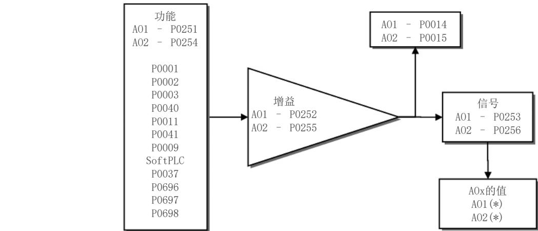
图 14.3：模拟输出出口的框图 - AOx
