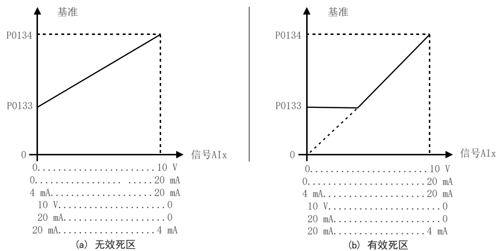
图 14.1: (a) 和 (b) - 带无效死区和有效死区的模拟输入
