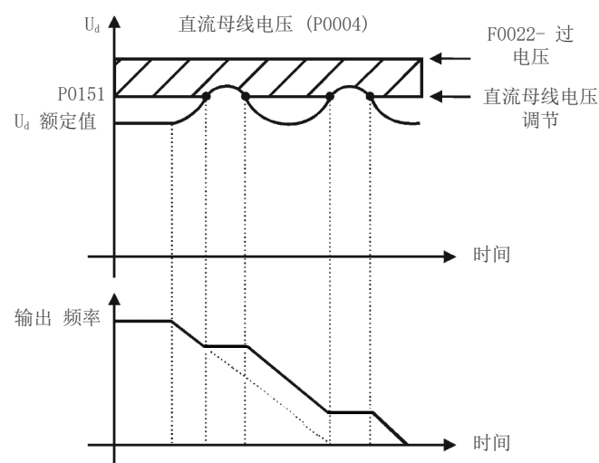
图 9.7: DC Link限压示例图 - 斜坡保持
