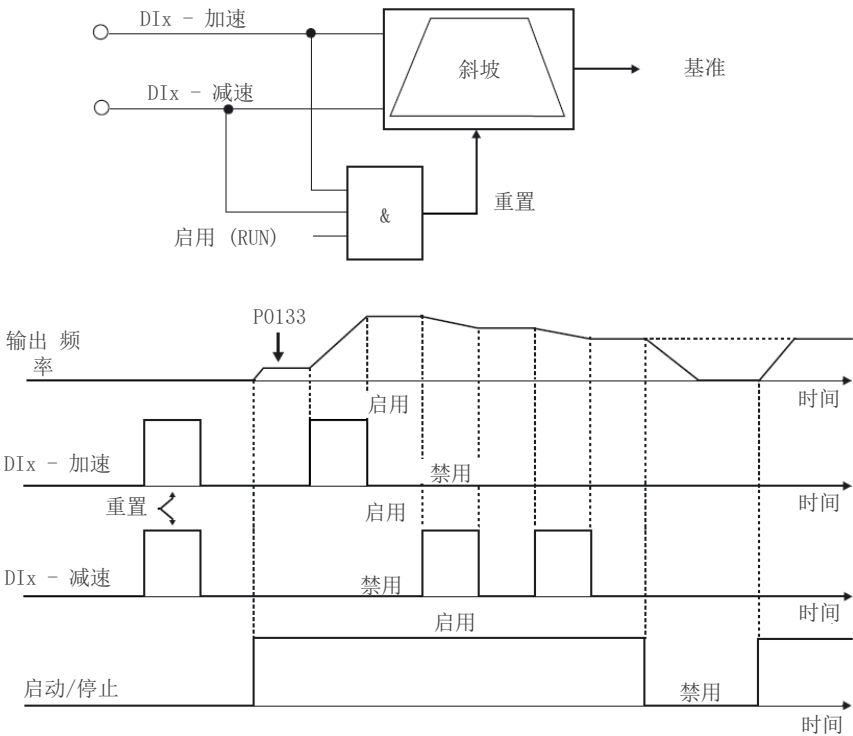
图 7.5: 电子电位计功能的工作图
