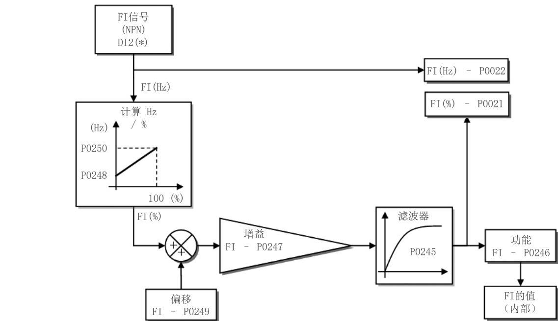
图 14.4: 频率输入框图 - FI (DI2)
