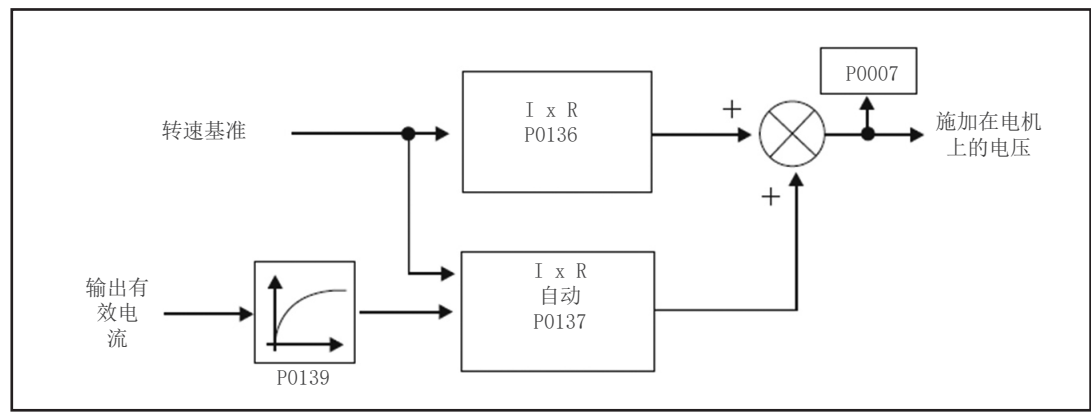
图 9.4: 自动转矩提升的框图
