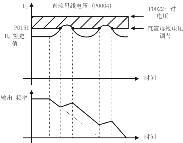
图 9.9: DC Link限压示例图 - 加速斜坡
