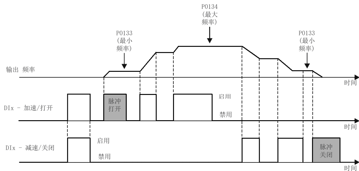
图 14.16: 打开加速/关闭减速的示例
