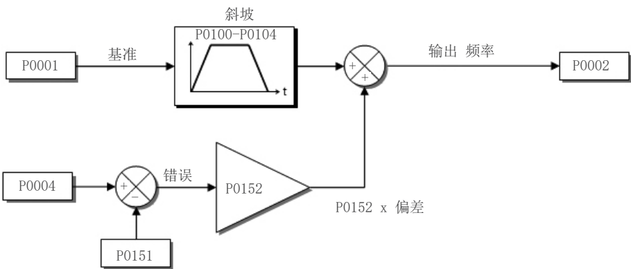
图 9.8: DC Link限压框图 - 加速斜坡
