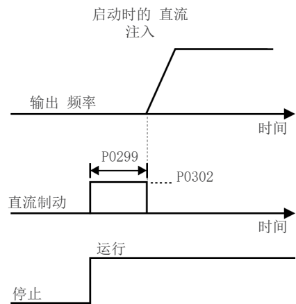
图 13.6: 启动时的直流动作
