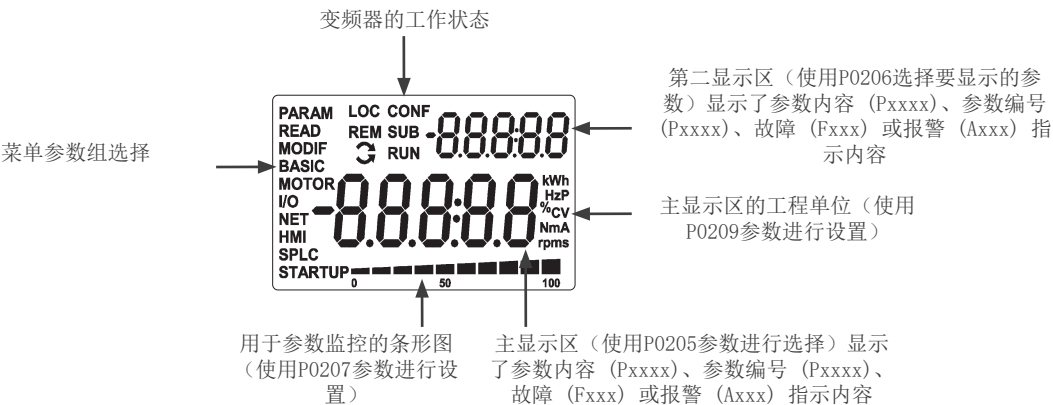
图 5.1：启动屏幕和显示区域
