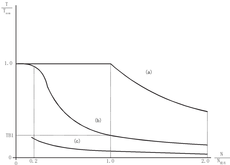
(a) 电机正常运行时输出的转矩，变频器工作于“电动机模式”（负荷转矩） (b) 使用最佳制动时产生的制动转矩 (c) 使用直流制动时产生的制动转矩
