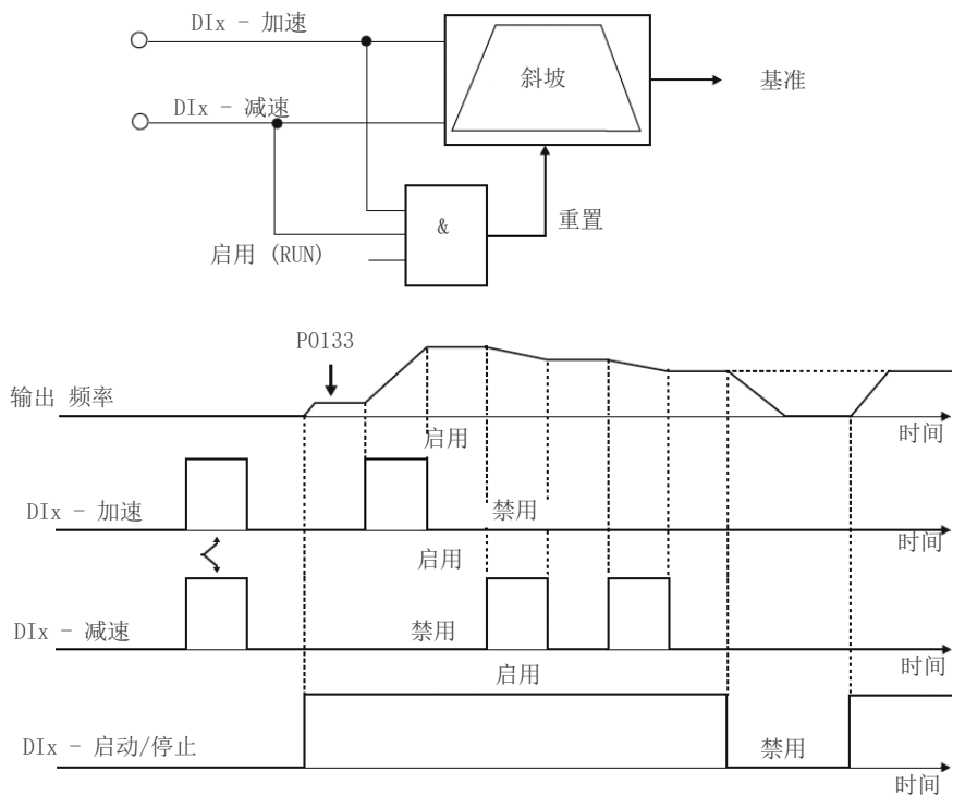
图 14.13：电子电位计功能示例
