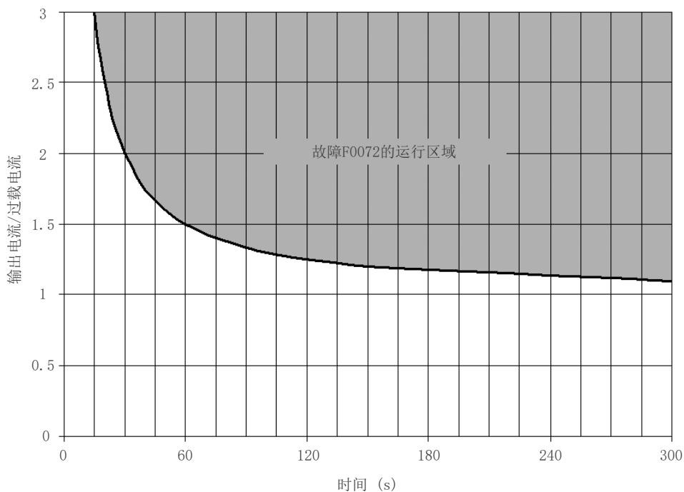
图 17.1: 电机过载动作
