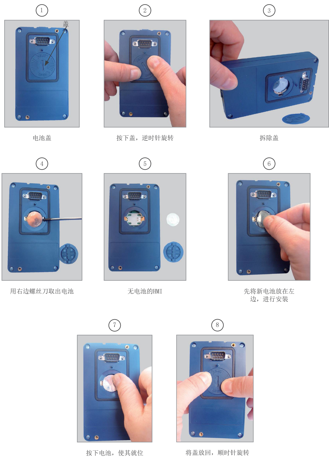
图 4.4：更换HMI电池
