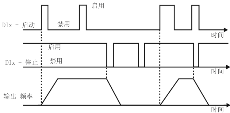
图 14.10：三线启动/停止功能示例
