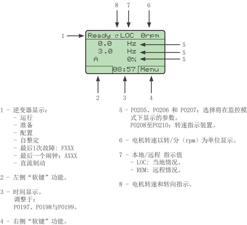
图 5.2：出厂设置时的监控模式屏幕
