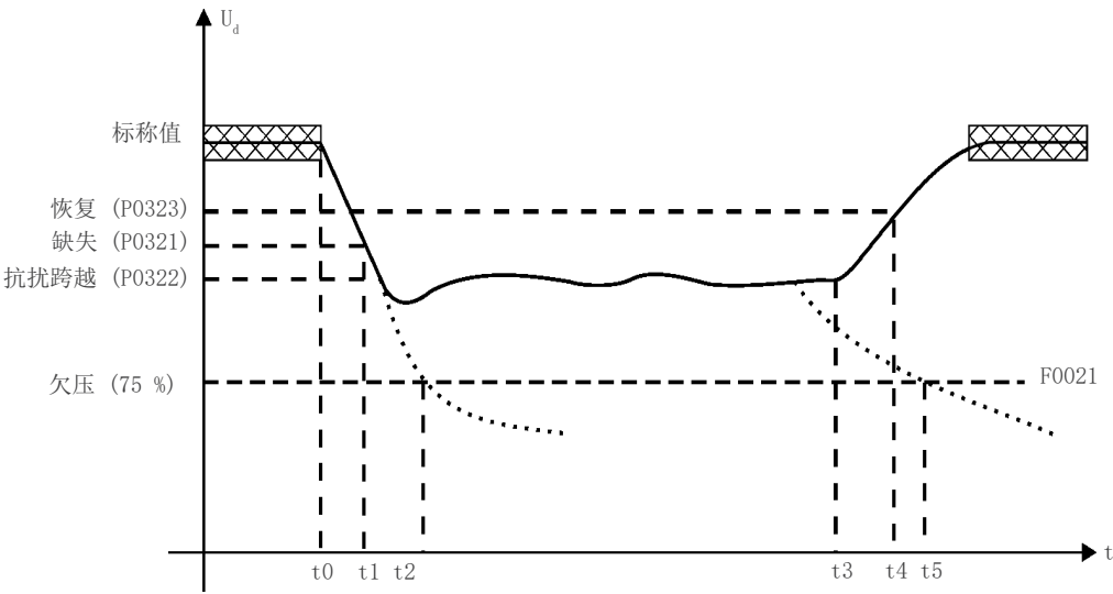
图 13.4: 矢量模式下的抗扰跨越功能
