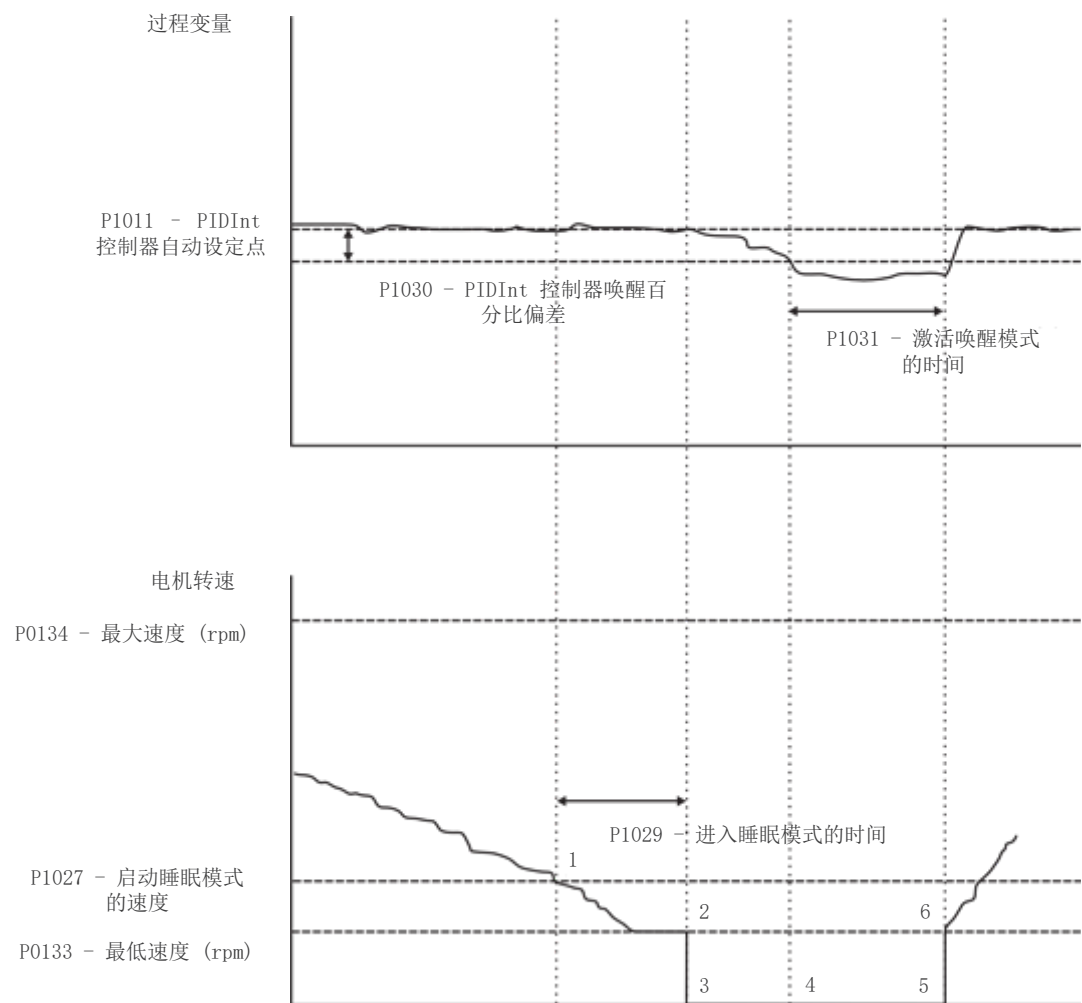
图 20.1: 睡眠和唤醒操作图
