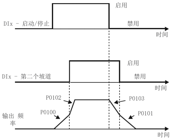
图 14.14：第二个斜坡函数的示例
