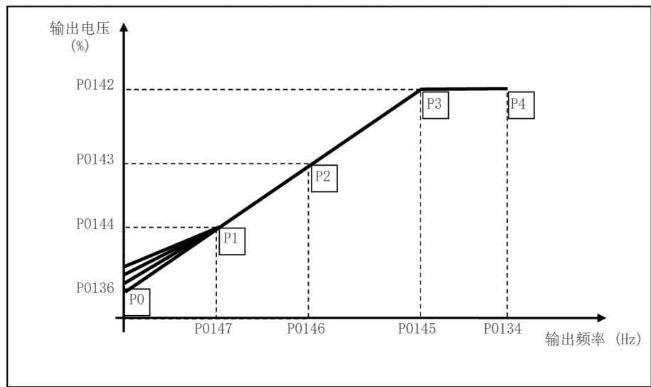
图 9.3: 转矩提升区
