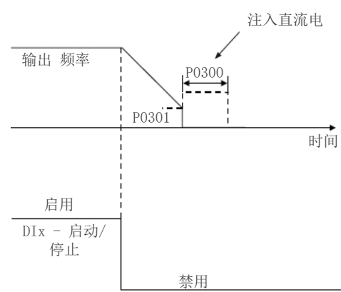
图 13.7：执行直流制动
