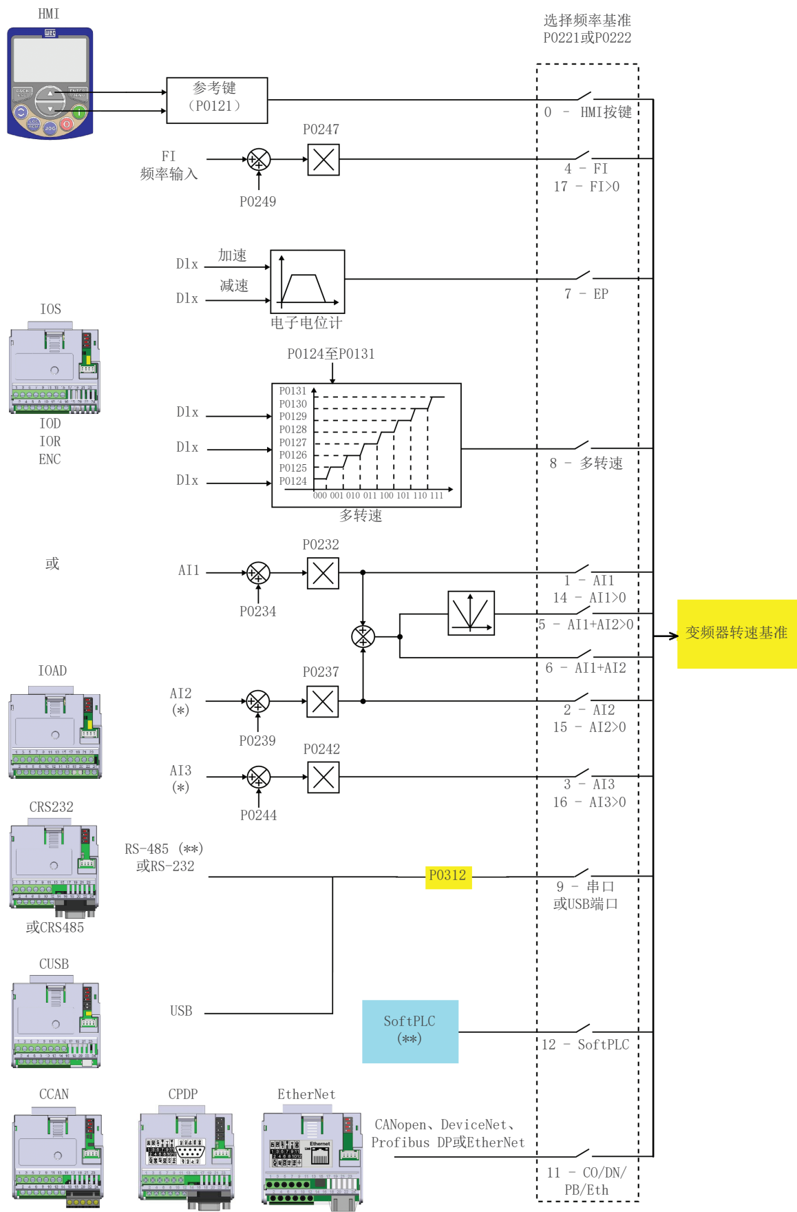
图 7.3: 选择转速基准的结构
