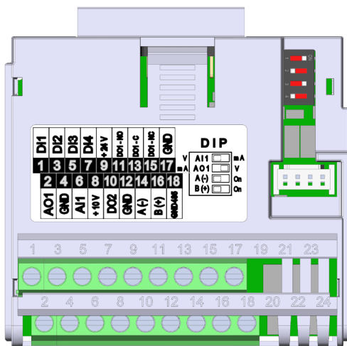
图 19.1: 插入模块CFW500-IOS
