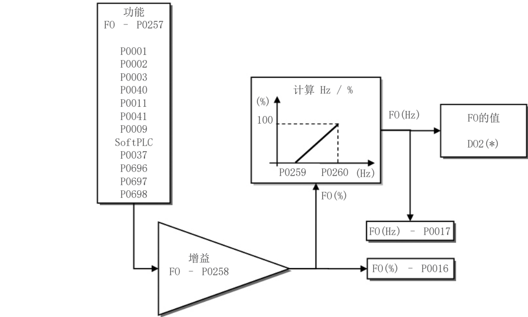
图 14.5: 频率输出F0(D02)的框图
