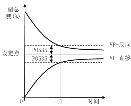
图 15.4: P0535定义的设置值确认带
