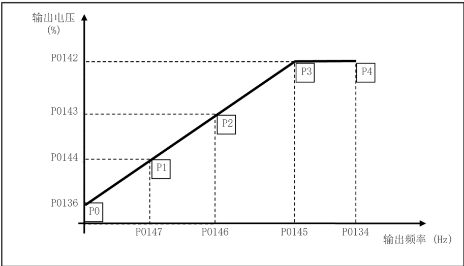
图 9.2: V/f曲线
