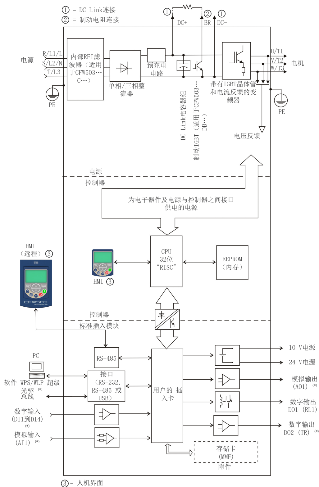
图 3.1: CFW503框图
