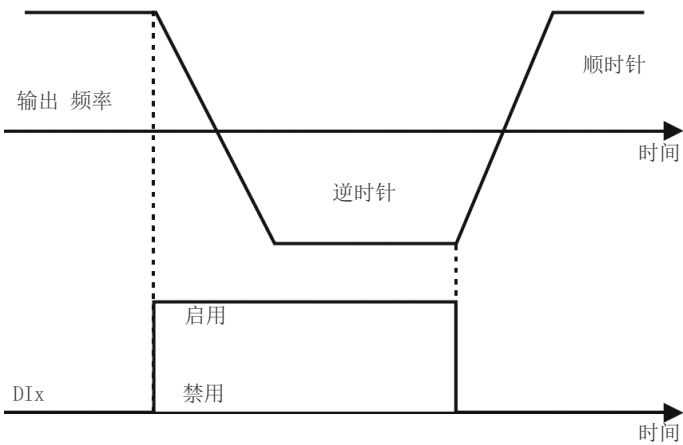
图 14.11: 旋转方向功能示例
