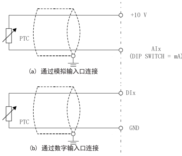
图 17.4: (a) 和 (b) - PTC与CFW503的接线
