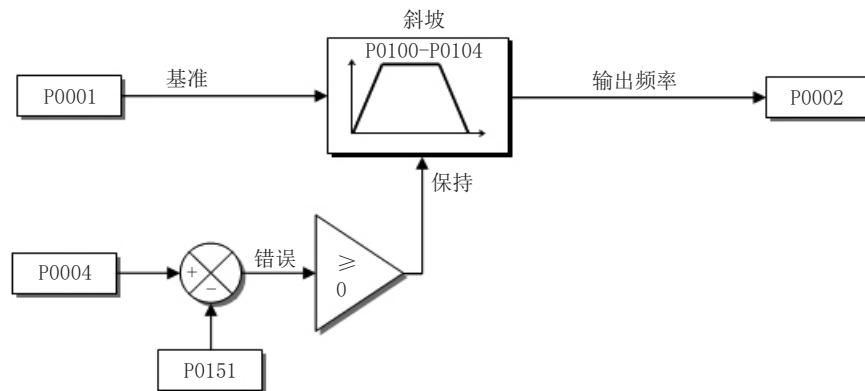
图 9.6: DC Link限压框图 - 斜坡保持
