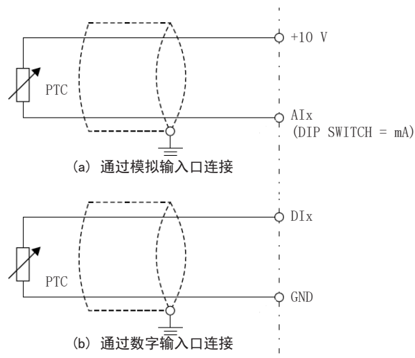
图 18.4: (a) 和 (b) - PTC与CFW500的接线
