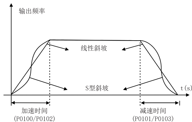
图 14.1: S或线性斜坡
