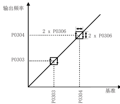
图 14.8: 执行回避频率
