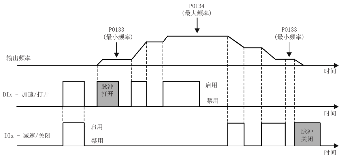
图 15.16: 打开加速/关闭减速的示例
