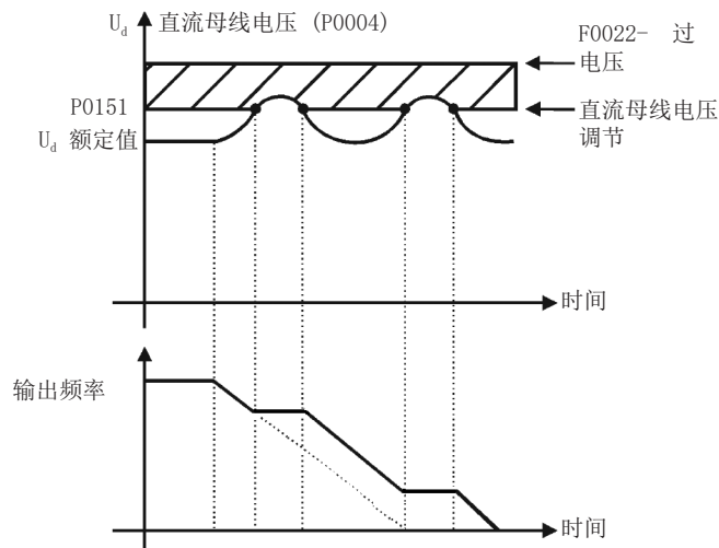
图 9.7: DC Link限压示例图 - 斜坡保持
