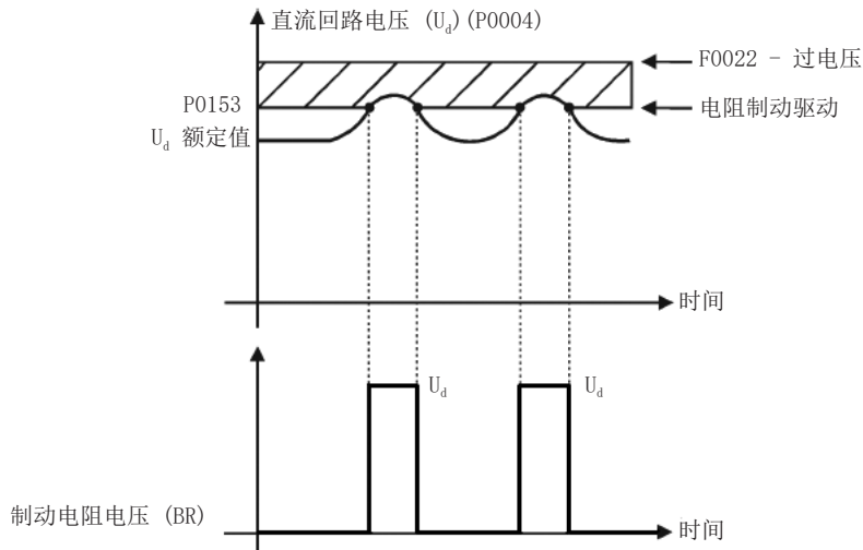
图 17.1: 变阻制动的动作曲线
