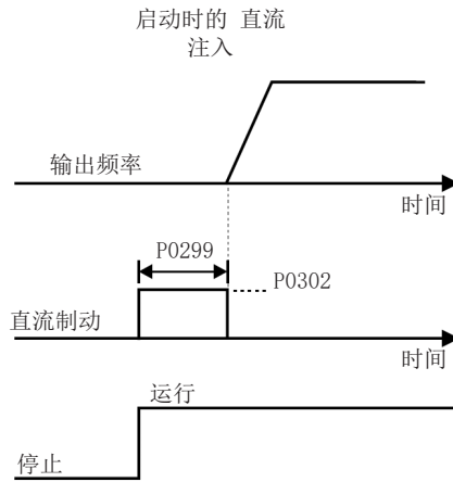
图 14.6: 启动时的直流动作
