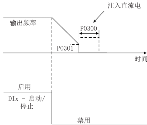
图 14.7: 执行直流制动
