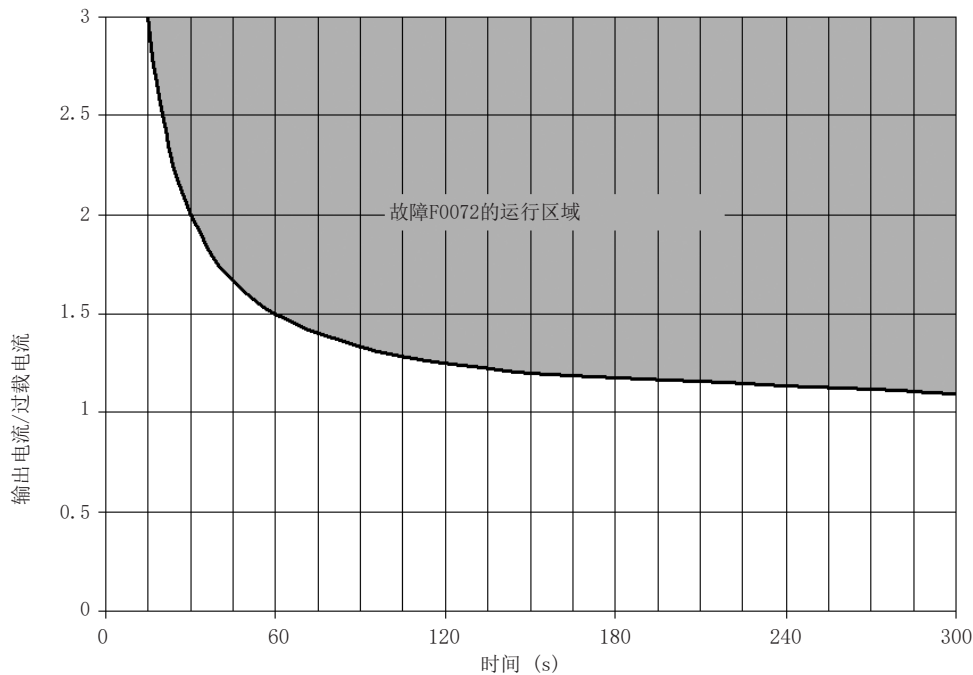
图 18.1: 电机过载动作
