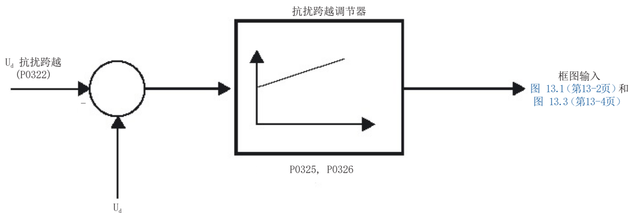
图 14.5: 抗扰跨越PI控制器
