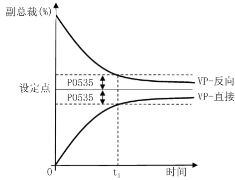
图 16.4: P0535定义的设置值确认带
