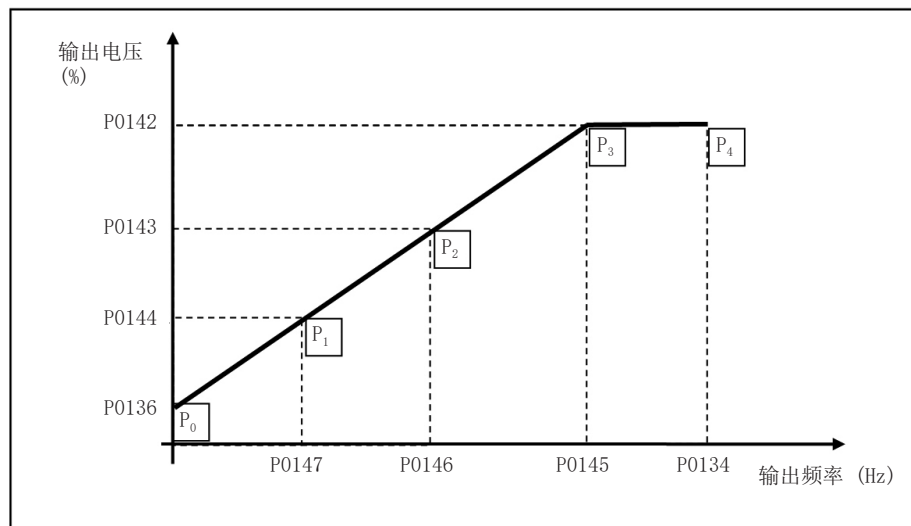
图 9.2: V/f曲线
