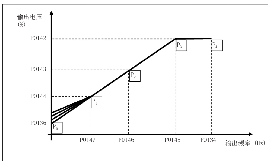
图 9.3: 转矩提升区
