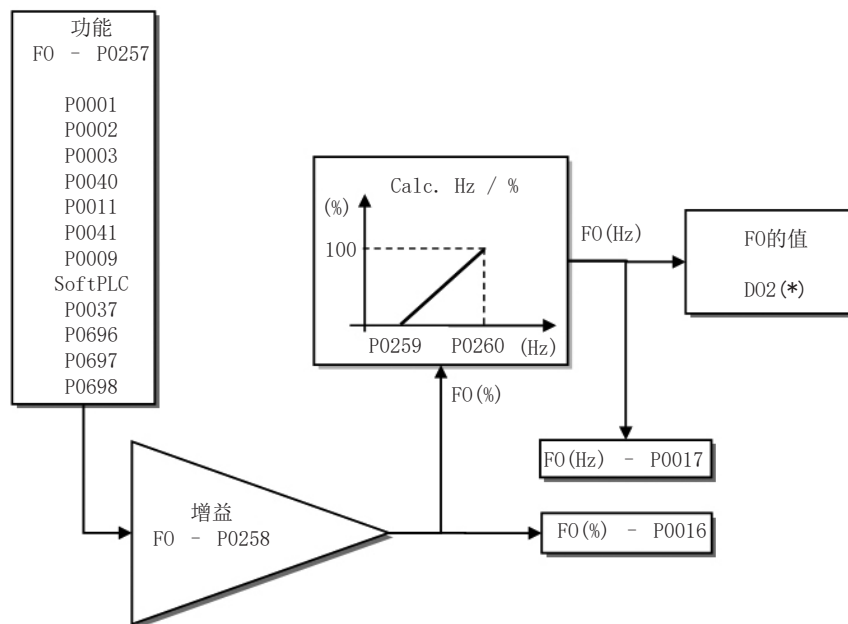
图 15.5: 频率输出FO (D02) 的框图
