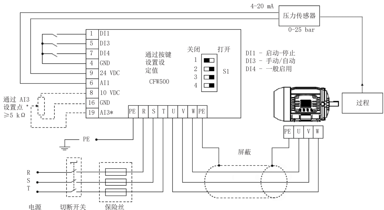
图 16.2: CFW500 PID控制器的应用示例
