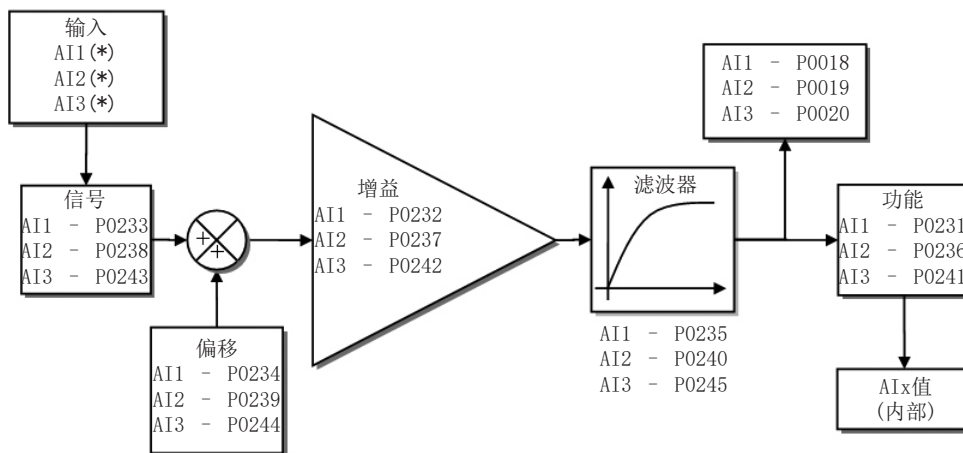
图 15.2: 模拟输入框图 - AI x
