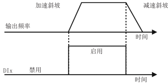
图 15.6: 启动/停止功能示例
