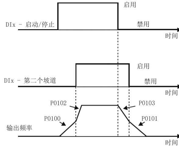
图 15.14: 第2斜坡功能示例
