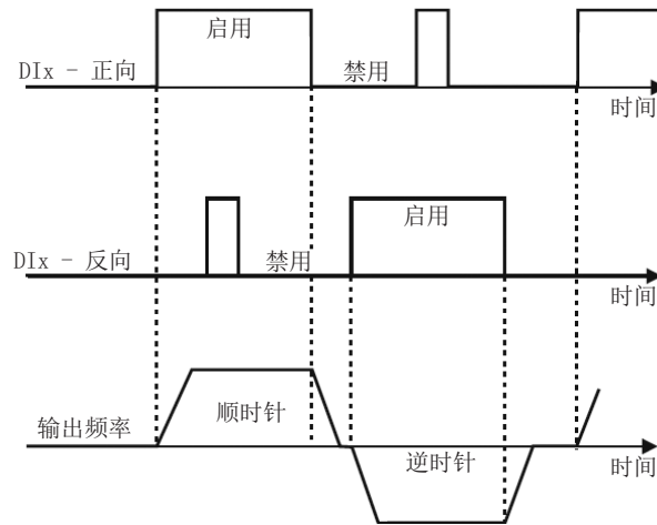
图 15.9: 正向转动/反向转动功能示例
