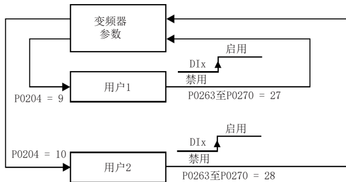
图 15.15: 用户1和用户2功能框图
