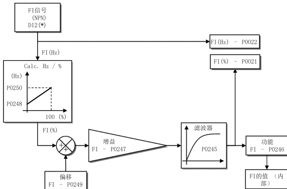
图 15.4: 频率输入框图 - FI (DI2)
