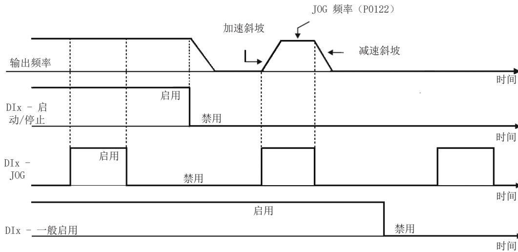
图 15.12: 点动功能示例
