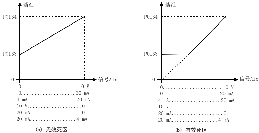
图 15.1: a) 和 (b) - 带无效死区和有效死区的模拟输入
