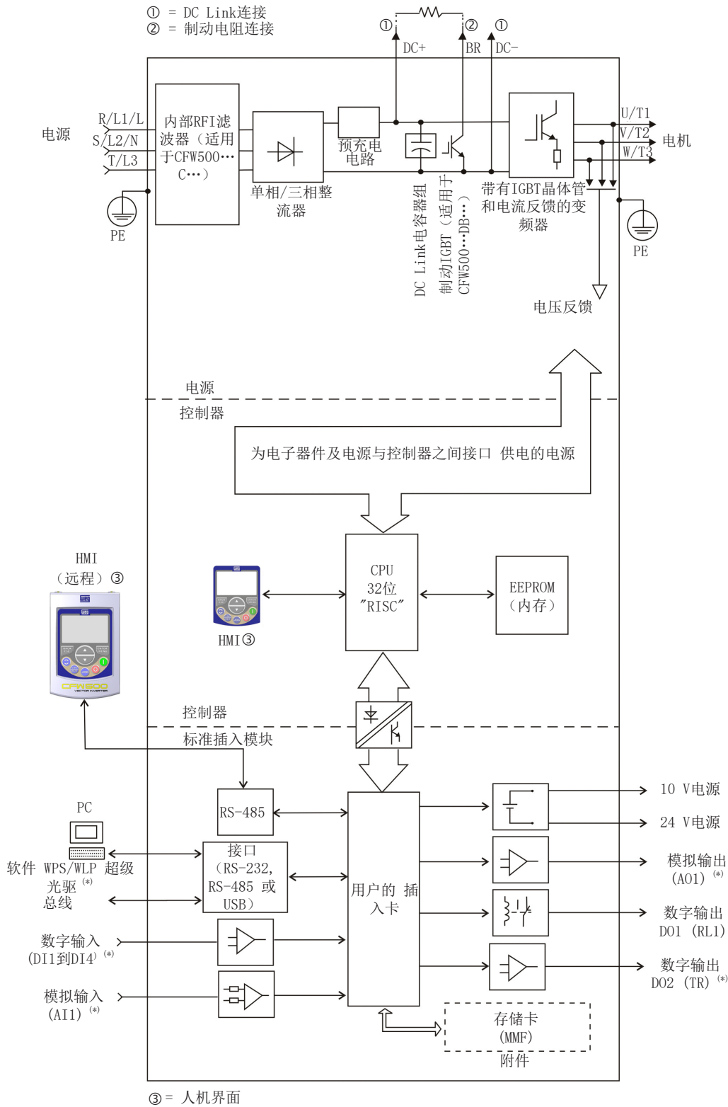
图 3.1: CFW500框图
