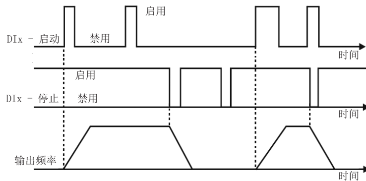
图 15.10: 三线启动/停止功能示例
